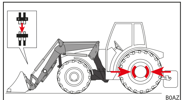
Фиг. 80 Свързване на верига за управление
