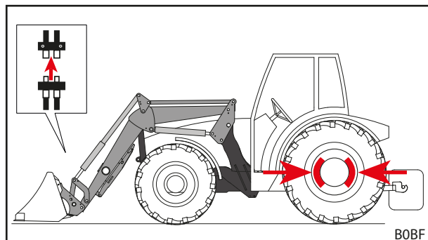
Фиг. 92 Освобождаване на хидравлични тръбопроводи
