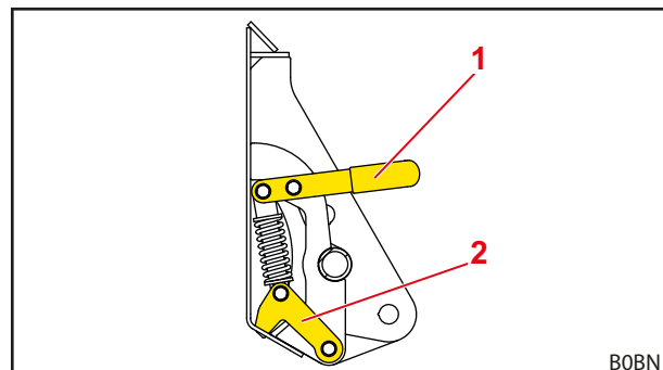
Фиг. 66 Механично заключване на инструмента Skid-Steer (отворено състояние)
