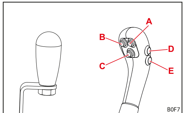
Фиг. 55 Лост за управление без бутони (вляво) и лост за управление с 5 бутона (вдясно)
