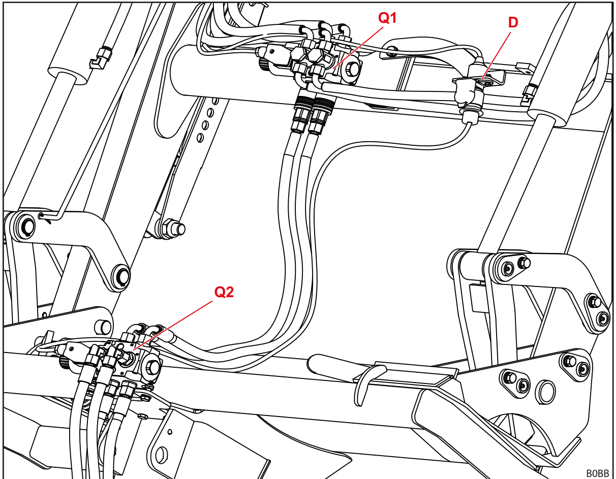
Фиг. 116 Разположение на хидравличните вентили за допълнителни функции
