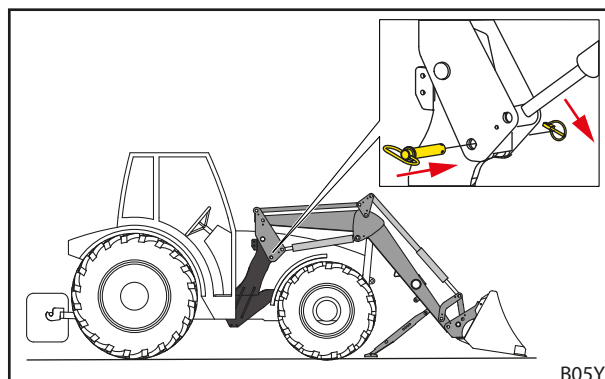
Фиг. 48 Вкарайте заключващите палци и ги подсигурете с шплинтове.
