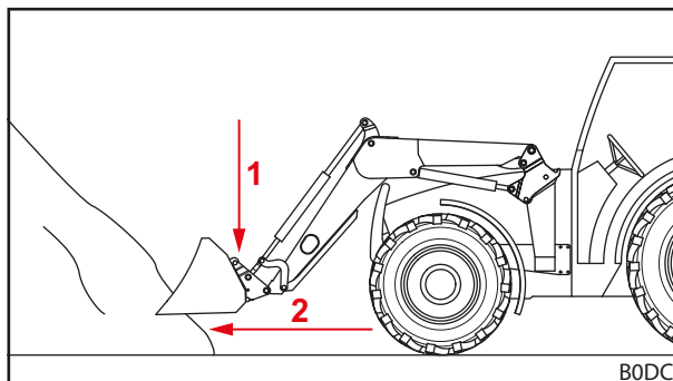
Фиг. 101 Спускане на предния товарач и вкарване право в материала за товарене
