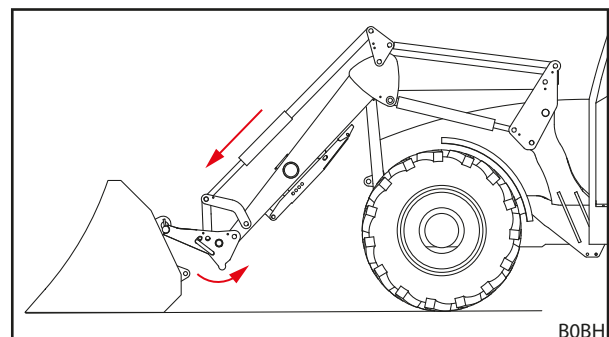
Фиг. 93 Откачване на сменната рама
