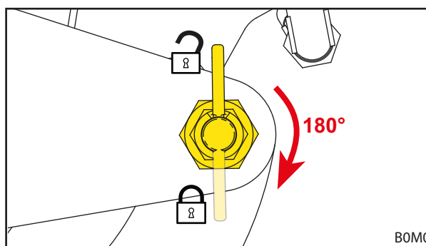
Фиг. 34 Приведете заключващия фиксатор в заключено положение
