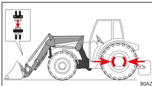
Фиг. 90 Свързване на верига за управление
