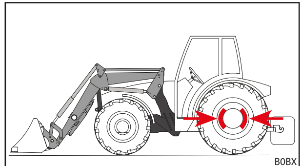
Фиг. 95 Позициониране на инструмента за оставяне и издърпване на ръчната спирачка
