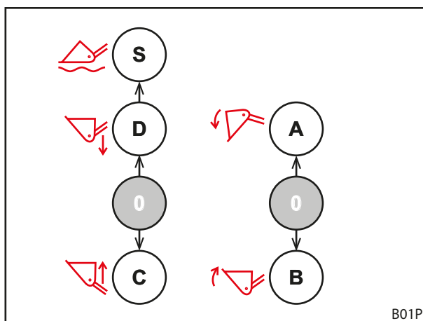
Фиг. 51 Разпределение при 2 лоста за управление
