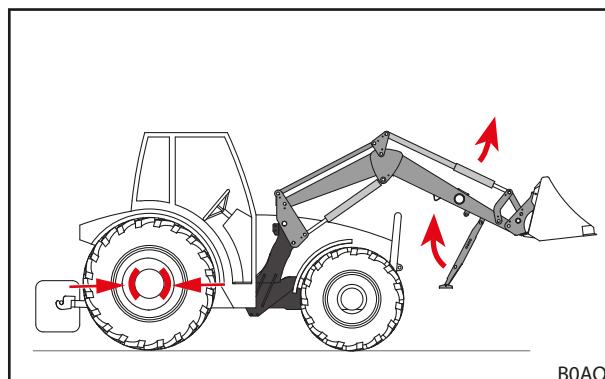
Фиг. 49 Сгъване на опорите за паркиране
