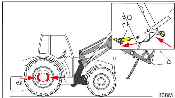
Фиг. 110 Издърпване на ръчната спирачка и освобождаване на заключването на предния товарач
