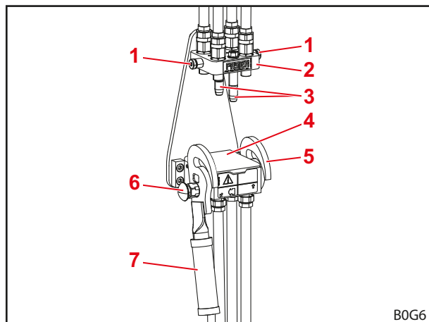
Фиг. 62 Разединен Hydro-Fix
