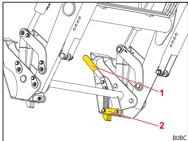
Фиг. 70 Механично заключване на инструмента Skid-Steer (заклучено състояние без инструмент)
