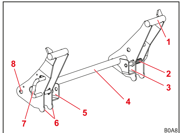
Фиг. 72 Заклучване на инструмента към сменна рама Euro
