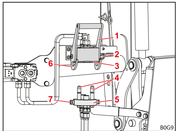
Фиг. 64 Разединено устройство за фиксиране на инструмента
