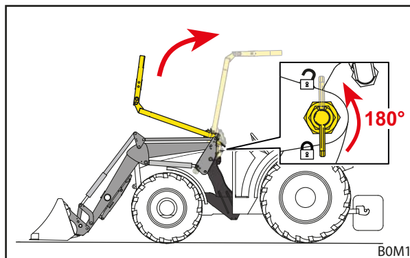
Фиг. 35 Вдигане на OPG
