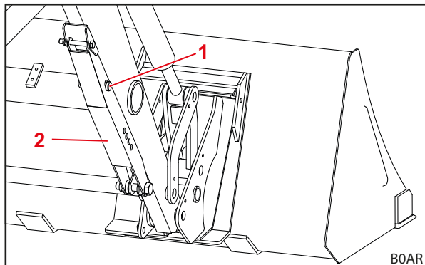
Фиг. 59 Сгъната опора за паркиране
