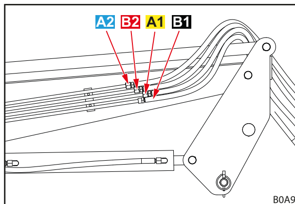
Фиг. 16 Хидравлични тръбопроводи
