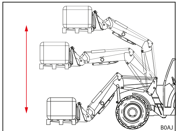
Фиг. 32 Паралелно направляване
