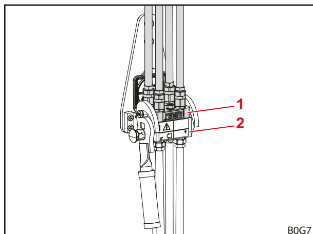
Фиг. 63 Свързан Hydro-Fix
