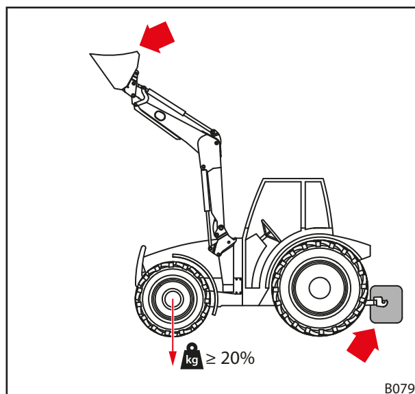
Фиг. 42 Натоварване при движение по пътища
