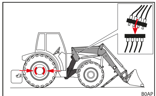
Фиг. 46 Изключване на трактора и свързване на хидравличните тръбопроводи
