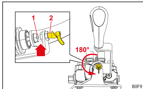
Фиг. 57 Деблокиран лост за управление
