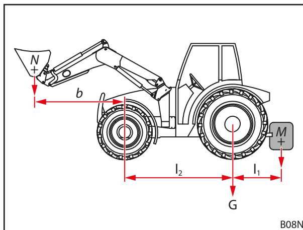
Фиг. 45 Изчисляване на статичната стабилност
