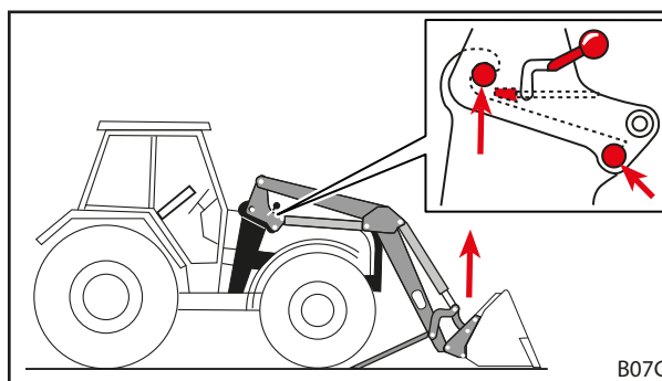
Фиг. 50 Използване на функцията за повдигане, докато палците на предния товарач попаднат в захващащите куки
