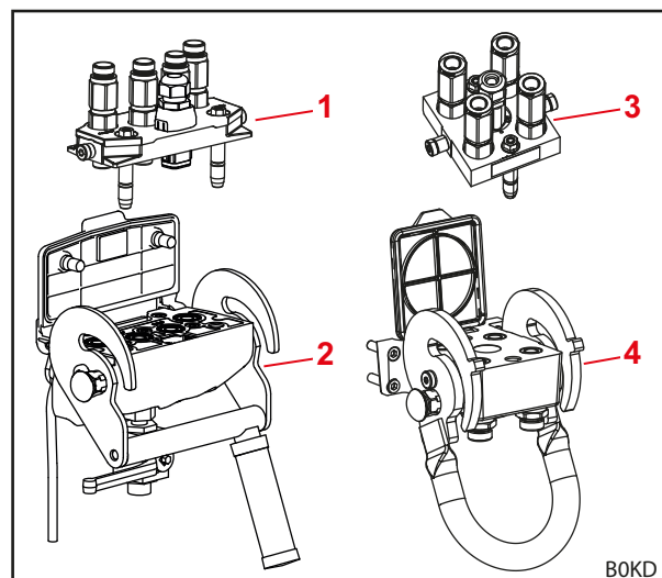
Фиг. 23 Конструкция на Hydro-Fix и мулти съединител
