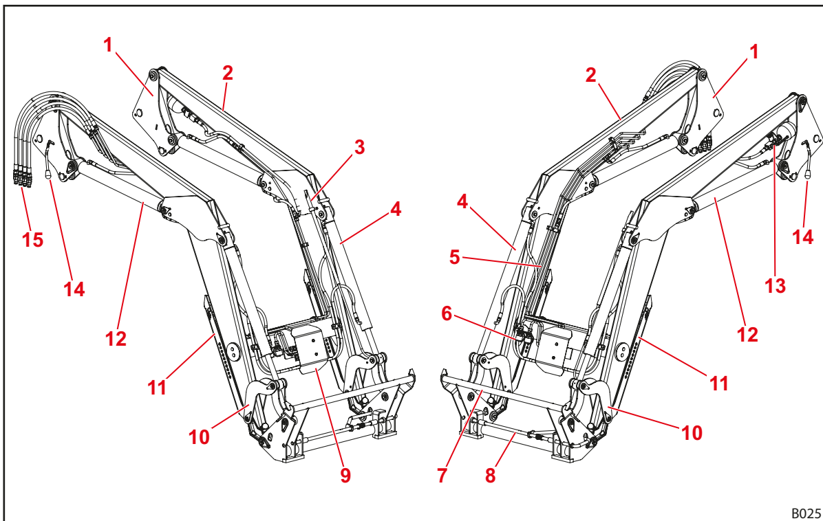
Фиг. 9 Предни товарачи H (без механично паралелно направляване)
