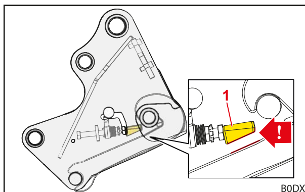
Фиг. 52 Правилно монтажное положение на затягащия клин
