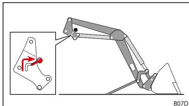
Фиг. 46 Отваряне на заключването на предния товарач
