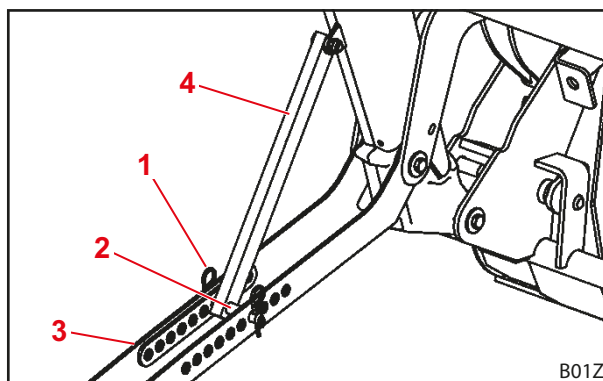
Фиг. 71 Опора за паркиране
