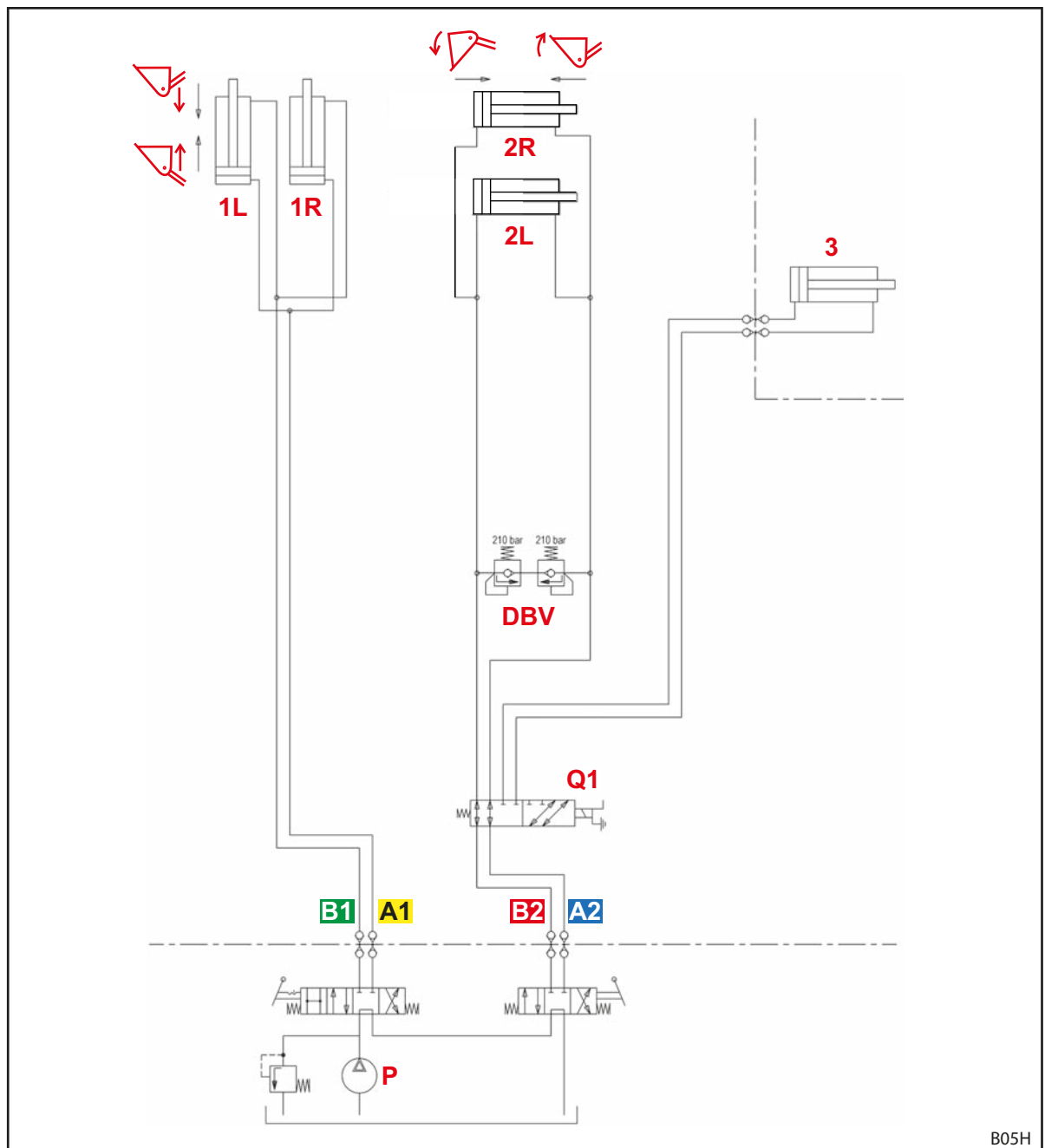
Фиг. 119 Хидравлична схема H
