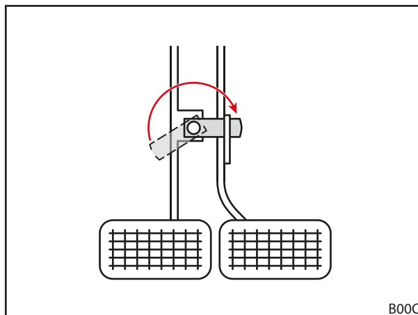
Фиг. 42 Свързване на спирачните педали
