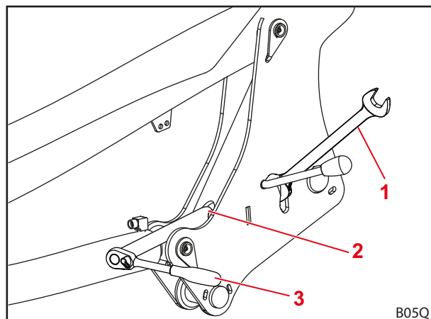
Фиг. 54 Поставяне на инструмента
