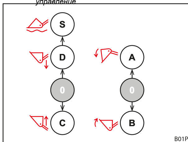
Фиг. 58 Разпределение при два лоста за управление
