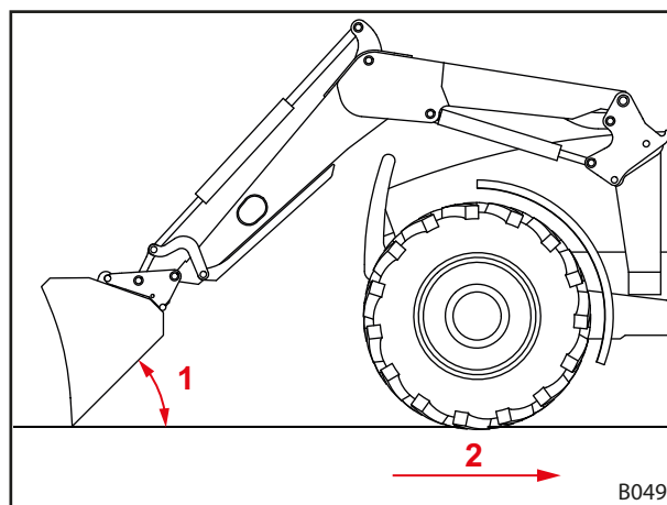
Фиг. 102 Подравняване назад
