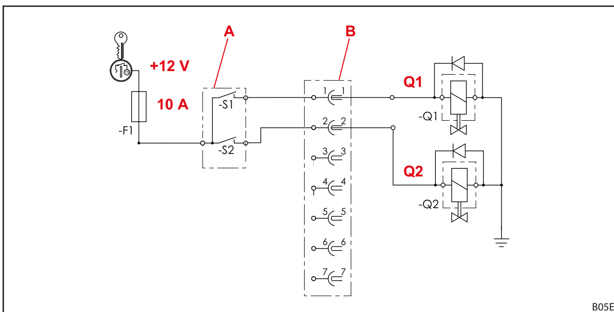
Фиг. 121 Електрическа схема
