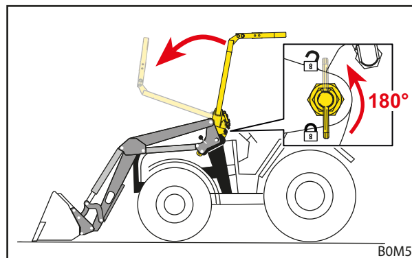
Фиг. 34 Спускане на OPG
