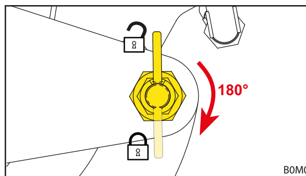
Фиг. 35 Приведете заключващия фиксатор в заключено положение
