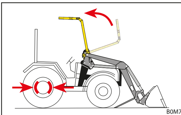
Фиг. 49 Вдигане на OPG
