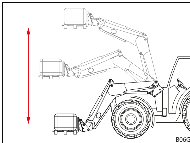
Фиг. 32 Механично паралелно направляване
