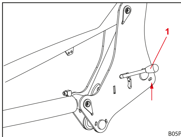
Фиг. 53 Отваряне на заключването на предния товарач
