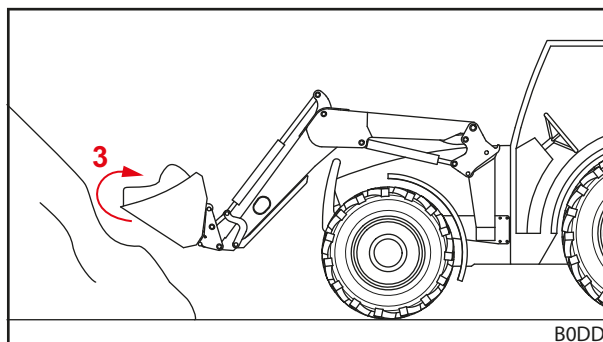
Фиг. 105 Накланяне на инструмента назад и поемане на товара
