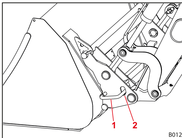
Фиг. 75 Механично заключване на инструмента
