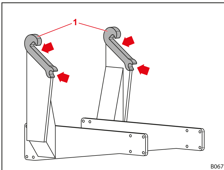
Фиг. 108 Места на смазване на гнездата на предния товарач
