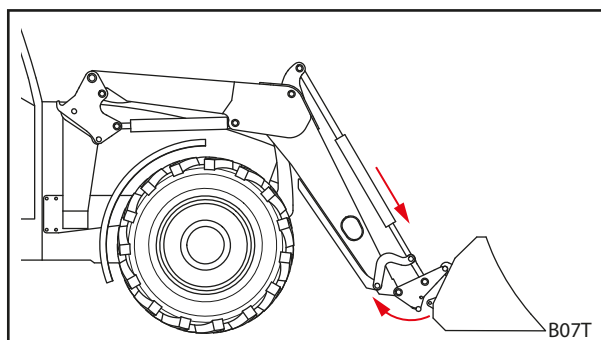
Фиг. 100 Откачване на сменната рама
