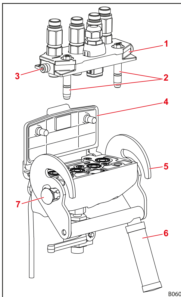
Фиг. 74 Hydro-Fix (пример: Hydro-Fix 4-точков)
