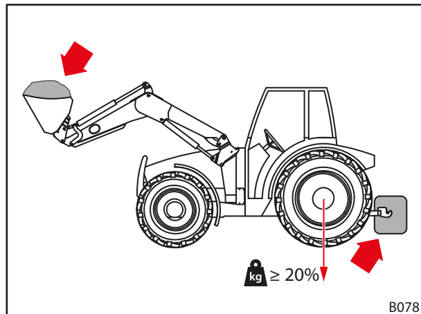
Фиг. 43 Натоварване при работи с предния товарач
