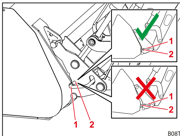
Фиг. 78 Проверка на положението на заключващия палец
