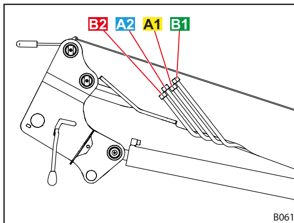
Фиг. 20 Хидравлични тръбопроводи
