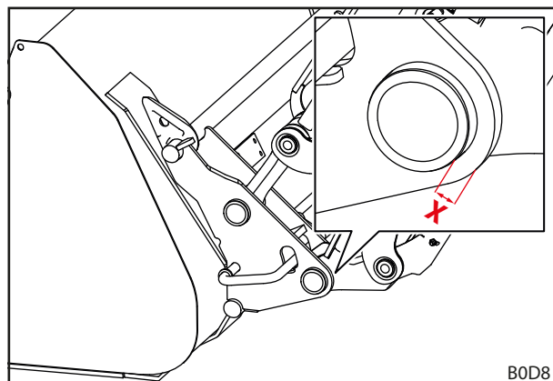
Фиг. 113 Степен на износване на сменяемата рама
