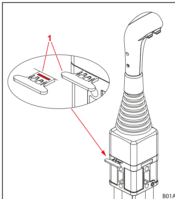
Фиг. 60 Блокировка на лоста за управление (хоризонтална блокировка)
