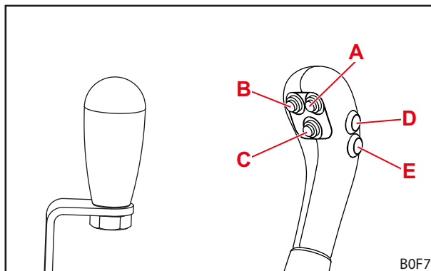
Фиг. 63 Лост за управление без бутони (вляво) и лост за управление с 5 бутон (вдясно)
