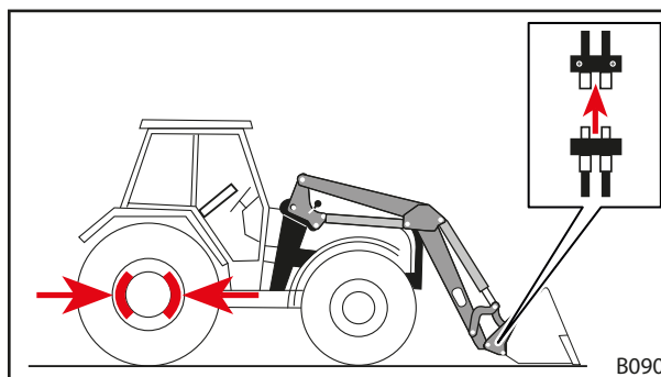
Фиг. 99 Освобождаване на хидравлични тръбопроводи
