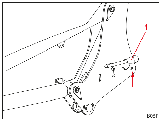
Фиг. 112 Проверка на заключването на предния товарач
