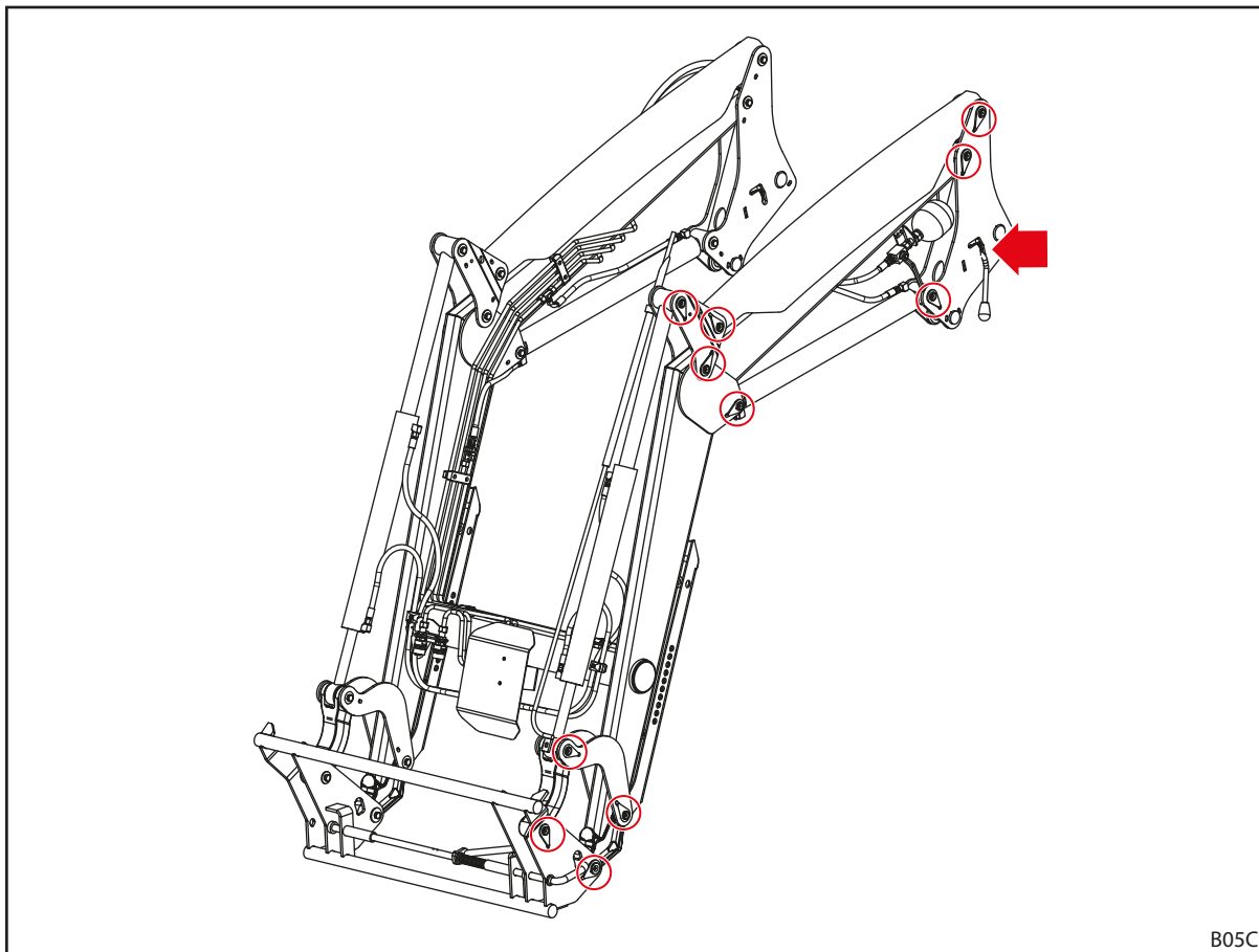
Фиг. 110 Места за смазване Р
