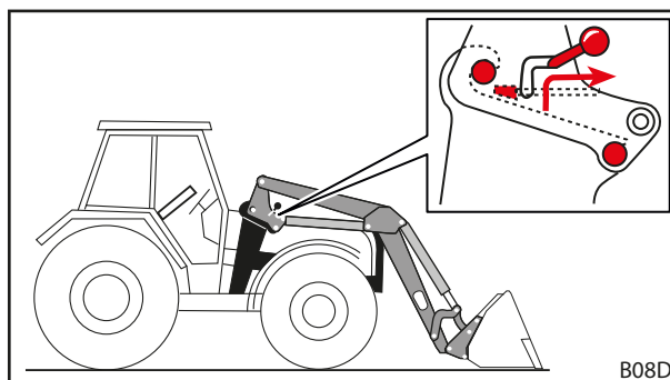
Фиг. 115 Освобождаване на заключването на предния товарач
