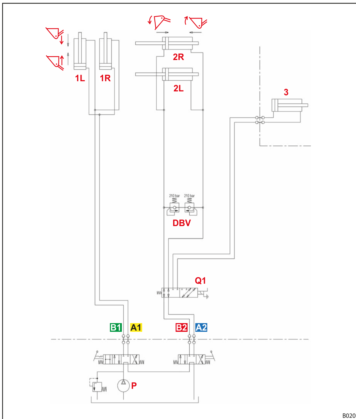
Фиг. 120 Хидравлична схема Р
