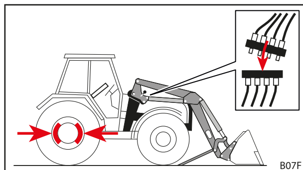
Фиг. 48 Изключване на трактора и свързване на хидравличните тръбопроводи
