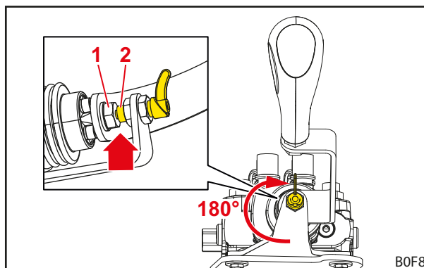
Фиг. 64 Блокиран лост за управление
