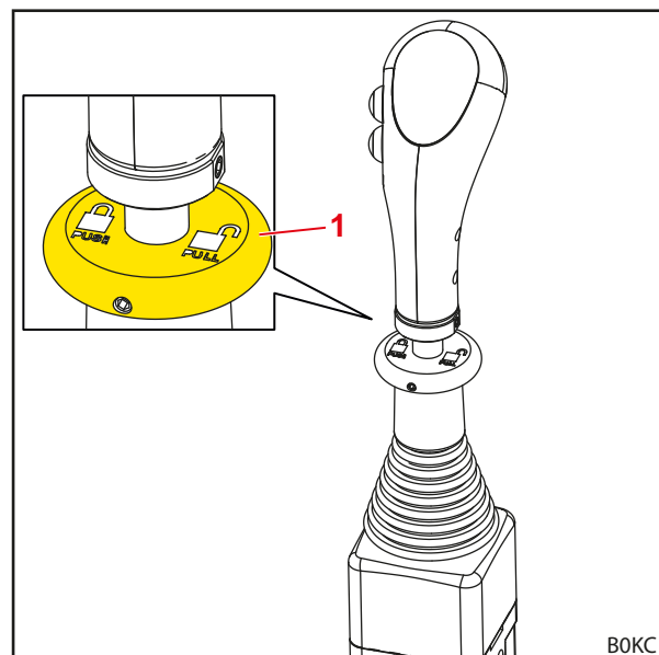
Фиг. 61 Блокировка на лоста за управление (вертикална блокировка)
