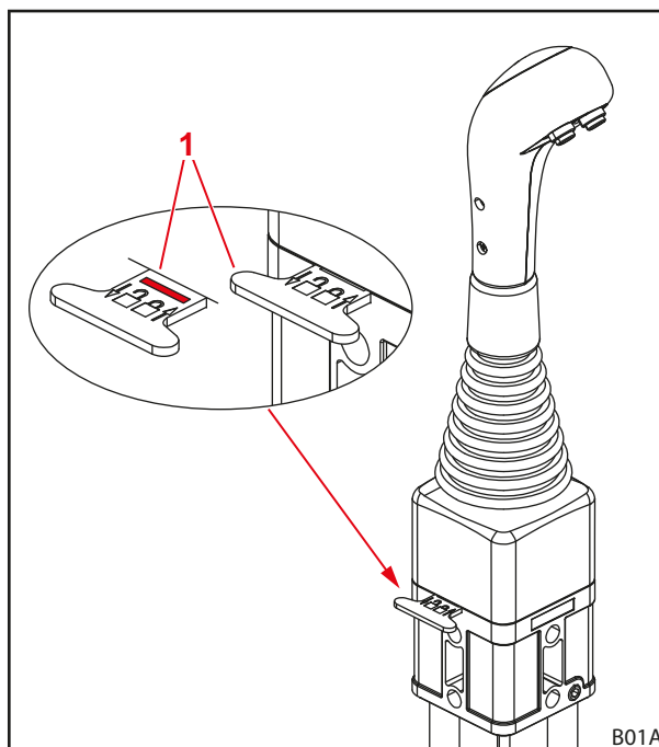
Фиг. 67 Блокировка на лоста за управление (хоризонтална блокировка)
