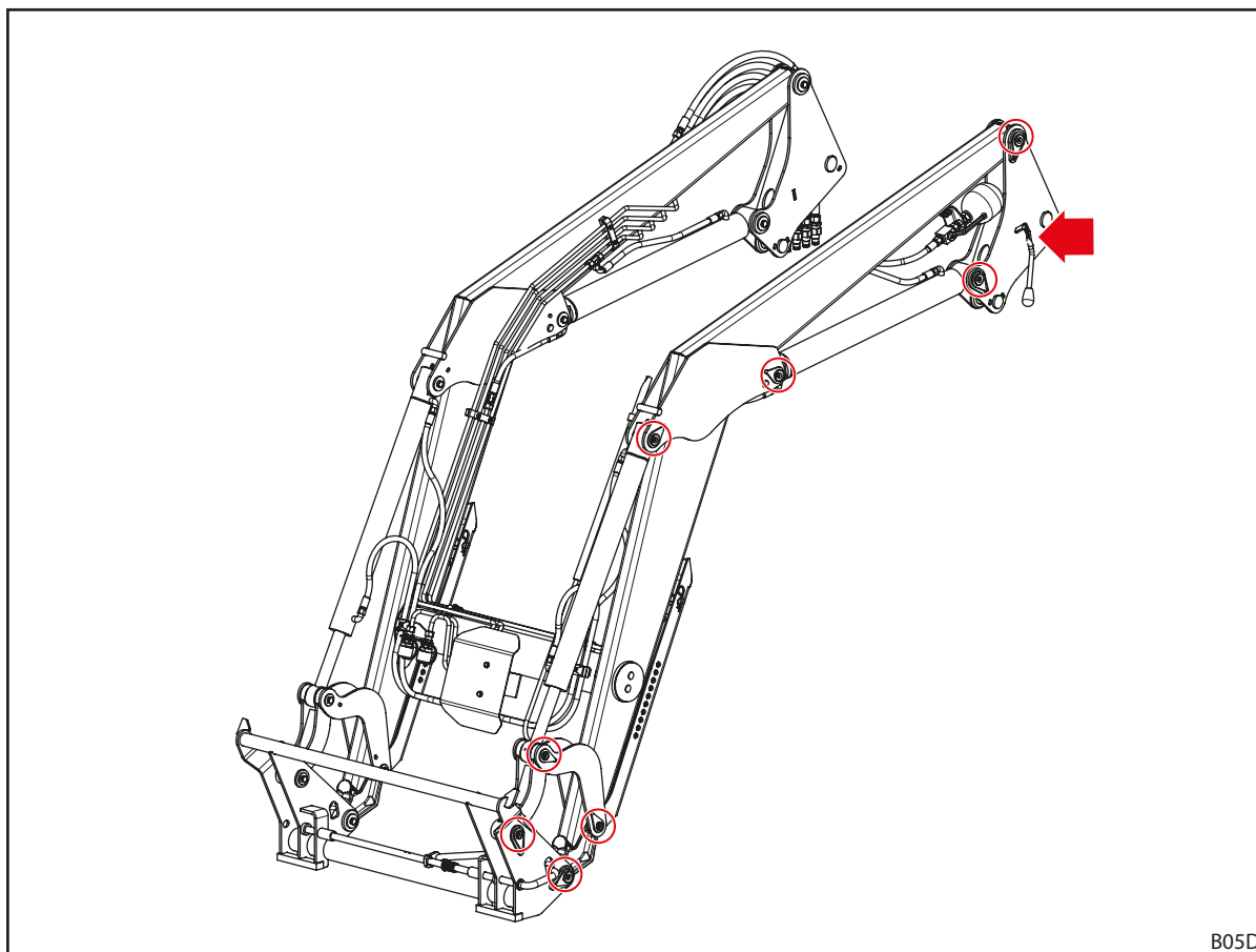
Фиг. 116 Места за смазване Н
