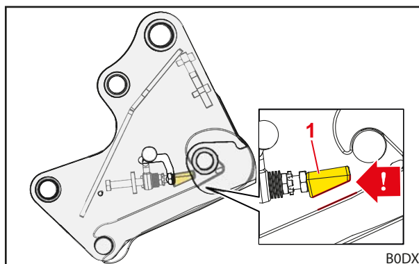
Фиг. 59 Правилно монтажно положение на затягащия клин
