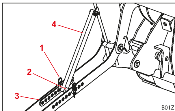
Фиг. 78 Опора за паркиране
