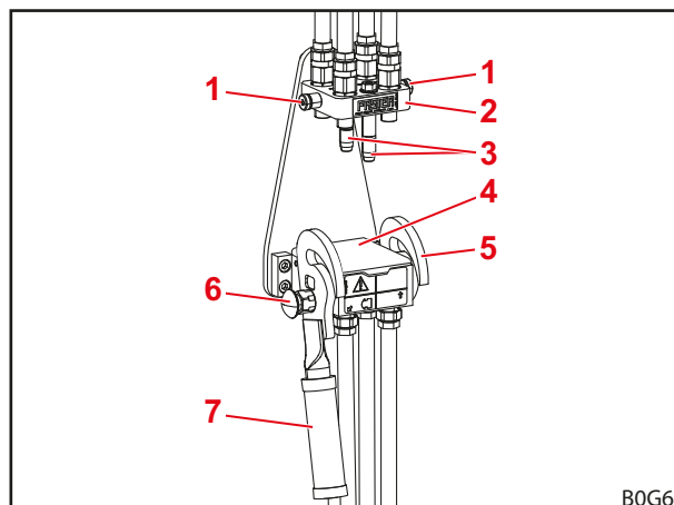
jn 54 Lahtiühendatud Hydro-Fix
