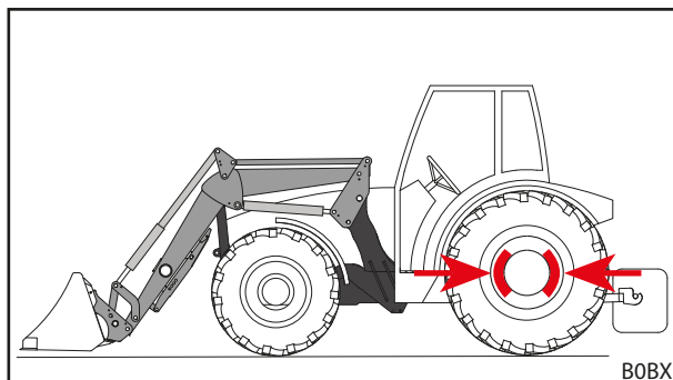
jn 83 Tööseadise positsioneerimine eemaldamiseks ja seisupiduri rakendamine
