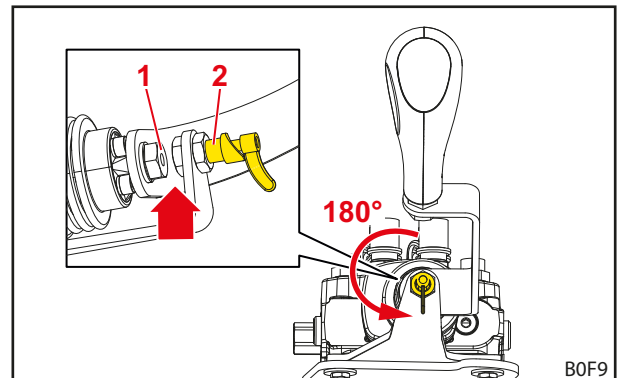
jn 49 Lukustusest vabastatud juhthoob
