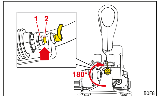
jn 48 Lukustatud juhthoob
