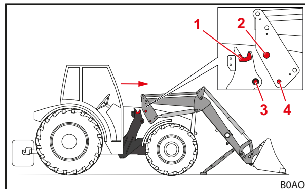
jn 38 Traktoriga tõstehaarade vahele sõitmine
