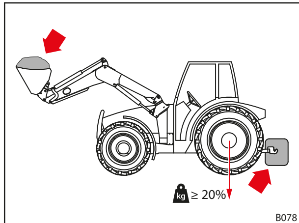
jn 34 Koormus lauplaaduriga tööde teostamisel
