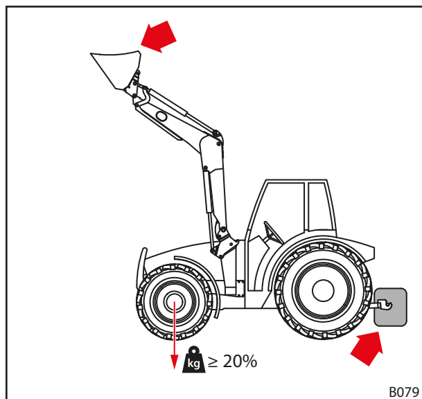
jn 35 Koormus üldkasutatavatel teedel sõitmisel
