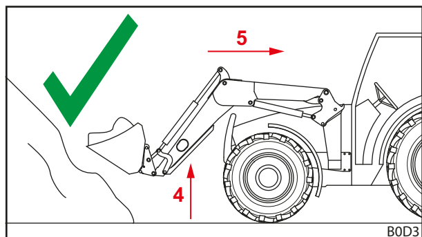
jn 95 Koormatud tööseadisega tagurdamine – õige
