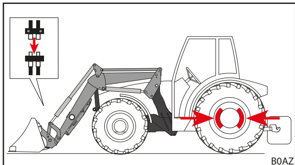
jn 77 Juhtkontuuri külgeühendamine
