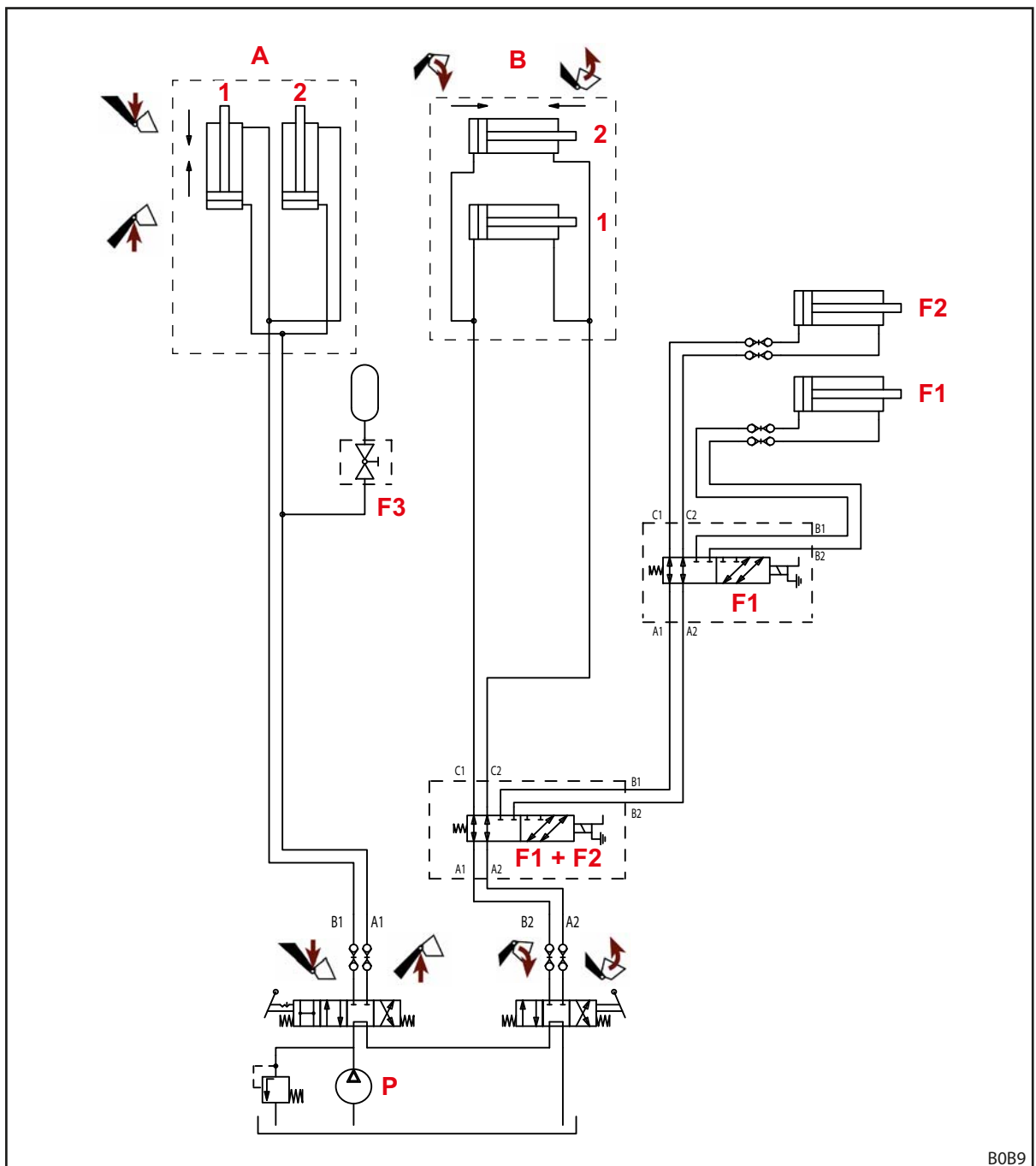
jn 105 FC hüdraulikaskeem
