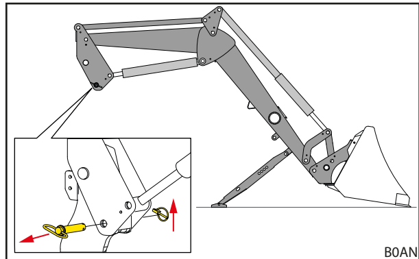
jn 37 Lauplaaduri lukustuse avamine
