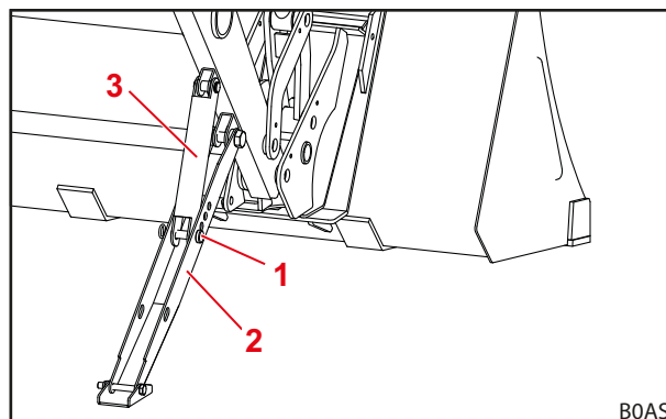
jn 52 Tugiseadis välja pööratud
