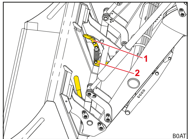
jn 61 Skid-Steeri tööseadise mehaaniline lukustus (lukustatud olek koos tööseadisega)
