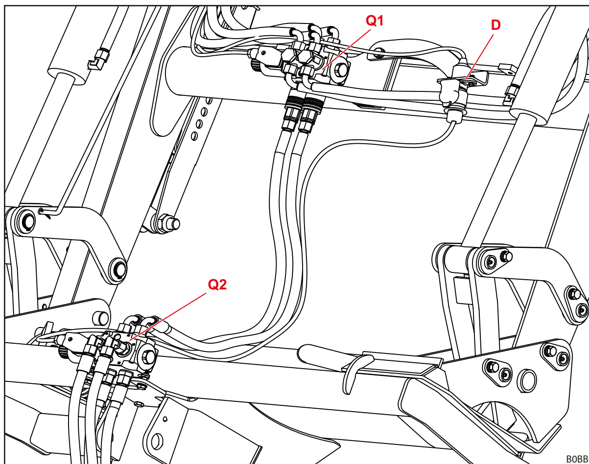
jn 107 Lisafunktsioonide hüdroventiilide paigutus
