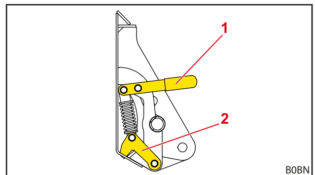
jn 58 Skid-Steeri tööseadise mehaaniline lukustus (avatud olekus)
