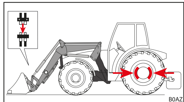
jn 72 Juhtkontuuri külgeühendamine
