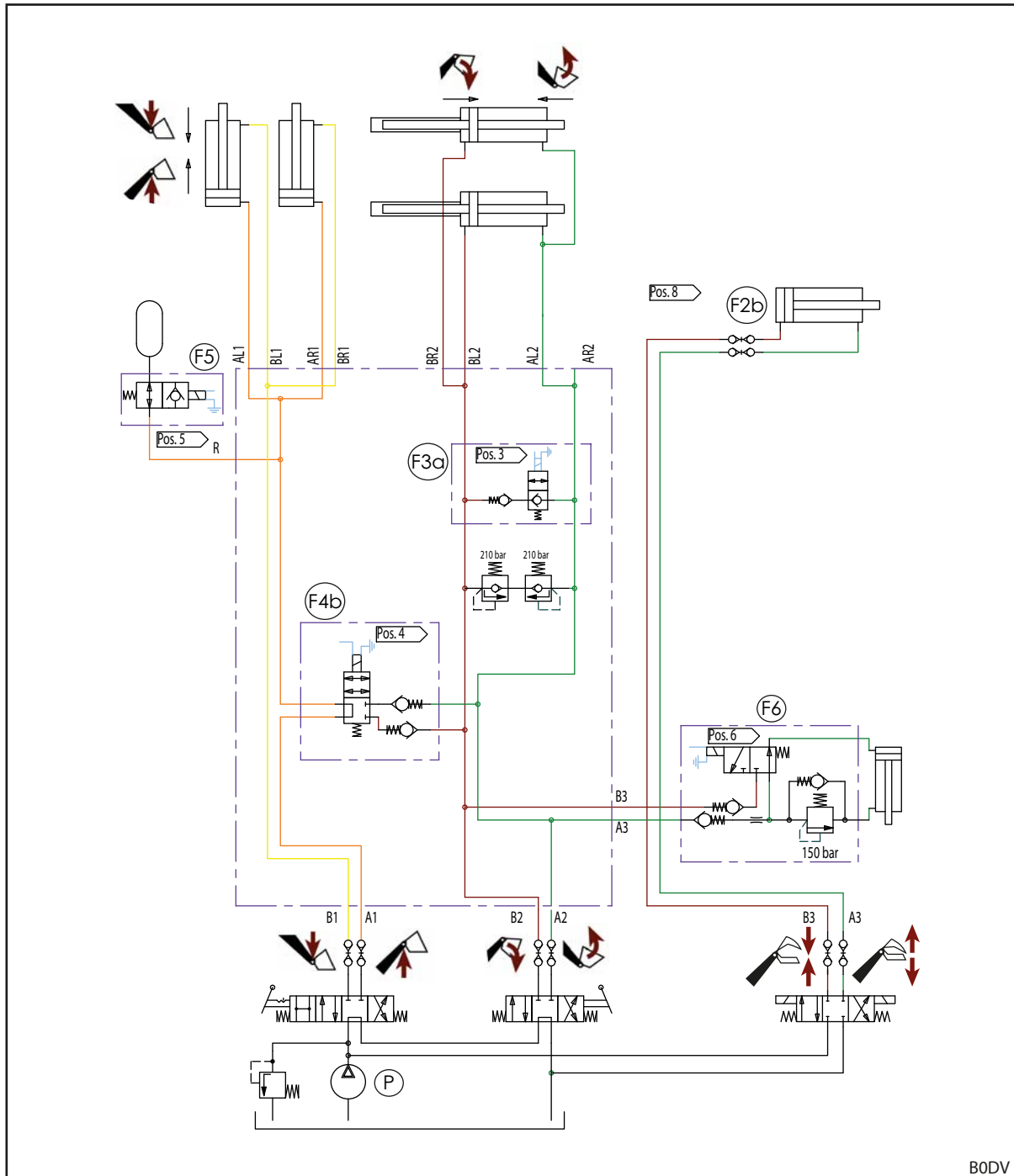
jin 130 Hüdralikaskeem FZ ja FZ-L (REAL 3 varustuse korral)
