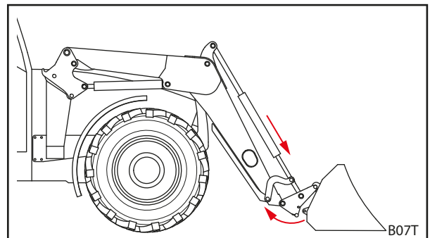
jn 106 Vahetusraami lahtihaakimine
