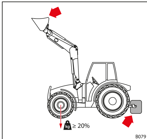
jn 45 Koormus üldkasutatavatel teedel sõitmisel
