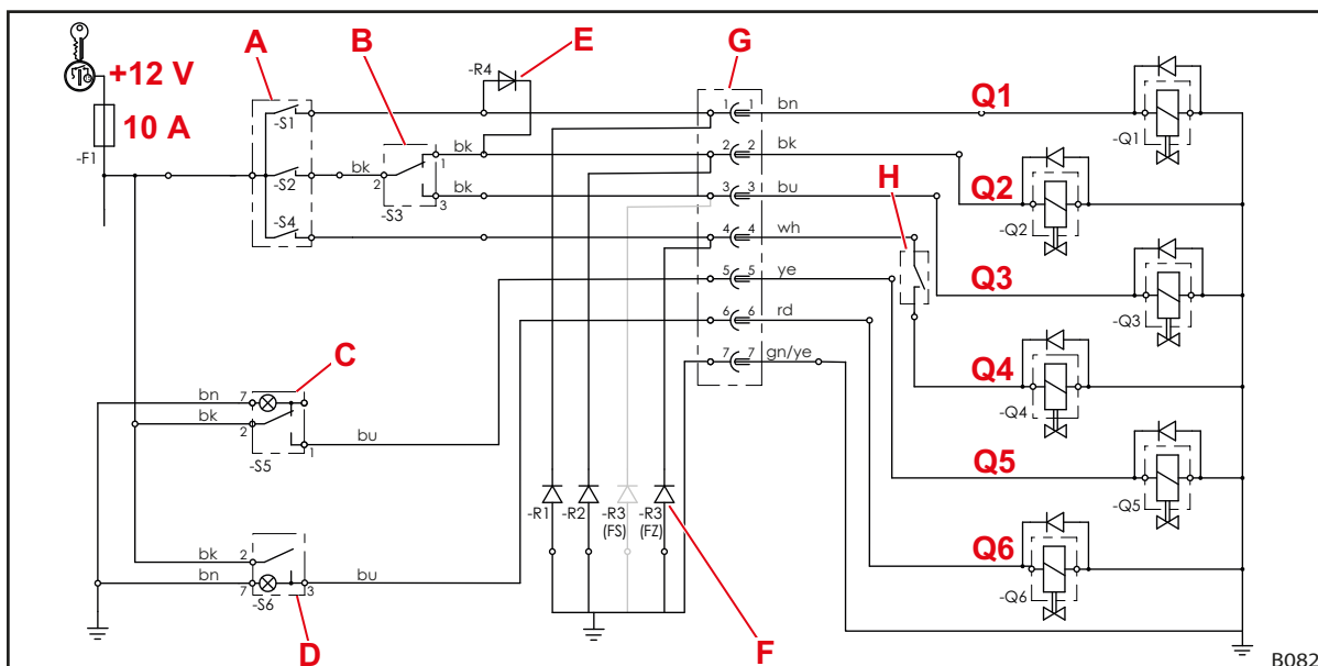
jn 131 Elektriskeem (3. ja 4. juhtkontuuriga varustuse korral)
