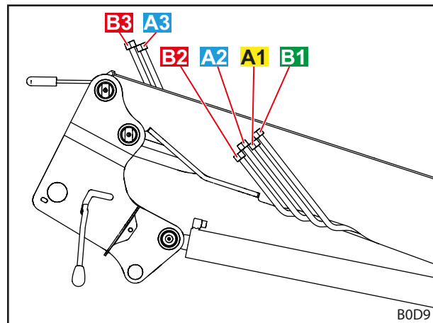
jn 18 Hüdrovoolikud (lisavarustus REAL 3 )
