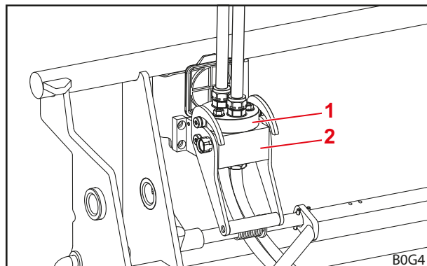
jn 79 Külgeühendatud tööseadis-Fix
