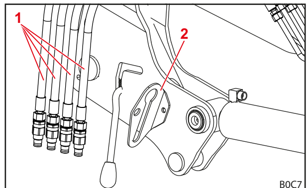
jn 126 Hüdrovoolikute fikseerimine muhvikinnitusse (pistikmuhvidega kujutis)
