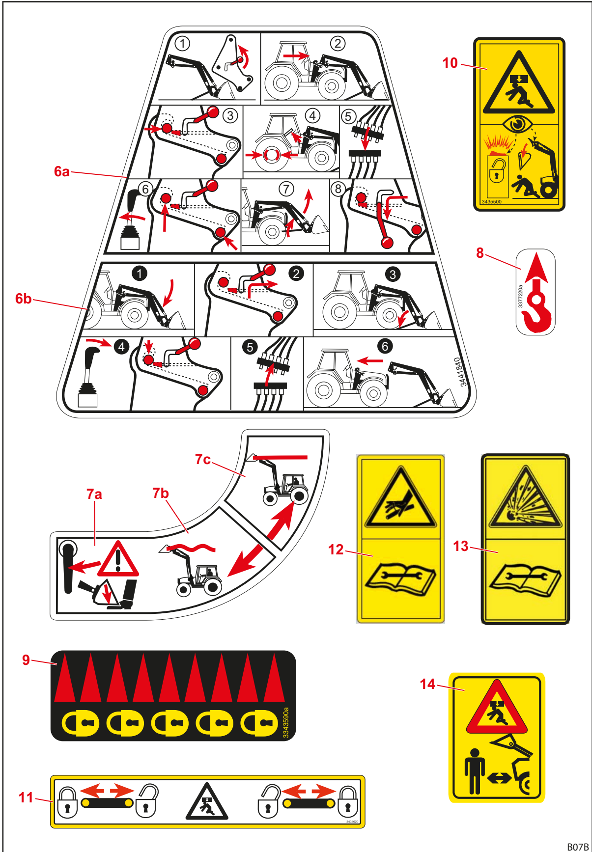
jn 6 Turvakleebiste asukohad 6-14
