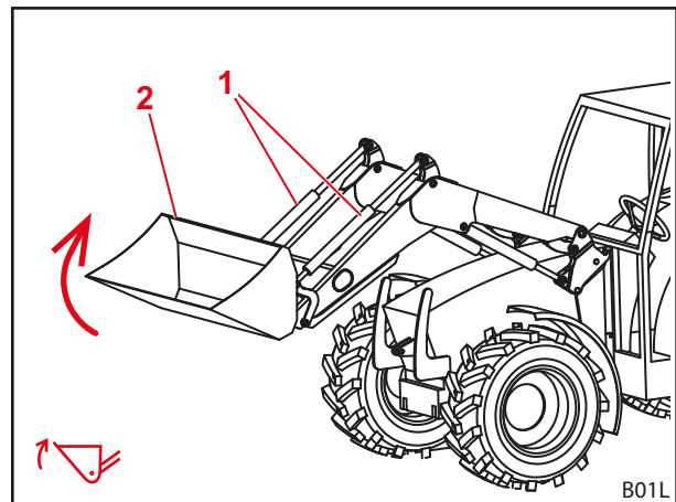
jn 29 Kopa täitmise funktsioon
