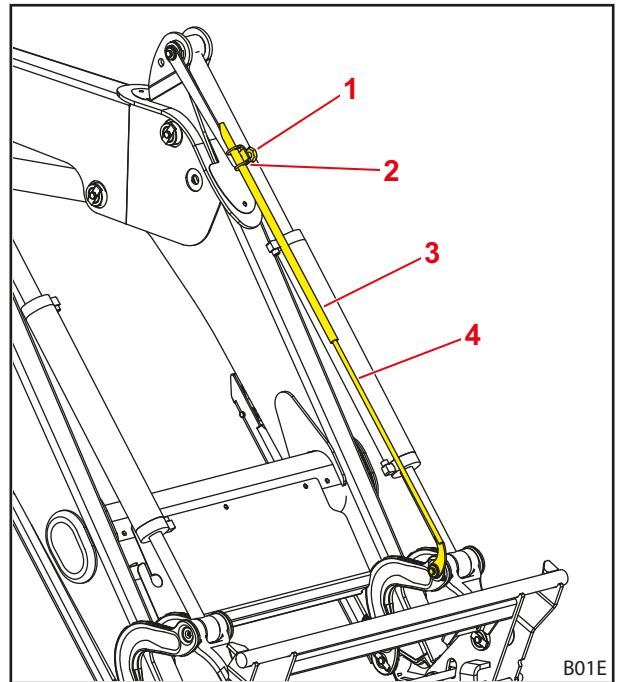
jn 32 Tööseadise asendi visuaalne näit
