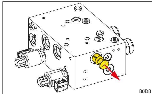
jn 72 Tõmmake REAL 3 -ventiili survealandusventiil välja.
