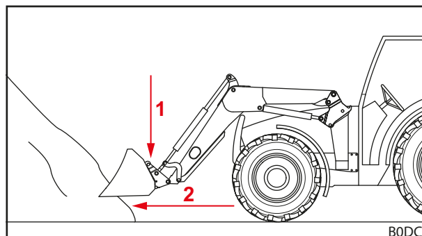
jn 109 Lauplaaduri langetamine ja sirgelt laaditava materjali sisse sõitmine
