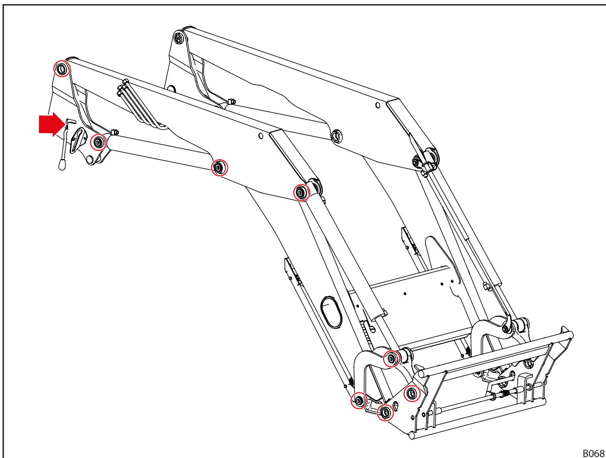
jn 114 FS määrimiskohad
