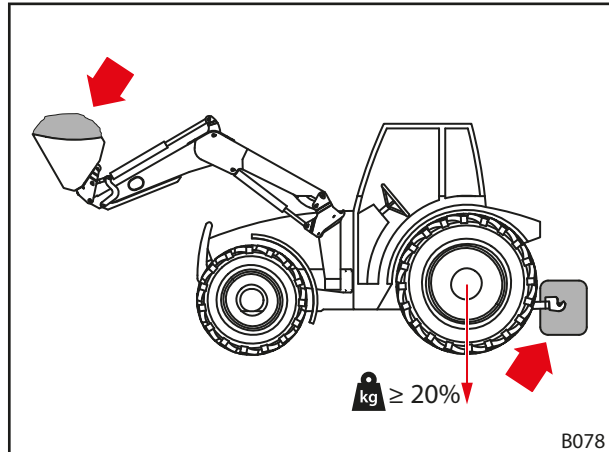
jn 44 Koormus lauplaaduriga tööde teostamisel
