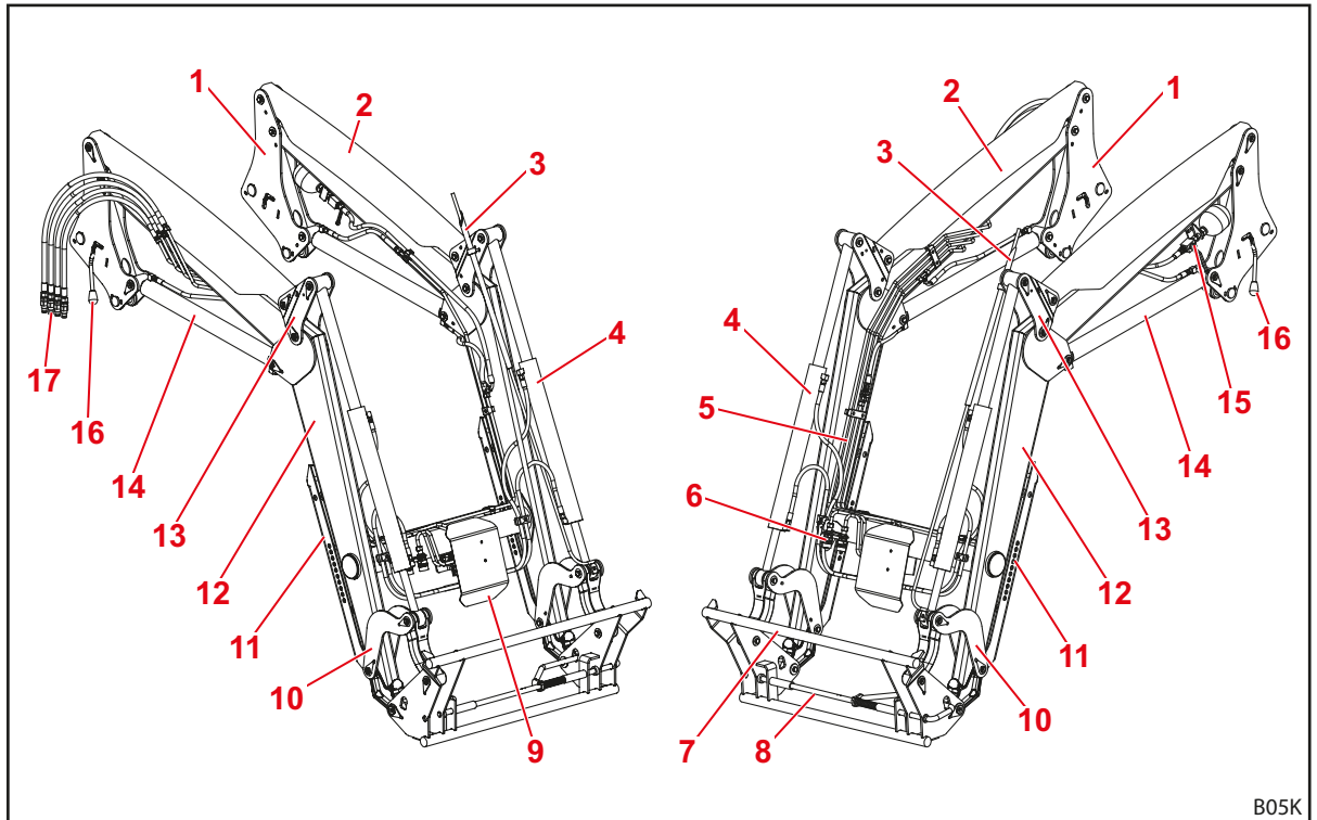
Kuva 10 Etukuormain P (mekaanisella suoraviivaisen liikkeen ohjaimella)
