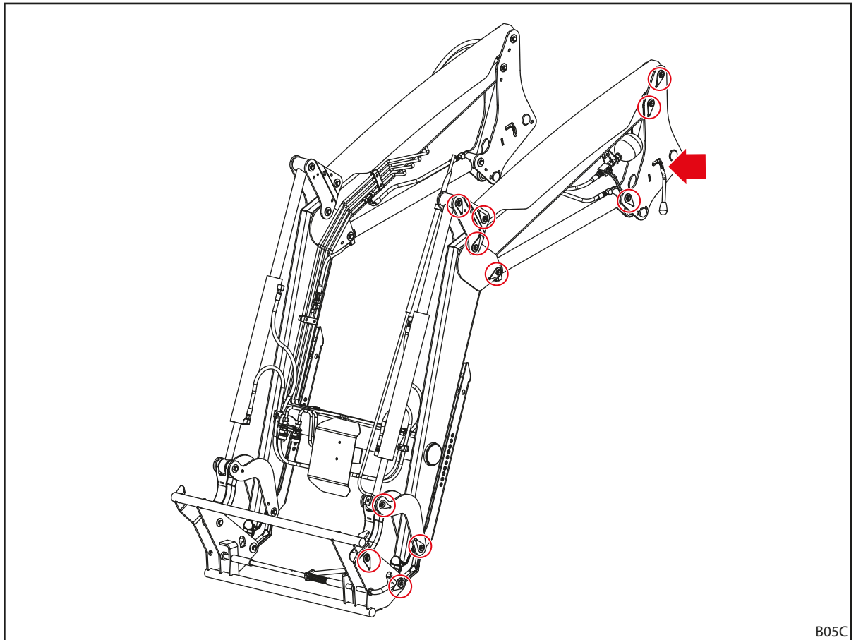
Kuva 110 Voitelukohdat P
