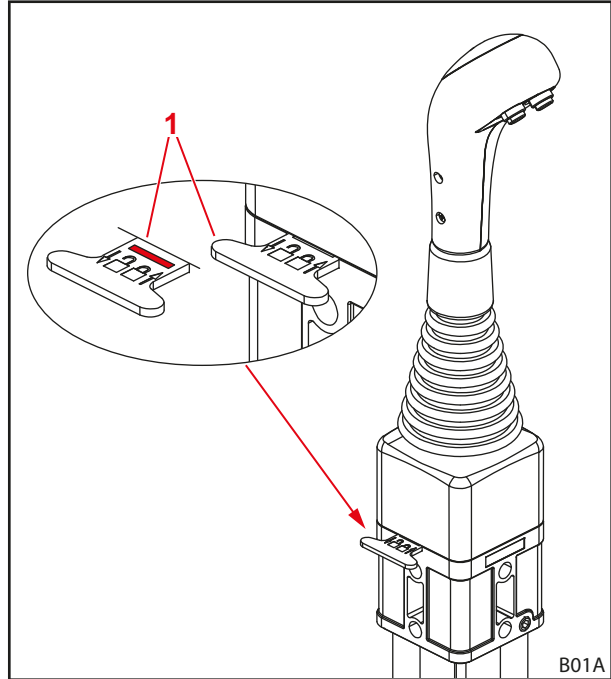
Kuva 60 Ohjausvivun lukitseminen (vaakasuora lukitus)
