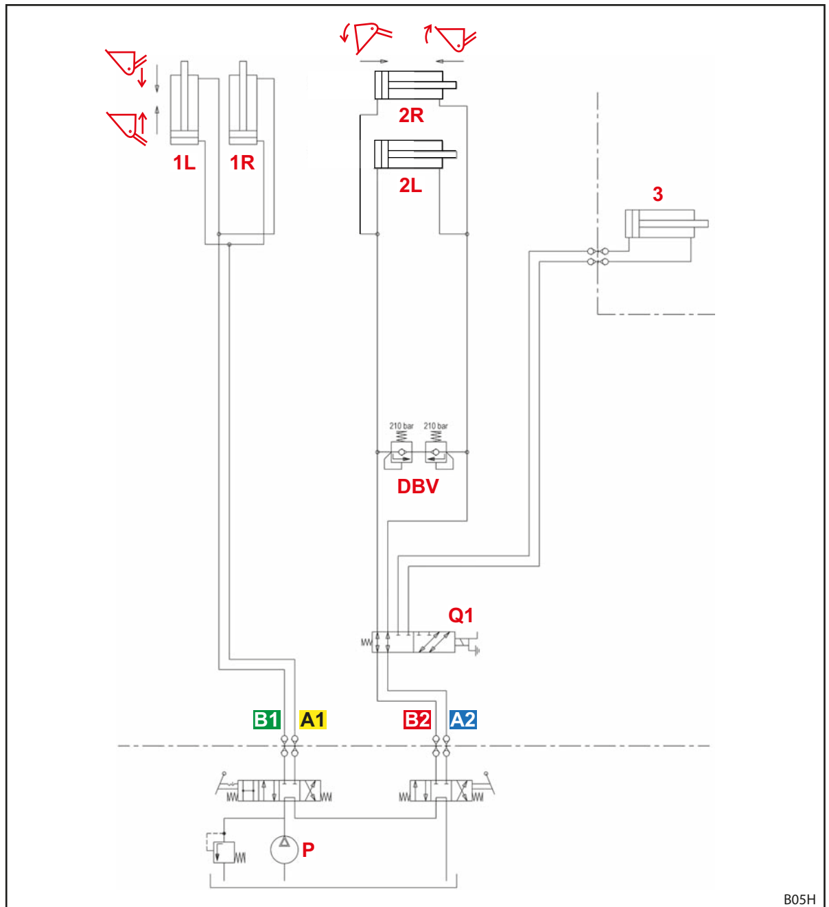
Kuva 119 Hydraulikkapiirustus H
