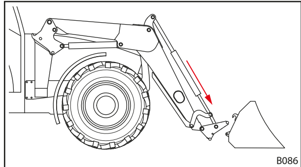
Kuva 89 Aisaston kohdistaminen
