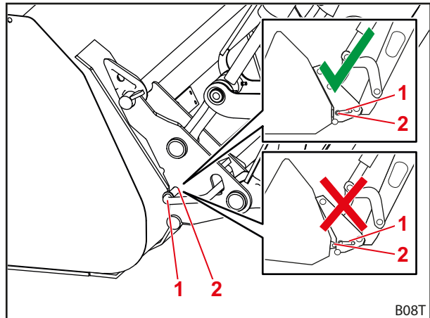
Kuva 78 Lukituspulttien sijainnin tarkastaminen
