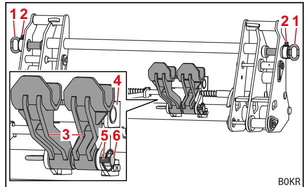
Kuva 86 Adapteri pysäköintiasennossa (vaihtorunko valmisteltu Euro-työkalua varten)
