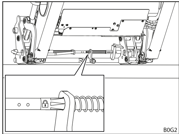
Kuva 77 Tarkasta työkalun lukitus tarran perusteella (yhdistelmävaihtorunko Euro-FR)
