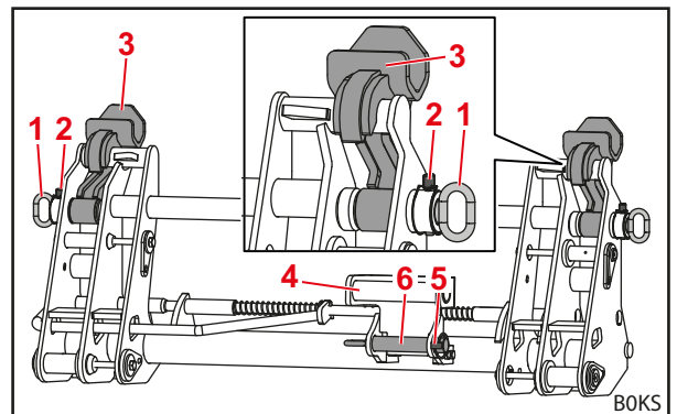
Kuva 87 Adapteri työasennossa (vaihtorunko valmisteltu FR-työkalua varten)
