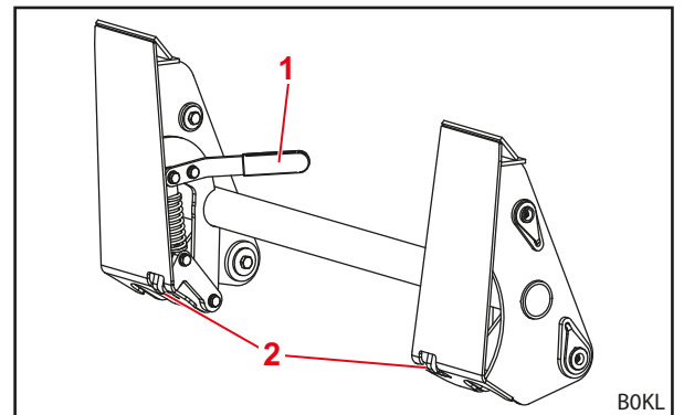
Kuva 14 Skid-Steer-vaihtorunko
