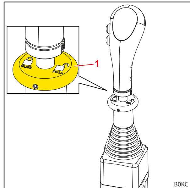
Kuva 61 Ohjausvivun lukitseminen (pystysuora lukitus)
