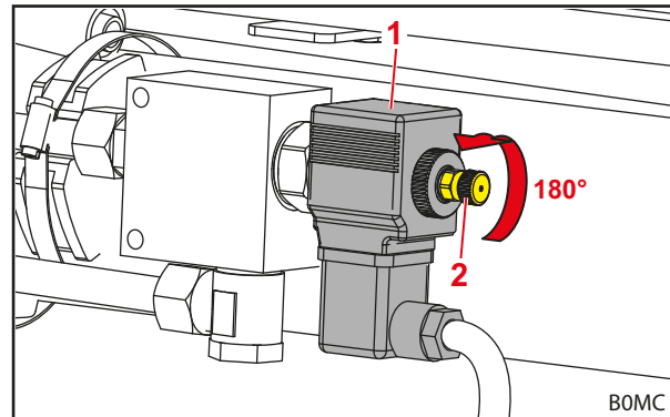
Kuva 33 Venttiilin avaaminen
