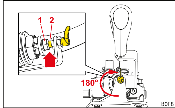
Kuva 64 Lukittu ohjausvipu
