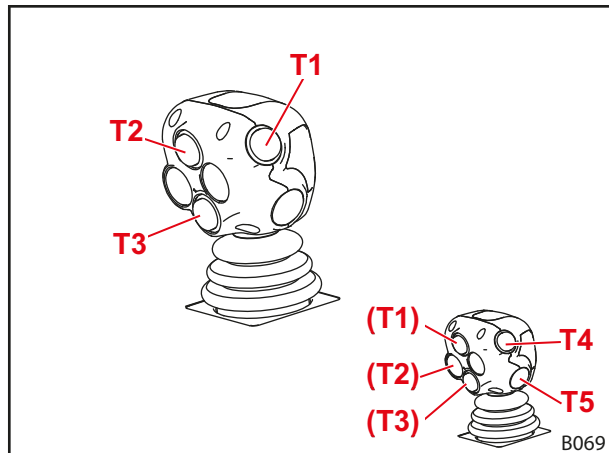
Kuva 69 STOLL Trac Control (3 painiketta)
