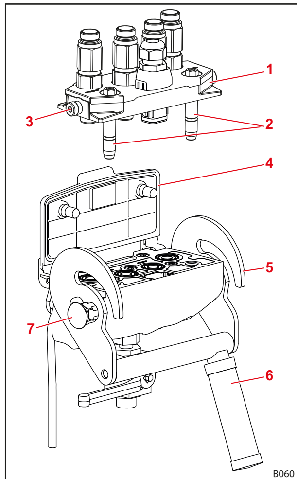
Kuva 74 Hydro-Fix (esimerkki: Hydro-Fix 4-kertainen)
