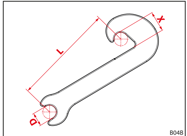
Kuva 111 Jarrutuskoukun kulumismitat
