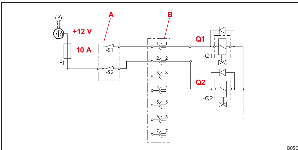
Kuva 121 Sähkökytkentäkaavio
