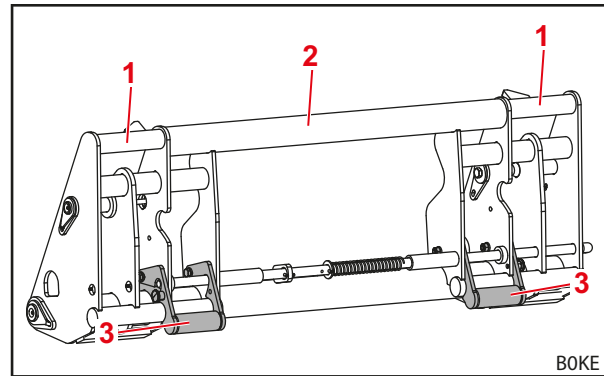
Kuva 15 Yhdistelmävaihtorunko Euro-SMS (valmisteltu Euro-työkalua varten)
