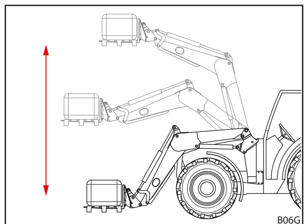
Kuva 32 Mekaaninen suoraviivaisen liikkeen ohjain
