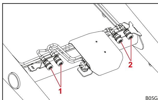
Kuva 39 Ylimääräinen 4. ohjauspiiri
