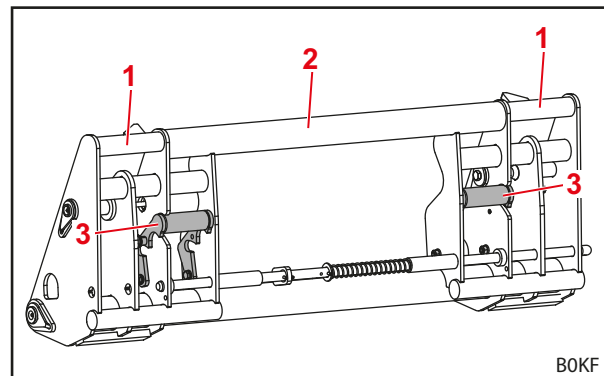
Kuva 16 Yhdistelmävaihtorunko Euro-SMS (valmisteltu SMS-työkalua varten)
