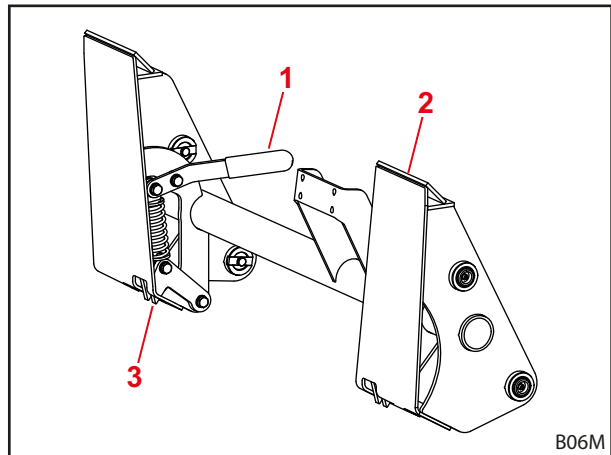
Kuva 25 Skid-Steer-vaihtorungon mekaaninen työkalun lukitus
