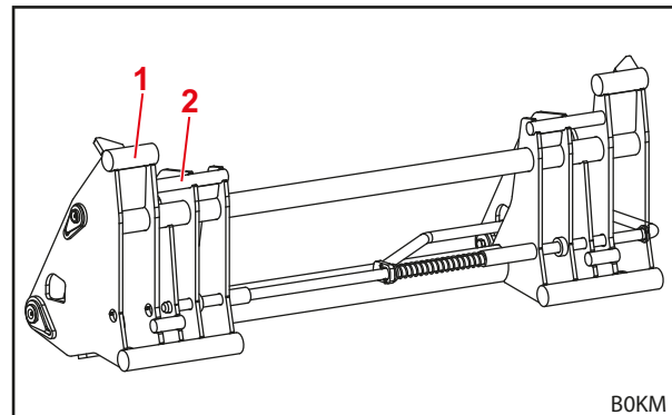
Kuva 17 Yhdistelmävaihtorunko Euro-Alö3
