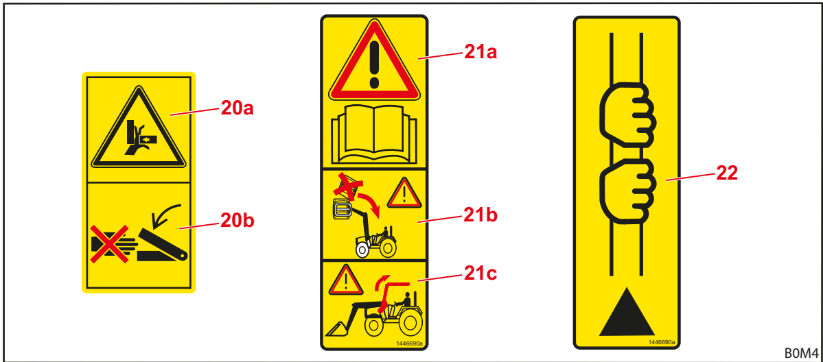
Kuva 8 Varoitustarrat
