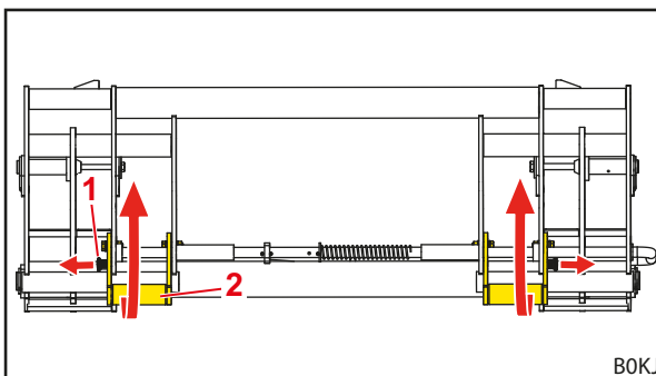
Kuva 84 Laitteistojen ylöskääntäminen
