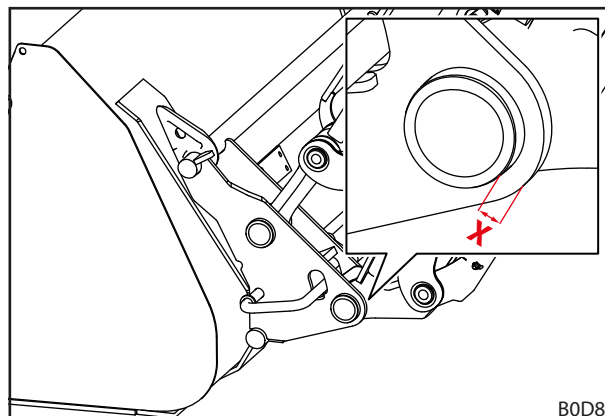
Kuva 113 Vaihtorungon kulumismitta
