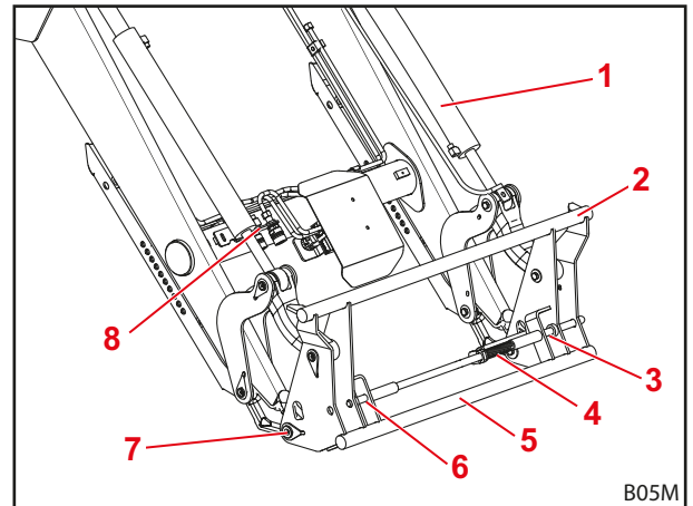
Kuva 13 Euro-vaihtorunko
