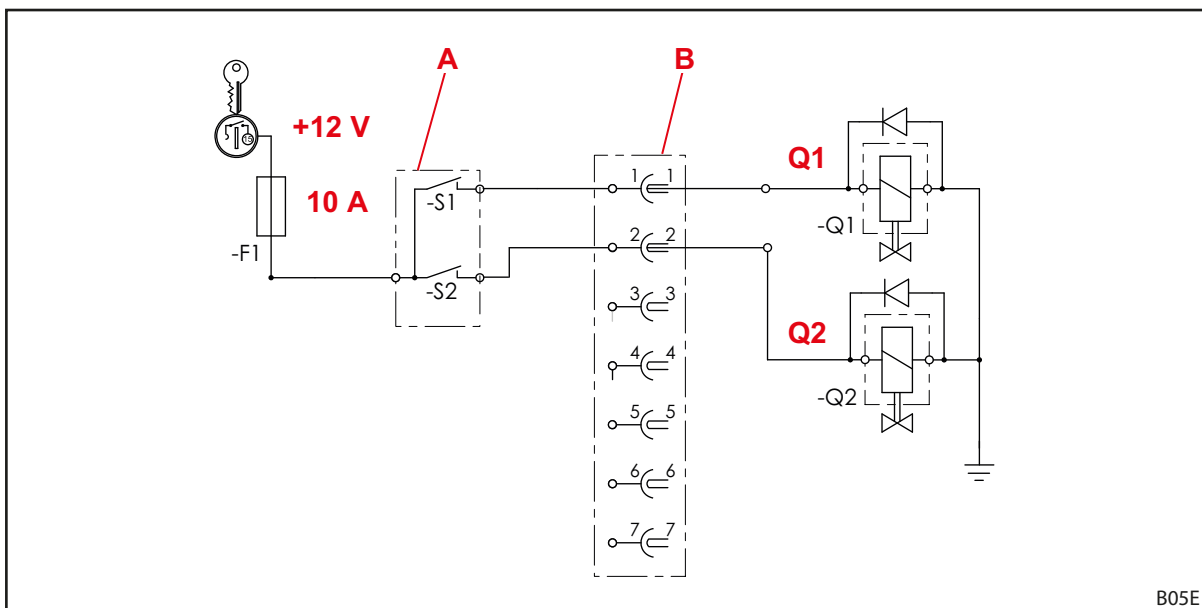
Kuva 128 Sähkökytkentäkaavio
