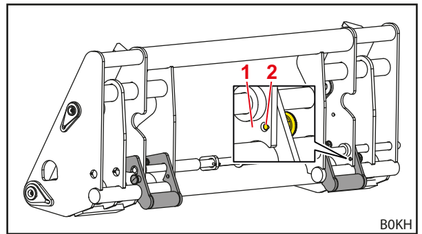
Kuva 90 Alaskäännetyt laitteistot
