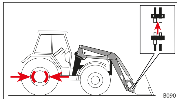
Kuva 106 Hydraulikkalinjojen irrotus
