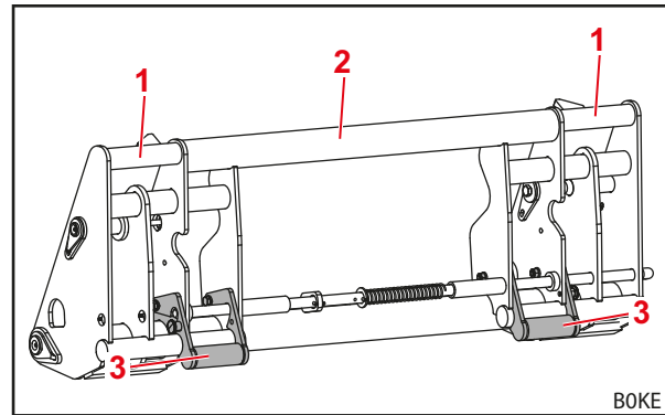
Kuva 17 Yhdistelmävaihtorunko Euro-SMS (valmisteltu Euro-työkalua varten)
