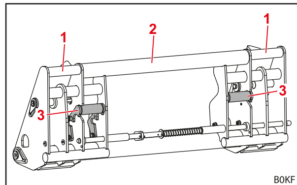
Kuva 18 Yhdistelmävaihtorunko Euro-SMS (valmisteltu SMS-työkalua varten)
