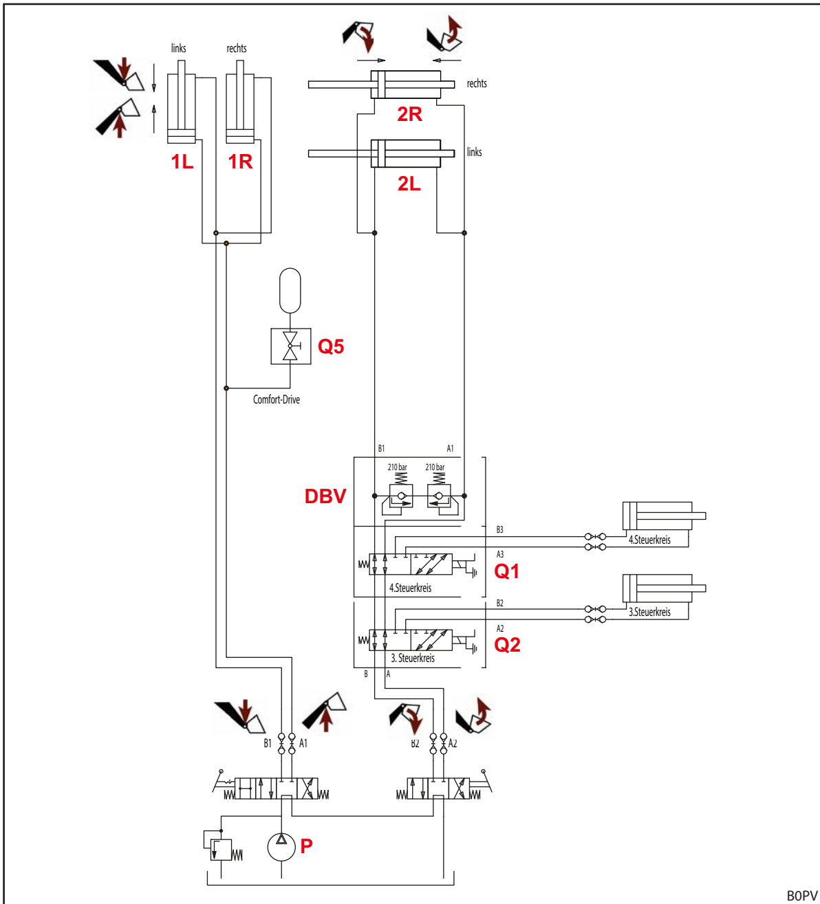
Kuva 127 Hydraulikkapiirustus P
