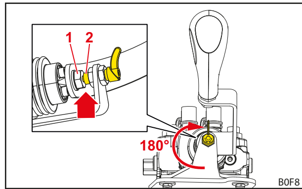
Kuva 71 Lukittu ohjausvipu
