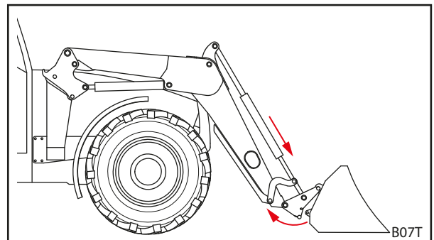
Kuva 107 Vaihtorungon irrottaminen
