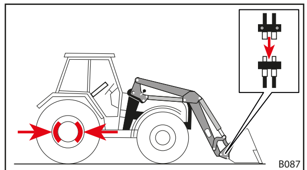
Kuva 100 Työkalun hydraulikkalinjojen liittäminen etukuormaimen liittimiin
