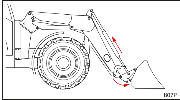
Kuva 106 Koukkuun kiinnitys
