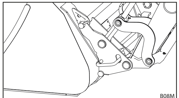
Kuva 95 Työkalun lukituksen avaaminen
