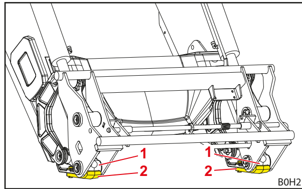
Kuva 14 Kulutusjalakset
