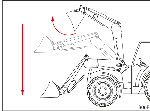
Kuva 33 Return-To-Level-toiminto
