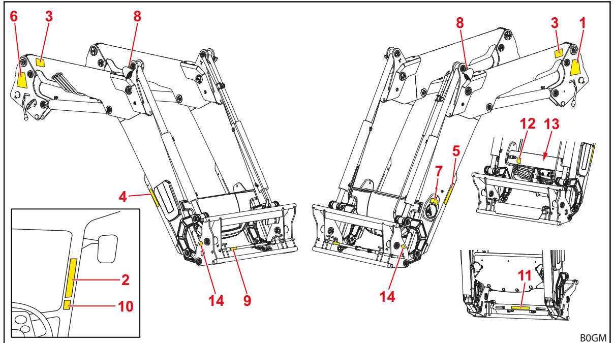
Kuva 4 Etukuormain FZ (kuva esimerkinomainen)
