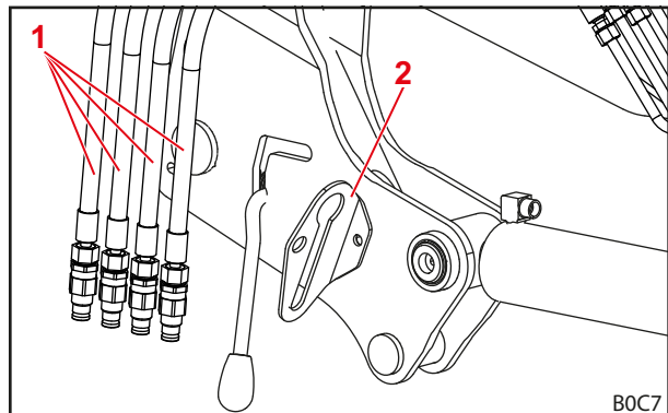
Kuva 130 Hydraulikkalinjojen kiinnittäminen kytkimen varteen (kuvassa pistoliitännöillä varustettuna)
