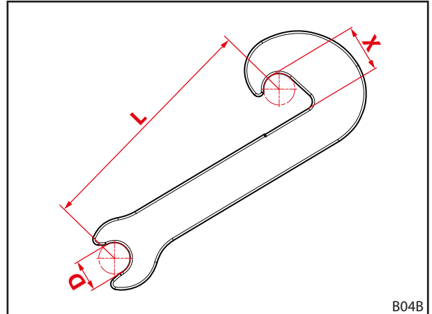
Kuva 120 Jarrutuskoukukun kulumismitat
