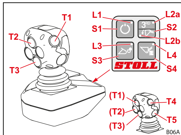
Kuva 70 STOLL Pro Control
