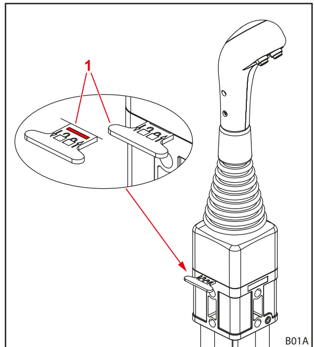
Kuva 68 Ohjausvivun lukitus
