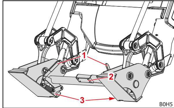
Kuva 13 Skid-Steer-vaihtorunko
