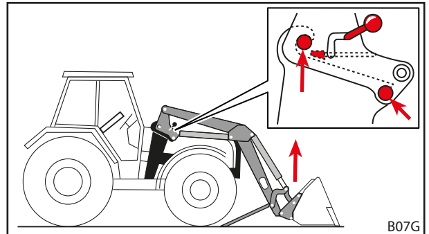
Kuva 53 Käytä nostotoimintoa, kunnes etukuormaimen pultit ovat kiinni jarrutuskoukuissa
