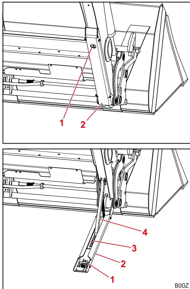
Kuva 78 Tukijalka
