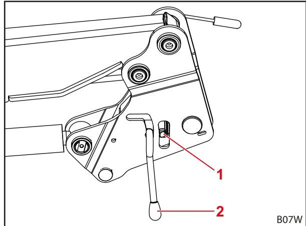
Kuva 122 Etukuormaimen lukituksen tarkastus
