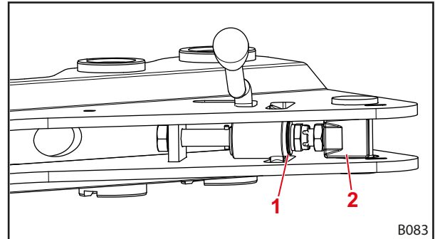
Kuva 63 Etukuormaimen lukituksen näkymä alhaalta päin
