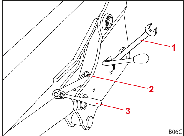
Kuva 57 Työkalun asettaminen paikalleen
