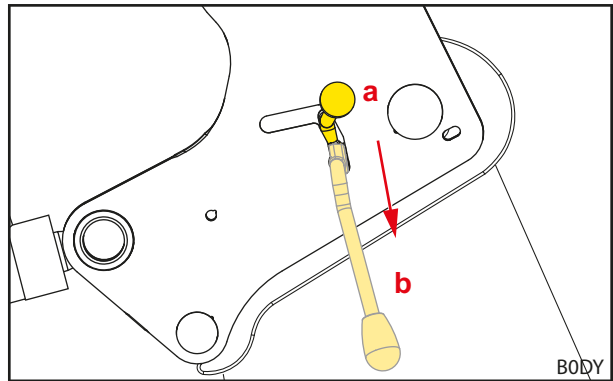
Kuva 58 Lukitusvivun kiristäminen
