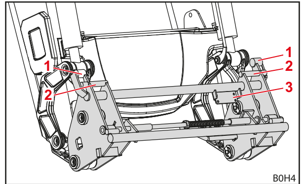
Kuva 12 Yhdistelmävaihtorunko Euro-ALö 3
