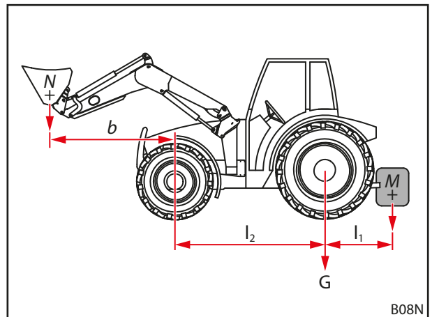
Kuva 49 Staattisen vakauden laskeminen
