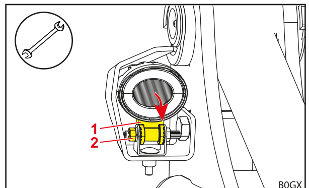
Kuva 45 Etuvalojen säätäminen pystysuunnassa
