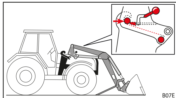
Kuva 51 Traktorin ajaminen aisastoon
