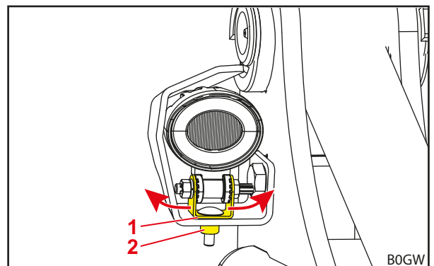
Kuva 44 Etuvalojen säätäminen vaakasuunnassa
