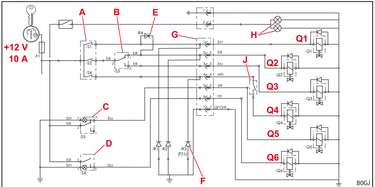
Kuva 137 Sähkökytkentäkaavio (jos varustukseen kuuluu 3. ja 4. ohjauspiiri)
