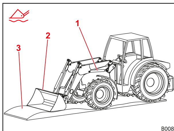
Kuva 29 Etukuormain kelluasennossa
