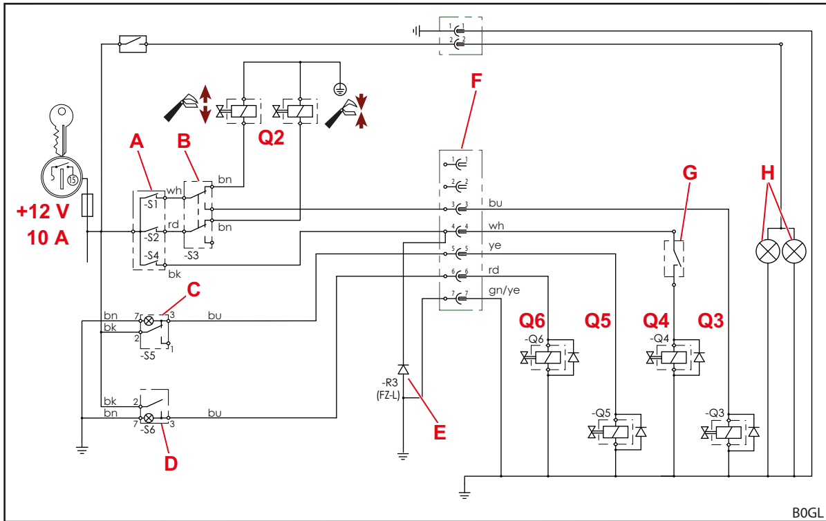
Kuva 138 Sähkökytkentäkaavio (jos varustukseen kuuluu REAL 3 )
