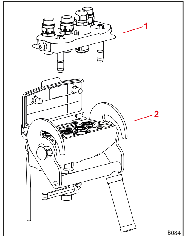
Kuva 20 Hydro-Fix-liitännän rakenne
