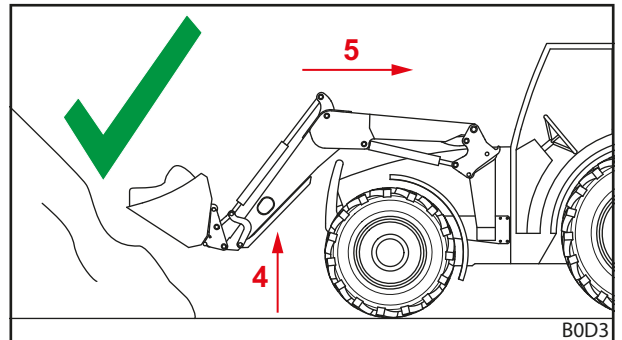
Kuva 116 Taaksepäin ajaminen kuorman kanssa – oikein
