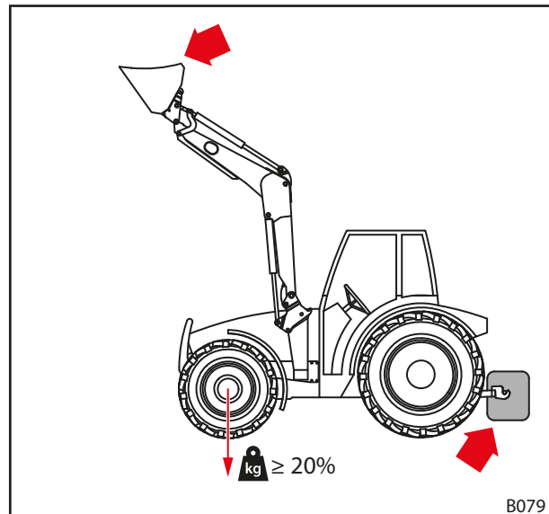
Kuva 48 Kuormitus julkisilla teillä ajettaessa
