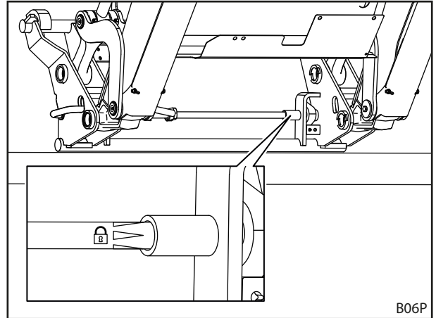
Kuva 85 Tarkasta työkalun lukitus tarran perusteella
