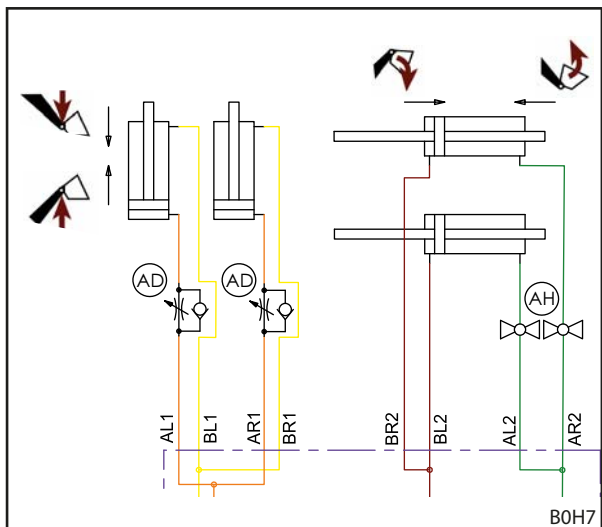
Kuva 136 Hydraulikkapiirustus laskemiskuristin
