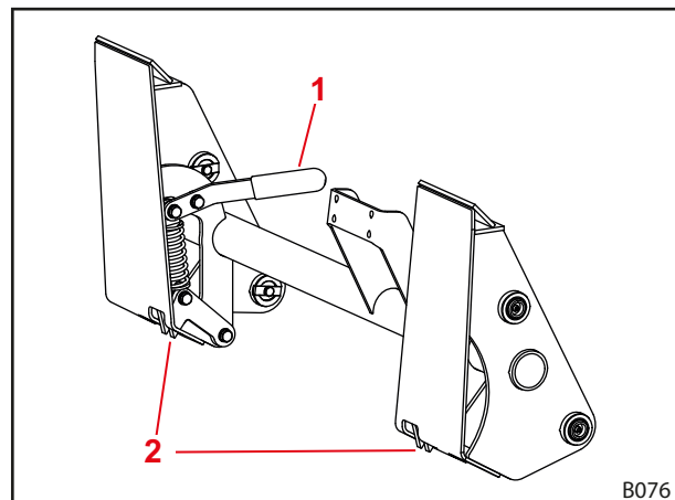
Kuva 88 Skid-Steer-vaihtorungon työkalun lukitus
