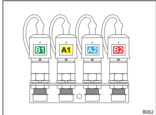
Kuva 17 Pistoliitännät liitettynä
