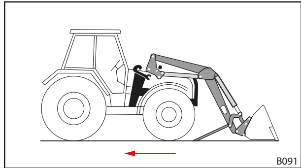
Kuva 129 Traktorin ajaminen takaperin ulos etukuormaimesta
