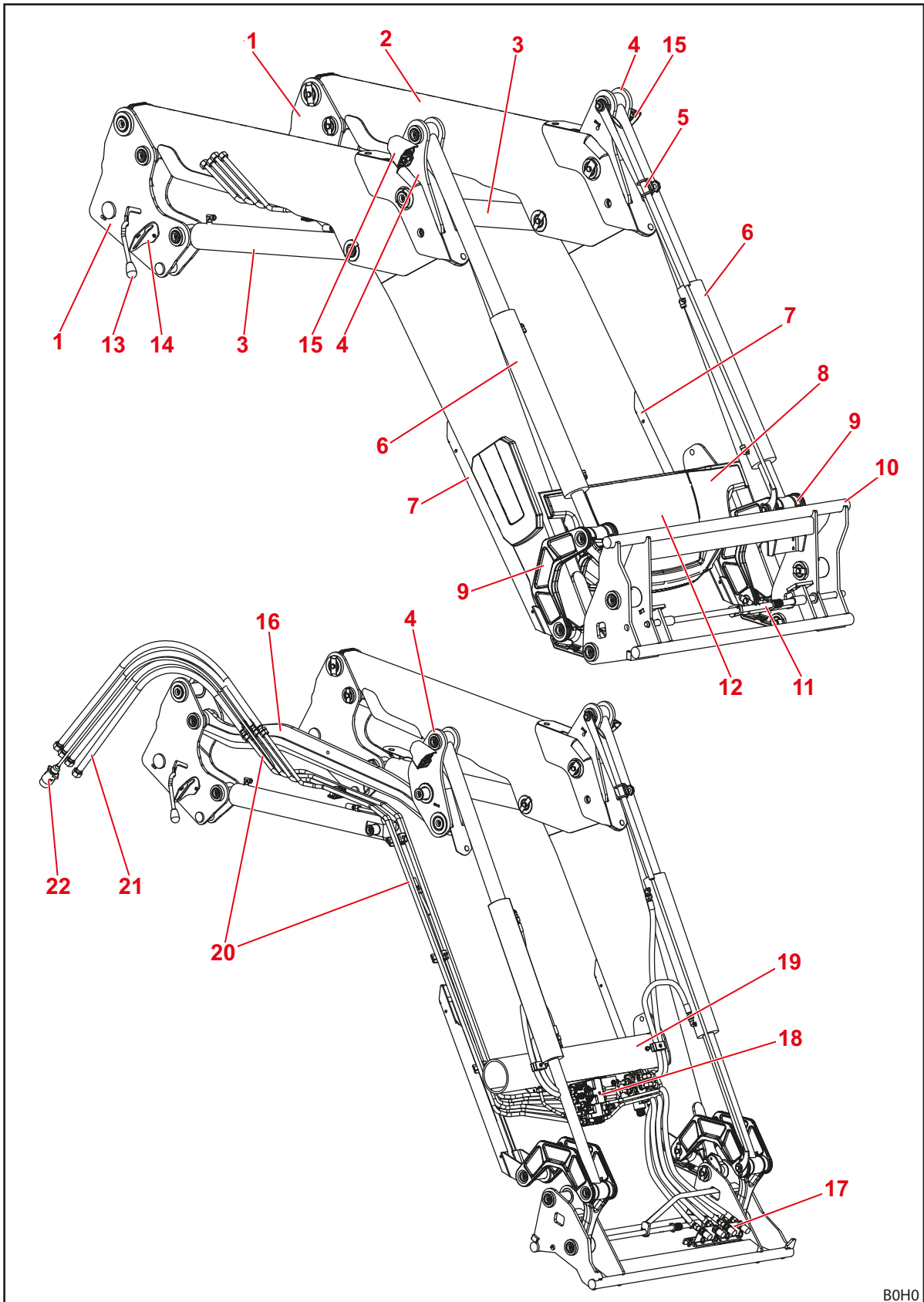
Kuva 8 Etukuormain FZ
