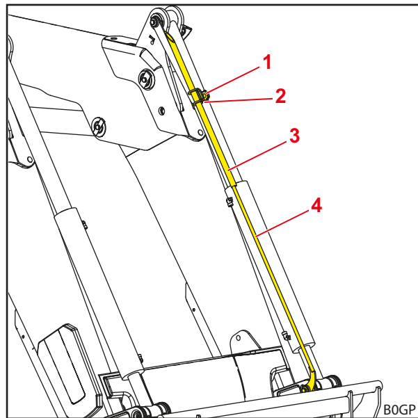
Kuva 30 Työkalun asennon näyttö
