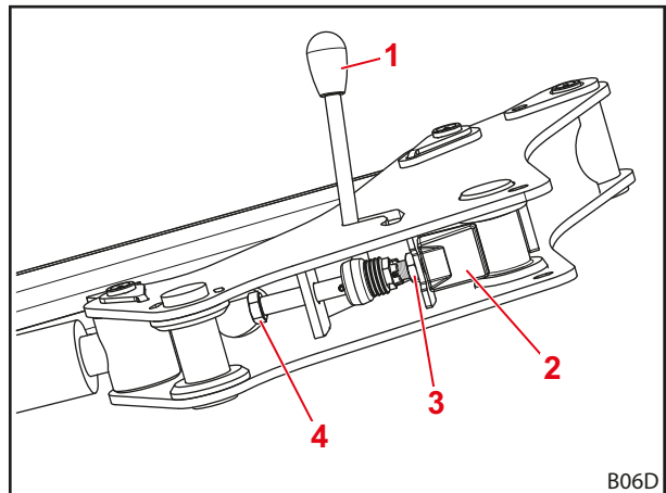
Kuva 59 Etukuormaimen lukituksen näkymä alhaalta päin
