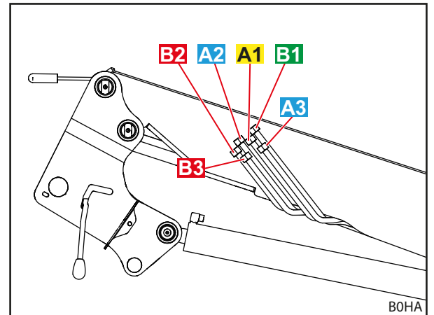
Kuva 16 Hydraulikkalinjat (erikoisvaruste REAL 3 )
