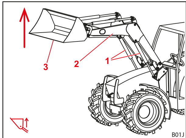
Kuva 25 Nosto-toiminto
