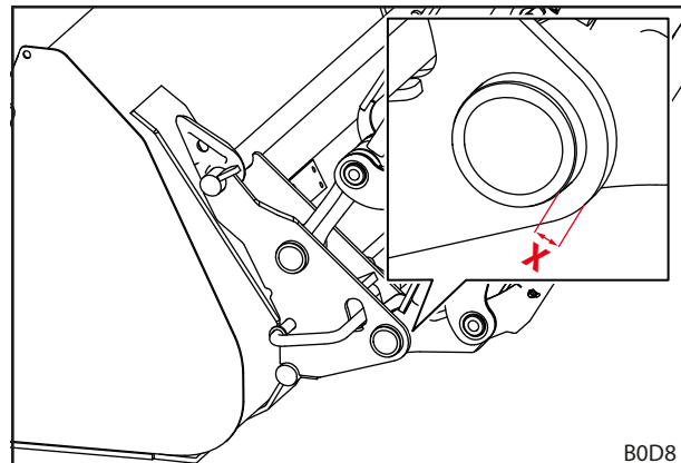
Kuva 124 Vaihtorungon kulumismitta
