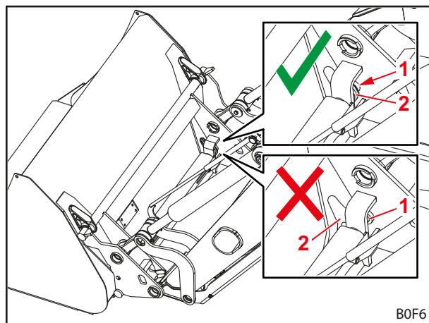
Kuva 93 Lukituspulttien sijainnin tarkastaminen
