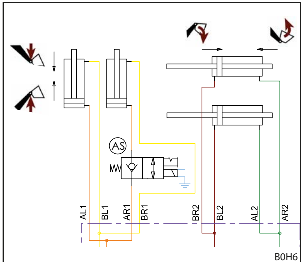
Kuva 135 Hydraulikkapiirustus laskemisen varmistus
