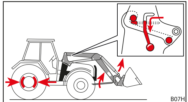
Kuva 54 Taita tukijalat sisään ja sulje etukuormaimen lukitus.
