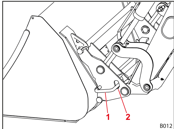
Kuva 84 Mekaaninen työkalun lukitus
