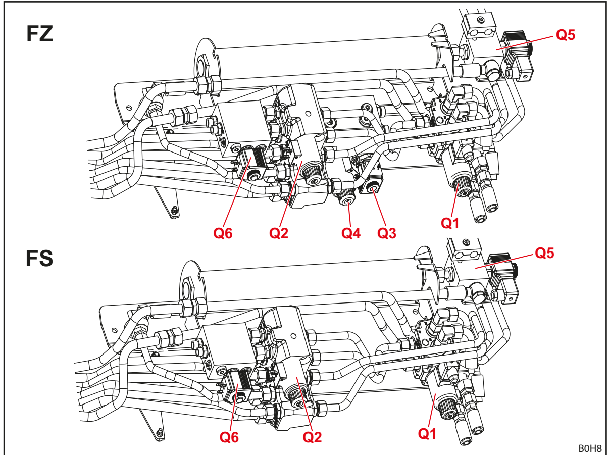
Kuva 139 Lisätoimintojen hydraulikkaventtiilien asettelu
