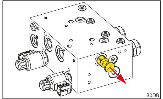
Kuva 76 Vedä REAL 3 -venttiin paineenalennusventtiili ulos
