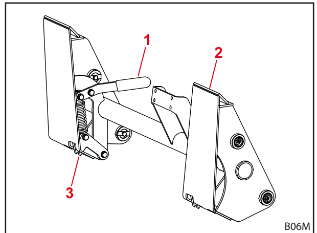
Kuva 24 Skid-Steer-vaihtorungon mekaaninen työkalun lukitus
