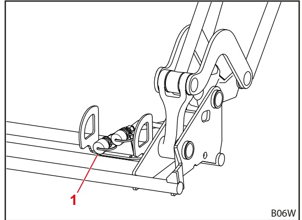
Kuva 37 REAL 3
