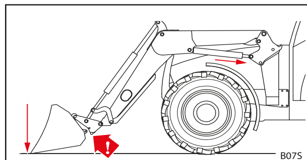
Kuva 89 Paina työkalu maahan
