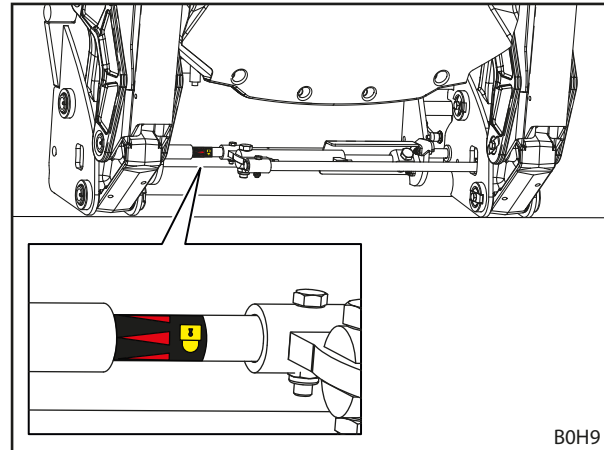
Kuva 92 Tarkasta työkalun lukitus tarran perusteella
