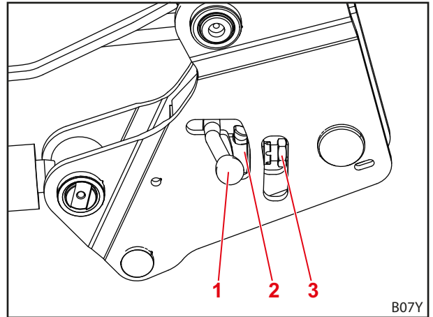
Kuva 60 Etukuormaimen lukituksen avaaminen
