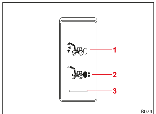
Kuva 77 Comfort-hydrauliikan kytkin
