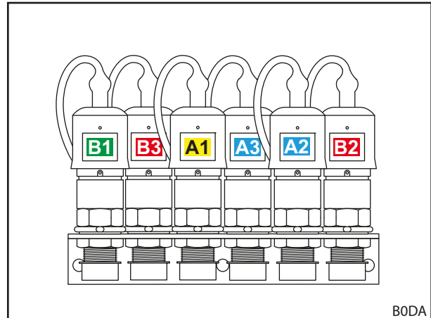
Kuva 18 Pistoliitännät liitettynä (erikoisvaruste REAL 3 )
