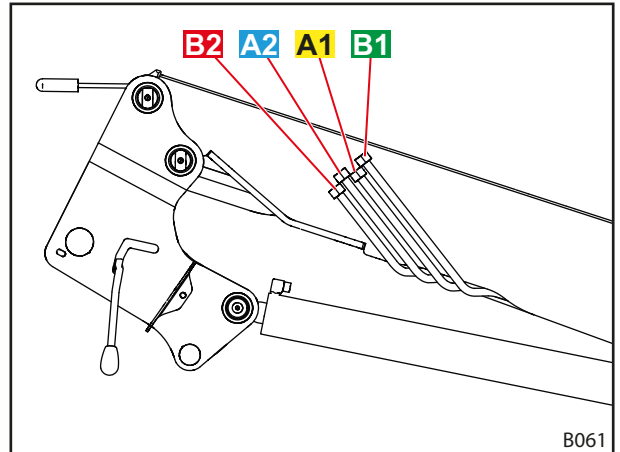
Kuva 15 Hydraulikkalinjat
