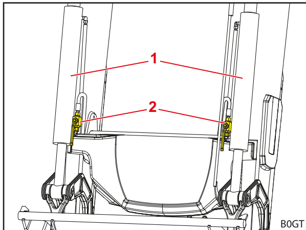
Kuva 42 Sulkuhanat työkalusylinterieissä
