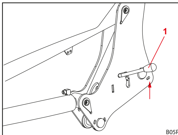
Fig. 53 Ouvrir le verrouillage du chargeur frontal
