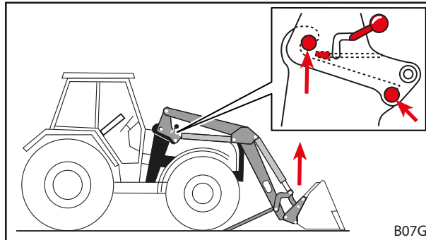
Fig. 50 Utiliser la fonction levage jusqu'à ce que les axes du chargeur frontal se trouvent dans le crochet d'arrêt
