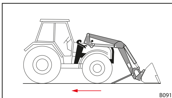
Fig. 118 Reculer le tracteur
