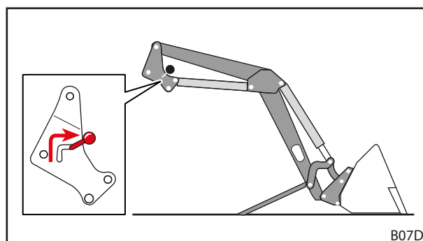
Fig. 46 Ouvrir le verrouillage du chargeur frontal
