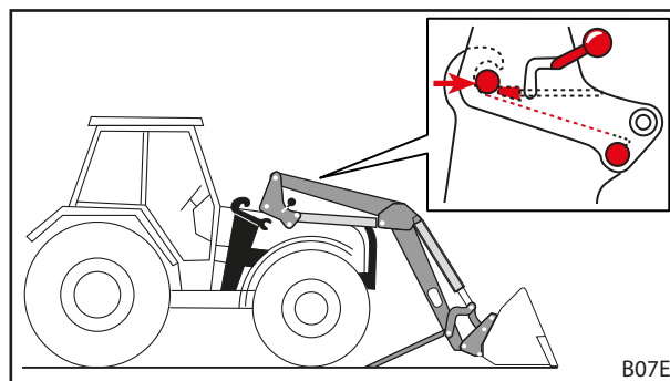
Fig. 47 Avancer le tracteur dans le brancard
