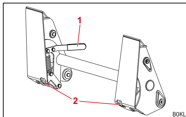
Fig. 14 Cadre porte-outils Skid Steer
