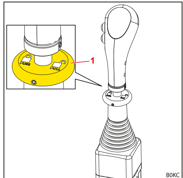
Fig. 61 Verrouillage du levier de commande (verrouillage vertical)
