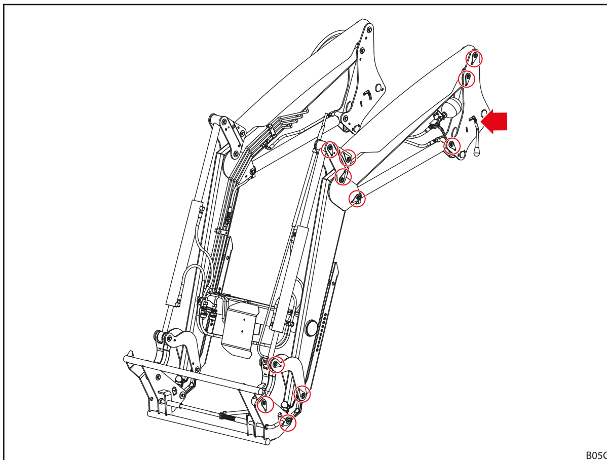
Fig. 110 Points de lubrification P
