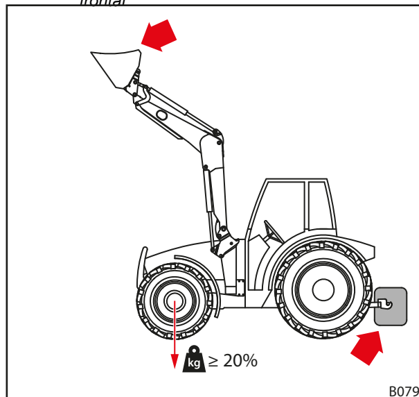
Fig. 44 Charge lors de la conduite sur route
