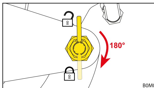
Fig. 35 Mettre le verrou à cran dans la position verrouillée
