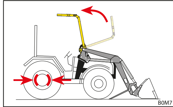
Fig. 49 Relever l'OPG
