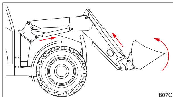
Fig. 92 Déclencher le verrouillage d'outil
