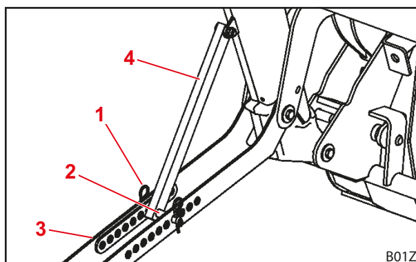
Fig. 71 Béquille
