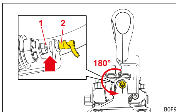
Fig. 65 Levier de commande déverrouillé
