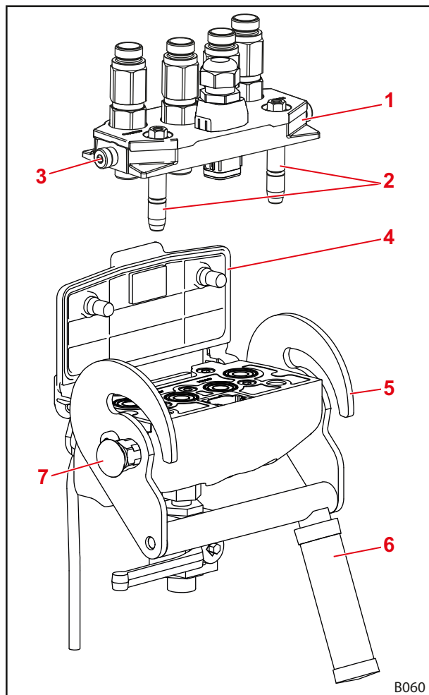
Fig. 74 Hydro-Fix (exemple : Hydro-fix quadruple)
