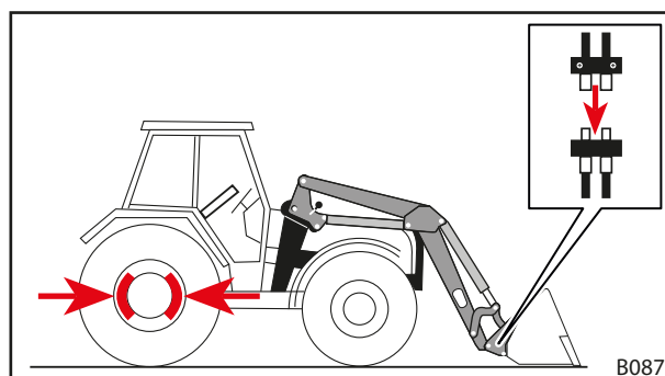
Fig. 93 Relier les conduites hydrauliques de l'outil avec les coupleurs du chargeur frontal
