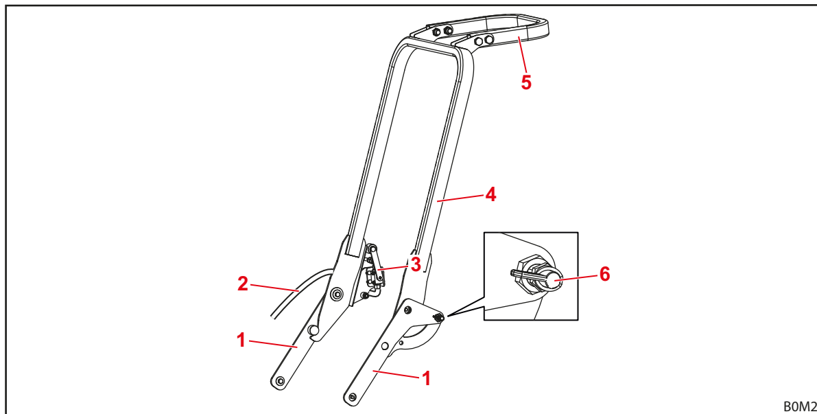
Fig. 11 Operator Protective Guard, OPG (illustration à titre d'exemple)
