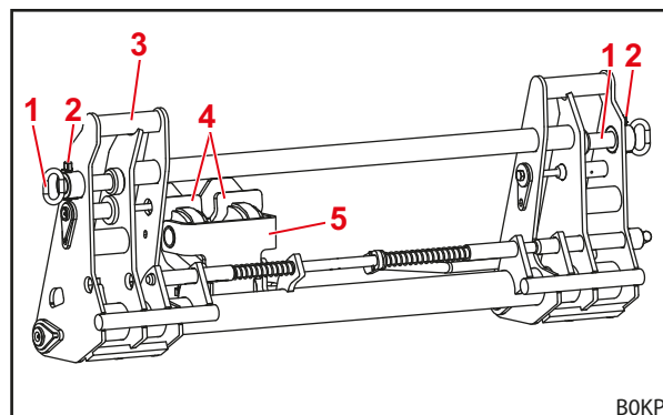
Fig. 18 Cadre porte-outils combiné Euro-FR (préparé pour l'outil Euro)
