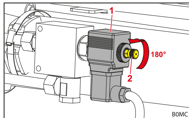
Fig. 33 Ouvrir la vanne
