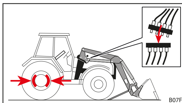
Fig. 48 Arrêter le tracteur et raccorder les conduites hydrauliques
