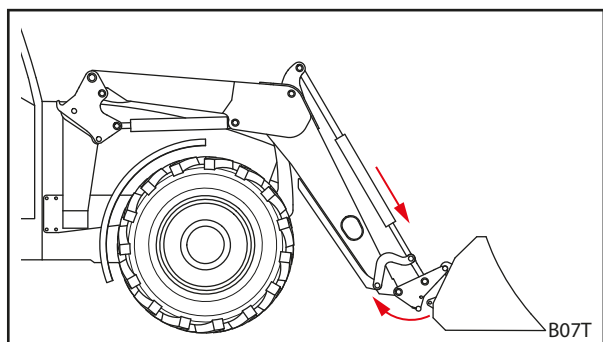
Fig. 100 Décrocher le cadre porte-outils
