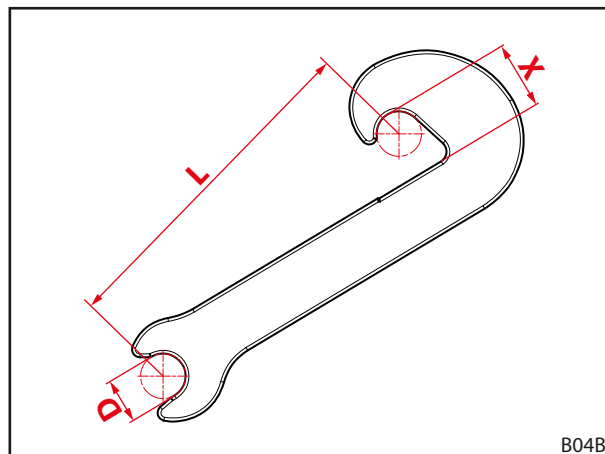
Fig. 111 Cotes d'usure du crochet
