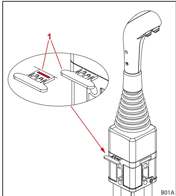
Fig. 60 Verrouillage du levier de commande (verrouillage horizontal)
