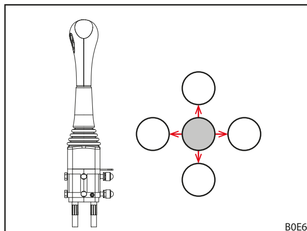
Fig. 62 Mettre tous les leviers de commande en fin de course
