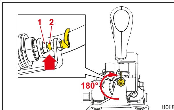
Fig. 64 Levier de commande verrouillé
