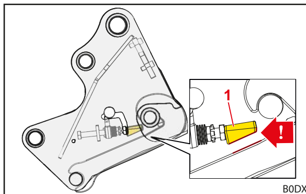
Fig. 52 Position correcte de la cale de serrage
