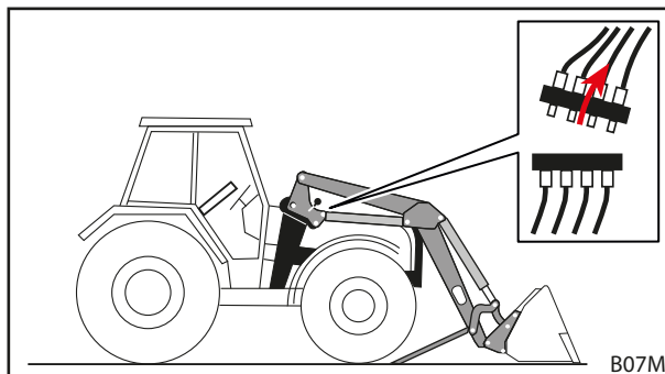
Fig. 117 Découpler le circuit hydraulique
