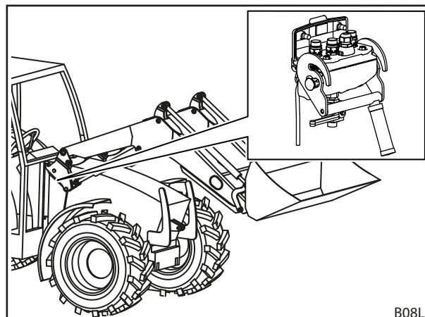
Fig. 22 Hydro-Fix : position sur le chargeur frontal
