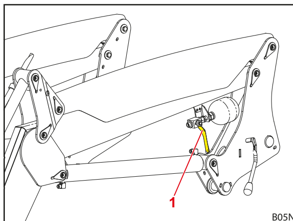
Fig. 40 Comfort-Drive à commande mécanique
