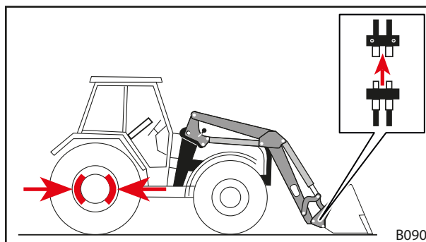
Fig. 99 Détacher les conduites hydrauliques
