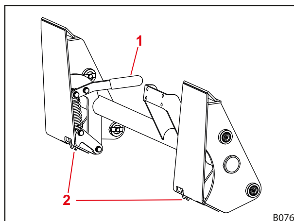
Fig. 80 Verrouillage de l'outil sur le cadre porte-outils Skid Steer
