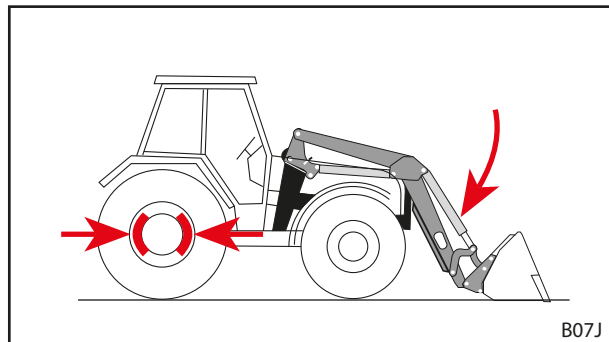
Fig. 114 Serrer le frein d'immobilisation et abaisser le chargeur frontal
