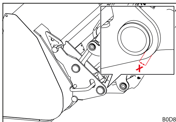
Fig. 113 Cote d'usure du cadre porte-outils
