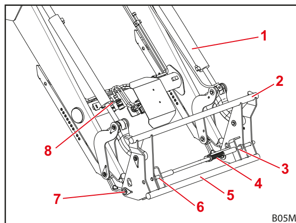
Fig. 13 Cadre porte-outils Euro
