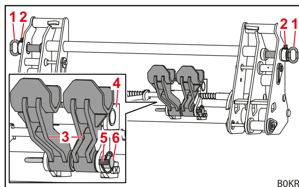
Fig. 86 Adaptateur en position de stationnement (cadre porte-outils préparé pour l'outil Euro)
