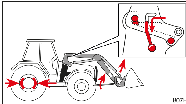
Fig. 51 Replier les béquilles et fermer le verrouillage du chargeur frontal
