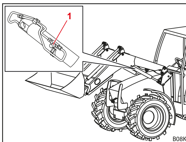
Fig. 41 Clapets limiteurs de descente
