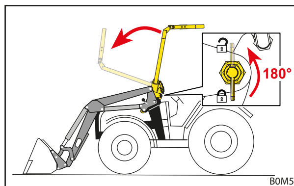
Fig. 34 Abaisser l'OPG
