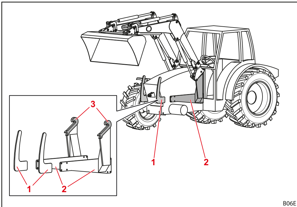
Fig. 12 Jeu de montage pour tracteur
