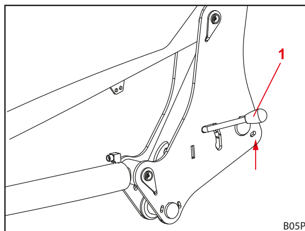
Fig. 112 Vérifier le verrouillage du chargeur frontal
