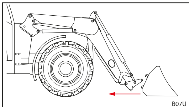
Fig. 101 S'éloigner
