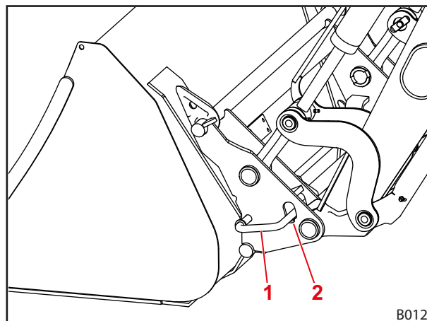
Fig. 75 Verrouillage mécanique de l'outil
