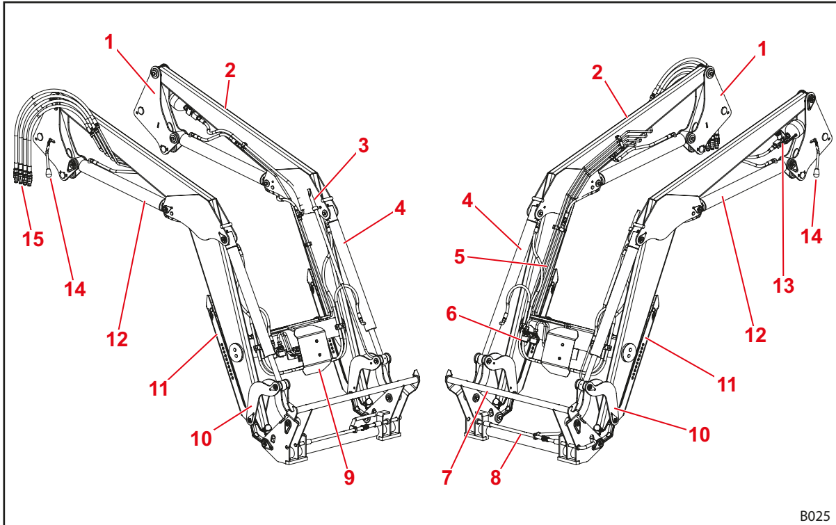
Σχ. 9 Εμπρόσθιος φορτωτής H (χωρίς μηχανικό παράλληλο οδηγό)
