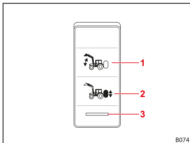
Σχ. 70 Διακόπτης για υδραυλικό σύστημα Comfort
