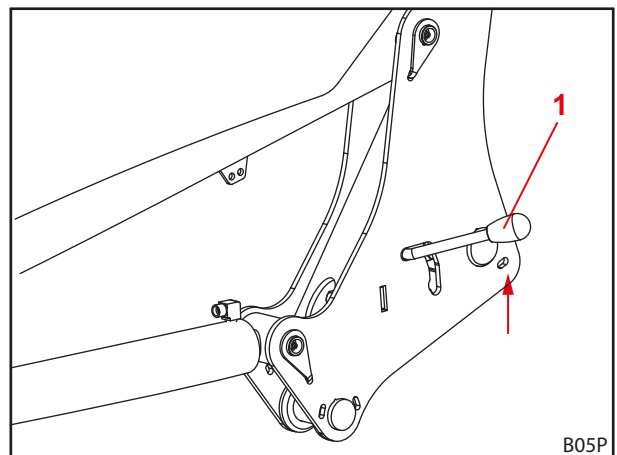
Σχ. 112 Έλεγχος κλειδώματος εμπρόσθιου φορτωτή
