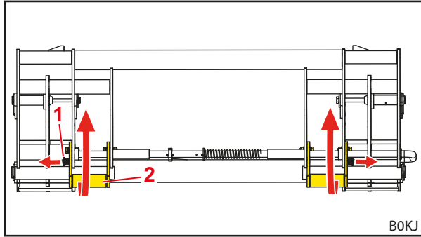
Σχ. 84 Ανέβασμα διατάξεων
