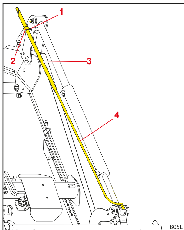
Σχ. 31 Οπτική ένδειξη για ρύθμιση εργαλείου
