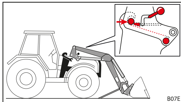
Σχ. 47 Εισαγωγή τρακτέρ στον περιστροφικό βραχίονα
