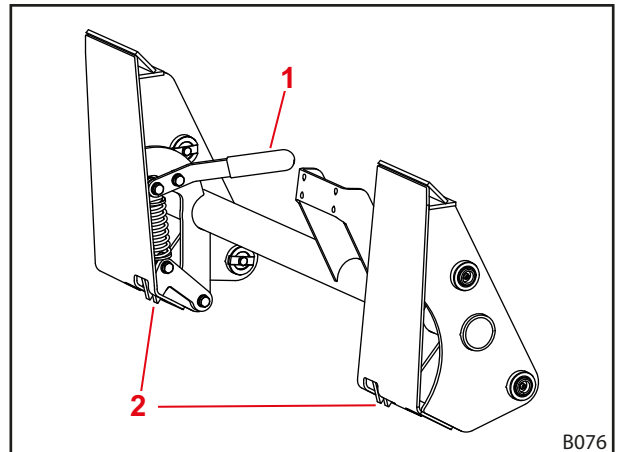
Σχ. 80 Μηχανισμός ασφάλισης εργαλείων στο πλαίσιο εναλλαγής Skid-Steer
