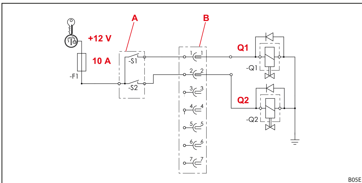
Σχ. 121 Ηλεκτρικό διάγραμμα συνδεσμολογίας
