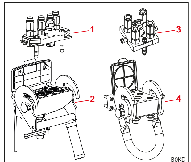
Σχ. 23 Διάταξη Hydro-Fix και πολυσυνδέσμου
