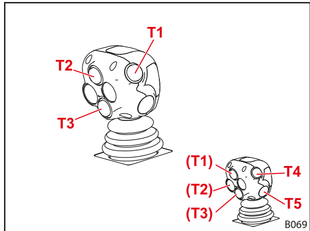
Σχ. 69 STOLL Trac Control (3 μπουτόν)
