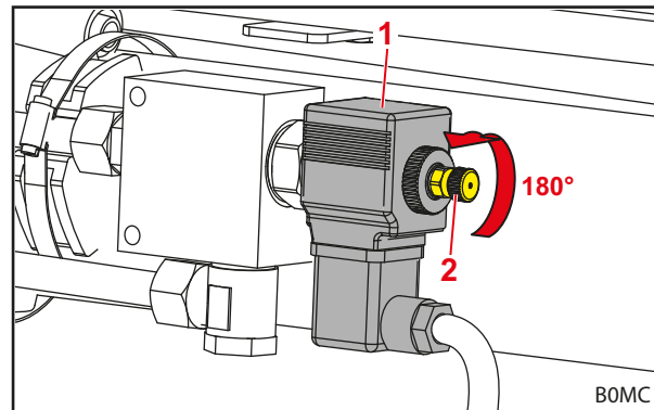
Σχ. 33 Ανοιγμα βαλβίδας
