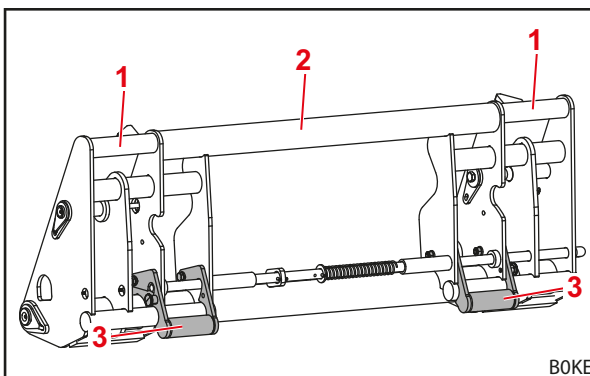
Σχ. 15 Σύνθετο πλαίσιο εναλλαγής Euro-SMS (προετοιμασμένο για εργαλείο Euro)
