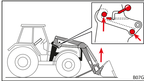
Σχ. 50 Χρήση λειτουργίας ανύψωσης, μέχρι να εφαρμόσουν οι πείροι του εμπρόσθιου φορτωτή στα άγκιστρα.
