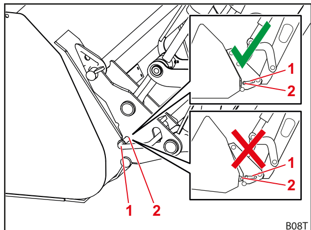
Σχ. 78 Έλεγχος θέσης πείρων ασφάλισης
