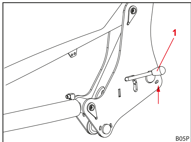
Σχ. 53 Ανοίγμα κλειδώματος εμπρόσθιου φορτωτή
