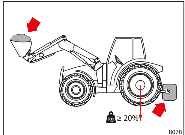
Σχ. 43 Φορτίο σε εργασίες με τον εμπρόσθιο φορτωτή
