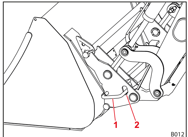
Σχ. 75 Μηχανικός μηχανισμός ασφάλισης εργαλείων
