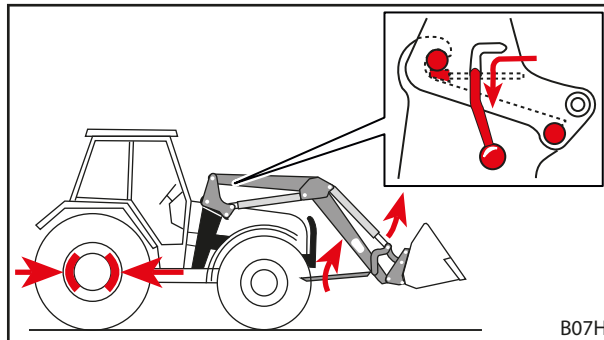
Σχ. 51 Κλείσιμο στηριγμάτων στάθμευσης και κλείσιμο κλειδώματος εμπρόσθιου φορτωτή
