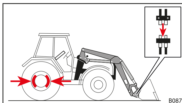
Σχ. 93 Σύνδεση υδραυλικών αγωγών εργαλείου με τους συνδέσμους του εμπρόσθιου φορτωτή
