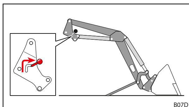
Σχ. 46 Άνοιγμα κλειδώματος εμπρόσθιου φορτωτή
