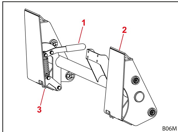
Σχ. 25 Μηχανικός μηχανισμός ασφάλισης εργαλείων στα πλαίσια εναλλαγής Skid-Steer
