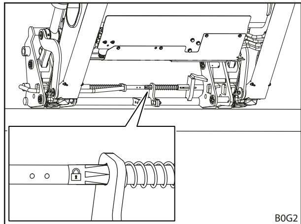
Σχ. 77 Έλεγχος μηχανισμού ασφάλισης εργαλείων με τη βοήθεια του αυτοκόλλητου (σύνθετο πλαίσιο εναλλαγής Euro-FR)
