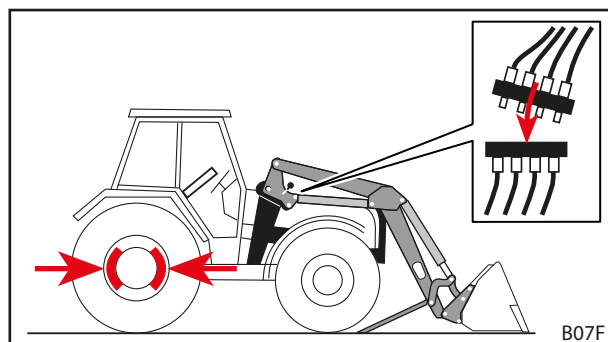
Σχ. 48 Απενεργοποιήστε το τρακτέρ και συνδέστε τους υδραυλικούς αγωγούς
