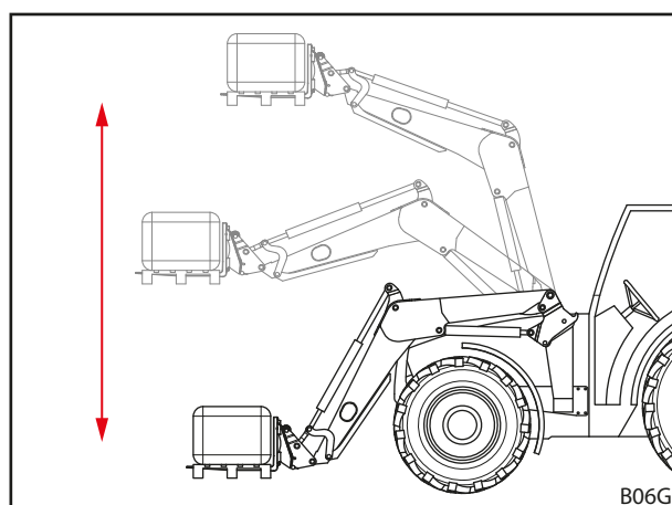
Σχ. 32 Μηχανικός παράλληλος οδηγός
