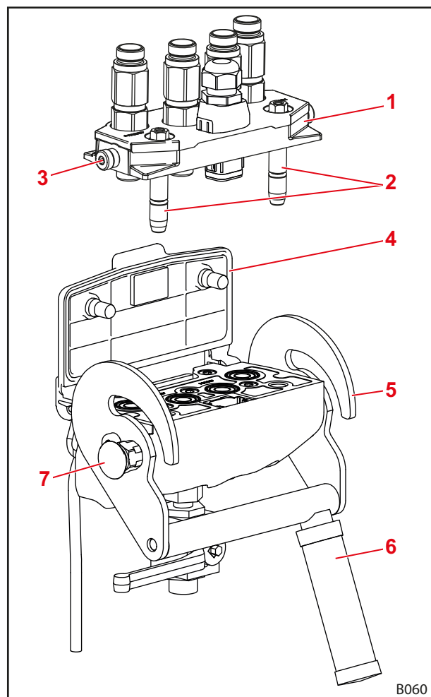
Σχ. 74 Hydro-Fix (παράδειγμα: Hydro-Fix 4-πλός)
