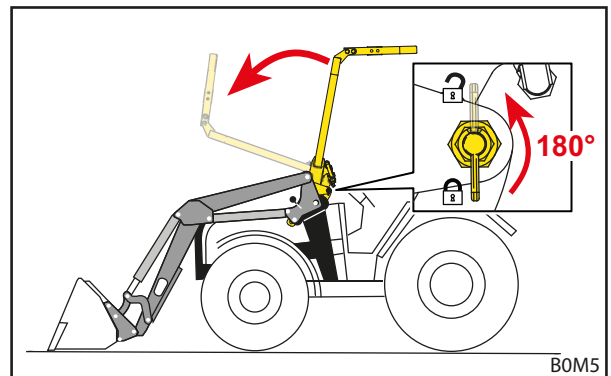
Σχ. 34 Κατέβασμα OPG
