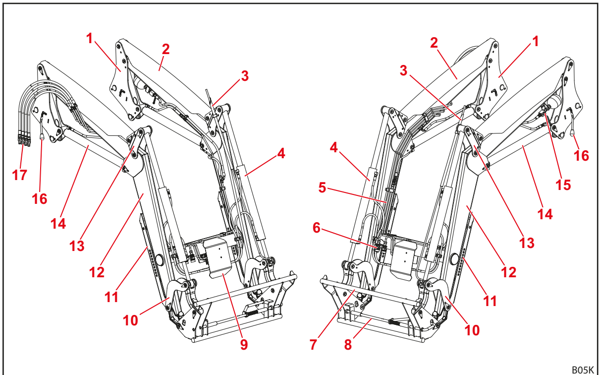
Σχ. 10 Εμπρόσθιος φορτωτής P (με μηχανικό παράλληλο οδηγό)
