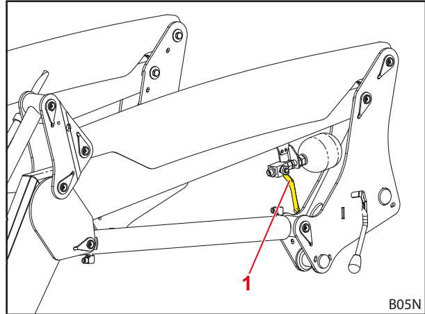
Σχ. 40 Μηχανικά ενεργοποιούμενο Comfort-Drive
