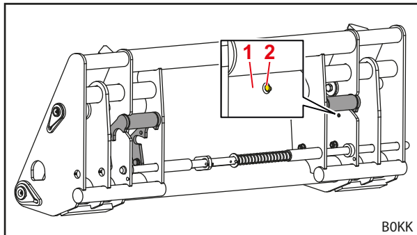
Σχ. 85 Ανεβασμένες διατάξεις (πίσω όψη)
