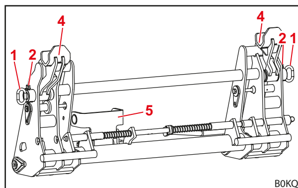
Σχ. 19 Σύνθετο πλαίσιο εναλλαγής Euro-FR (προετοιμασμένο για εργαλείο FR)
