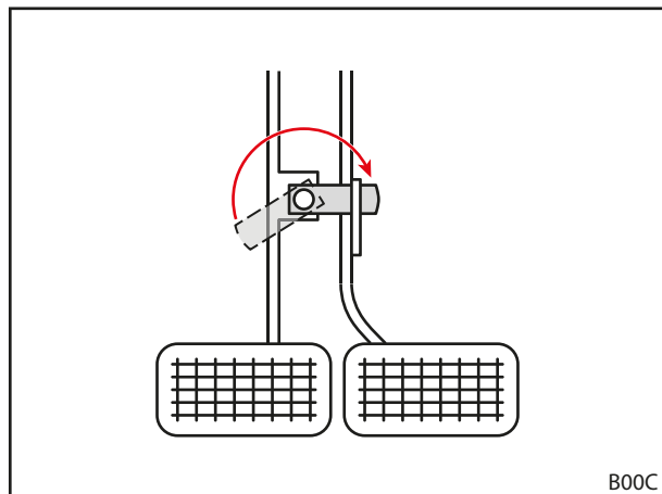
Σχ. 42 Σύνδεση πεντάλ φρένων
