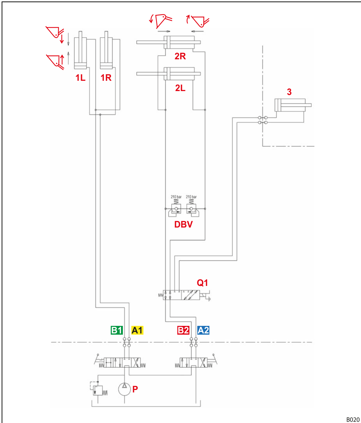
Σχ. 120 Υδραυλικό σχέδιο P
