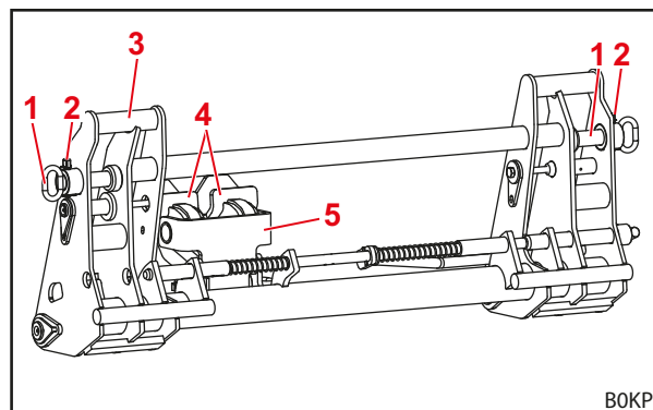
Σχ. 18 Σύνθετο πλαίσιο εναλλαγής Euro-FR (προετοιμασμένο για εργαλείο Euro)
