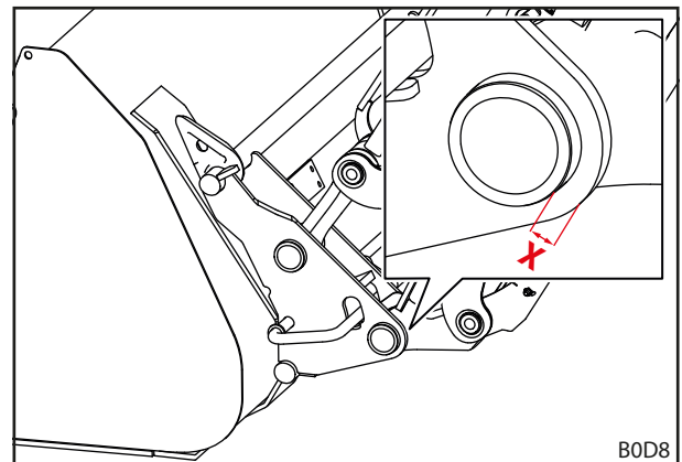
Σχ. 113 Βαθμός φθοράς του πλαισίου εναλλαγής
