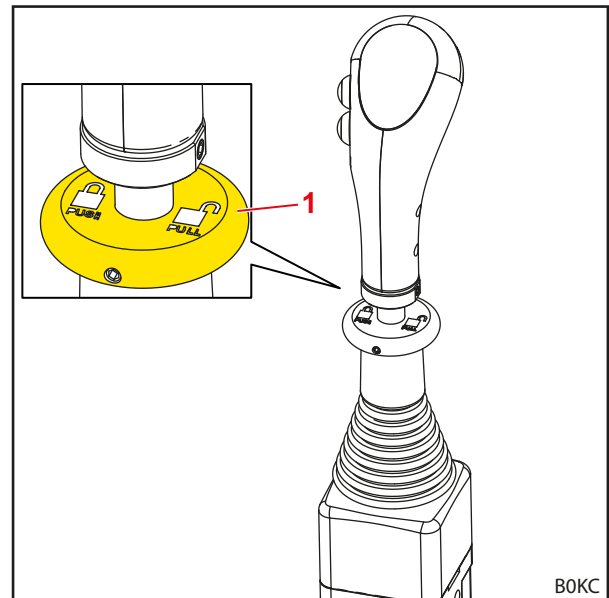
Σχ. 61 Ασφάλιση του μοχλού χειρισμού (κάθετος μηχανισμός ασφάλισης)
