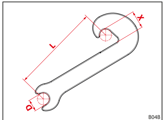
Σχ. 111 Διαστάσεις φθοράς του άγκιστρου
