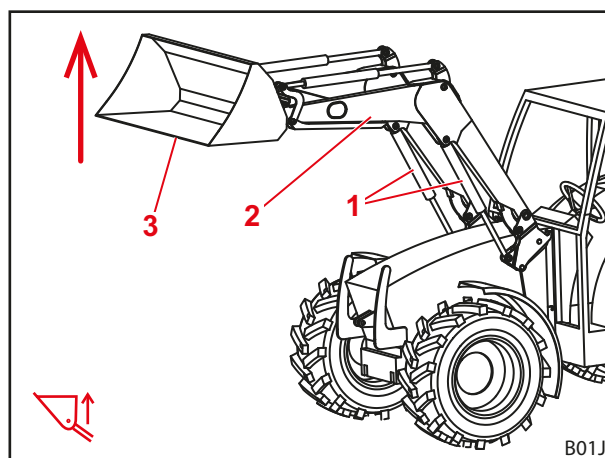
Σχ. 26 Λειτουργία ανύψωσης
