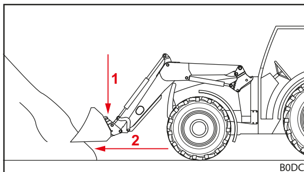
Σχ. 107 Κατεβάστε τον εμπρόσθιο φορτωτή και οδηγήστε σε ευθεία προς το φορτίο
