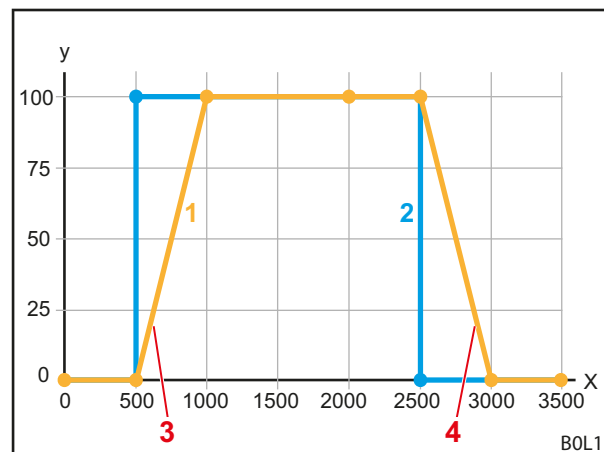
Σχ. 31 Ρυθμιζόμενη συμπεριφορά απόκρισης
