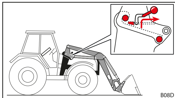
Σχ. 121 Λύσιμο κλειδώματος εμπρόσθιου φορτωτή
