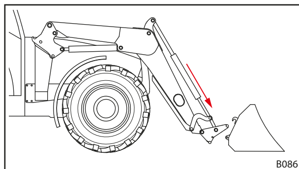
Σχ. 94 Ρύθμιση θέσης περιστροφικού βραχίονα
