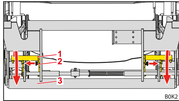
Σχ. 86 Κατέβασμα διατάξεων
