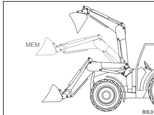
Σχ. 30 Επιστροφή στη θέση
