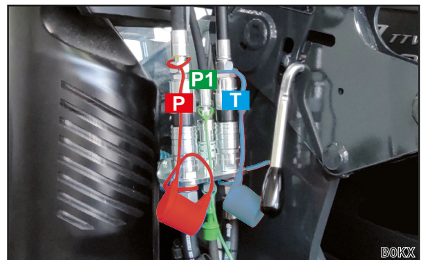
Σχ. 17 Συνδεδεμένοι κουμπωτοί σύνδεσμοι
