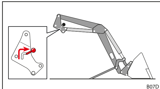
Σχ. 52 Άνοιγμα κλειδώματος εμπρόσθιου φορτωτή
