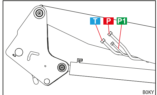
Σχ. 16 Υδραυλικοί σωλήνες
