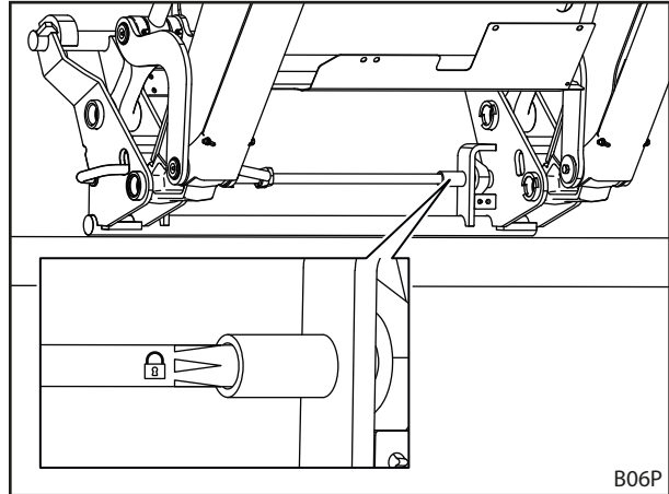
Σχ. 77 Έλεγχος μηχανισμού ασφάλισης εργαλείων με τη βοήθεια του αυτοκόλλητου
