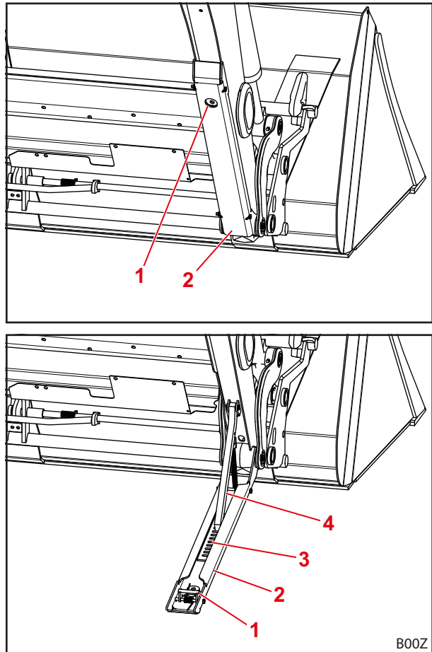
Σχ. 70 Στήριγμα στάθμευσης
