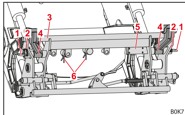
Σχ. 14 Σύνθετο πλαίσιο εναλλαγής Euro-MX (προετοιμασμένο για εργαλείο MX)
