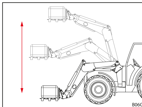
Σχ. 41 Μηχανικός παράλληλος οδηγός
