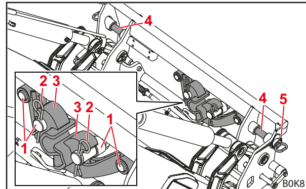
Σχ. 91 Προσαρμογείς σε θέση στάσης (πλαίσιο εναλλαγής προετοιμασμένο για εργαλείο Euro)
