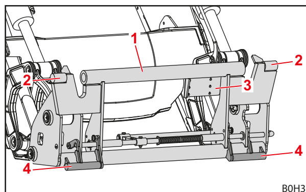
Σχ. 11 Σύνθετο πλαίσιο εναλλαγής Euro-SMS (προετοιμασμένο για εργαλείο Euro)
