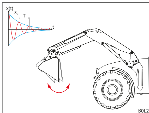
Σχ. 34 Ανακίνηση κουβά
