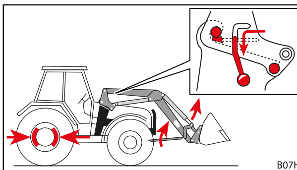
Σχ. 56 Κλείσιμο στηριγμάτων στάθμευσης και κλείσιμο κλειδώματος εμπρόσθιου φορτωτή
