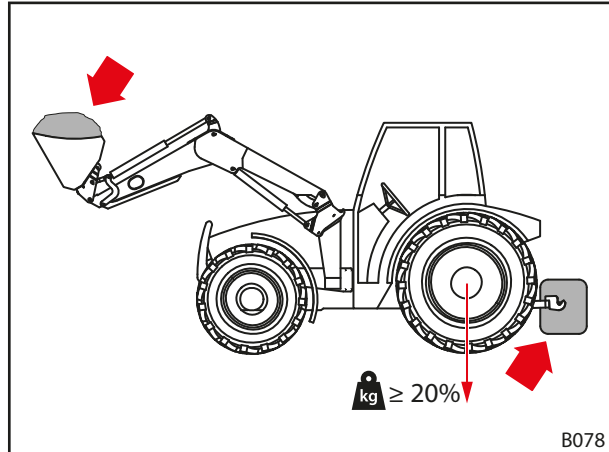
Σχ. 49 Φορτίο σε εργασίες με τον εμπρόσθιο φορτωτή
