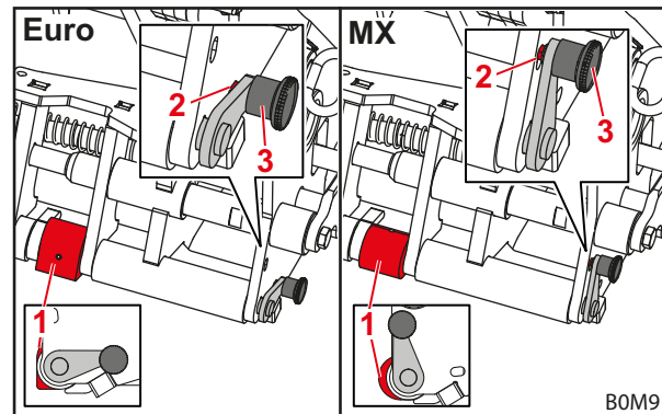
Σχ. 90 Θέση του μίνι πείρου κλειδώματος
