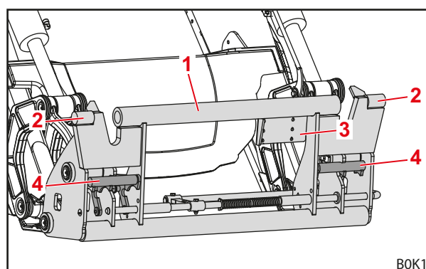
Σχ. 12 Σύνθετο πλαίσιο εναλλαγής Euro-SMS (προετοιμασμένο για εργαλείο SMS)
