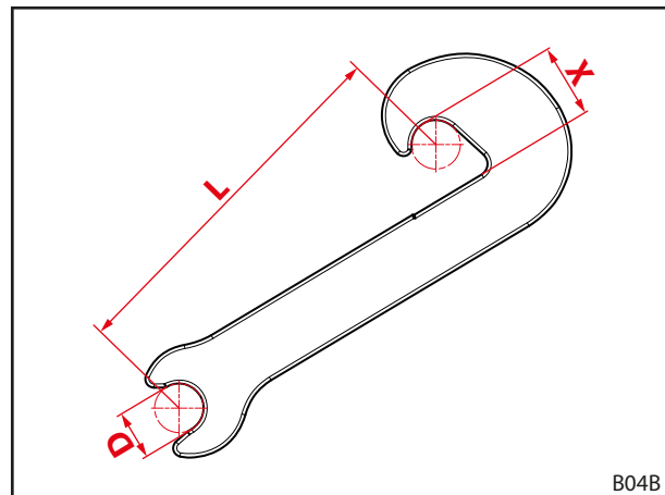
Σχ. 115 Διαστάσεις φθοράς του άγκιστρου
