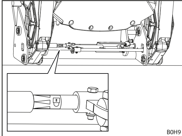
Σχ. 82 Έλεγχος μηχανισμού ασφάλισης εργαλείων με τη βοήθεια του αυτοκόλλητου
