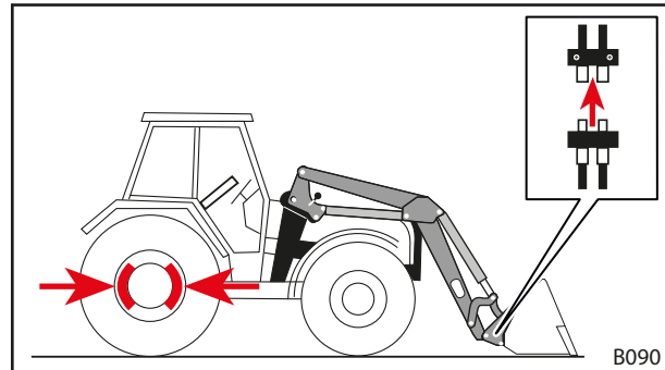
Σχ. 102 Λύσιμο υδραυλικών αγωγών
