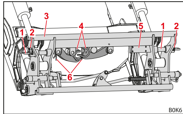
Σχ. 13 Σύνθετο πλαίσιο εναλλαγής Euro-MX (προετοιμασμένο για εργαλείο Euro)
