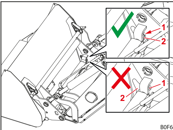
Σχ. 84 Έλεγχος θέσης πείρων ασφάλισης
