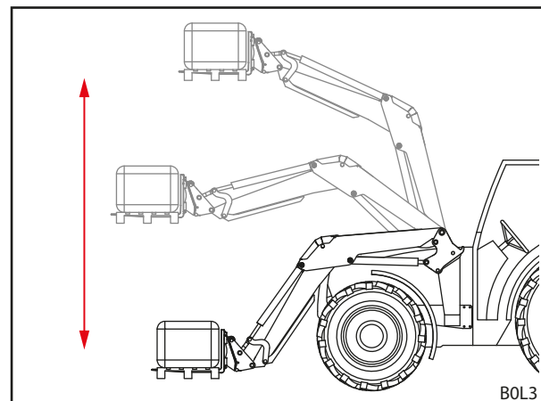
Σχ. 27 Ηλεκτρονικός παράλληλος οδηγός
