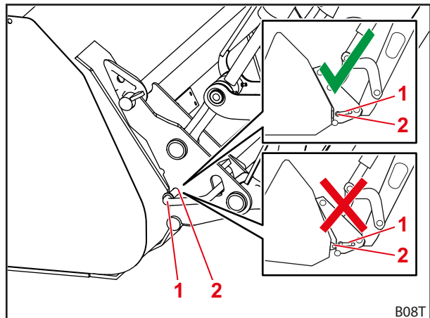
Σχ. 79 Έλεγχος θέσης πείρων ασφάλισης
