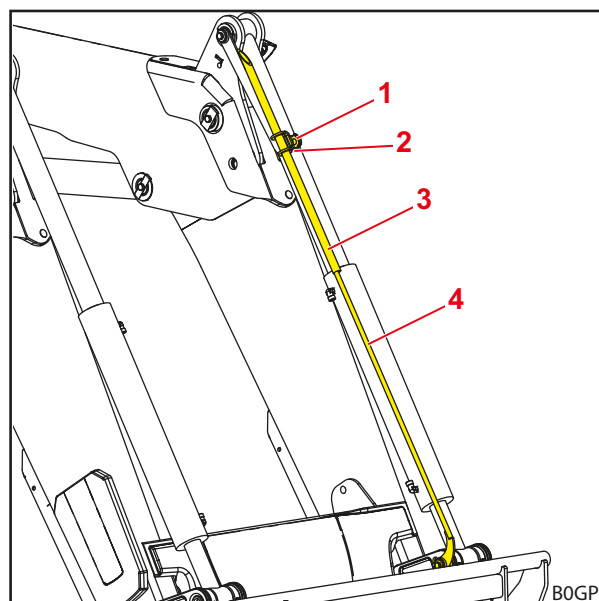
Σχ. 40 Οπτική ένδειξη για τη θέση του εργαλείου
