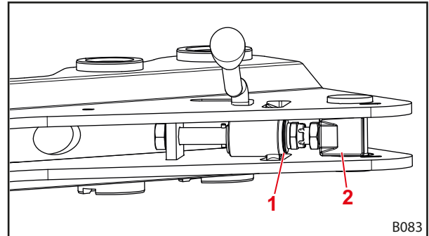
Σχ. 65 Όψη του κλειδώματος του εμπρόσθιου φορτωτή από κάτω
