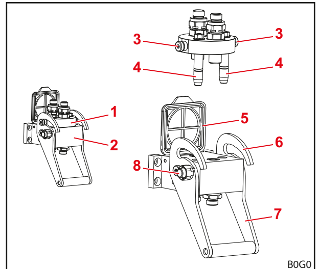
Σχ. 21 Διάταξη στερέωσης εργαλείων
