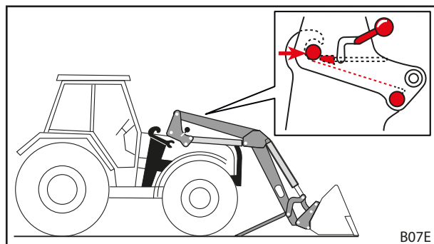
Σχ. 53 Εισαγωγή τρακτέρ στον περιστροφικό βραχίονα
