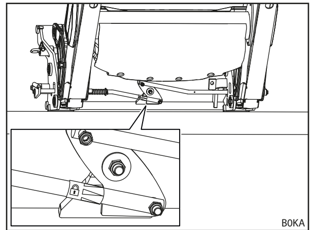
Σχ. 78 Έλεγχος μηχανισμού ασφάλισης εργαλείων με τη βοήθεια του αυτοκόλλητου (σύνθετο πλαίσιο εναλλαγής Euro-MX)
