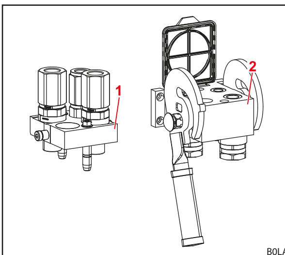
Σχ. 19 Διάταξη Hydro-Fix
