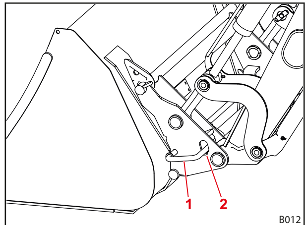
Σχ. 76 Μηχανικός μηχανισμός ασφάλισης εργαλείων
