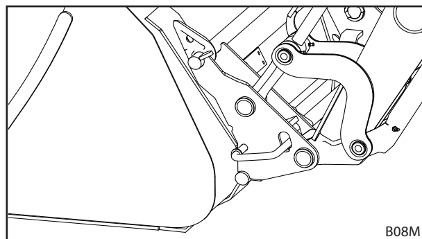
Σχ. 93 Ανοίγμα μηχανισμού ασφάλισης εργαλείου
