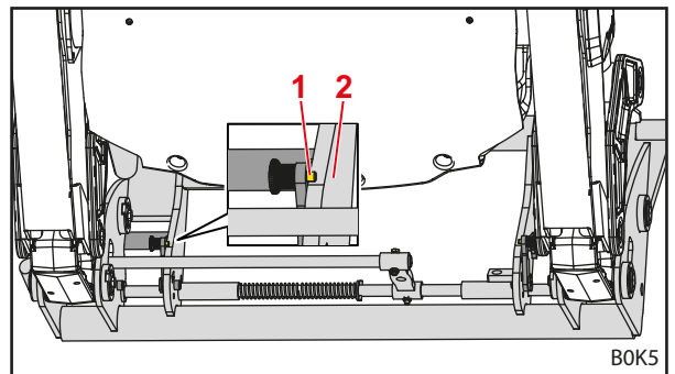
Σχ. 89 Ανεβασμένες διατάξεις (πίσω όψη)
