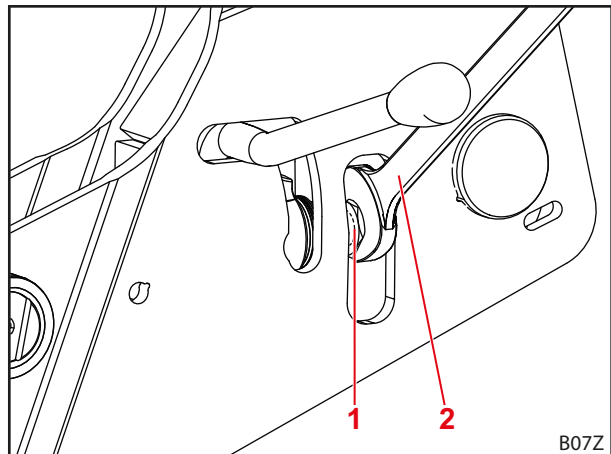
Σχ. 66 Σφίξτε το κόντρα παξιμάδι
