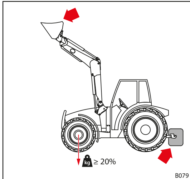
Σχ. 50 Φορτίο σε διαδρομές στον δρόμο
