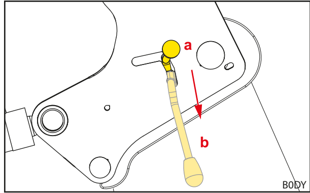
Σχ. 60 Διαδικασία σύσφιξης του μοχλού ασφάλισης
