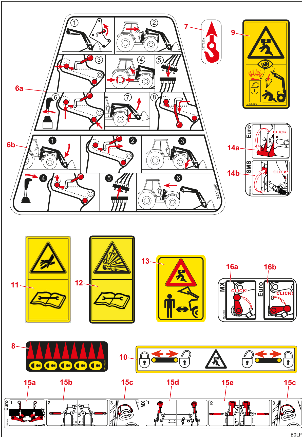
Σχ. 6 Αυτοκόλλητα ασφαλείας θέση 6-16
