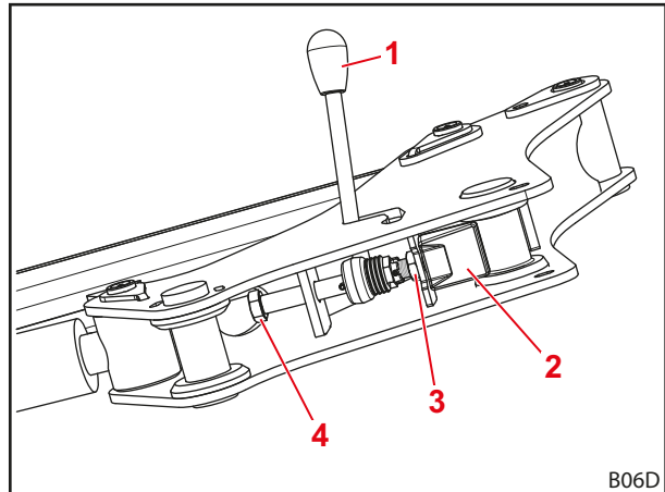
Σχ. 61 Όψη του κλειδώματος του εμπρόσθιου φορτωτή από κάτω
