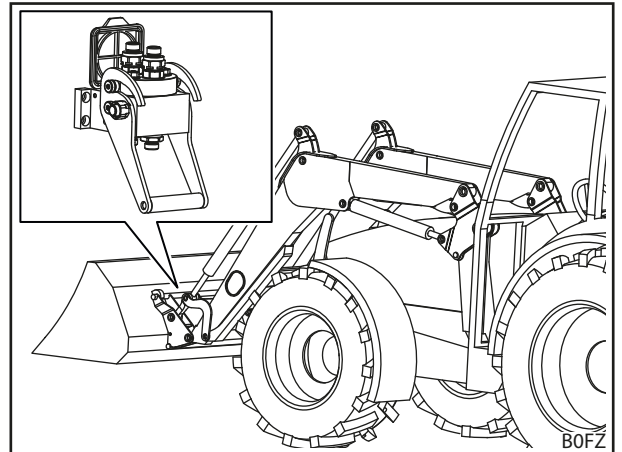
Σχ. 20 Στερέωση εργαλείων: Θέση στον εμπρόσθιο φορτωτή
