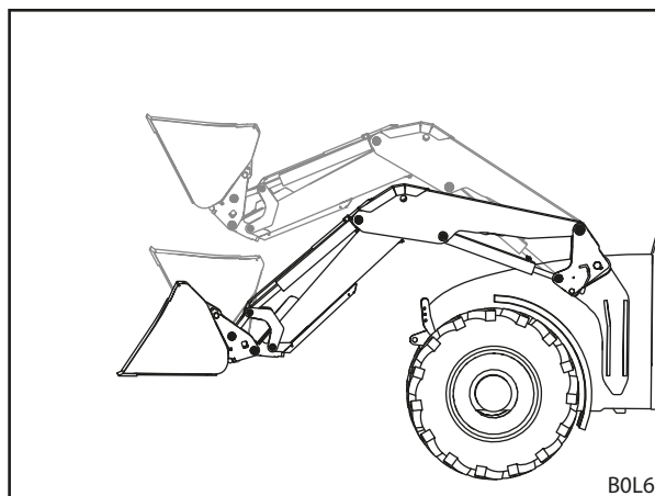
Σχ. 38 Κύκλος κίνησης
