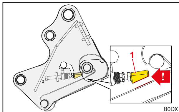
Σχ. 57 Σωστή θέση τοποθέτησης της σφήνας σύσφιξης
