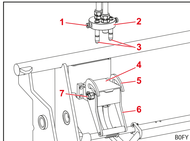
Σχ. 74 Αποσυνδεδεμένη στερέωση εργαλείων
