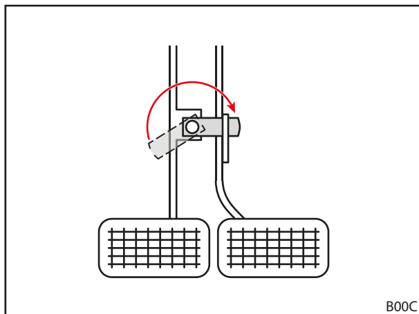
Σχ. 48 Σύνδεση πεντάλ φρένων
