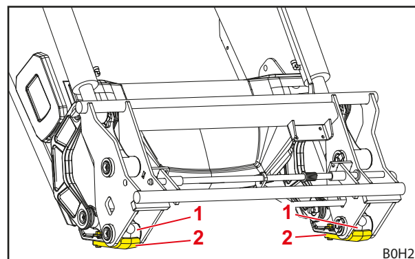
Σχ. 15 Πέδιλα φθοράς
