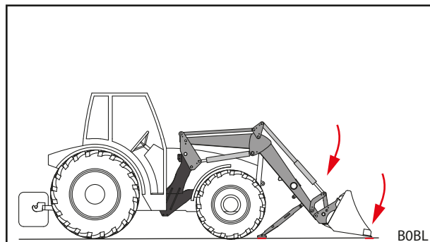
Fig. 102 Frontlader neerlaten en werktuig storten
