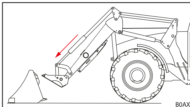
Fig. 69 Arm positioneren
