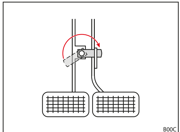
Fig. 33 Rempedalen verbinden
