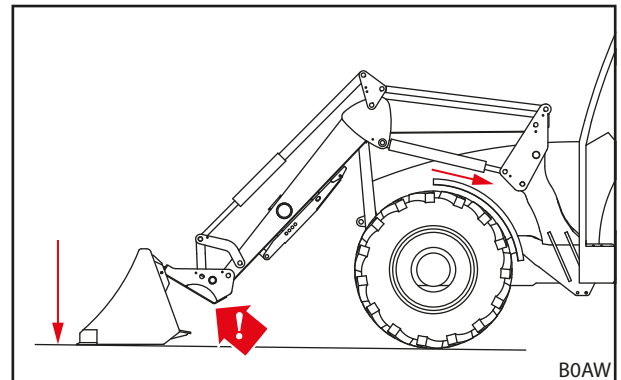
Fig. 66 Werktuig op de bodem drukken
