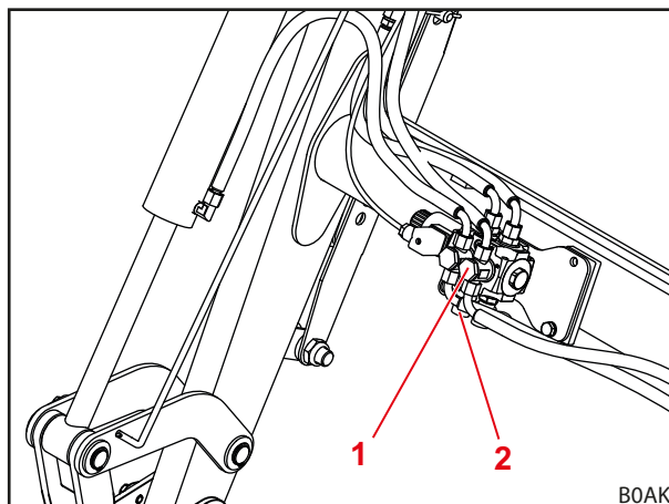
Fig. 30 Bijkomende 3e stuurkring
