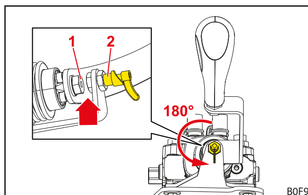
Fig. 49 Ontgrendelde bedieningshendel
