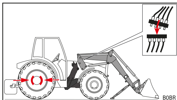
Fig. 103 Hydraulica afkoppelen
