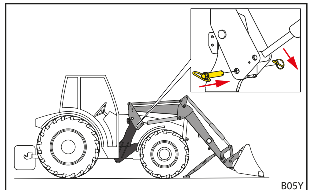
Fig. 40 Vergrendelingspen aanbrengen en met borgpen beveiligen
