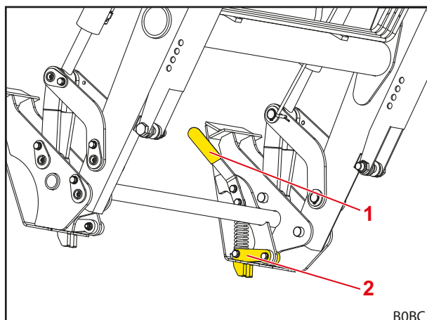
Fig. 62 Mechanische werktuigvergrendeling Skid-Steer (vergrendelde toestand zonder werktuig)
