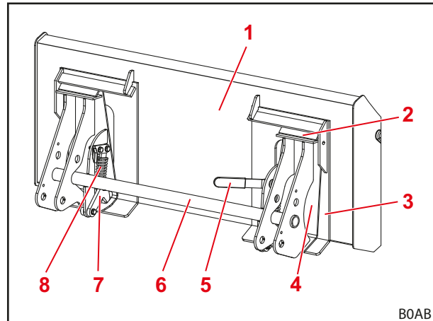
Fig. 20 Geopende vergrendeling
