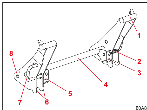
Fig. 64 Werktuigvergrendeling aan het Euro-wisselframe
