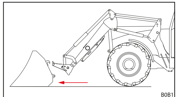
Fig. 74 Benaderen
