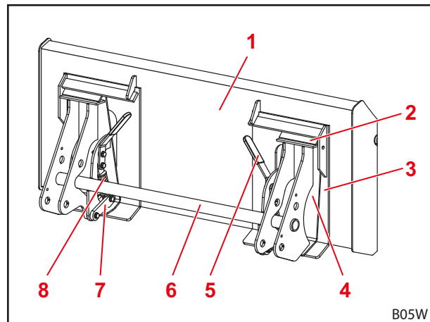
Fig. 21 Gesloten vergrendeling
