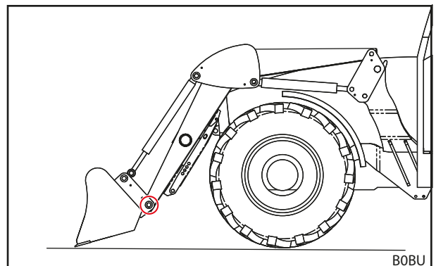
Fig. 89 Onderste pen uittrekken
