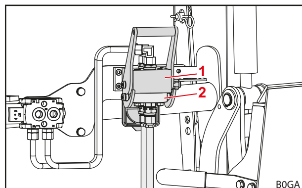
Fig. 57 Aangekoppeld werktuig-fix
