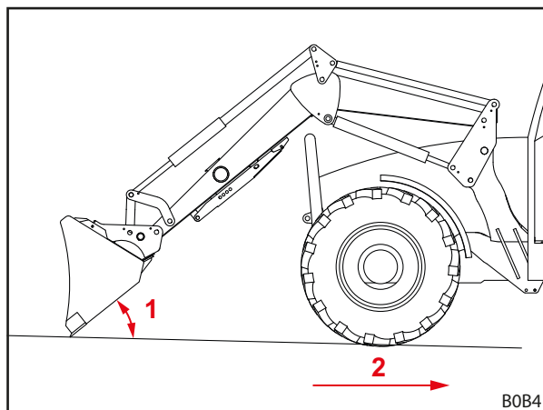
Fig. 91 Achteruit egaliseren
