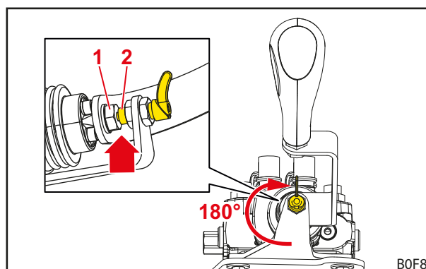
Fig. 48 Vergrendelde bedieningshendel
