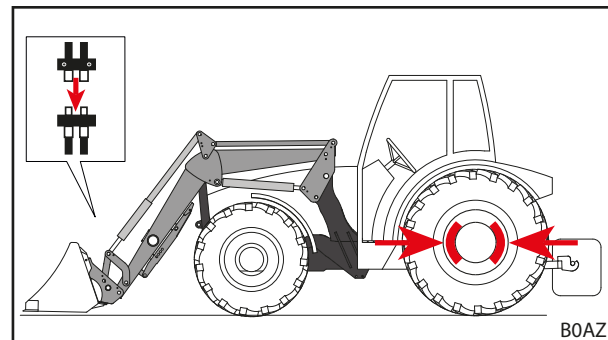
Fig. 77 Stuurkring aankoppelen
