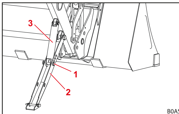
Fig. 52 Parkeersteun uitgeklaapt
