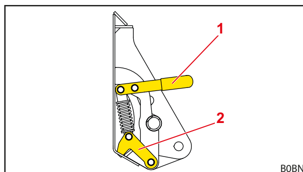
Fig. 58 Mechanische werktuivergrendeling Skid-Steer (geopende toestand)
