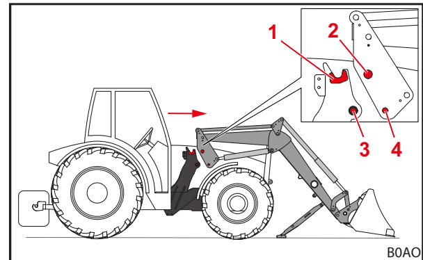
Fig. 38 Tractor in de arm rijden
