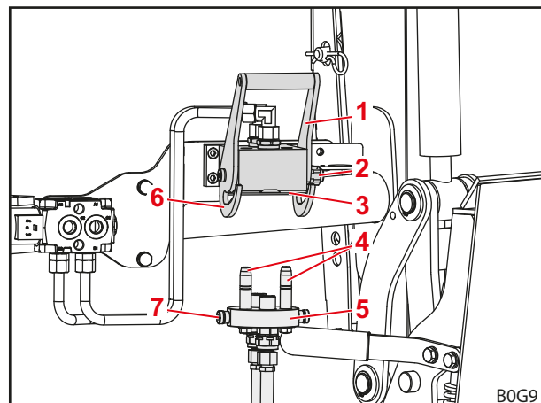
Fig. 56 Afgekoppelde werktuig-fix
