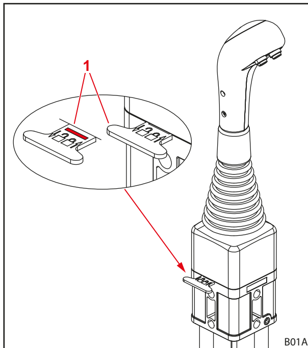
Fig. 45 Vergrendeling van de bedieningshendel
