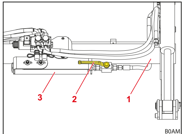
Fig. 32 Met de hand bediende Comfort-Drive (hendelpositie Comfort-Drive aan)
