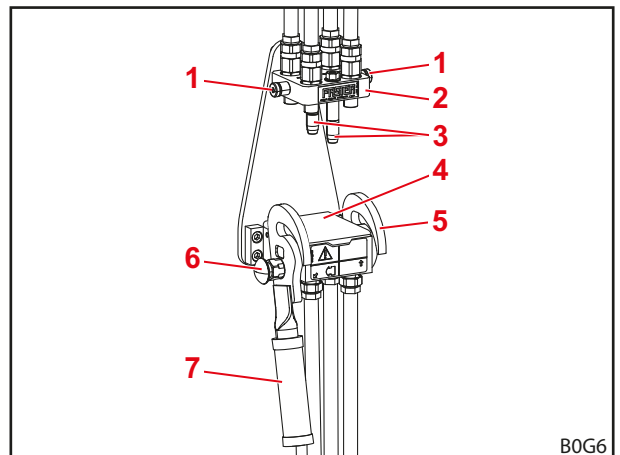
Fig. 54 Afgekoppelde Hydro-Fix
