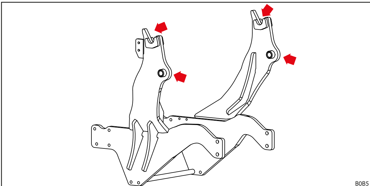
Fig. 96 Smeerpunten frontlader-opneempunten
