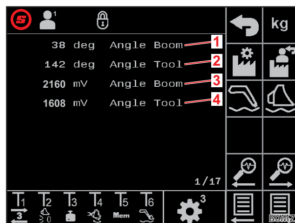
Fig. 37 Hoeksensoren van zwenkarm en werktuig
