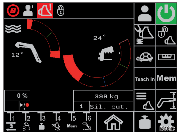
Fig. 36 Weergave Kantelbescherming
