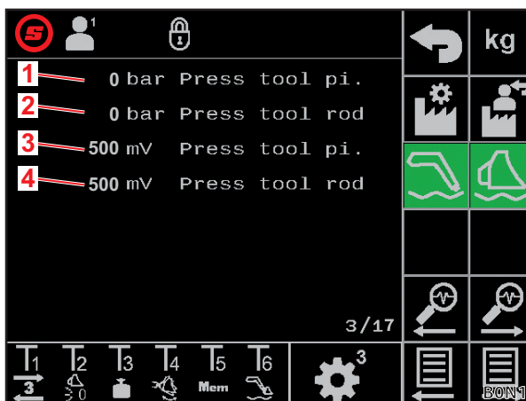
Fig. 39 Druksensoren van het werktuig
