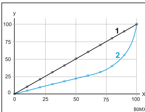
Fig. 25 Grafiek fijnbesturing
