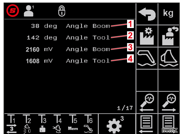
Mynd 37 Hornskynjarar fyrir arm og verkfæri
