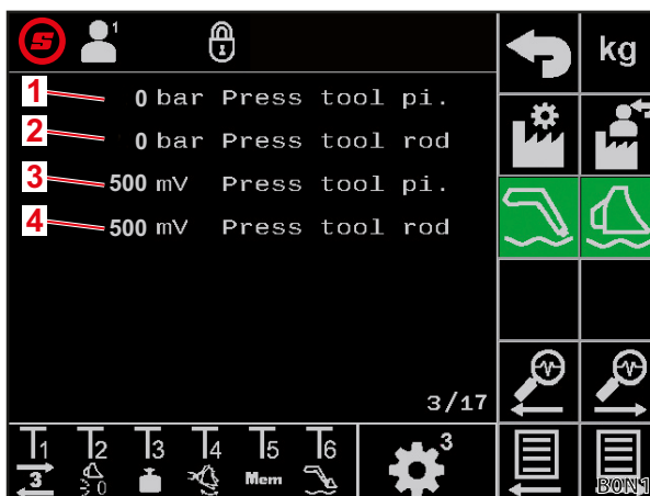
Mynd 39 Þrýstinemar verkfæris
