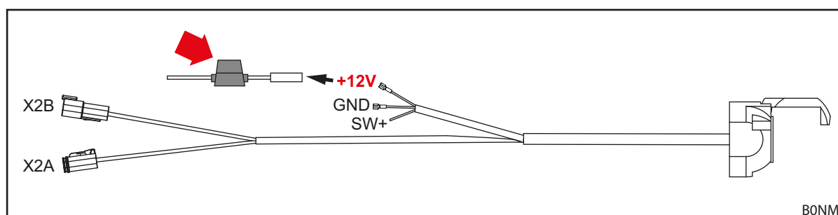
Mynd 53 STOLL-ISOBUS-leiðsluknippi
