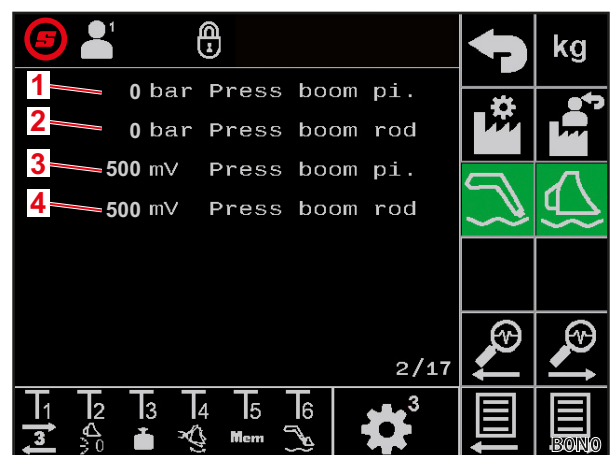
Mynd 38 Þrýstinemar armsins
