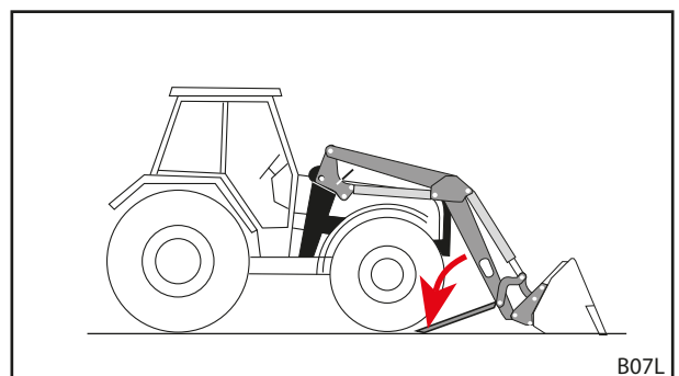
Mynd 127 Stoðfætur settir niður
