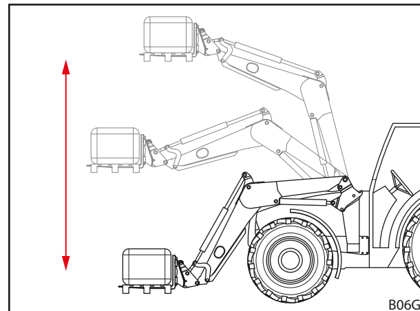
Mynd 31 Hallastýring
