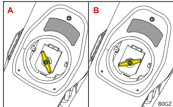
Mynd 39 Stöður stangar fyrir Comfort-Drive
