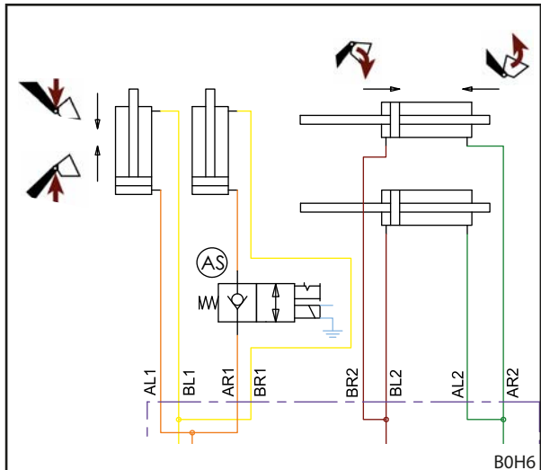
Mynd 135 Yfirlitsmynd af vökvakerfi sigvarnar
