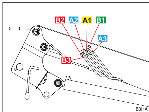
Mynd 16 Glussalagnir (aukabúnaðurinn REAL 3 )
