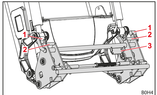
Mynd 12 Fjölskiptigrind Euro-Alö 3
