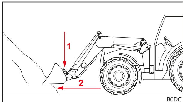
Mynd 113 Ámoksturstækið lækkað og ekið beint inn í það sem á að moka
