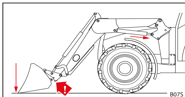
Mynd 94 Verkfærinu þrýst niður að jörðu
