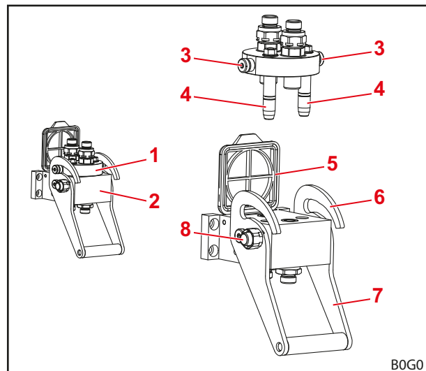
Mynd 22 Uppbygging verkfæristöngs
