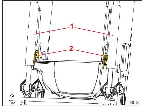
Mynd 42 Kranar á verkfæristjökkum
