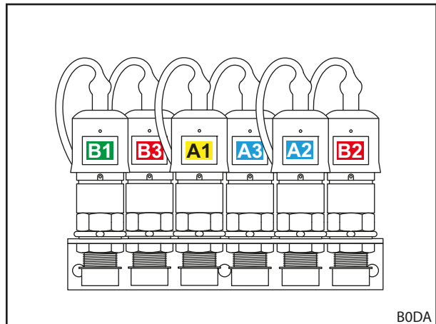
Mynd 18 Hraðtengi tengd (aukabúnaðurinn REAL 3 )
