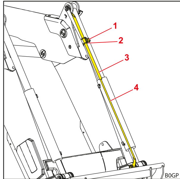
Mynd 30 Vísir fyrir stillingu verkfæris
