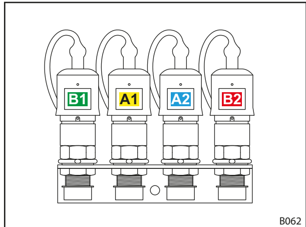
Mynd 17 Hraðtengi tengd
