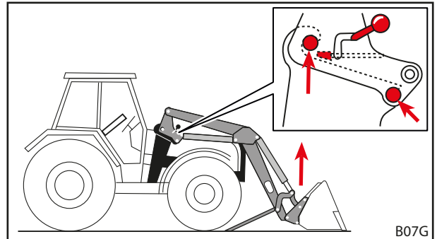
Mynd 53 Lyft þar til boltar ámoksturstækisins eru í gripkrókunum
