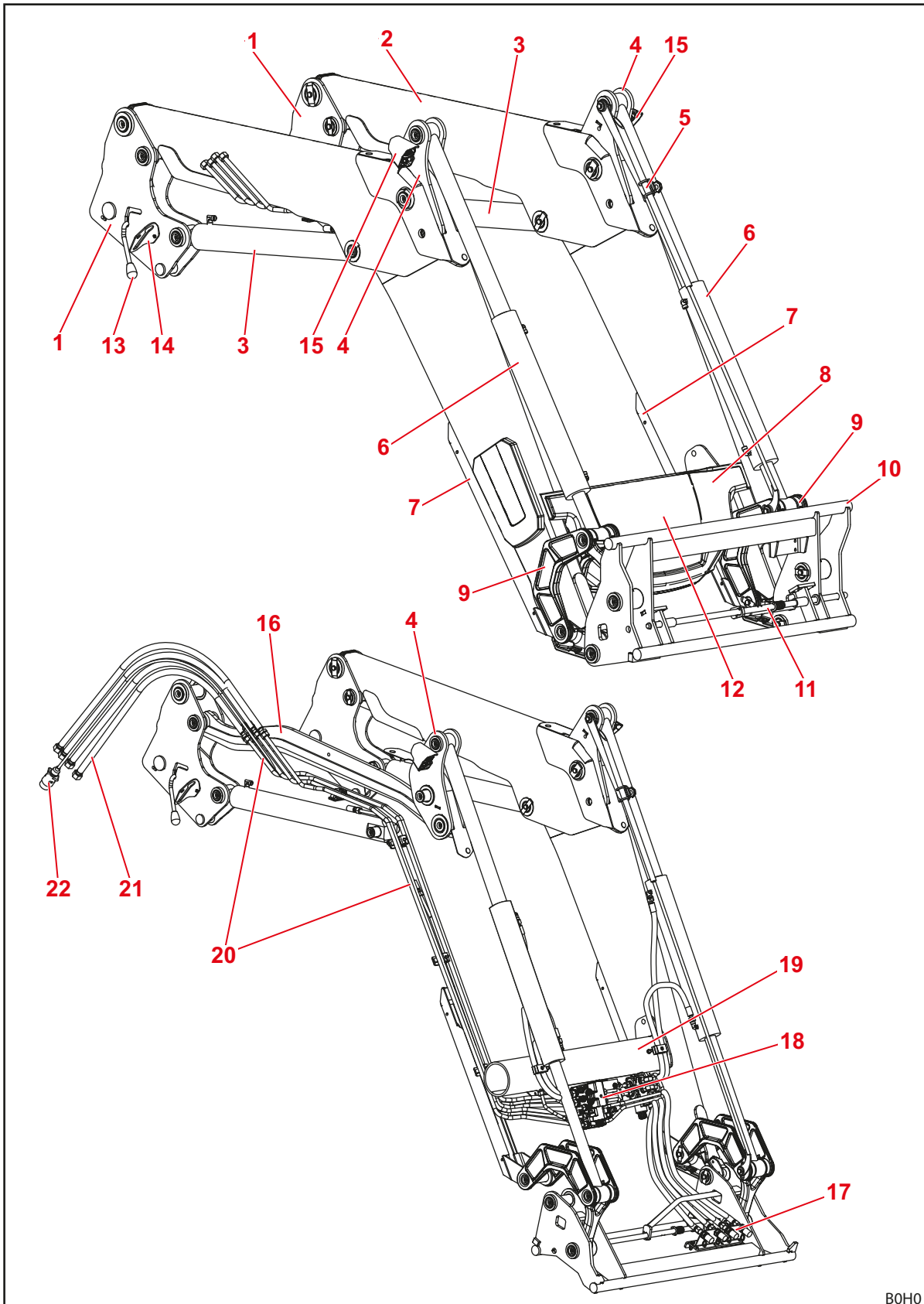
Mynd 8 FZ-ámoksturstæki
