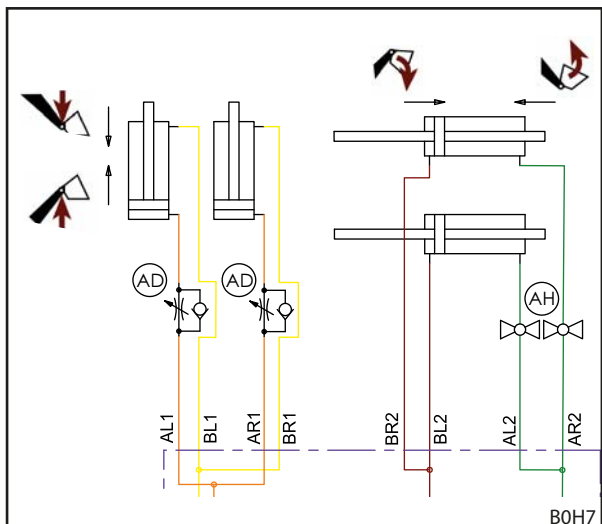
Mynd 136 Yfirlitsmynd af vökvakerfi lækkunarloka
