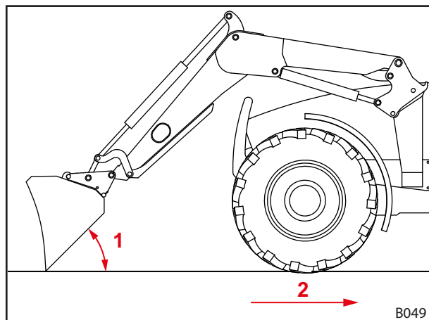
Mynd 111 Slétt úr jarðvegi aftur á bak
