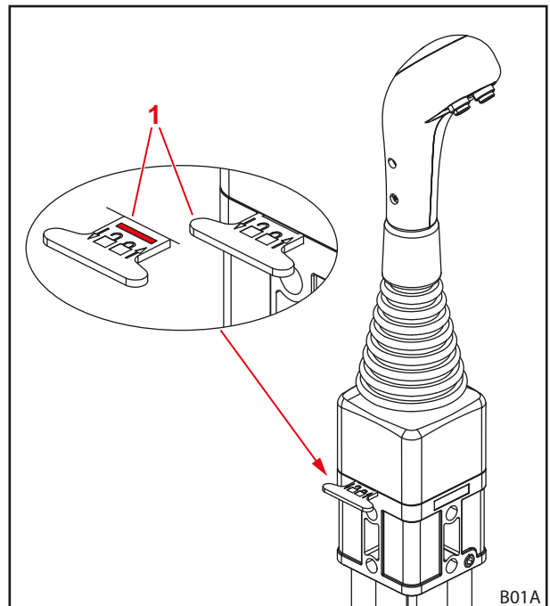
Mynd 68 Læsing stjórnstangarinnar
