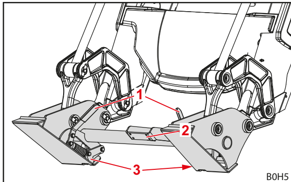
Mynd 13 Skid-Steer-skiptigrind
