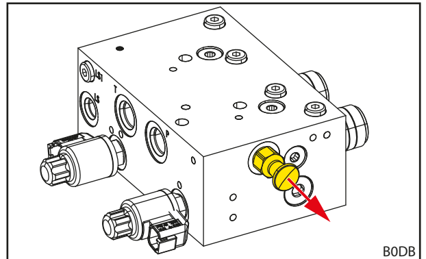
Mynd 76 Afléttiloki á REAL 3 -ventlinum dreginn út
