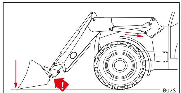
Mynd 87 Verkfærinu þrýst niður að jörðu
