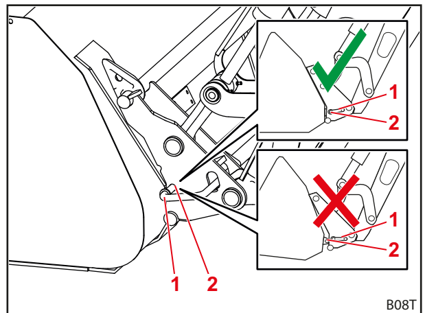
Mynd 86 Staða lásbolta athuguð
