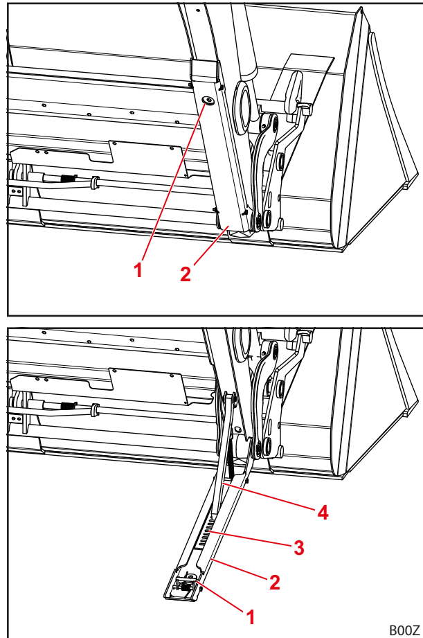
Mynd 78 Stoðfótur
