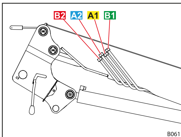
Mynd 15 Glussalagnir
