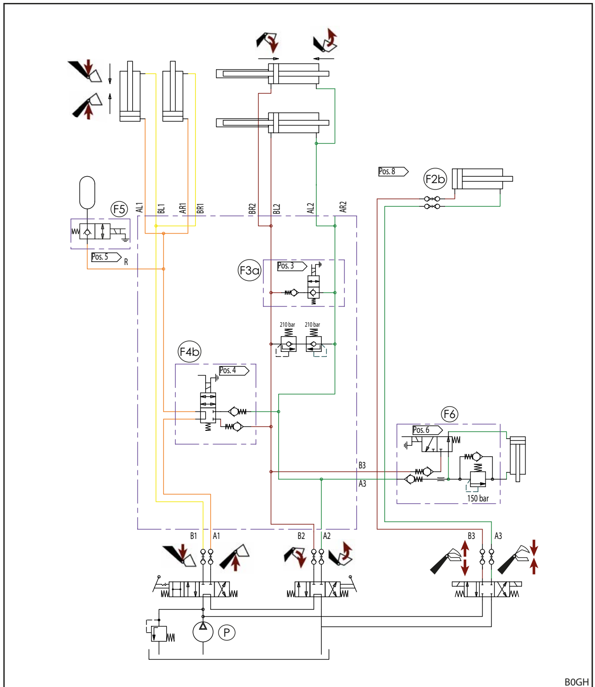
Mynd 134 Yfirlitsmynd af vökvakerfi FZ og FZ-L (með REAL 3 )
