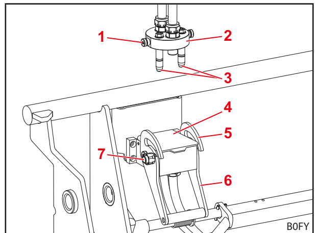
Mynd 82 Aftengt verkfærastengi
