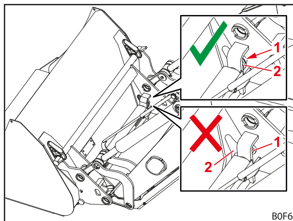
Mynd 93 Staða lásbolta athuguð
