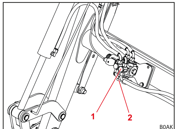
Fig. 30 3° circuito di comando aggiuntivo
