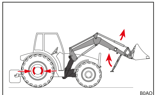
Fig. 41 Ripiegare i piedini
