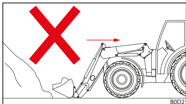
Fig. 94 Retromarcia sotto carico – errato
