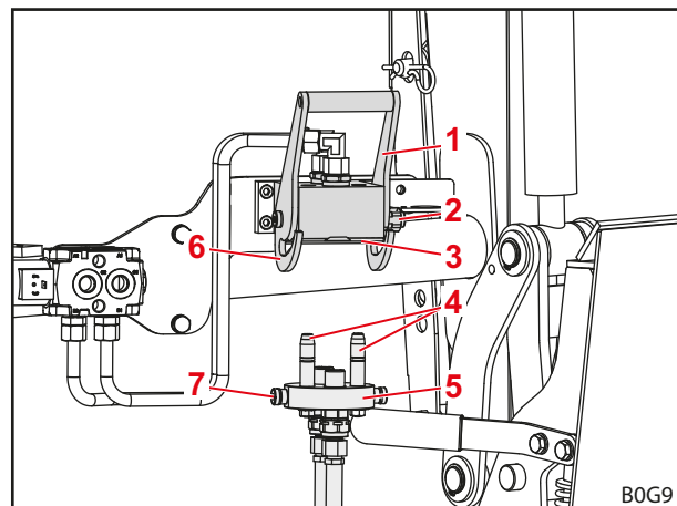
Fig. 56 Dispositivo Fix per attrezzo scollegato
