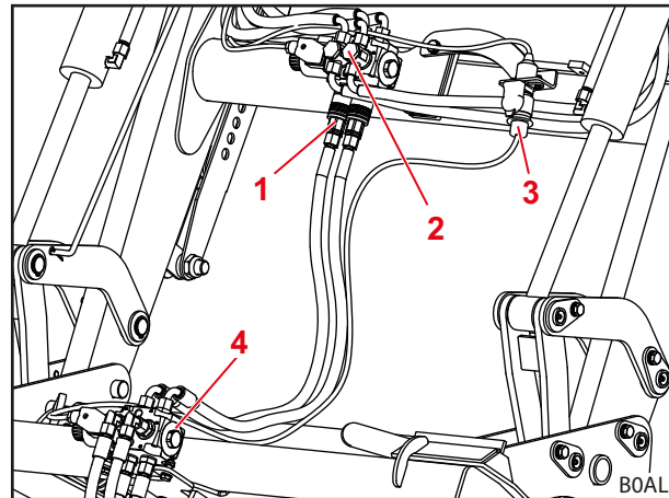
Fig. 31 4° circuito di comando aggiuntivo
