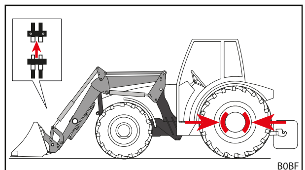
Fig. 84 Distacco tubature idrauliche
