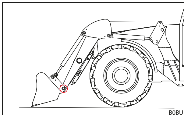
Fig. 89 Estrarre i perni inferiori
