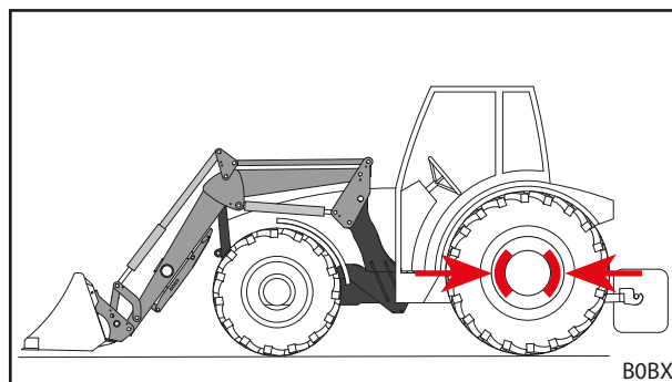
Fig. 87 Posizionare l'attrezzo da deporre e tirare il freno di stazionamento
