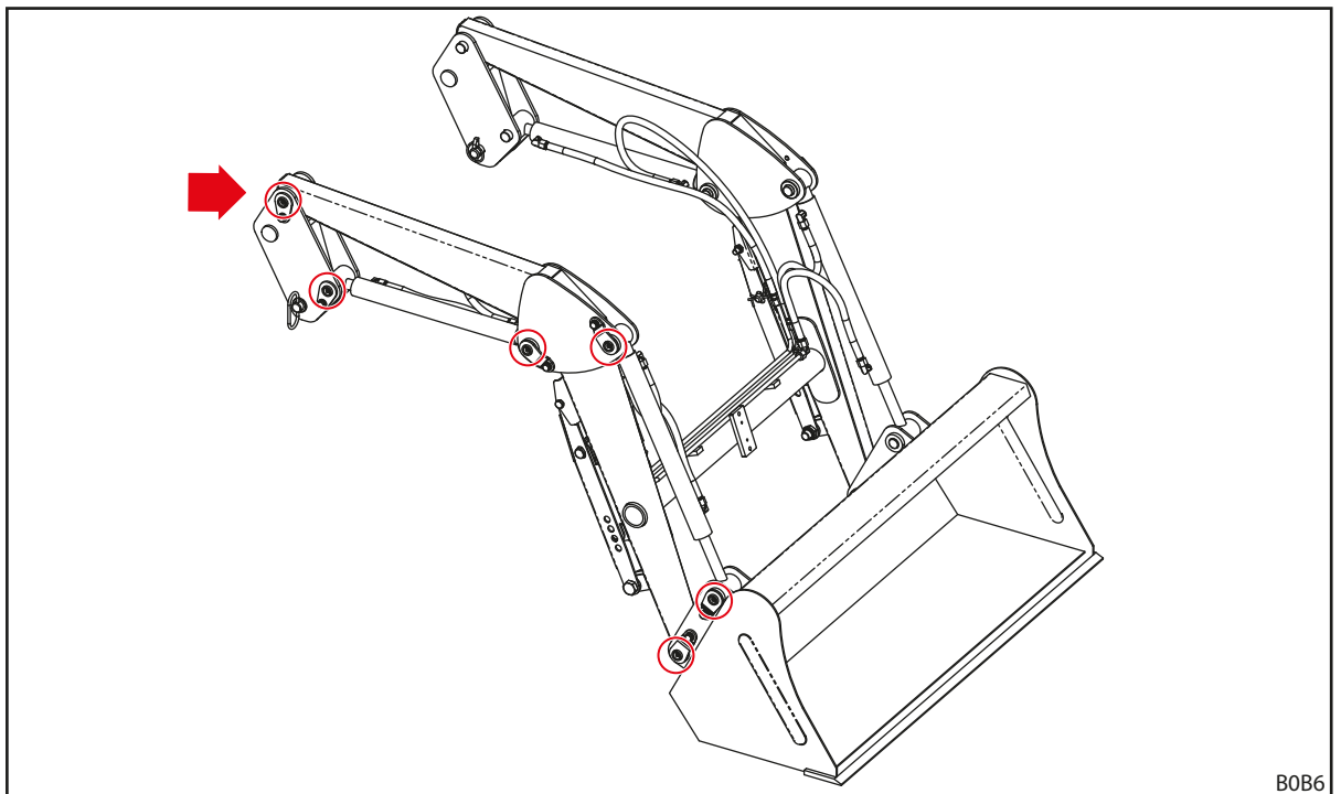
Fig. 97 Punti di lubrificazione L
