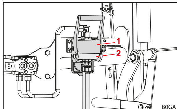
Fig. 57 Dispositivo Fix per attrezzo collegato
