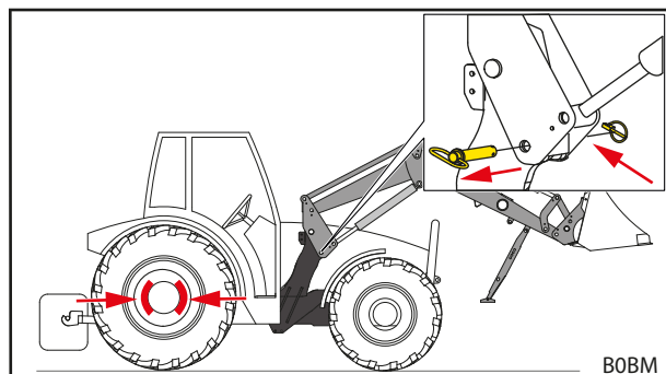
Fig. 101 Tirare il freno di stazionamento e sbloccare il dispositivo per il bloccaggio del caricatore frontale
