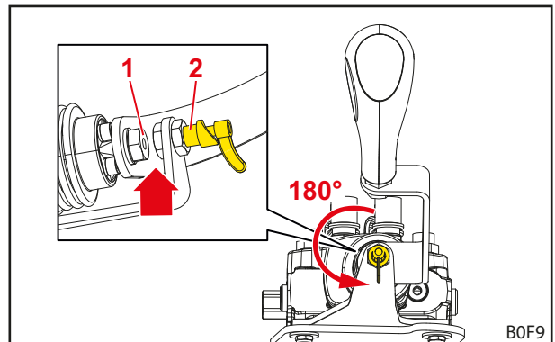
Fig. 49 Leva di comando sbloccata
