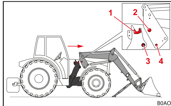
Fig. 38 Inserimento trattore nel braccio oscillante
