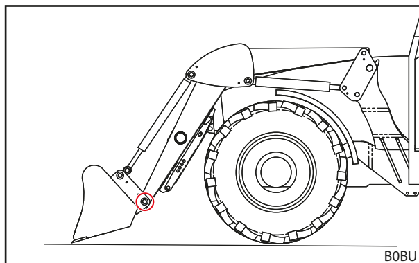
Fig. 79 Collegare l'attrezzo agendo sui fori perno inferiori
