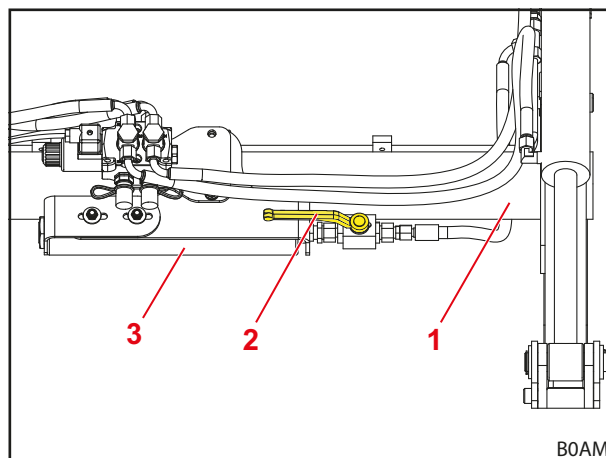
Fig. 32 Comfort-Drive ad azionamento manuale (posizione leva Comfort-Drive on)
