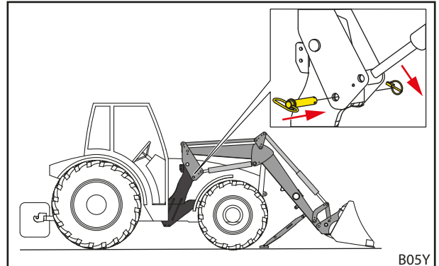
Fig. 40 Inserire i perni di bloccaggio e bloccarli con spine a scatto
