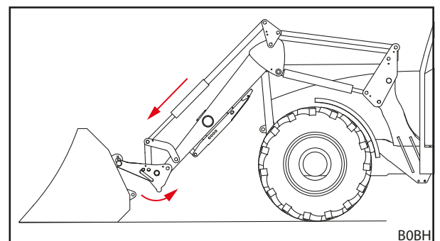
Fig. 85 Sgancio del telaio intercambiabile
