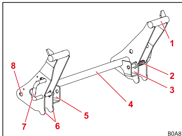
Fig. 64 Dispositivo di bloccaggio dell'attrezzo sul telaio intercambiabile Euro
