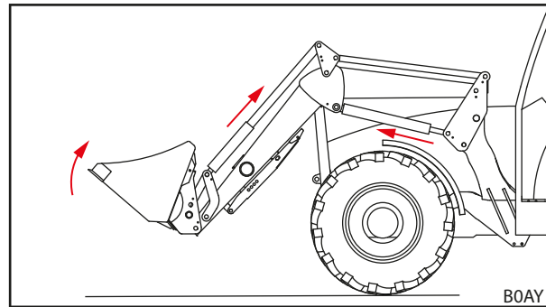
Fig. 71 Attivare il dispositivo per il bloccaggio degli attrezzi
