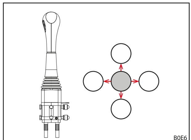
Fig. 46 Spostare la leva di comando in tutte le posizioni finali
