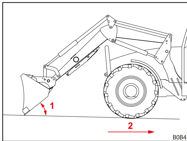
Fig. 91 Lavori di spianamento in retromarcia
