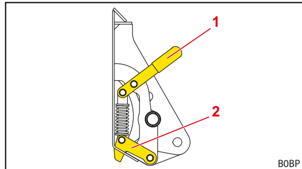
Fig. 59 Bloccaggio meccanico dell'attrezzo Skid-Steer (stato semichiuso)
