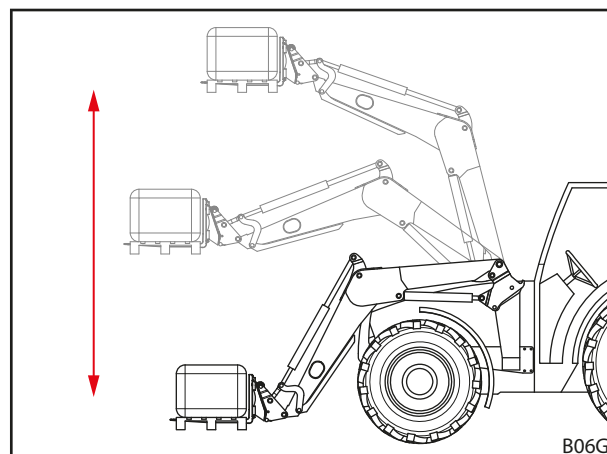
Fig. 31 Guida parallela
