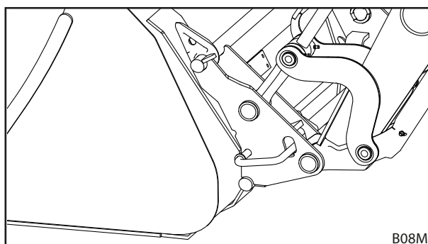
Fig. 95 Aprire il dispositivo per il bloccaggio degli attrezzi
