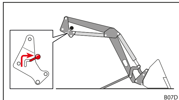
Fig. 50 Apertura del dispositivo di blocco del caricatore frontale
