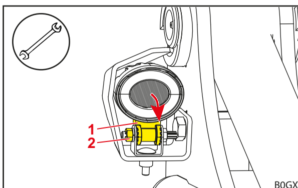
Fig. 45 Regolazione verticale dei fari
