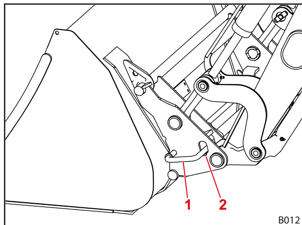
Fig. 84 Bloccaggio meccanico degli attrezzi
