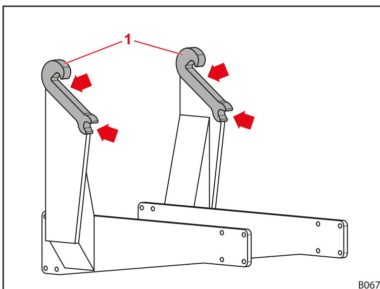
Fig. 117 Punti di lubrificazione degli attacchi del caricatore frontale
