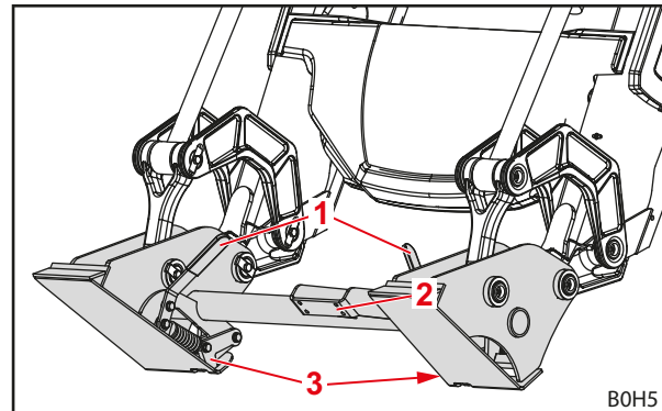
Fig. 13 Telaio intercambiabile Skid-Steer
