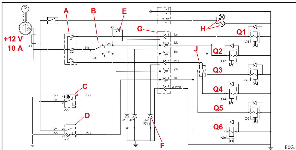
Fig. 137 Schema elettrico (se dotato di 3° e 4° circuito di comando)
