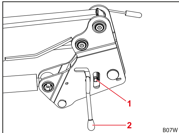
Fig. 122 Verificare il dispositivo di bloccaggio del caricatore frontale
