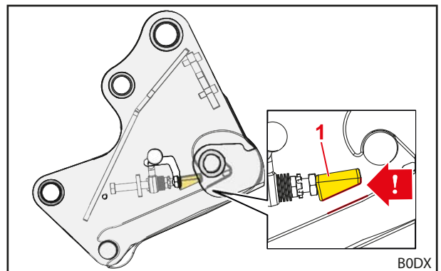
Fig. 55 Posizione di montaggio corretta del cuneo di bloccaggio
