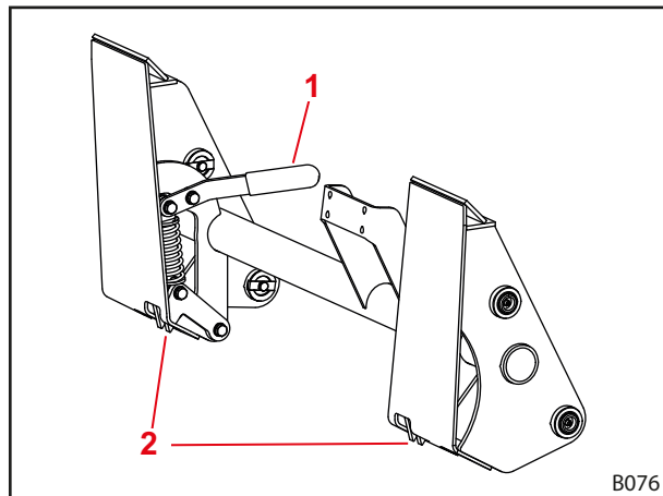
Fig. 88 Dispositivo per il bloccaggio degli attrezzi sul telaio intercambiabile Skid-Steer
