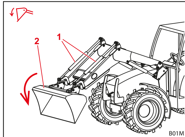
Fig. 28 Funzione sbennamento
