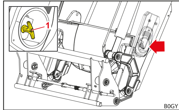
Fig. 38 Comfort-Drive ad azionamento manuale
