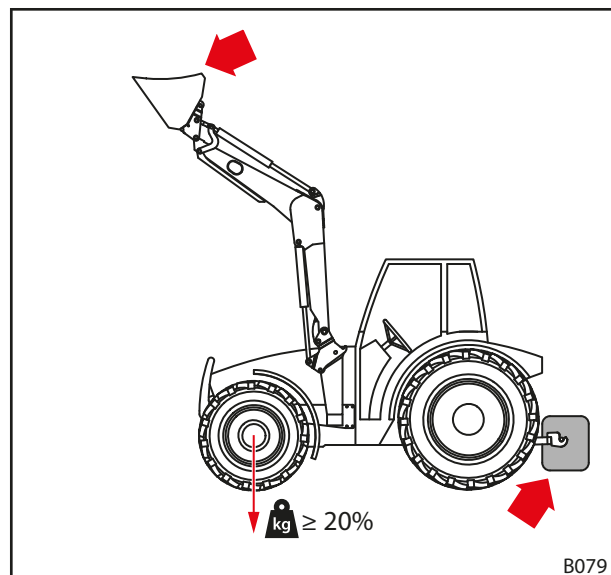
Fig. 48 Carico applicato durante la marcia su strada
