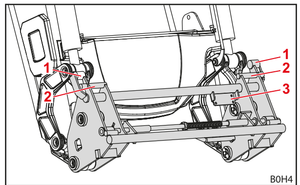
Fig. 12 Telaio intercambiabile combinato Euro-Alö 3
