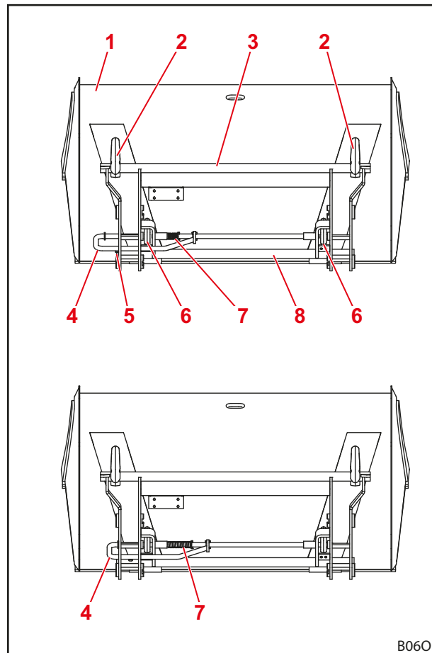
Fig. 23 Dispositivo di bloccaggio aperto (sopra) e chiuso (sotto)
