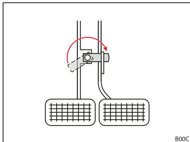
Fig. 46 Collegamento dei pedali dei freni
