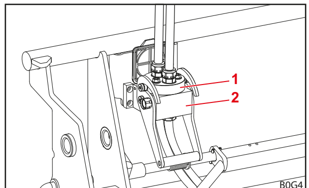
Fig. 83 Dispositivo Fix per attrezzo collegato
