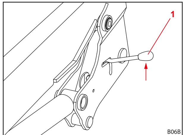
Fig. 56 Apertura del dispositivo di blocco del caricatore frontale
