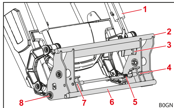
Fig. 10 Telaio intercambiabile Euro
