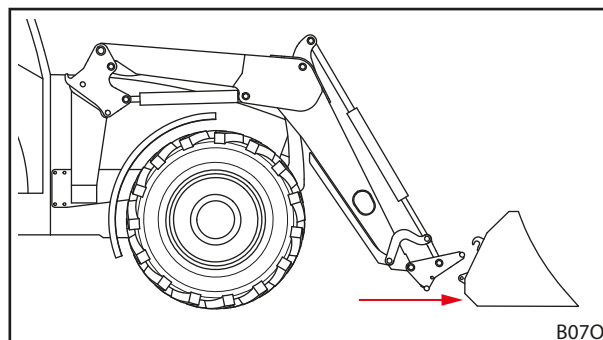
Fig. 105 Avvicinamento
