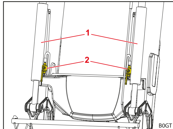
Fig. 42 Rubinetti d'intercettazione sui cilindri attrezzo
