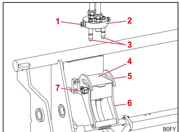
Fig. 82 Dispositivo Fix per attrezzo scollegato
