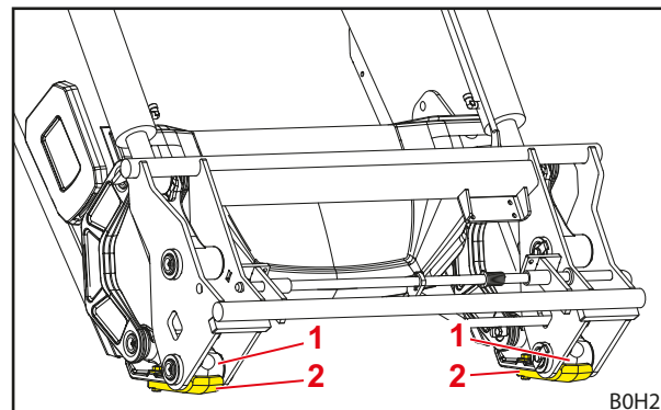
Fig. 14 Pattini di usura
