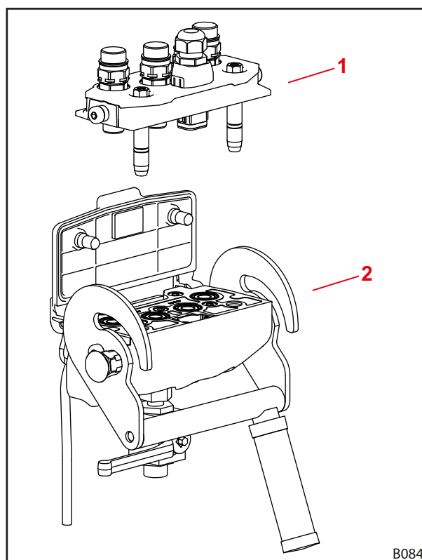
Fig. 20 Struttura Hydro-Fix
