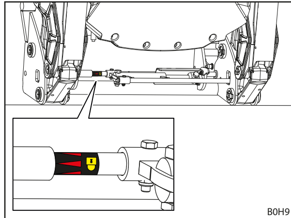
Fig. 92 Controllare il dispositivo per il bloccaggio degli attrezzi sulla base dell'etichetta
