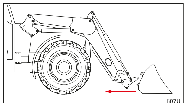
Fig. 110 Allontanamento
