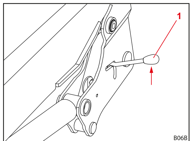
Fig. 121 Verificare il dispositivo di bloccaggio del caricatore frontale
