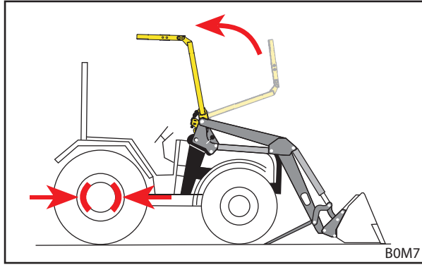
Fig. 56 Ribaltare verso l'alto l'OPG
