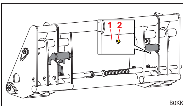
Fig. 92 Perni d'aggancio orientati verso l'alto (vista da dietro)
