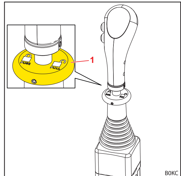
Fig. 68 Bloccaggio della leva di comando (dispositivo di bloccaggio verticale)
