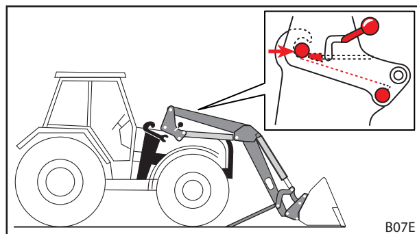
Fig. 54 Inserire il trattore nel braccio oscillante
