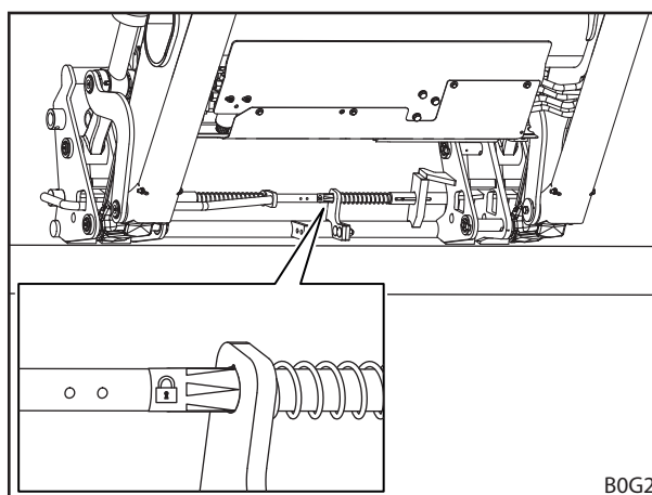
Fig. 84 Controllare il dispositivo per il bloccaggio degli attrezzi sulla base dell'etichetta (telaio intercambiabile combinato Euro-FR)
