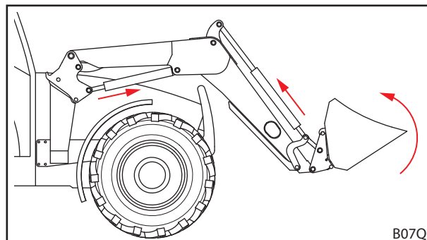
Fig. 99 Attivare il dispositivo per il bloccaggio degli attrezzi
