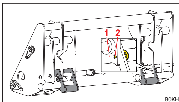
Fig. 90 Perna di aggancio orientati verso il basso
