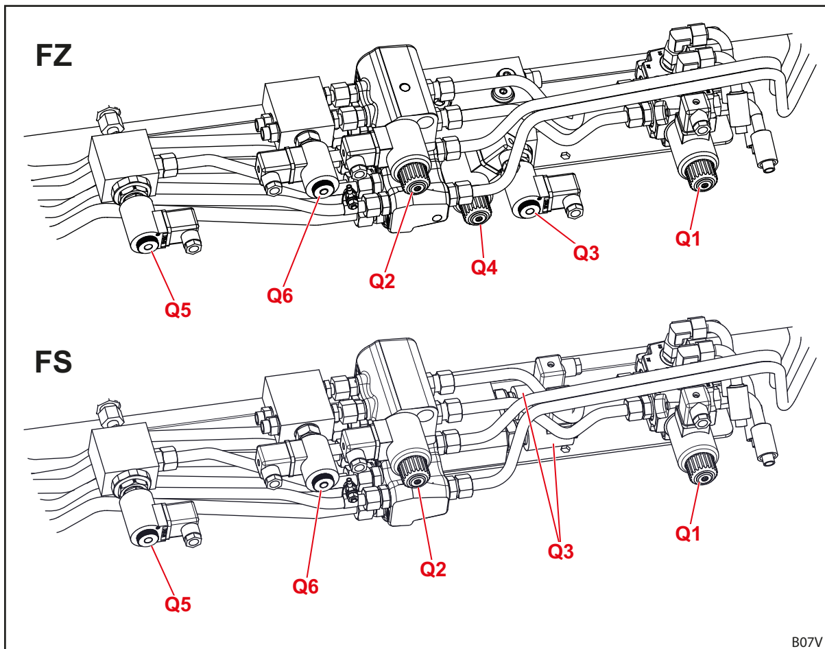
Sl. 133 Raspored hidrauličnih ventila za dodatne funkcije
