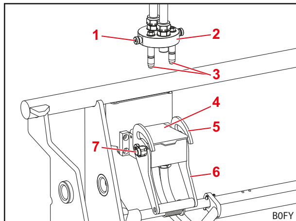
Sl. 78 Odvojena spojka Implement-Fix
