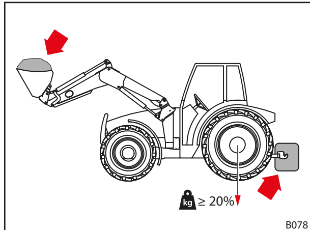
Sl. 44 Opterećenje kod radova s prednjim utovarivačem
