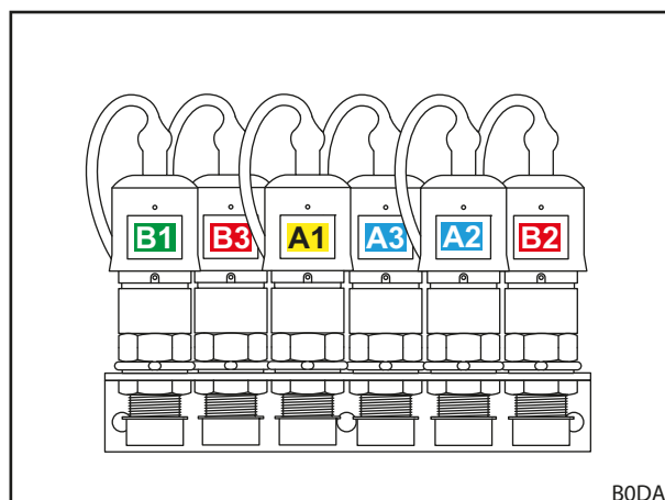
Sl. 20 Utične spojke spojene (opcija REAL 3 )
