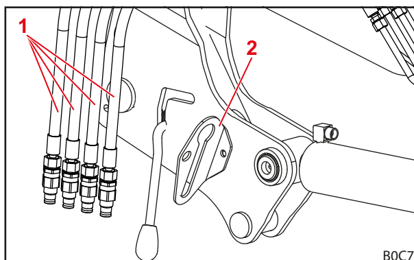
Sl. 126 Hidrauličke vodove objesite u držače spojke (prikaz s utičnim spojkama).
