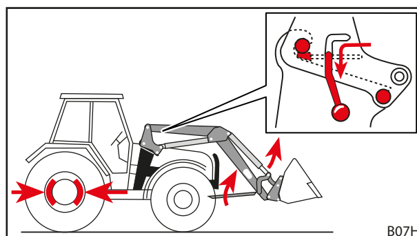
Sl. 51 Sklapanje potpornih nožica i zatvaranje blokade prednjeg utovarivača
