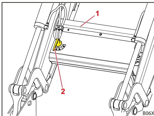
Sl. 40 Rukom aktivirani Comfort Drive
