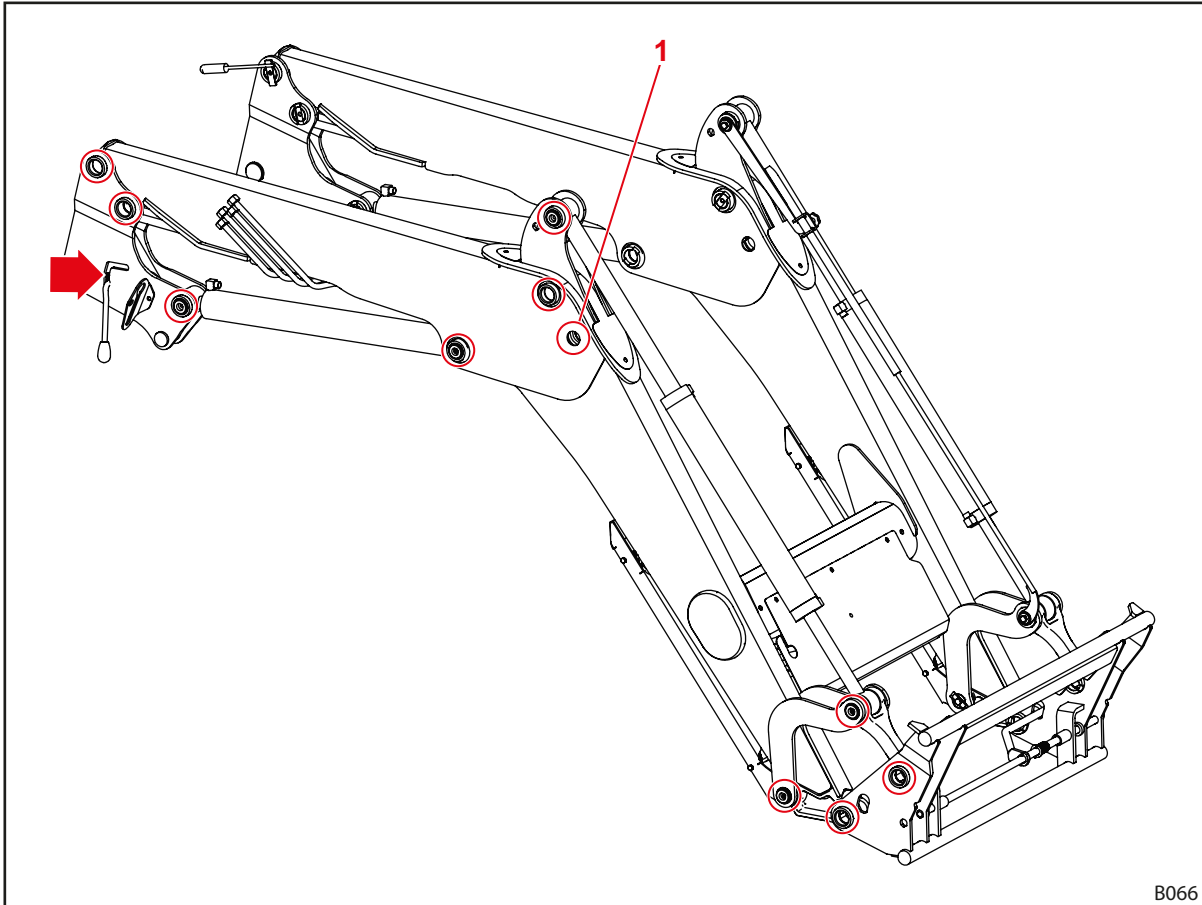
Sl. 115 Mjesta podmazivanja FZ
