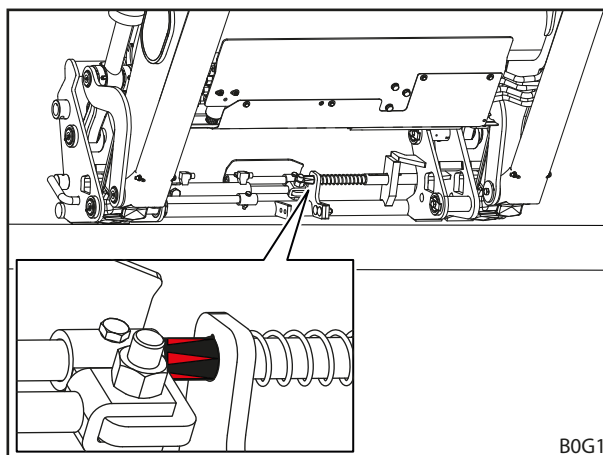
Sl. 88 Provjera blokade opreme na temelju naljepnice
