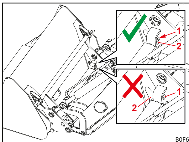
Sl. 90 Provjera položaja svornjaka blokade
