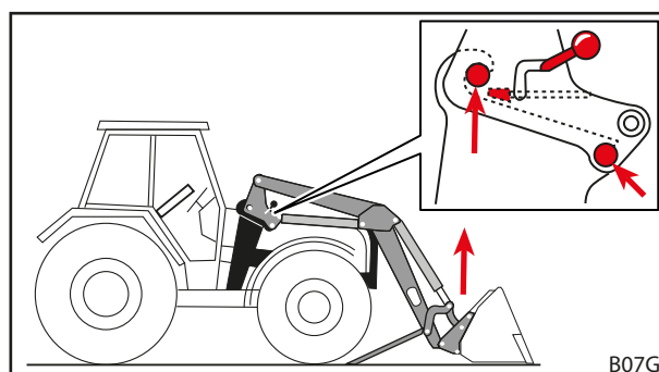
Sl. 50 Upotrebljavajte funkciju Podizanje sve dok svornjaci prednjeg utovarivača ne nalegnu u prihvatne kuke
