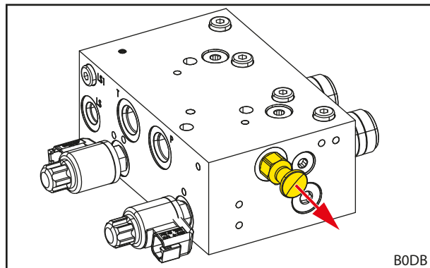
Sl. 72 Izvlačenje ventila za tlačno rasterećenje na ventilu REAL 3
