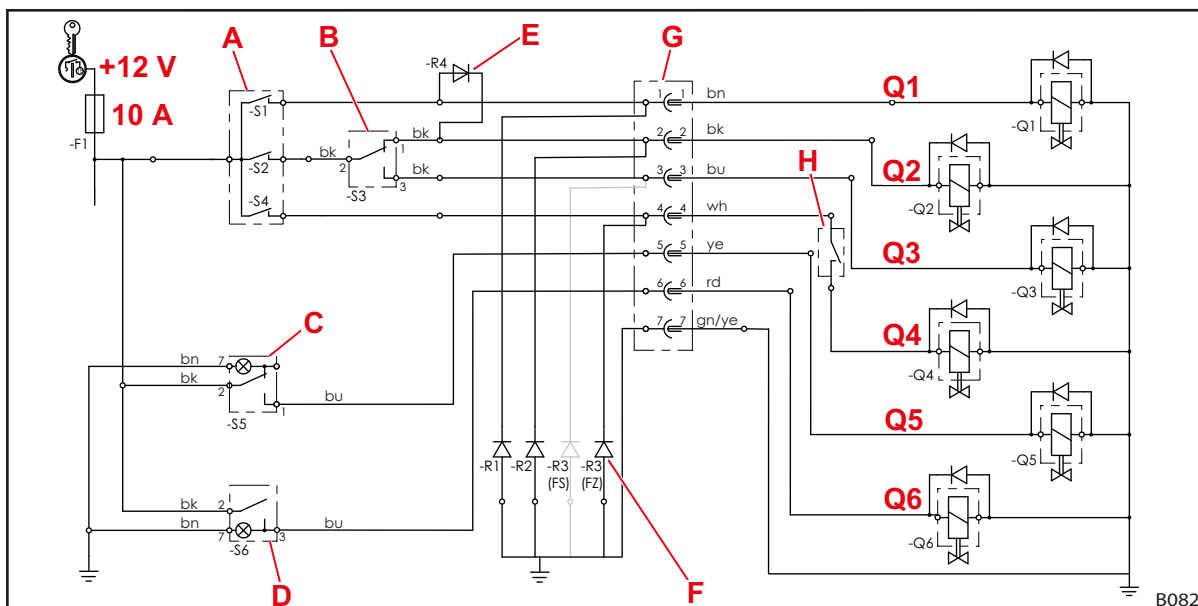
Sl. 131 Električna shema spoja (kod opremljenosti 3. i 4. upravljačkim krugom)
