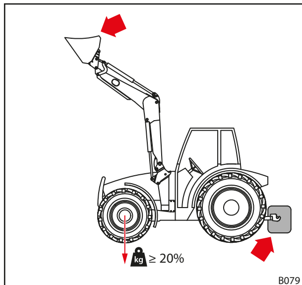
Sl. 45 Opterećenje kod vožnji cestom
