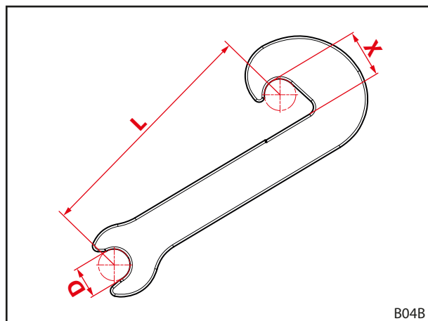
Sl. 116 Mjera istrošenosti prihvatne kuke
