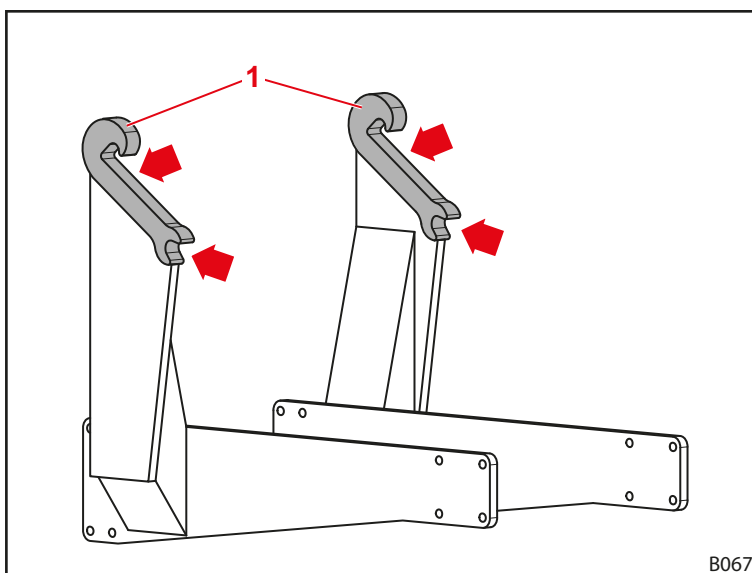
Att. 117 Frontālā iekrāvēja stiprinājuma vietu eļļošanas vietas
