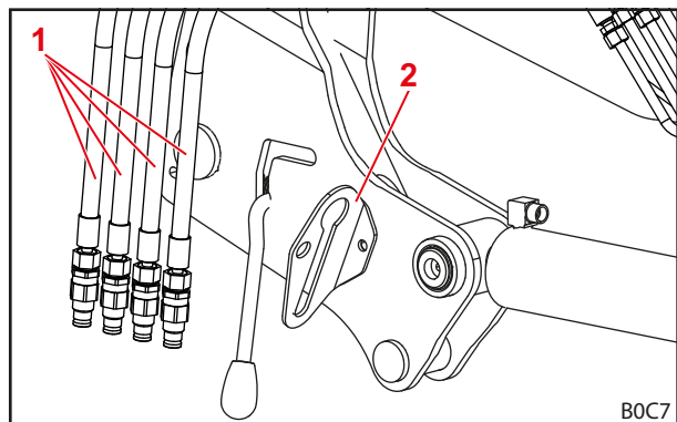
Att. 130 Hidraulisko šļūteņu iekabināšana savienojuma turētājā (attēlots ar spraudsavienojumiem)
