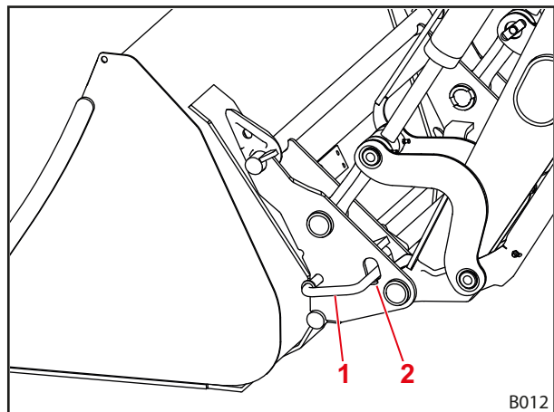
Att. 84 Mehāniskais aprīkojuma fiksators
