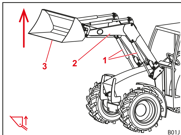
Att. 25 Celšanas funkcija
