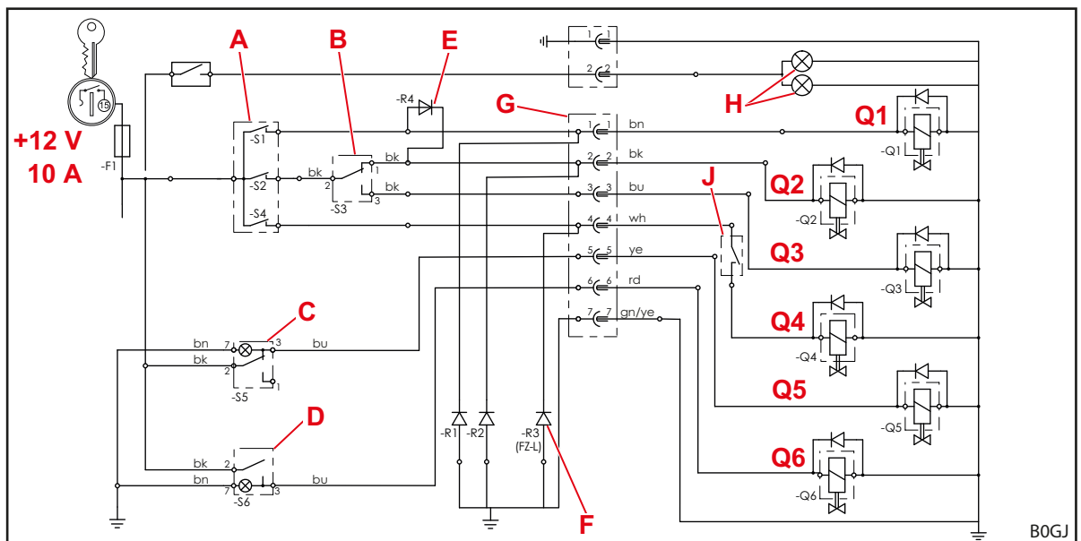
Att. 137 Elektriskā shēma (aprīkojumam ar 3. un 4. hidraulisko izvadu)
