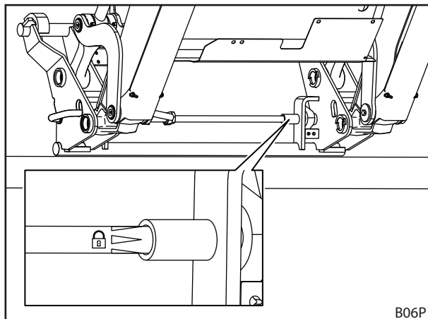
Att. 85 Pārbaudiet aprīkojuma fiksatoru, ievērojot uzlīmi
