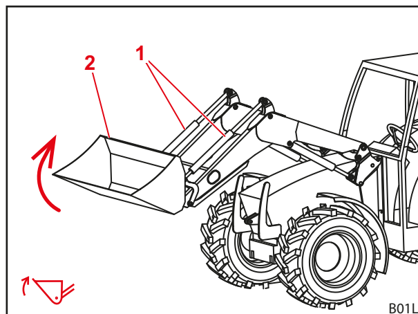
Att. 27 Grābšanas funkcija
