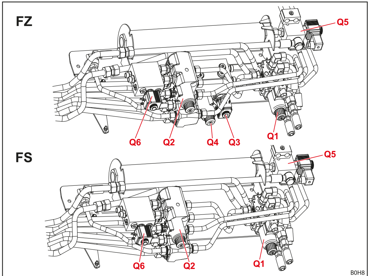
Att. 139 Papildfunkciju hidrovārstu izvietojums
