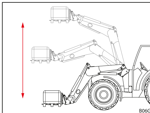
Att. 31 Paralēlā vadība
