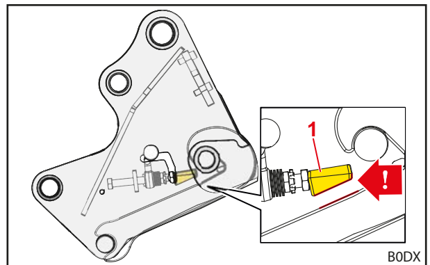
Att. 55 Iespīlēšanas ķīļa pareiza montāžas pozīcija
