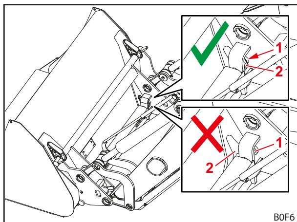
Att. 93 Pārbaudiet fiksācijas tapu pozīciju
