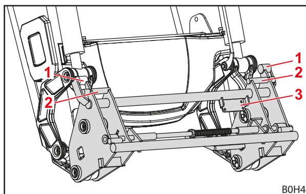
Att. 12 Kombinētais nomaīņas rāmis Euro-Alö3
