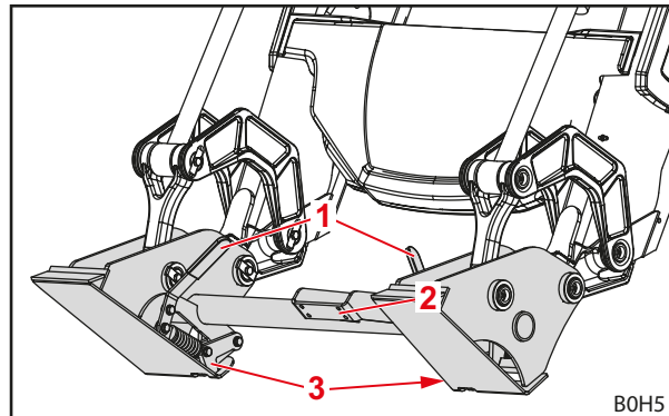
Att. 13 Skid-Steer nomaiņas rāmis
