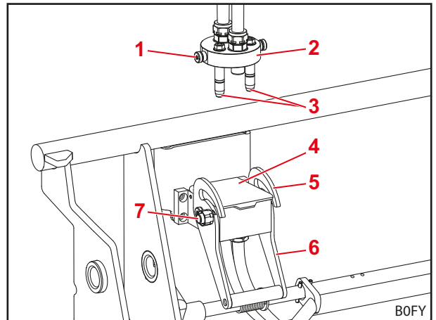
Att. 82 Atvienots aprīkojuma fiksators
