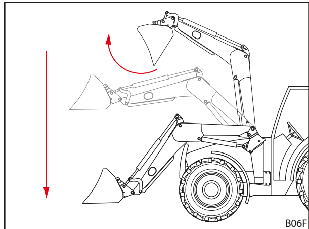
Att. 33 Return-To-Level funkcija
