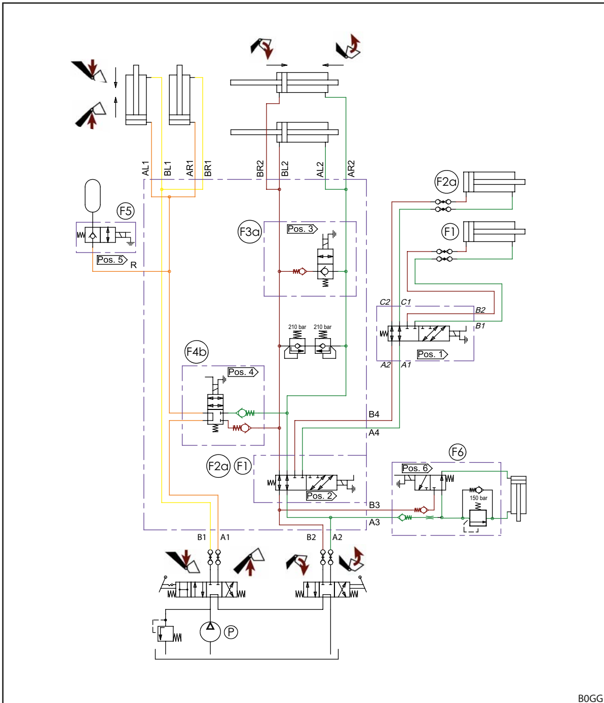
Att. 133 Hidrauliskās sistēmas shēma FZ un FZ-L (aprīkojumam ar 3. un 4. hidraulisko izvadu)
