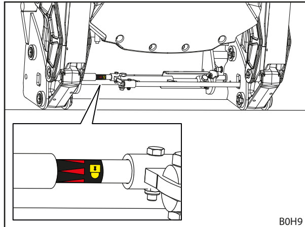
Att. 92 Pārbaudiet aprīkojuma fiksatoru, ievērojot uzlīmi
