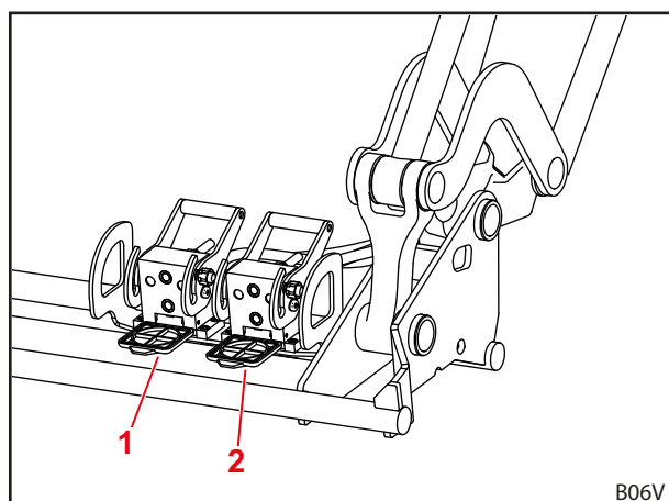
Att. 36 Papildu 4. hidrauliskais izvads
