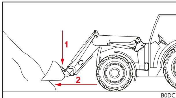
Att. 113 Nolaidiet frontālo iekrāvēju un taisni iebrauciet kravā
