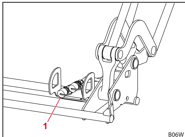
Att. 35 Papildu 3. hidrauliskais izvads
