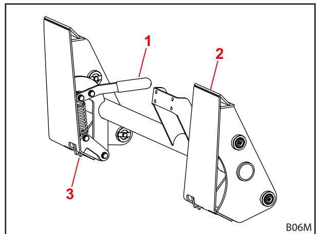
Att. 24 Mehāniskā aprīkojuma fiksators pie Skid-Steer nomaiņas rāmja
