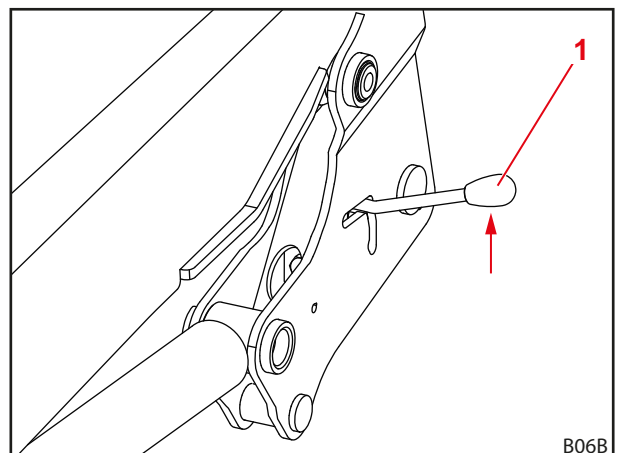
Att. 56 Frontālā iekrāvēja fiksatora atvēršana
