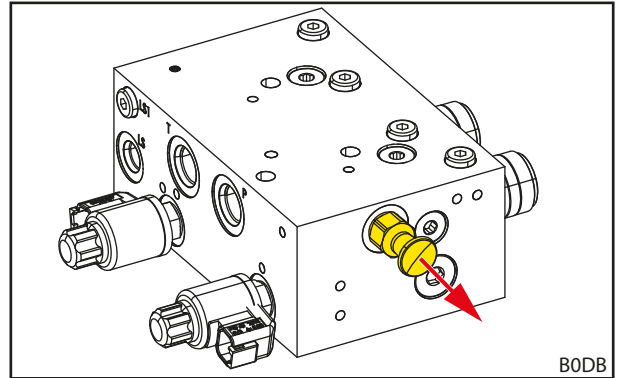
Att. 76 Spiediena atslogošanas vārsta pie REAL 3 vārsta izvilkšana
