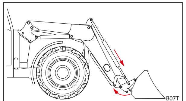
Att. 109 Nomainas rāmja izkabināšana
