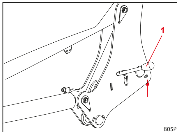
Pav. 112 Priekinio krautuvo fiksatoriaus tikrinimas
