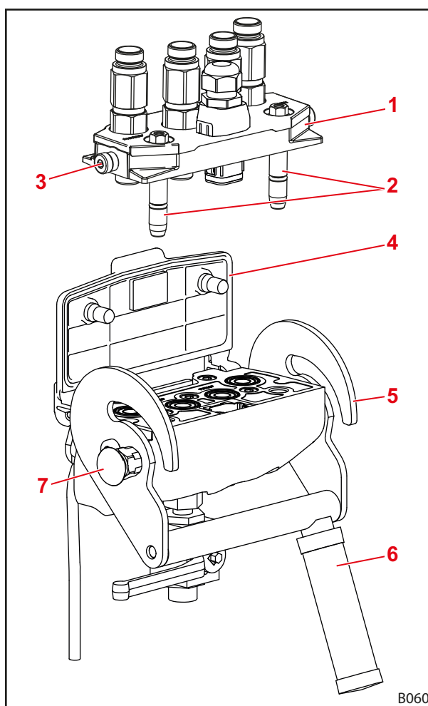
Pav. 74 „Hydro-Fix“ (pavyzdys: 4 dalių „Hydro-Fix“)
