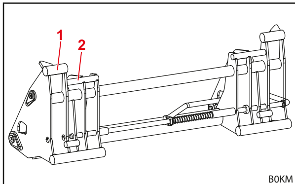
Pav. 17 Kombinuotasis keičiamasis rėmas „Euro-Alö3“
