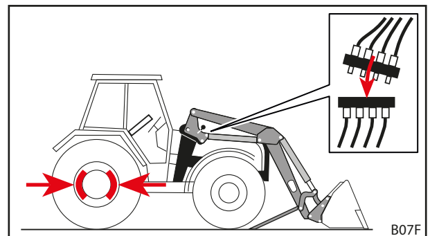
Pav. 48 Traktoriaus išjungimas ir hidraulinių linijų prijungimas
