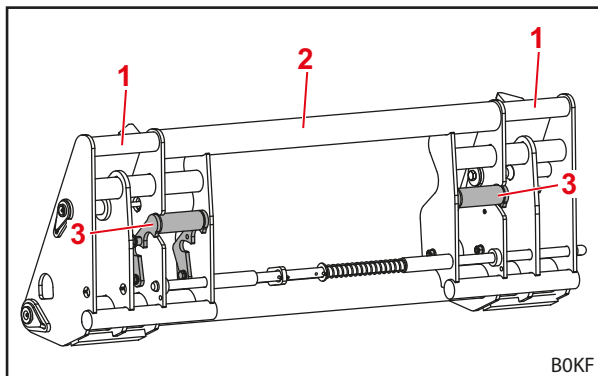
Pav. 16 Kombinuotasis keičiamasis rėmas „Euro-SMS“ (paruoštas SMS padargui)
