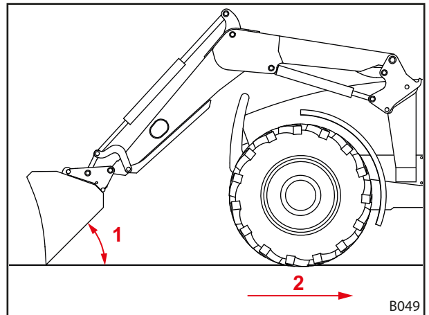
Pav. 102 Lyginimas atbuline eiga
