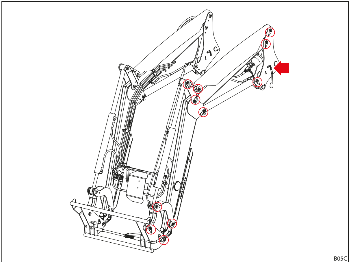
Pav. 110 P tepimo vietos
