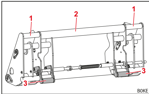
Pav. 15 Kombinuotasis keičiamasis rėmas „Euro-SMS“ (paruoštas „Euro“ padargui)
