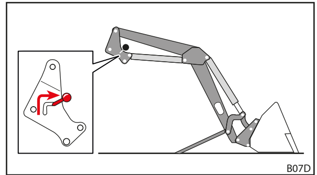
Pav. 46 Priekinio krautuvo fiksatoriaus atidarymas
