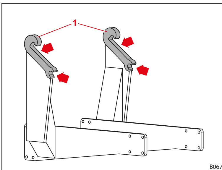
Pav. 108 Priekinio krautuvo laikiklių tepimo vietos
