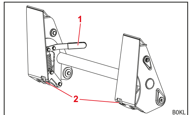
Pav. 14 Keičiamasis rėmas „Skid-Steer“
