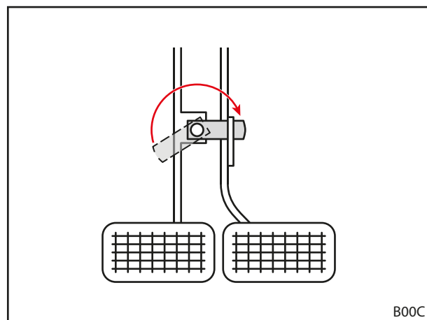
Pav. 42 Stabdžių pedalų sujungimas
