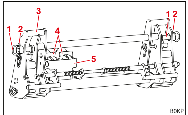
Pav. 18 Kombinuotasis keičiamasis rėmas „Euro-FR“ (paruoštas „Euro“ padargui)
