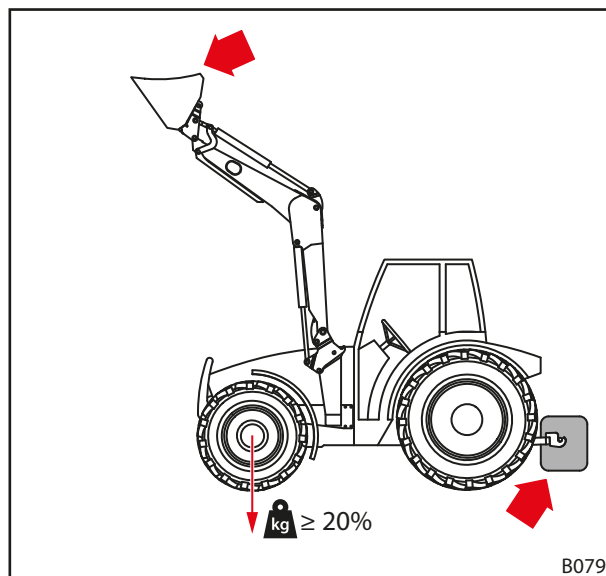
Pav. 44 Balastas, važiuojant keliais
