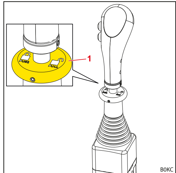
Pav. 61 Valdymo svirties fiksavimas (vertikalus fiksatorius)
