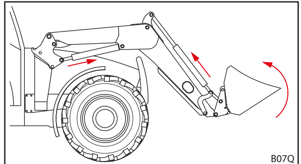
Pav. 92 Padargo fiksatoriaus aktyvinimas
