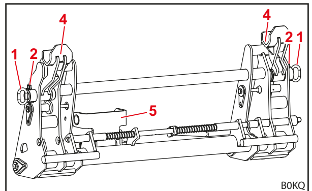
Pav. 19 Kombinuotasis keičiamasis rėmas „Euro-FR“ (paruoštas FR padargui)
