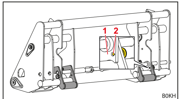
Pav. 83 Pasukti į apačią prispaudikliai
