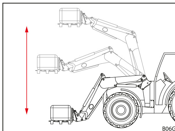
Pav. 32 Mechaninė lygiagreto nukreipimo sistema
