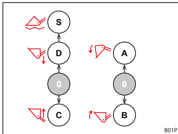
Pav. 58 Paskirstymas, kai yra dvi valdymo svirtys
