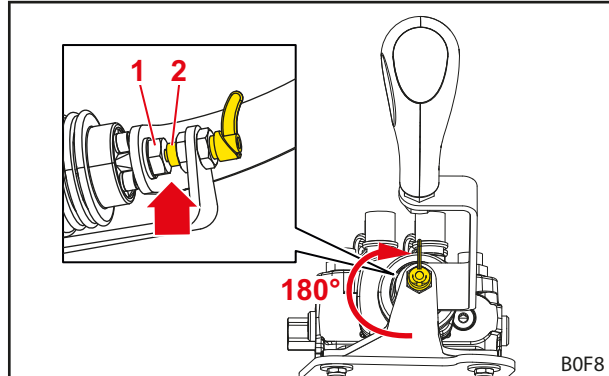
Pav. 64 Užblokuota valdymo svirtis
