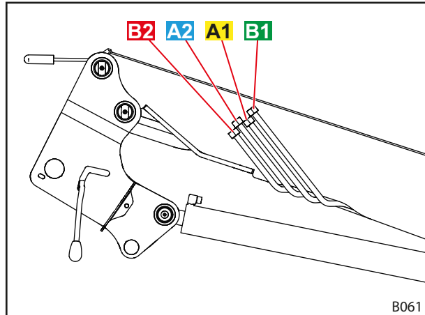
Pav. 20 Hidraulinės linijos
