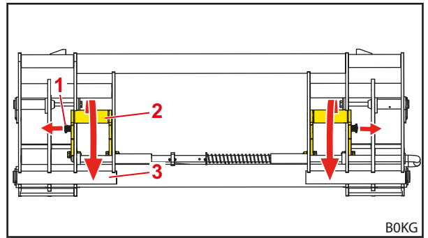
Pav. 82 Prispaudiklių pasukimas į apačią
