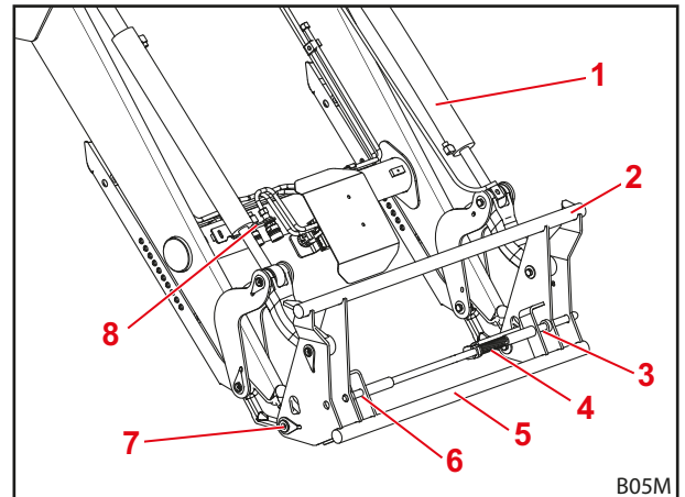
Pav. 13 Keičiamasis rėmas „Euro“
