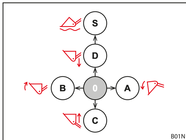
Pav. 57 Paskirstymas, kai yra viena valdymo svirtis
