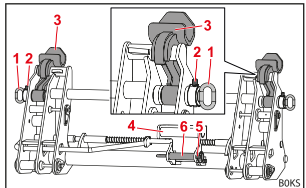
Pav. 87 Adapteris darbo padėtyje (keičiamasis rėmas paruoštas FR padargui)
