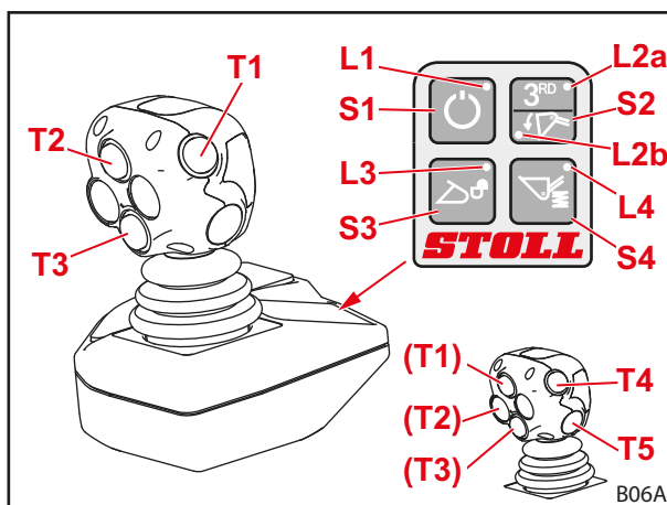
Pav. 67 „STOLL Pro Control“
