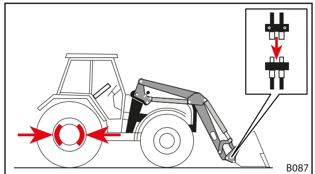
Pav. 93 Padargo hidraulinių linijų sujungimas su priekinio padargo jungtimis
