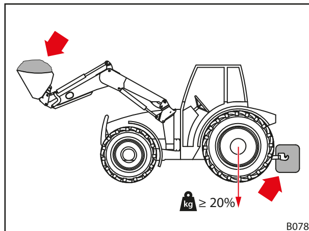
Pav. 43 Balastas, dirbant su priekiniu krautuvu
