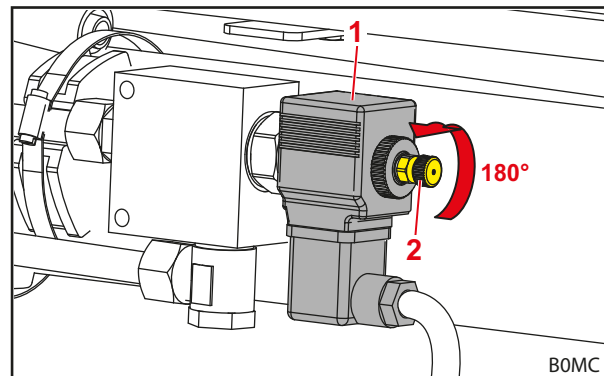
Pav. 33 Vožtuvo atidarymas
