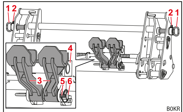
Pav. 86 Adapteris stovėjimo padėtyje (keičiamasis rėmas paruoštas „Euro“ padargui)
