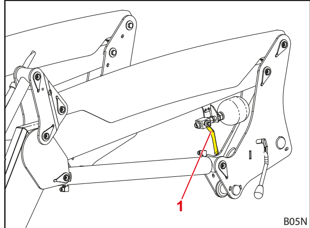
Pav. 40 Mechaniniu būdu aktyvinama „Comfort-Drive“
