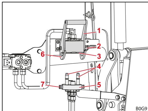
Rys. 56 Odłączone osprzęt Fix
