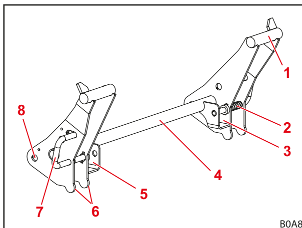
Rys. 22 Ramka wymienna Euro
