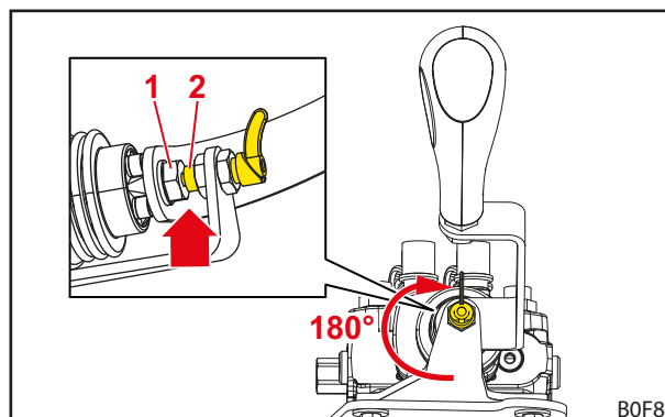
Rys. 48 Zablokowana dźwignia obsługi
