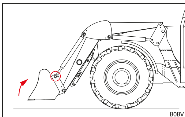
Rys. 80 Łączenie osprzętu na górze z siłownikami hydraulicznymi
