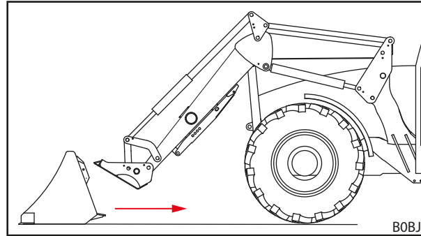
Rys. 86 Odjeżdżanie
