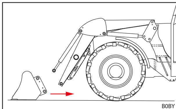
Rys. 90 Odjeżdżanie
