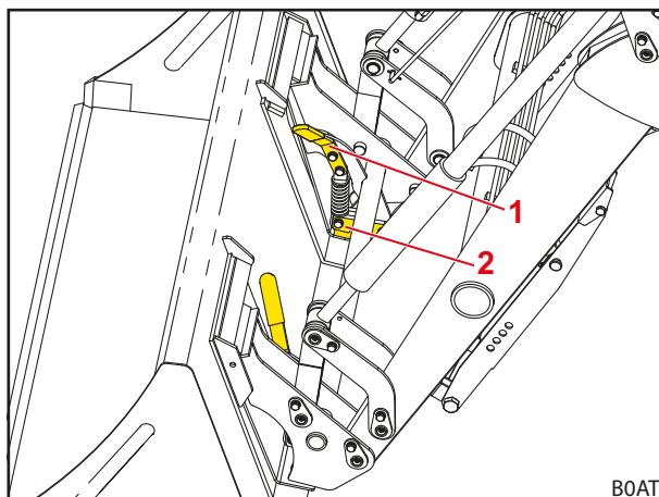
Rys. 61 Mechaniczna blokada osprzętu Skid-Steer (stan zablokowania z osprzętem)
