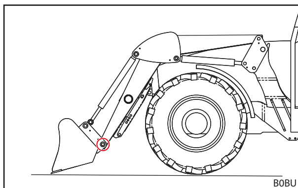
Rys. 79 Łączenie osprzętu w dolnych otworach na sworznie
