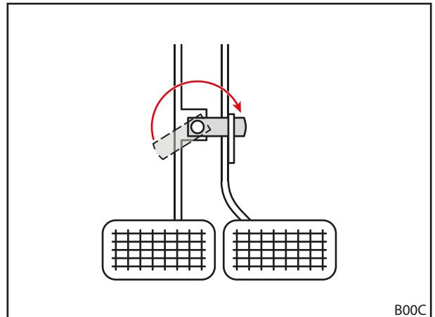
Rys. 33 Łączenie pedałów hamulca
