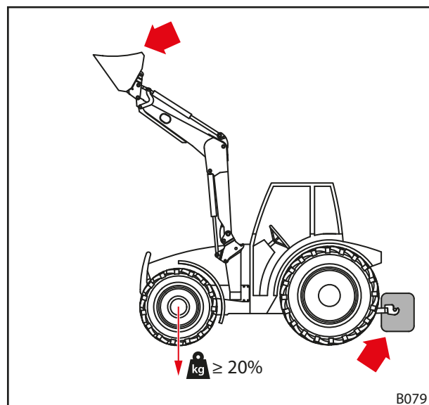
Rys. 35 Obciążenie podczas jazdy po drogach
