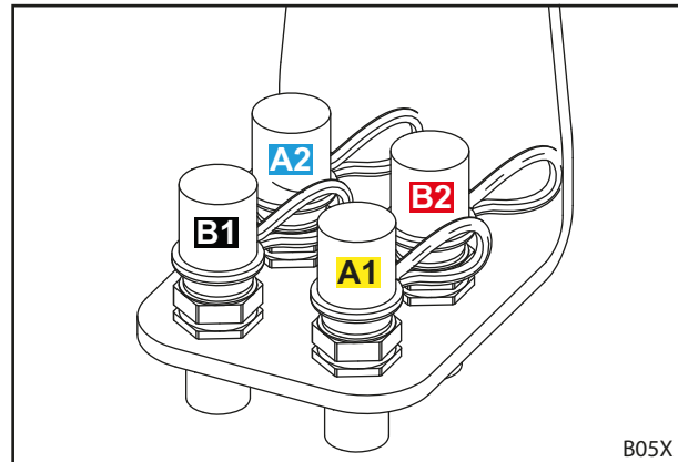
Rys. 14 Wtyki złączek wtykowych przy elemencie montażowym
