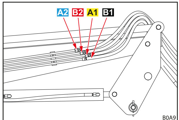
Rys. 13 Przewody hydrauliczne
