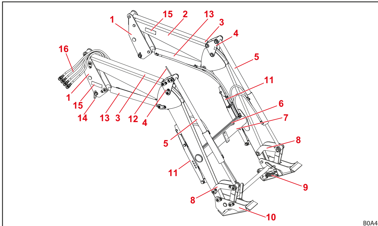
Rys. 8 Ładowacz czołowy P (rysunek przykładowy)
