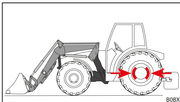
Rys. 83 Ustawianie osprzętu przed odłożeniem i zaciągnięcie hamulca postojowego
