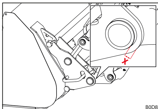
Rys. 100 Wymiar zużycia ramki wymiennej
