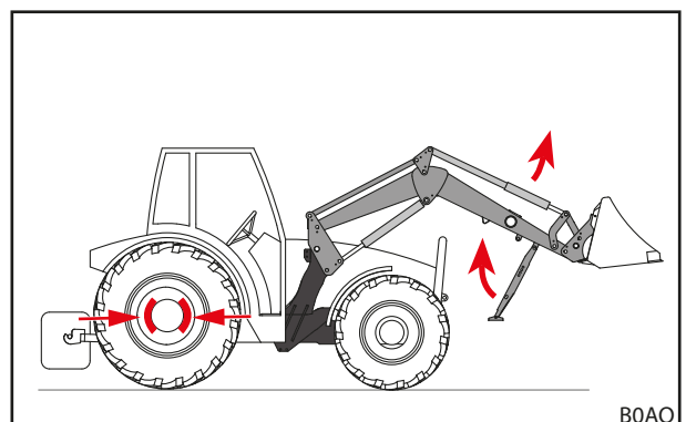
Rys. 41 Składanie podpór
