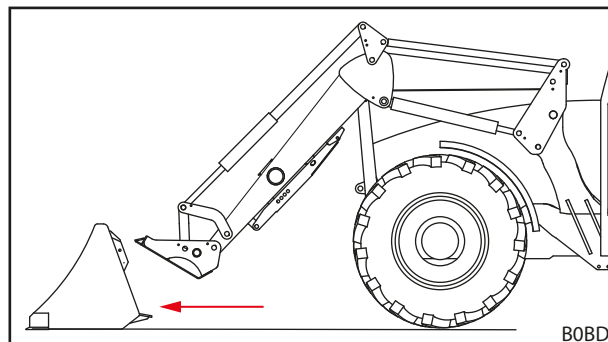
Rys. 68 Dojeżdżanie
