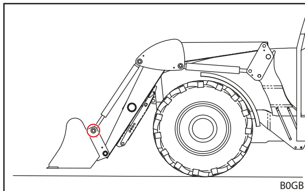
Rys. 88 Wysuwanie górnych sworzni
