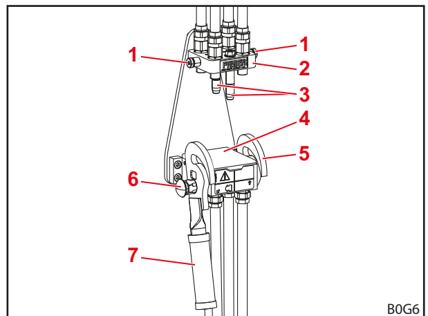
Rys. 54 Odłączona złączka Hydro-Fix
