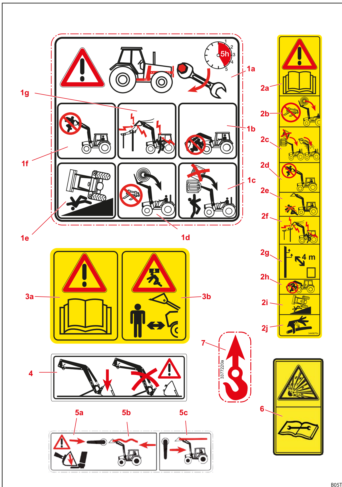
Rys. 5 Naklejki bezpieczeństwa
