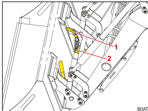
Rys. 67 Otwieranie blokady osprzętu
