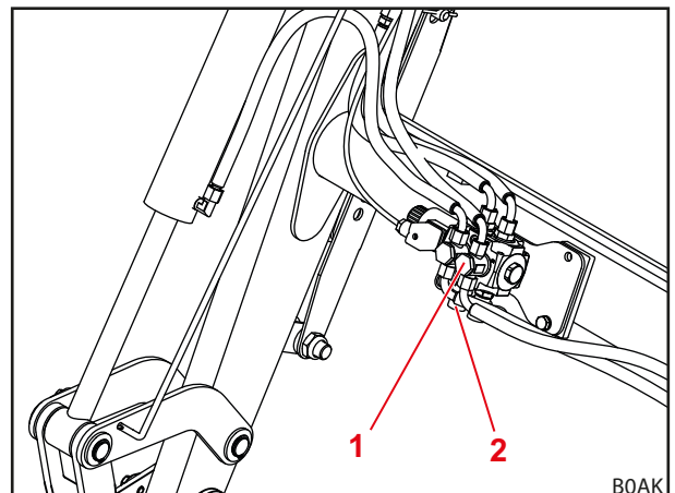
Rys. 30 Dodatkowy 3. obwód sterowniczy
