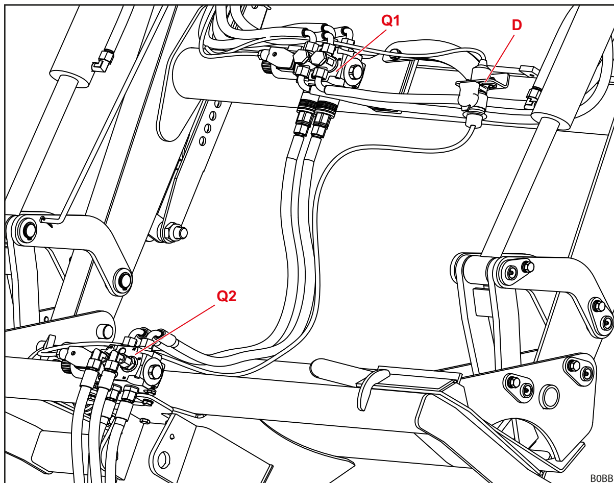
Rys. 107 Rozmieszczenie zaworów hydraulicznych funkcji dodatkowych
