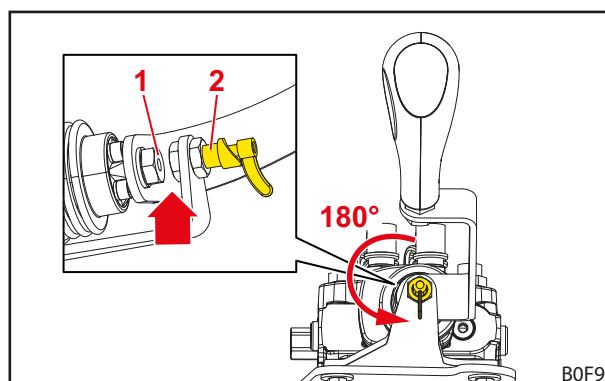
Rys. 49 Odblokowana dźwignia obsługi
