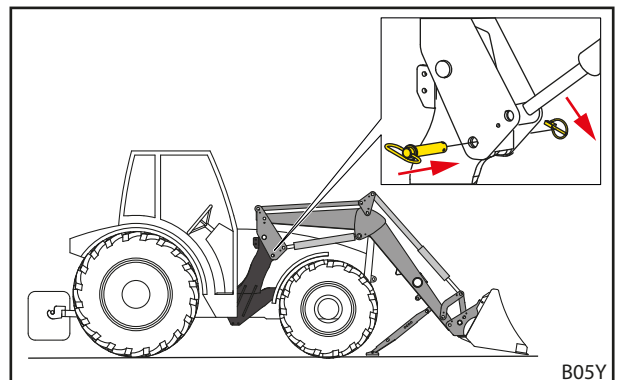
Rys. 40 Zakładanie sworznia blokującego i zabezpieczanie składaną zawleczką
