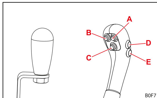
Rys. 47 Dźwignia obsługi bez przycisków (z lewej) i dźwignia obsługi z 5 przyciskami (z prawej)
