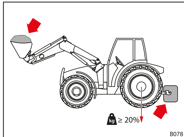
Rys. 34 Balast przy pracach z użyciem ładowacza czołowego
