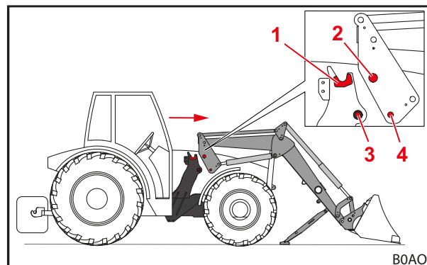
Rys. 38 Wjeżdżanie ciągnikiem w wysięgnik
