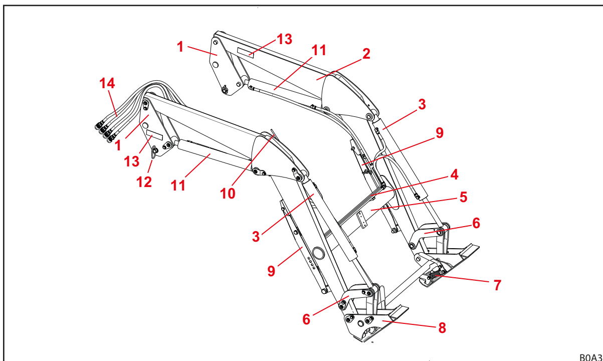
Rys. 7 Ładowacz czołowy H (rysunek przykładowy)
