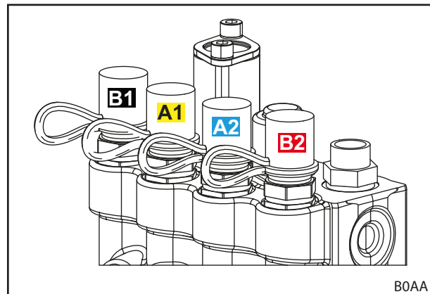
Rys. 15 Wtyki złączek wtykowych bezpośrednio przy zaworze hydraulicznym
