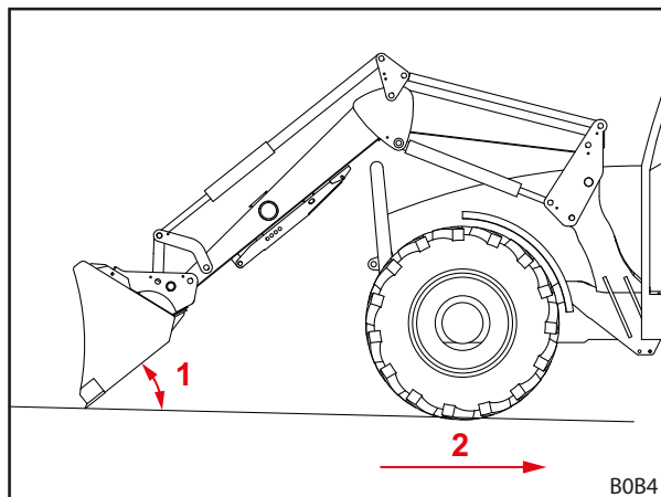
Rys. 91 Równanie do tyłu
