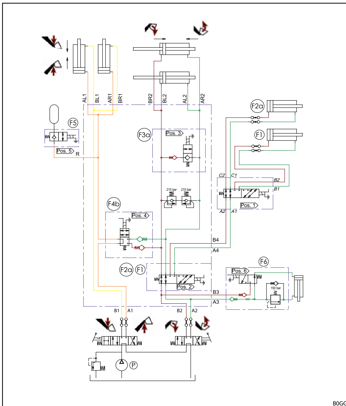
Rys. 155 Schemat hydrauliczny FZ i FZ-L (w przypadku wyposażenia z 3. i 4. obwodem sterowniczym)
