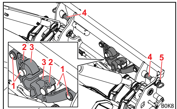
Rys. 115 Adapter w pozycji parkowania (ramka wymienna przygotowana pod osprzęt Euro)
