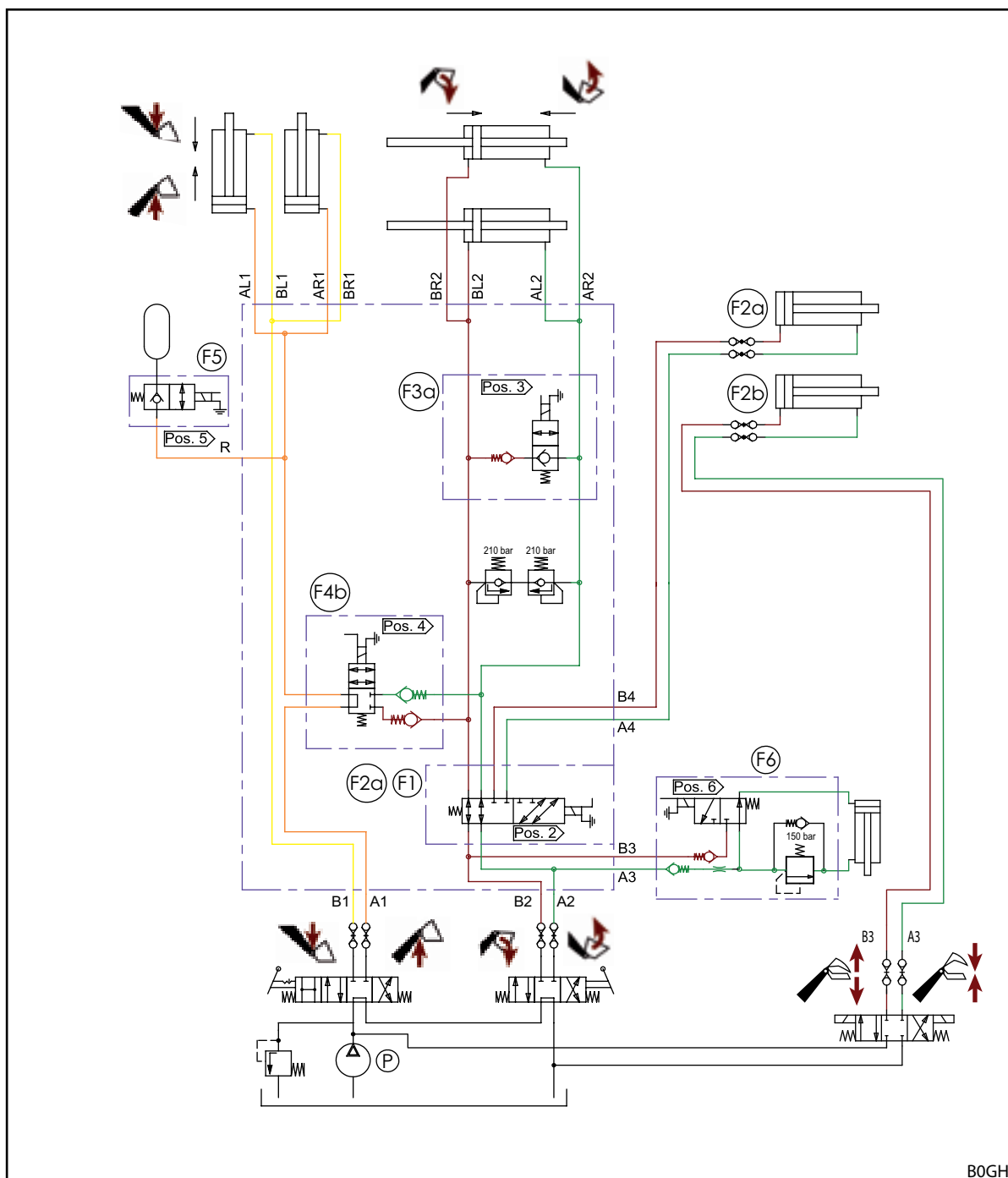
Rys. 156 Schemat hydrauliczny FZ i FZ-L (w przypadku wyposażenia z REAL 3 )
