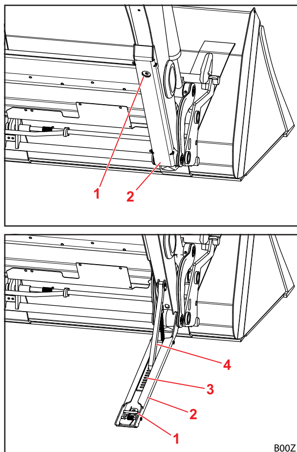
Rys. 91 Podpora
