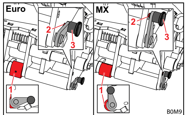
Rys. 114 Pozycje miniaturowego zatrzasku
