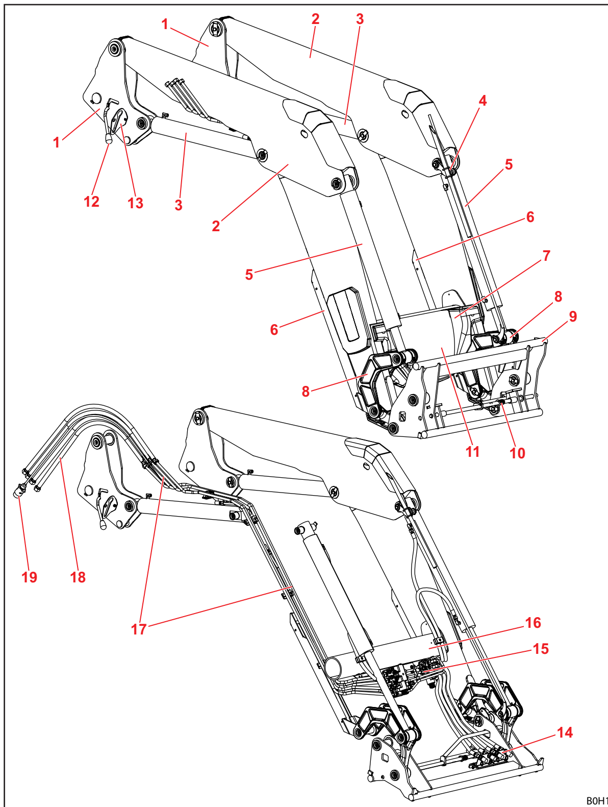
Rys. 9 Ładowacz czołowy FS
