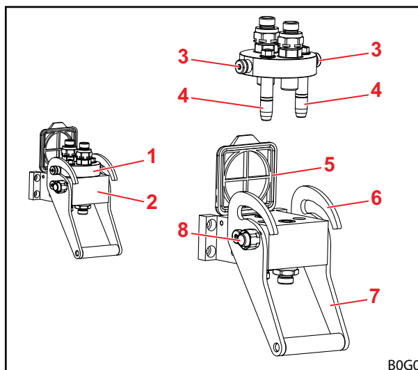
Rys. 28 Budowa osprzęt Fix
