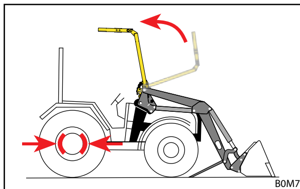
Rys. 64 Podnoszenie konstrukcji OPG
