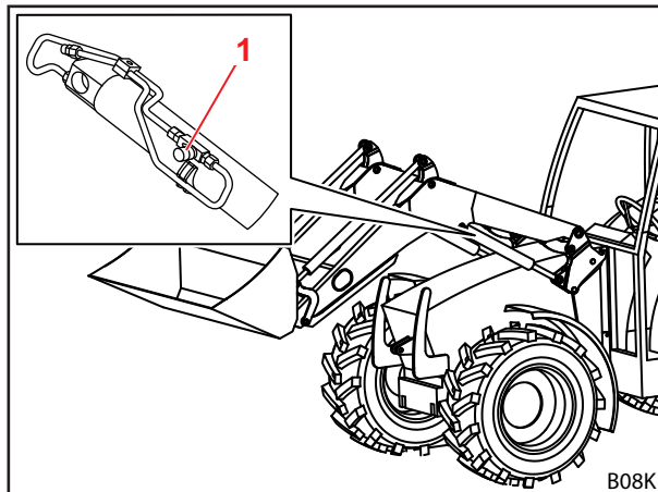
Rys. 52 Dławik opuszczania
