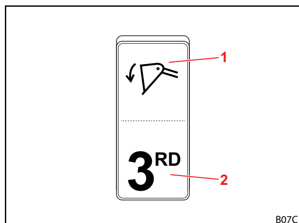
Rys. 86 Przełącznik szybkiego opróżniania i 3. obwodu sterowniczego
