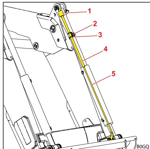
Rys. 40 Czujnik Return-To-Level przy wskaźniku
