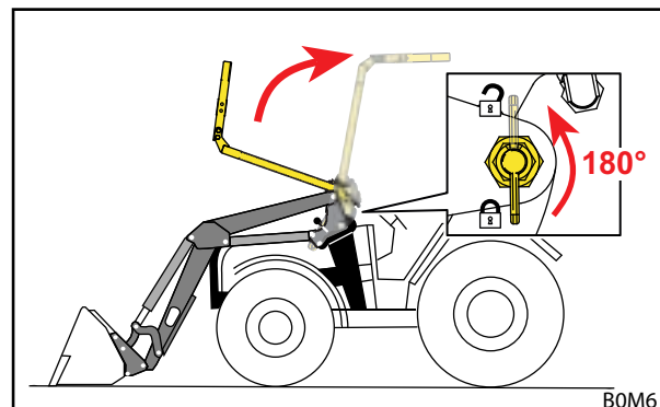
Rys. 44 Podnoszenie konstrukcji OPG
