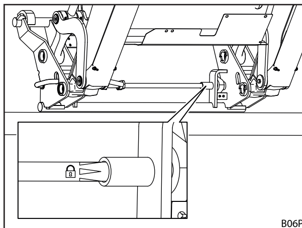
Rys. 98 Kontrola blokady osprzętu za pomocą naklejki
