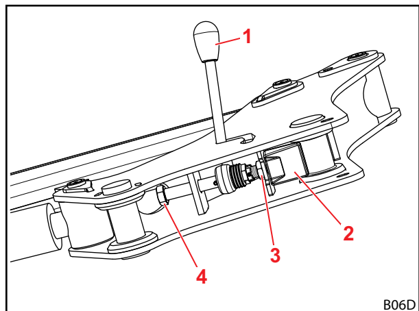
Rys. 71 Widok blokady ładowacza czołowego od dołu
