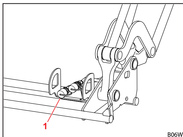
Rys. 46 Dodatkowy 3. obwód sterowniczy
