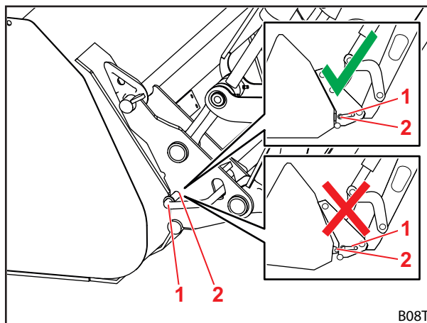
Rys. 100 Kontrola położenia sworzni blokujących
