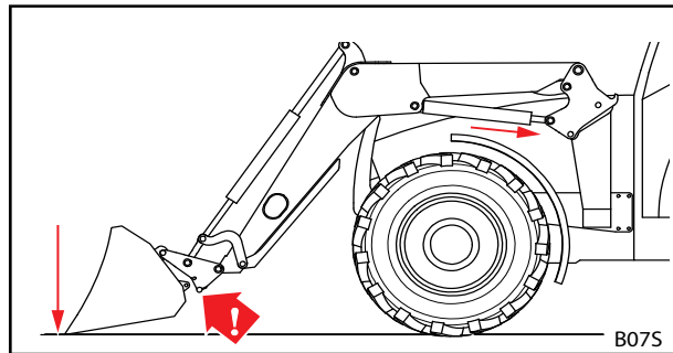
Rys. 109 Dociskanie osprzętu do podłoża
