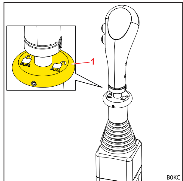
Rys. 81 Blokada dźwigni obsługi (pionowa blokada)
