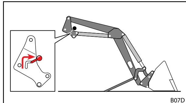
Rys. 61 Otwieranie blokady ładowacza czołowego
