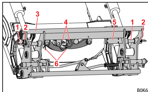
Rys. 17 Kombinowana ramka wymienna Euro-MX (przygotowana pod osprzęt Euro)
