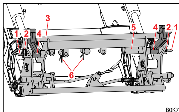
Rys. 18 Kombinowana ramka wymienna Euro-MX (przygotowana pod osprzęt MX)
