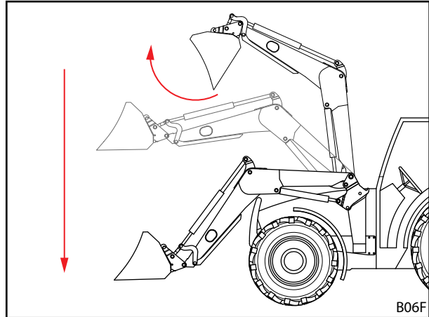
Rys. 39 Funkcja Return-To-Level
