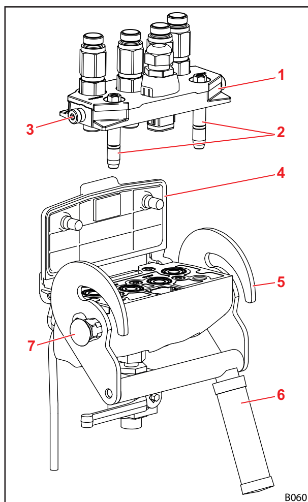
Rys. 94 Hydro-Fix (przykład: Hydro-Fix 4-złączkowy)
