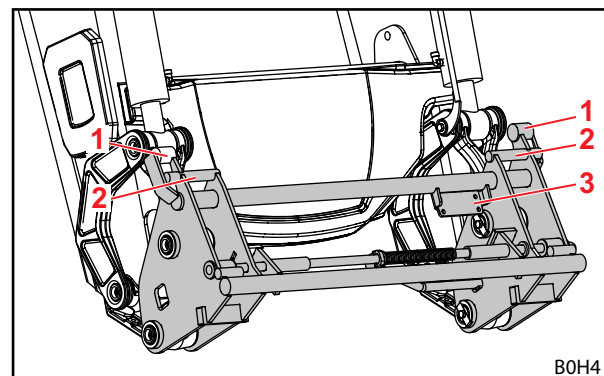
Rys. 16 Kombinowana ramka wymienna Euro-Alö3
