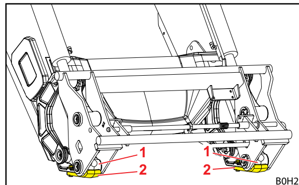
Rys. 20 Płozy trudnościeralne
