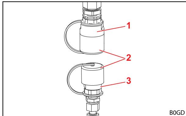
Rys. 93 Złączki gwintowane (rysunek przykładowy)
