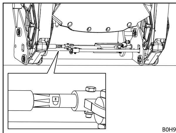
Rys. 106 Kontrola blokady osprzętu za pomocą naklejki
