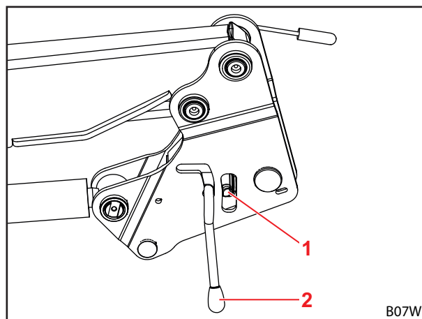
Rys. 144 Kontrola blokady ładowacza czołowego
