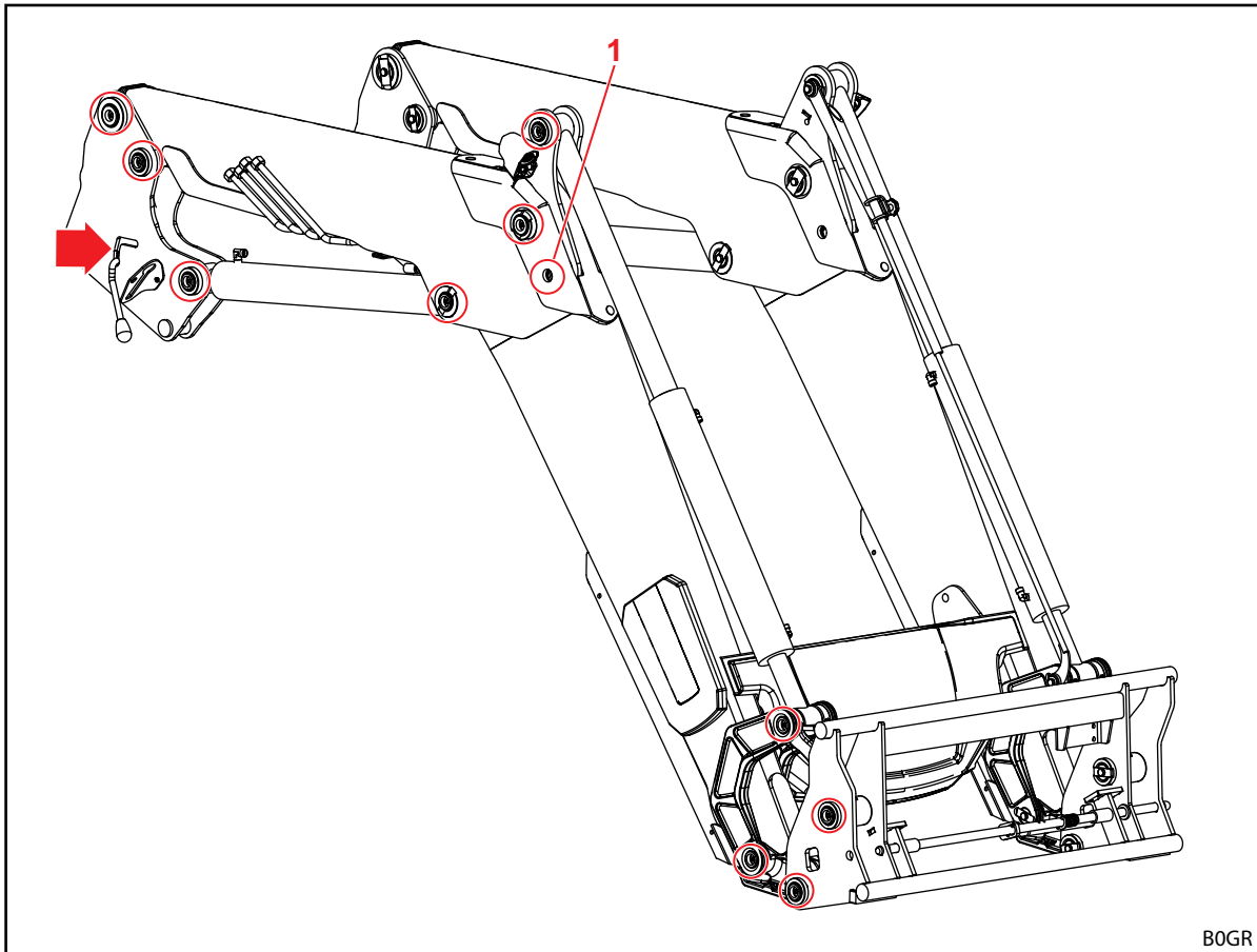
Rys. 141 Punkty smarowania FZ
