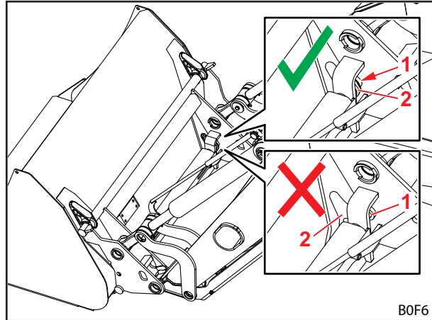
Rys. 108 Kontrola położenia sworzni blokujących
