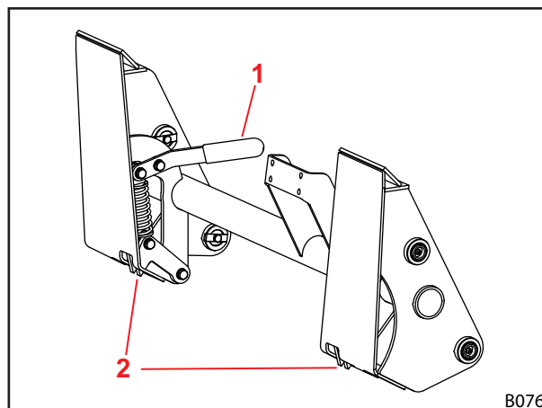
Rys. 102 Blokada osprzętu przy ramce wymiennej Skid-Steer
