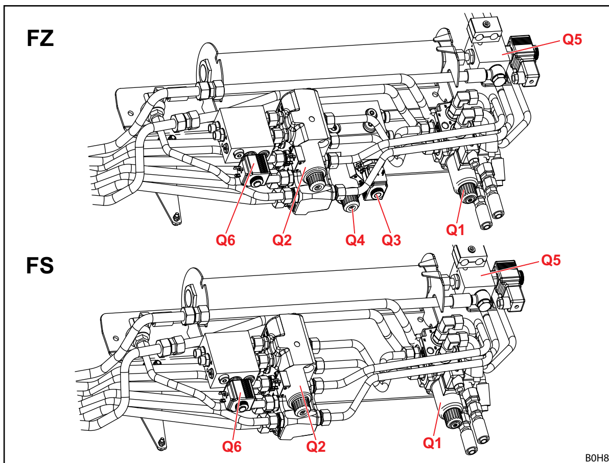
Rys. 161 Rozmieszczenie zaworów hydraulicznych funkcji dodatkowych
