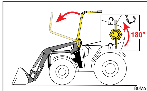
Rys. 42 Opuszczanie konstrukcji OPG
