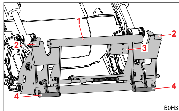
Rys. 14 Kombinowana ramka wymienna Euro-SMS (przygotowana pod osprzęt Euro)
