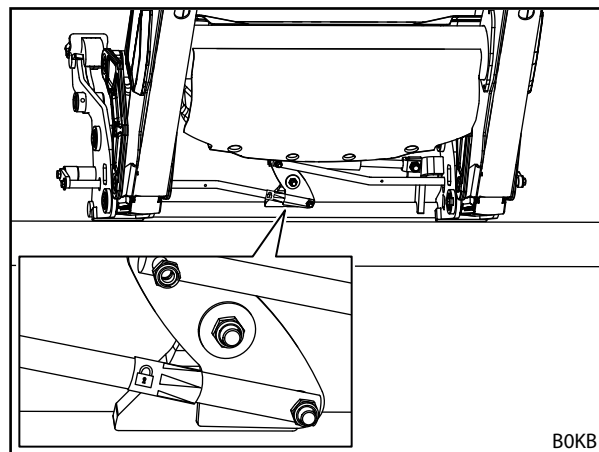
Rys. 107 Kontrola blokady osprzętu za pomocą naklejki
