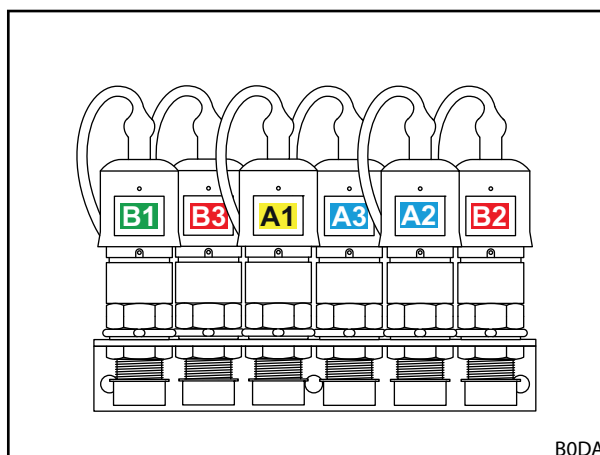
Rys. 24 Złączki wtykowe połączone (opcja REAL 3 )
