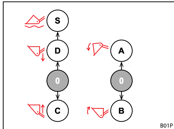
Rys. 78 Przyporządkowanie w przypadku 2 dźwigni obsługi
