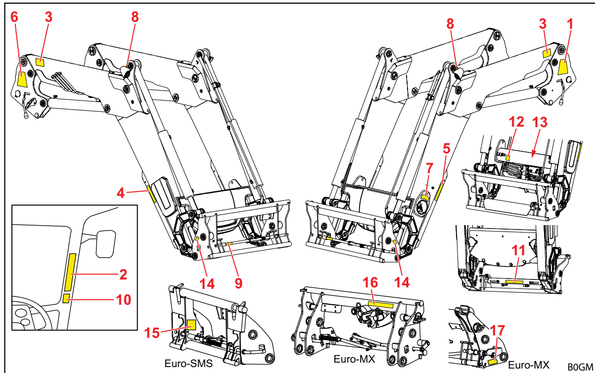
Rys. 4 Ładowacz czołowy FZ (rysunek przykładowy)
