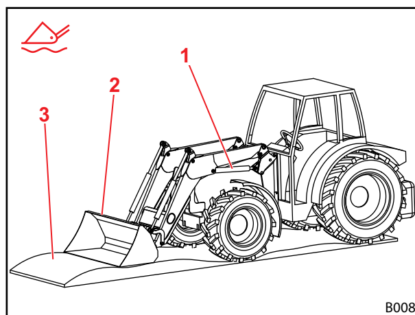
Rys. 35 Ładowacz czołowy w pozycji pływającej
