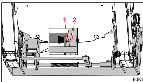
Rys. 113 Uniesione ograniczniki (widok od tyłu)
