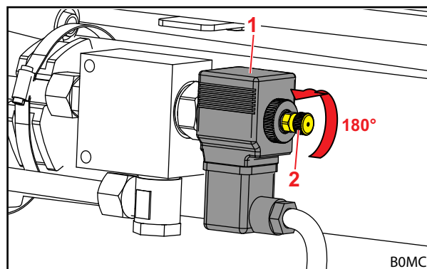
Rys. 41 Otwieranie zaworu
