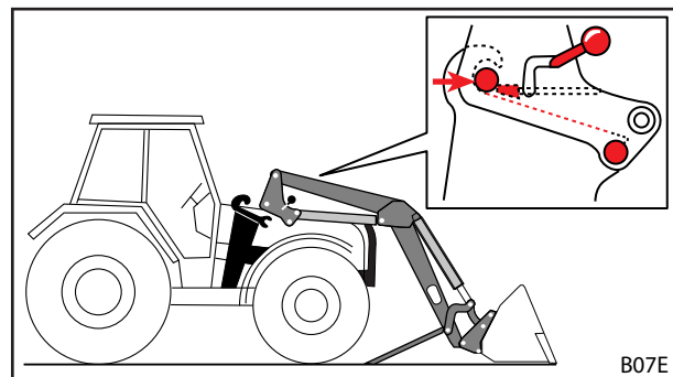
Rys. 62 Wjeżdżanie ciągnikiem w wysięgnik
