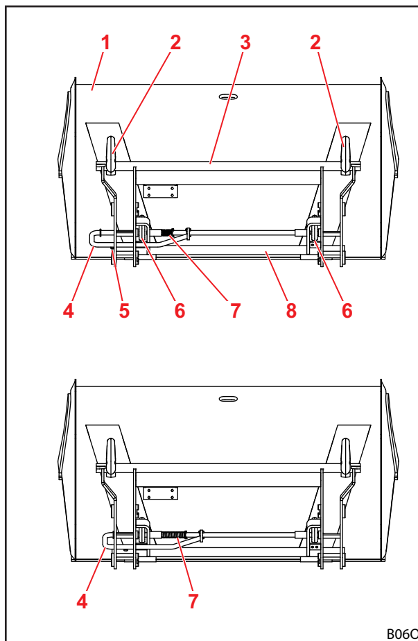
Rys. 29 Otwarta (u góry) i zamknięta (na dole) blokada
