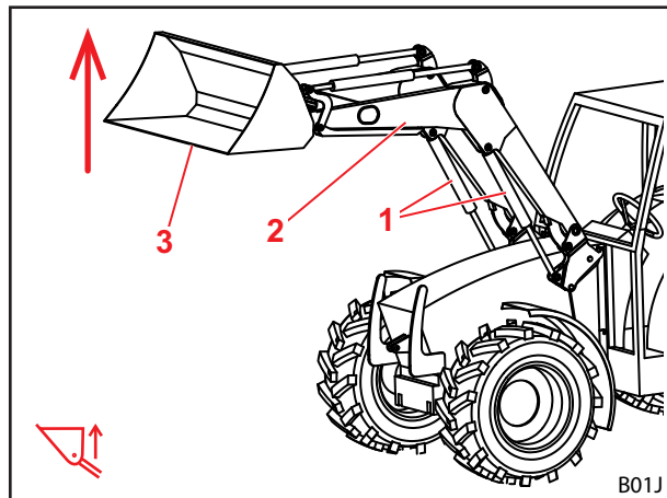
Rys. 31 Funkcja podnoszenia
