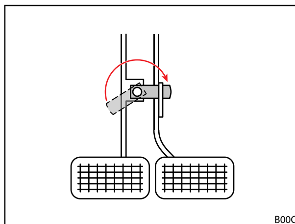
Rys. 57 Łączenie pedałów hamulca
