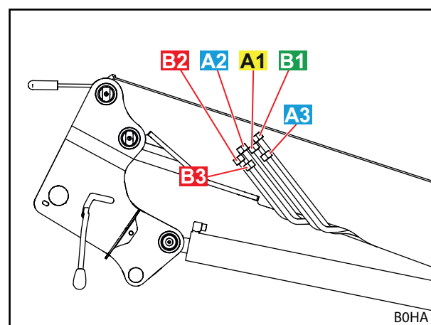
Rys. 22 Przewody hydrauliczne (opcja REAL 3 )
