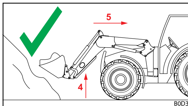
Rys. 138 Cofanie z ładunkiem – dobrze
