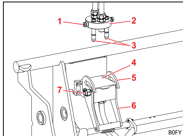
Rys. 95 Odłączone osprzęt Fix
