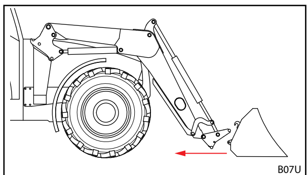
Rys. 132 Odjeżdżanie
