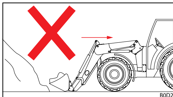
Rys. 137 Cofanie z ładunkiem – źle
