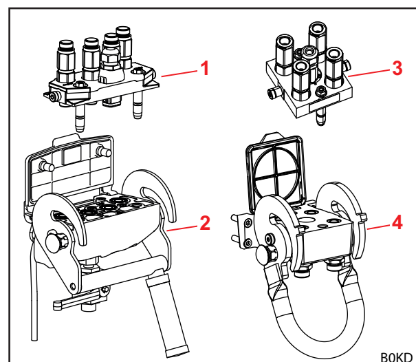
Rys. 26 Budowa Hydro-Fix i multizłącza
