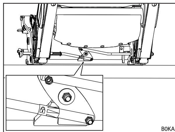
Rys. 99 Kontrola blokady osprzętu za pomocą naklejki (kombinowana ramka wymienna Euro-MX)
