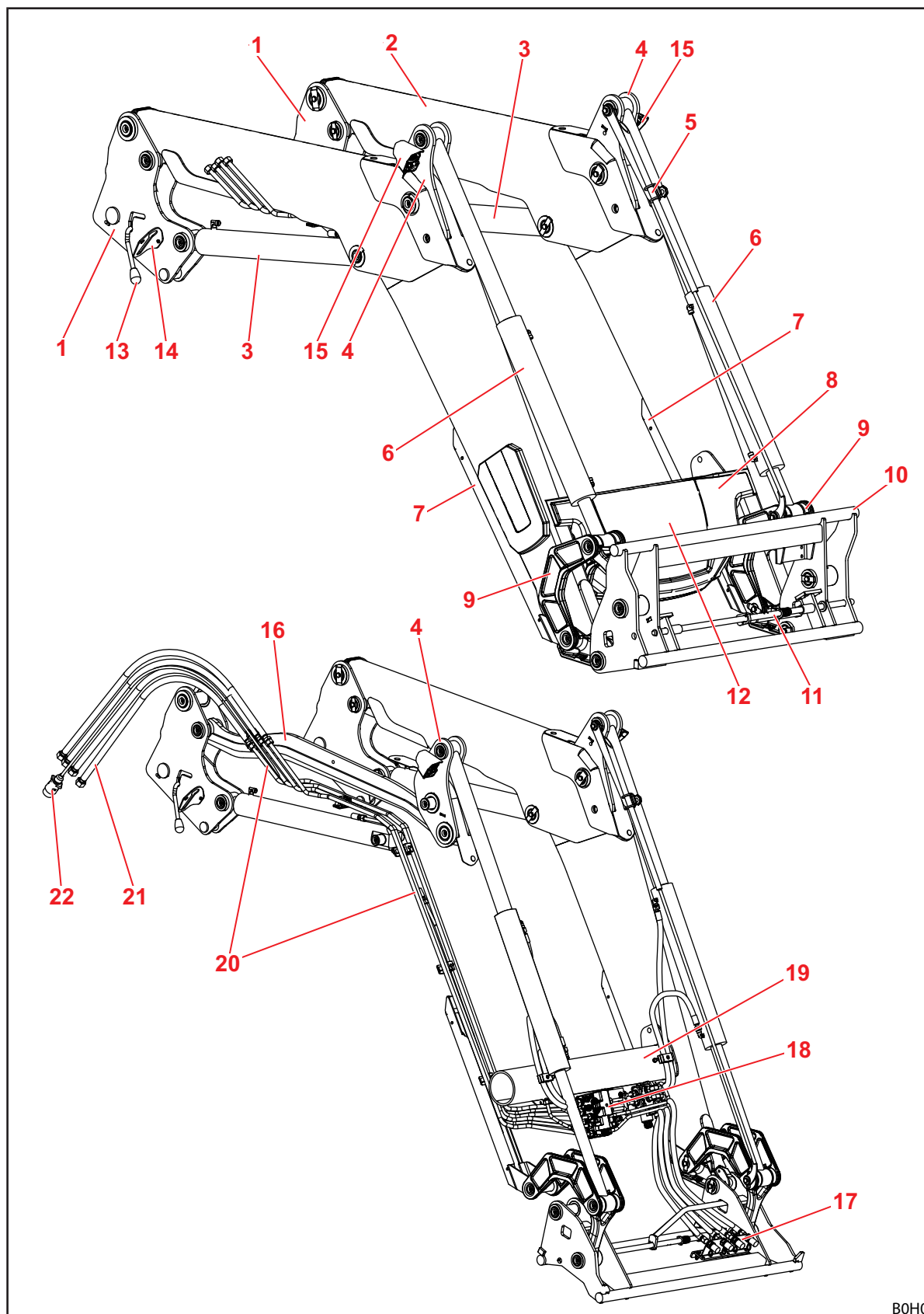
Rys. 10 Ładowacz czołowy FZ
