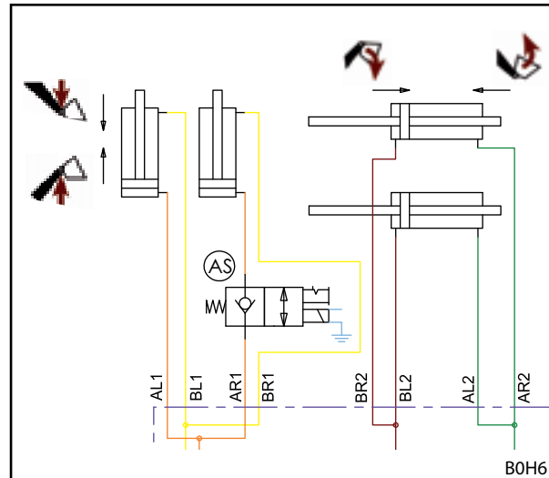
Rys. 157 Schemat hydrauliczny zabezpieczenia przed opadnięciem
