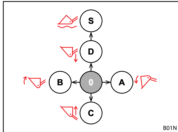
Rys. 77 Przyporządkowanie w przypadku jednej dźwigni obsługi
