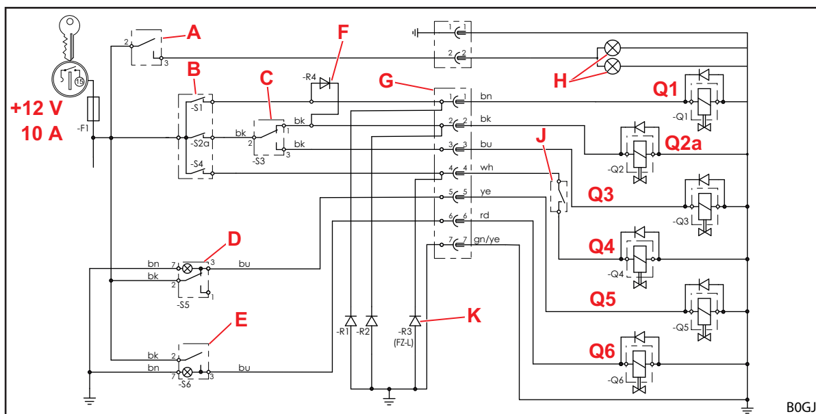
Rys. 159 Schemat elektryczny (w przypadku wyposażenia z 3. i 4. obwodem sterowniczym)
