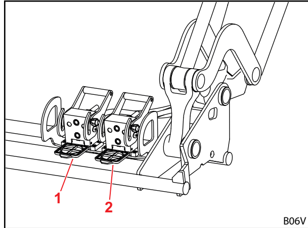
Rys. 47 Dodatkowy 4. obwód sterowniczy
