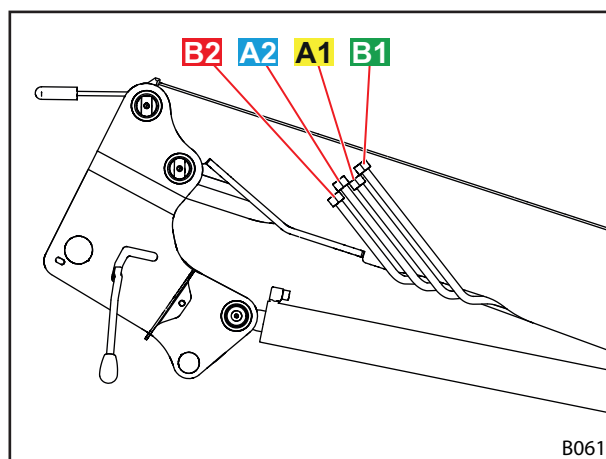
Rys. 21 Przewody hydrauliczne
