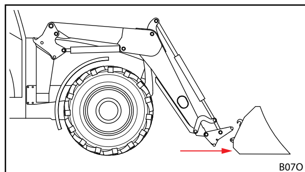
Rys. 127 Dojeżdżanie
