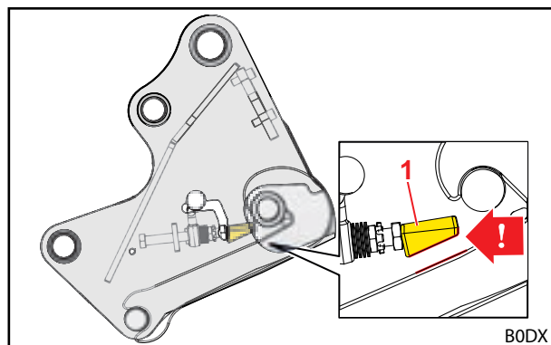
Rys. 67 Poprawne położenie montażowe klina zaciskowego
