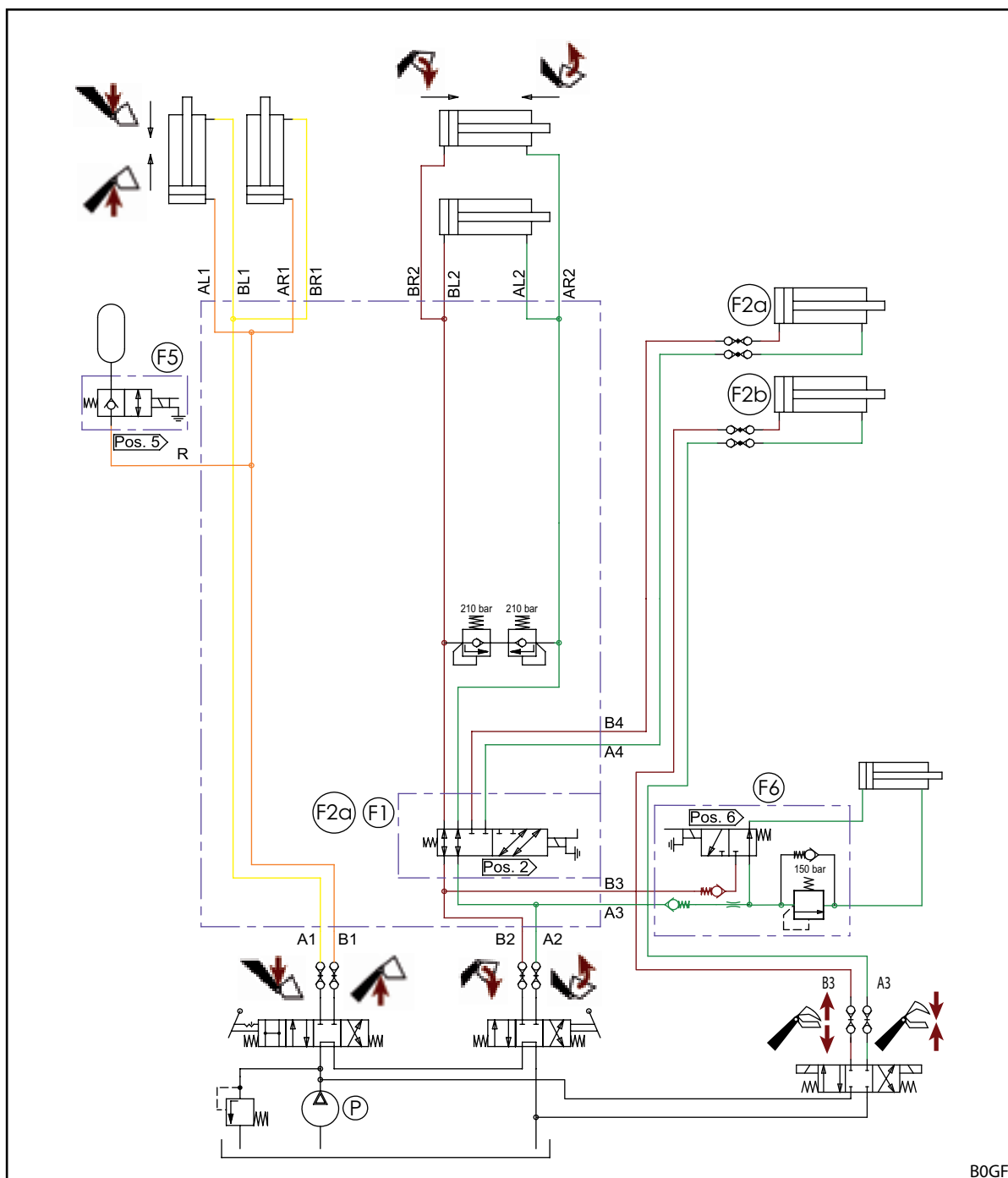
Rys. 154 Schemat hydrauliczny FS (w przypadku wyposażenia z REAL 3 )
