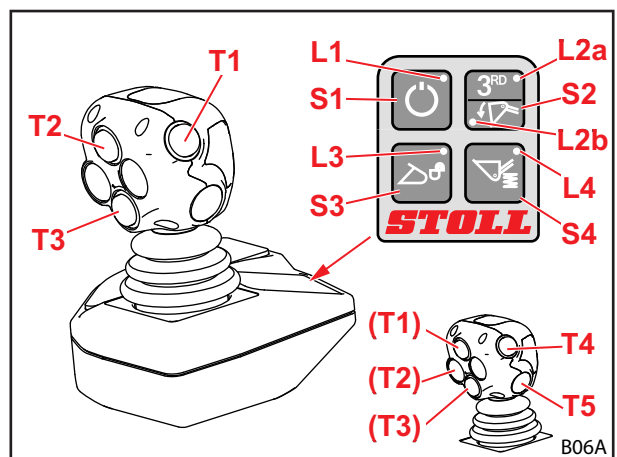
Rys. 83 STOLL Pro Control
