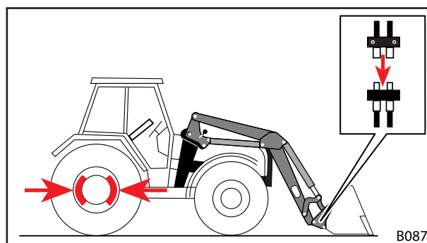
Rys. 122 Łączenie przewodów hydraulicznych osprzętu ze złączkami ładowacza czołowego
