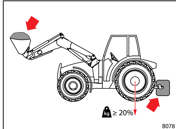
Rys. 58 Balast przy pracach z użyciem ładowacza czołowego
