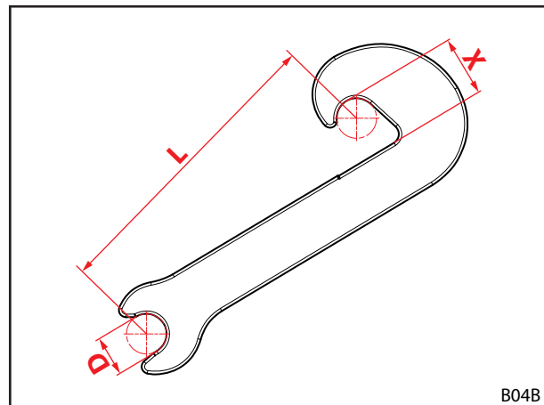
Rys. 142 Wymiary zużycia haka
