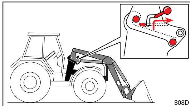
Rys. 148 Zwalnianie blokady ładowacza czołowego
