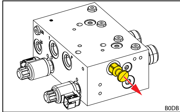
Rys. 89 Wyciąganie zaworu upustowego na zaworze REAL 3
