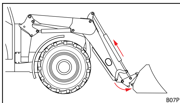
Rys. 125 Zaczepianie
