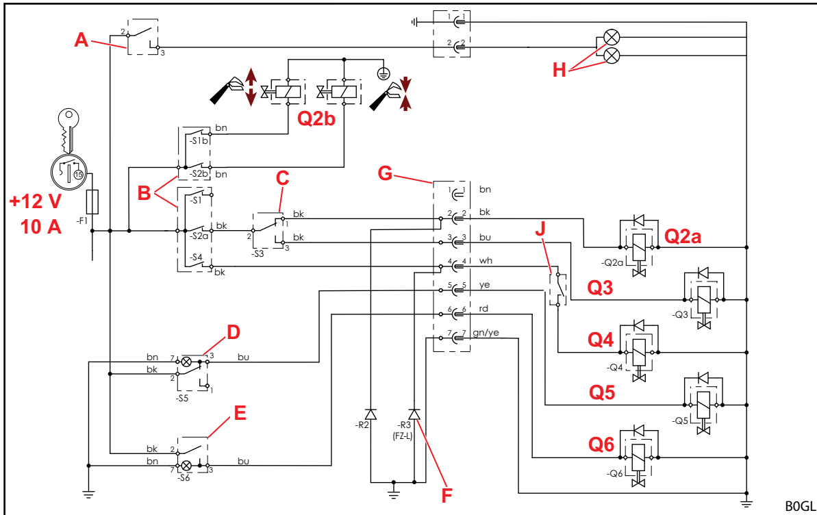
Rys. 160 Schemat elektryczny (w przypadku wyposażenia z REAL 3 )
