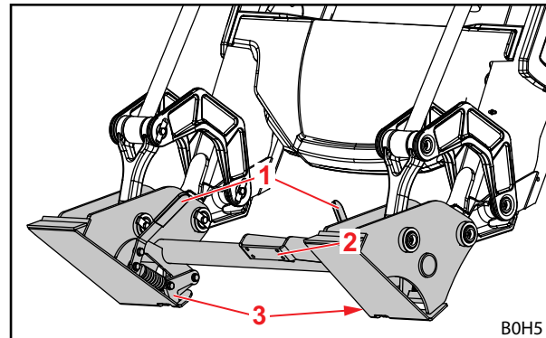
Rys. 19 Ramka wymienna Skid-Steer
