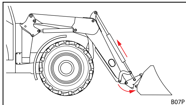
Rys. 120 Zaczepianie
