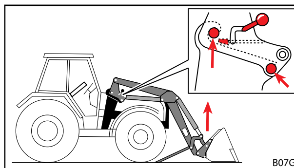
Rys. 65 Użycie funkcji Podnoszenie w celu objęcia sworzni ładowacza czołowego hakami
