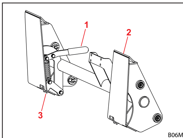
Rys. 30 Obsługa mechanicznej blokady osprzętu przy ramce wymiennej Skid-Steer
