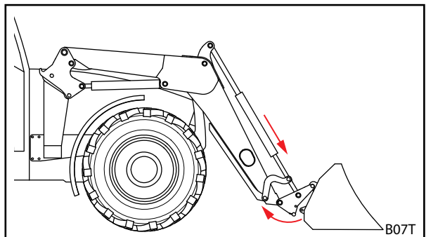
Rys. 131 Odczepianie ramki wymiennej
