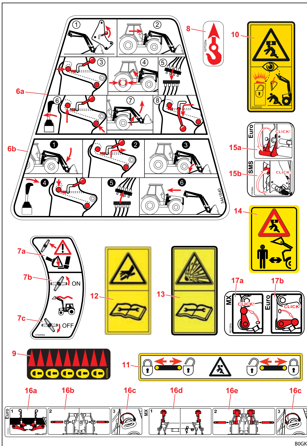
Rys. 6 Naklejki bezpieczeństwa, pozycja 6–17
