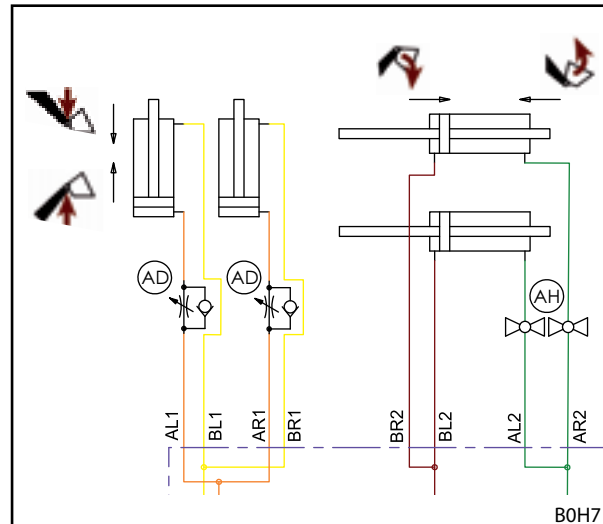
Rys. 158 Schemat hydrauliczny dławika opuszczania
