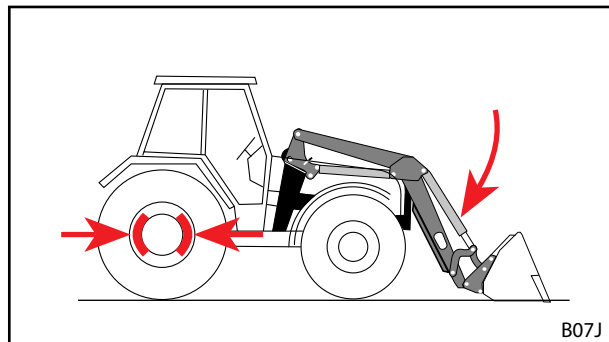
Rys. 147 Zaciągnąć hamulec postojowy i opuścić ładowacz czołowy.
