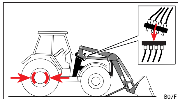
Rys. 63 Wyłączanie ciągnika i podłączanie przewodów hydraulicznych
