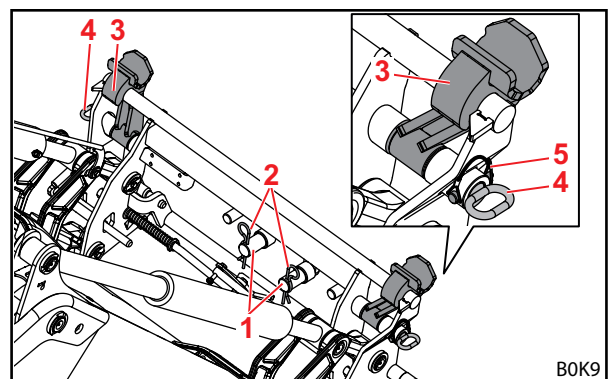
Rys. 116 Adapter w pozycji roboczej (ramka wymienna przygotowana pod osprzęt MX)
