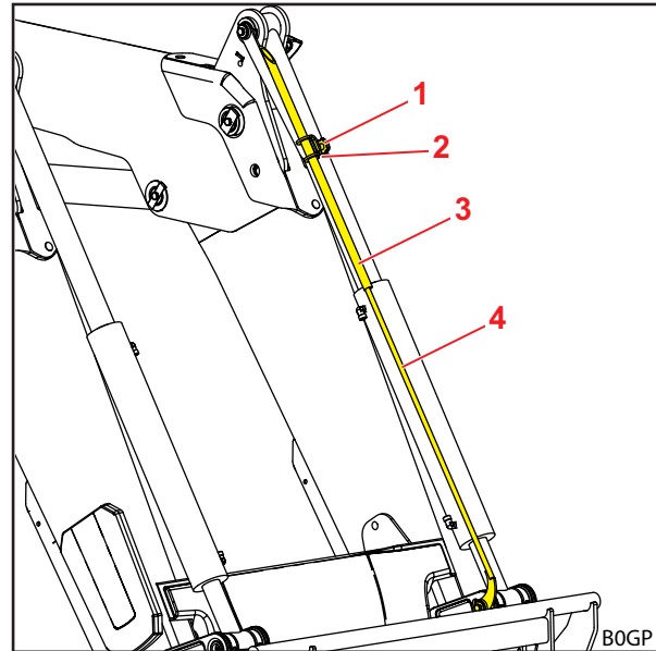
Rys. 36 Wskaźnik pozycji osprzętu
