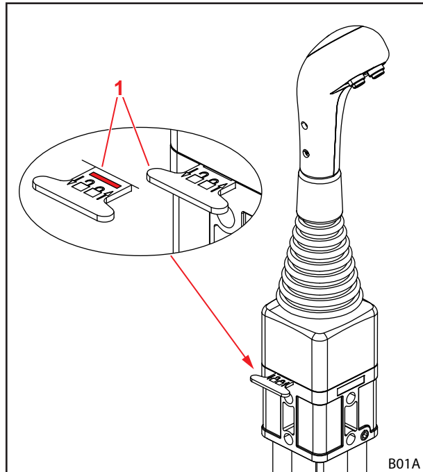
Rys. 80 Blokada dźwigni obsługi (pozioma blokada)
