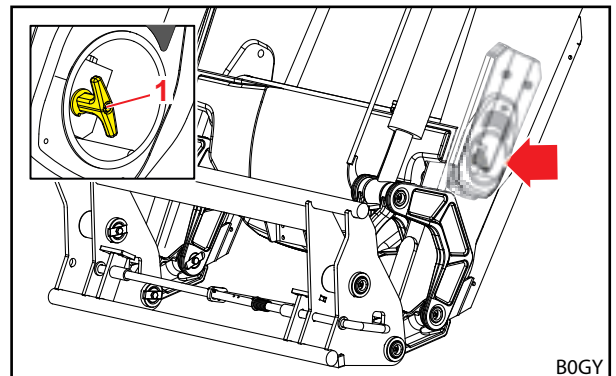
Rys. 49 Mechanicznie sterowany Comfort Drive
