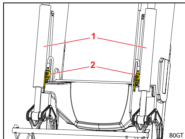
Rys. 53 Zawory odcinające na siłownikach osprzętu
