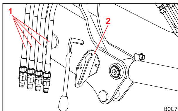
Rys. 152 Zawieszanie przewodów hydraulicznych w uchwycie złącza (widok ze złączkami wtykowymi)
