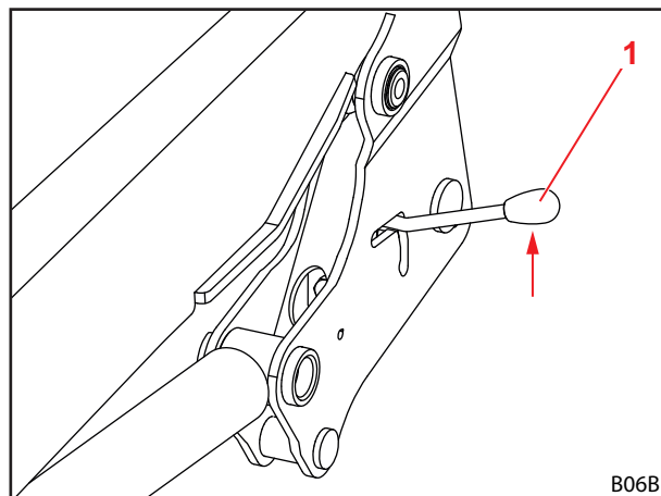
Rys. 68 Otwieranie blokady ładowacza czołowego
