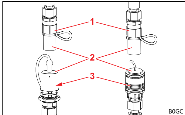
Rys. 92 Złączki wtykowe (przykładowe rysunki)
