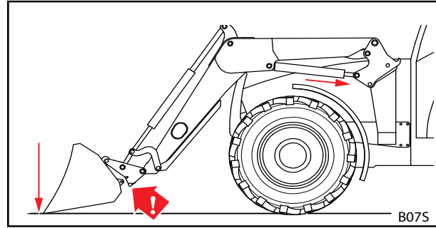
Rys. 103 Dociskanie osprzętu do podłoża
