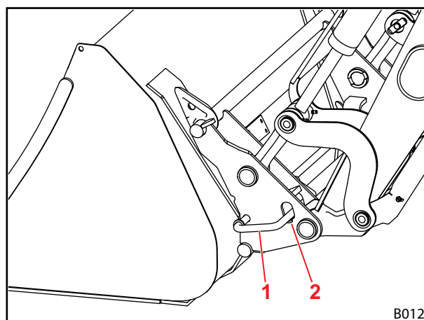
Rys. 97 Mechaniczna blokada osprzętu
