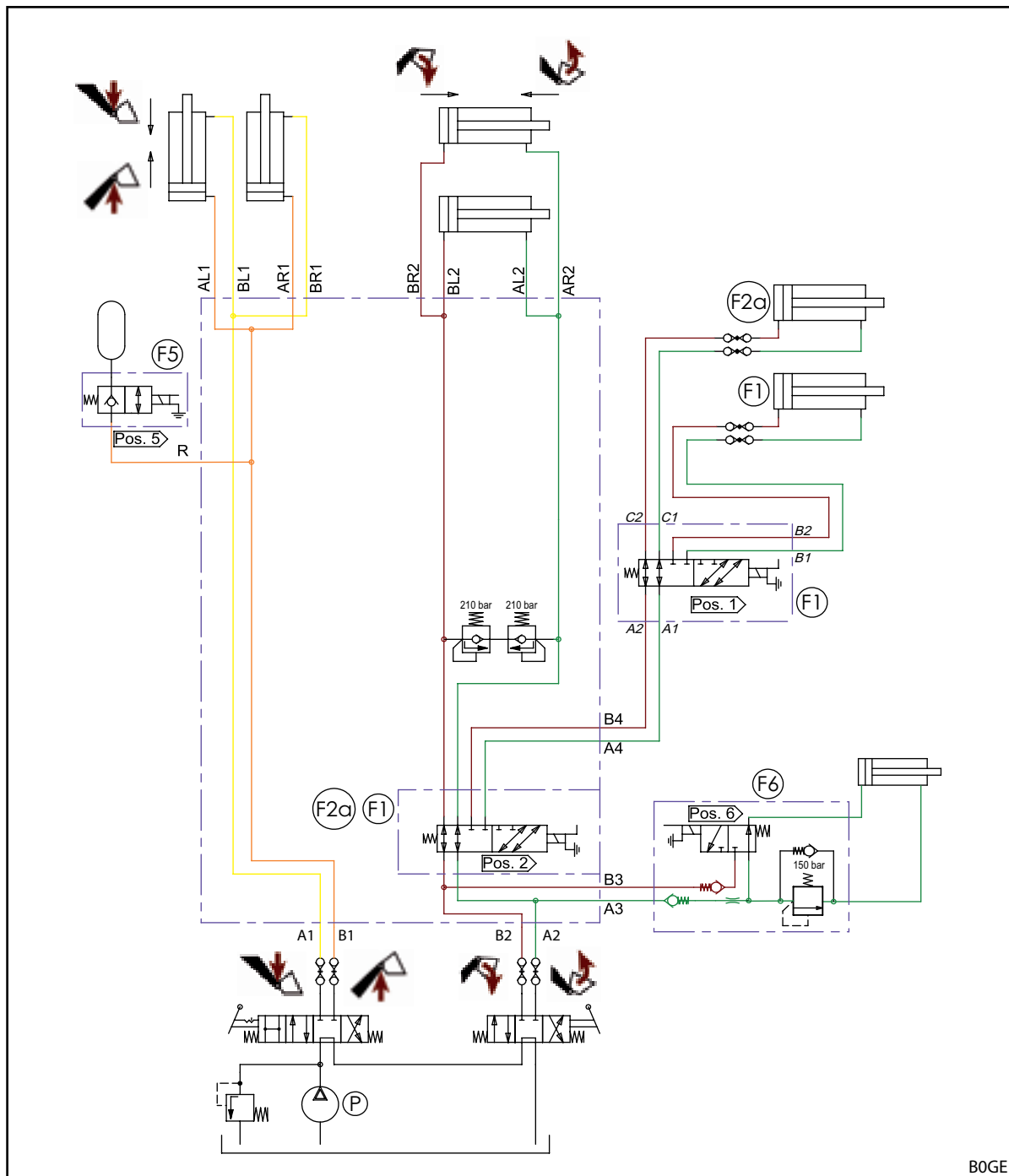
Rys. 153 Schemat hydrauliczny FS (w przypadku wyposażenia z 3. i 4. obwodem sterowniczym)
