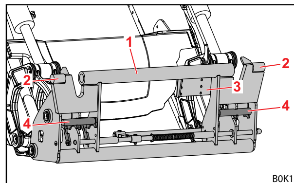
Rys. 15 Kombinowana ramka wymienna Euro-SMS (przygotowana pod osprzęt SMS)
