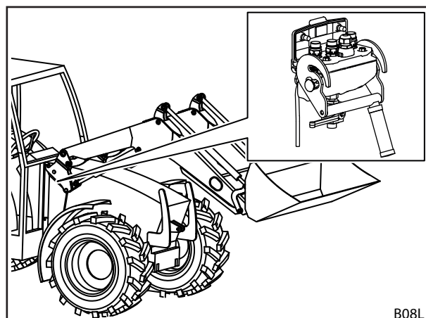
Rys. 25 Hydro-Fix: pozycja na ładowaczu czołowym
