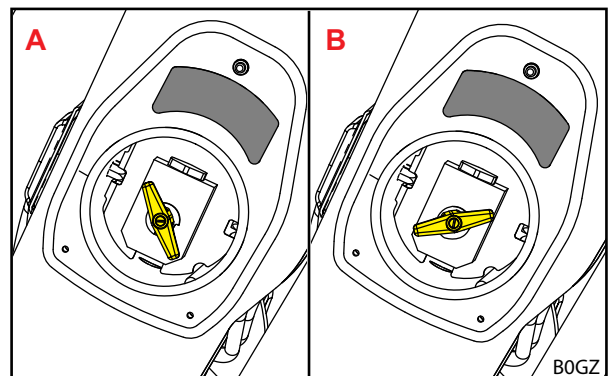
Rys. 50 Pozycje dźwigni Comfort-Drive
