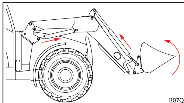
Rys. 121 Zwalniania blokady osprzętu
