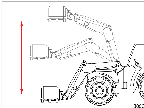
Rys. 37 Mechaniczne prowadzenie równoległe
