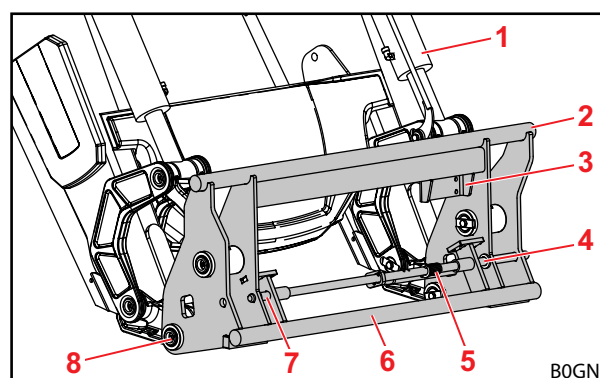
Rys. 13 Ramka wymienna Euro
