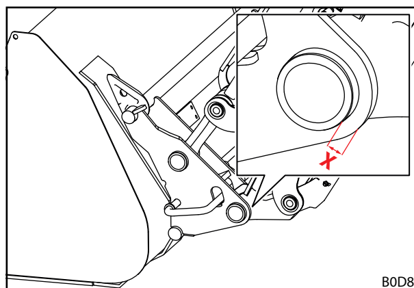
Rys. 146 Wymiar zużycia ramki wymiennej
