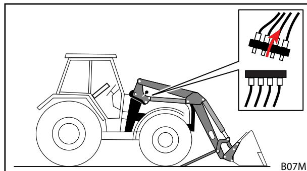
Rys. 150 Odłączanie układu hydraulicznego
