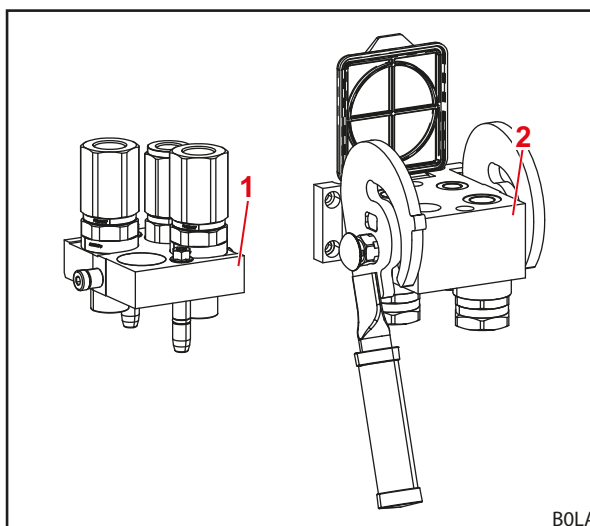
Rys. 19 Budowa Hydro-Fix
