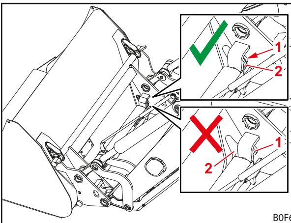
Rys. 84 Kontrola położenia sworzni blokujących
