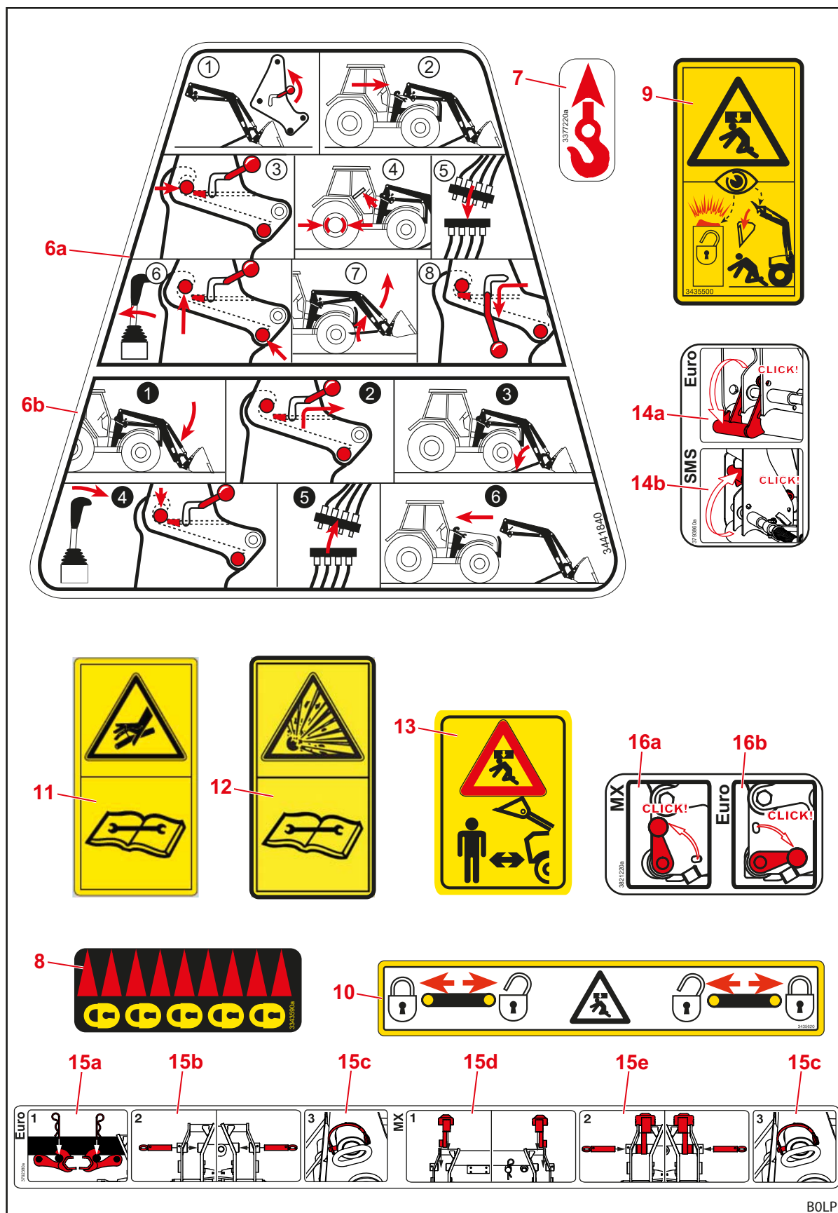
Rys. 6 Naklejki bezpieczeństwa, pozycja 6–16
