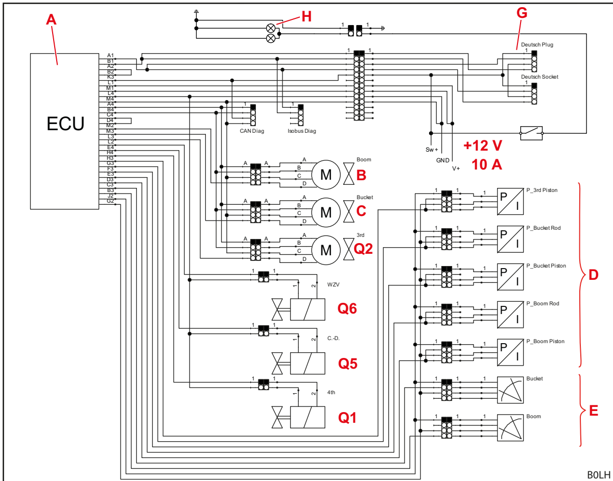
Rys. 127 Schemat elektryczny
