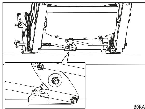
Rys. 78 Kontrola blokady osprzętu za pomocą naklejki (kombinowana ramka wymienna Euro-MX)
