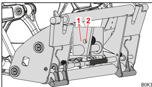
Rys. 87 Opuszczone ograniczniki
