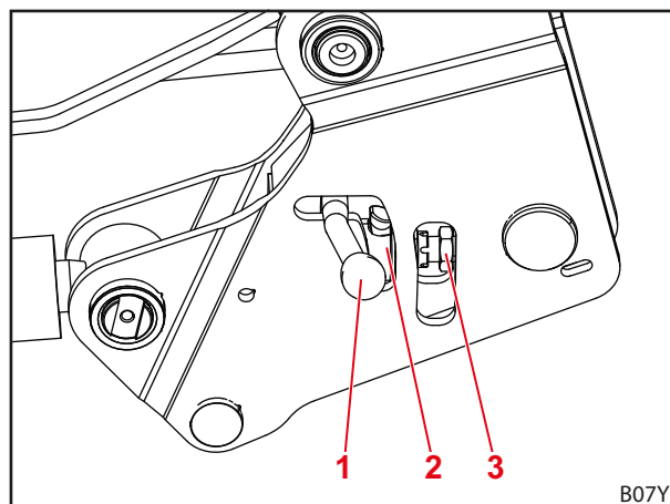
Rys. 62 Otwieranie blokady ładowacza czołowego
