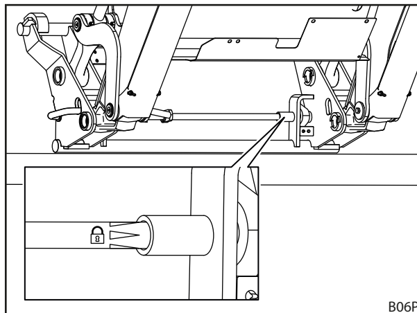
Rys. 77 Kontrola blokady osprzętu za pomocą naklejki
