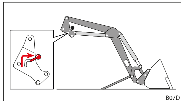
Rys. 52 Otwieranie blokady ładowacza czołowego
