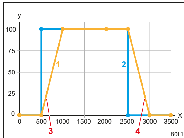
Rys. 31 Regulowana charakterystyka zadziałania
