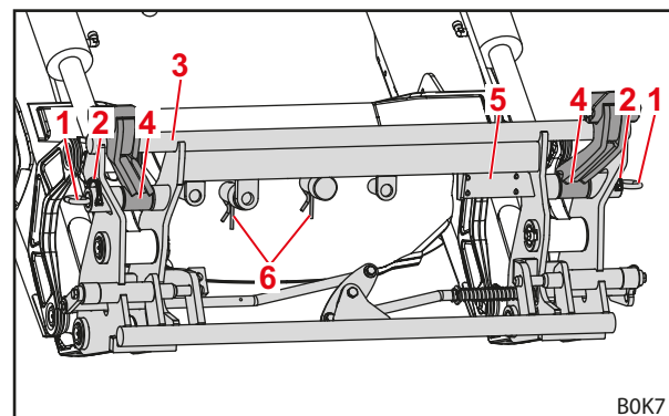
Rys. 14 Kombinowana ramka wymienna Euro-MX (przygotowana pod osprzęt MX)
