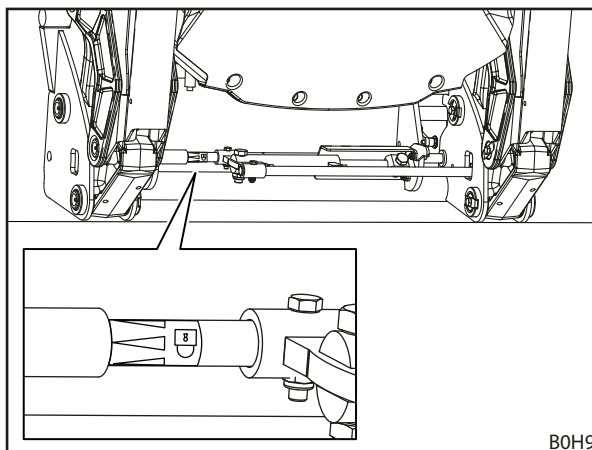
Rys. 82 Kontrola blokady osprzętu za pomocą naklejki
