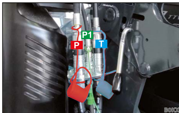
Rys. 17 Podłączone złączki wtykowe
