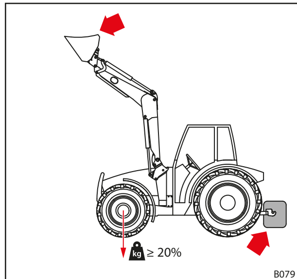
Rys. 50 Obciążenie podczas jazdy po drogach
