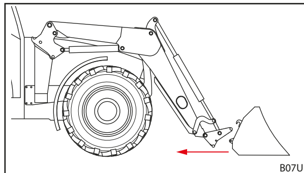
Rys. 104 Odjeżdżanie
