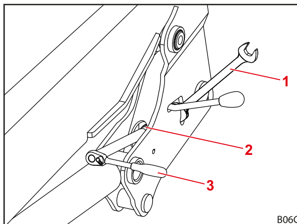
Rys. 59 Przykładanie osprzętu
