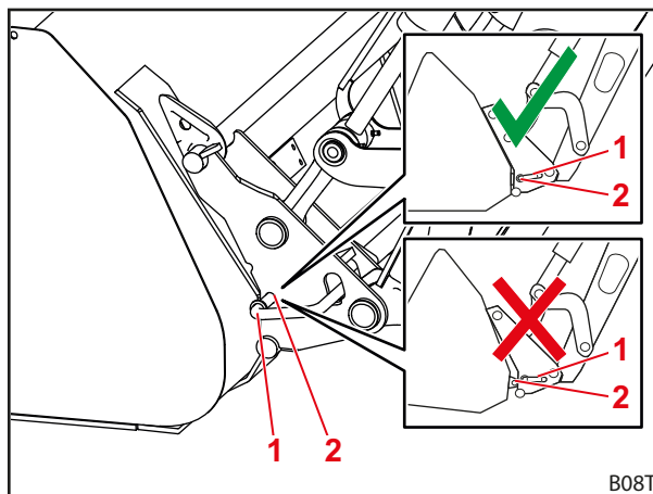
Rys. 79 Kontrola położenia sworzni blokujących
