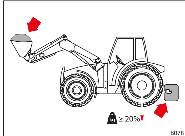
Rys. 49 Balast przy pracach z użyciem ładowacza czołowego
