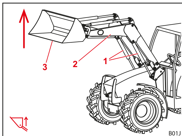
Rys. 23 Funkcja podnoszenia
