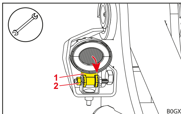
Rys. 47 Ustawianie reflektora w pionie
