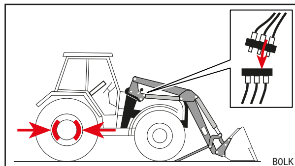
Rys. 54 Wyłączanie ciągnika i podłączanie przewodów hydraulicznych
