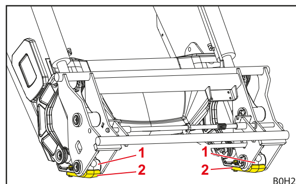
Rys. 15 Płozy trudnościeralne
