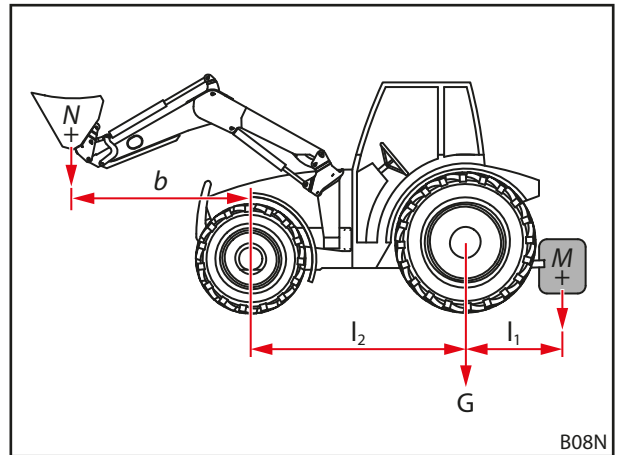
Rys. 51 Obliczanie stabilności statycznej
