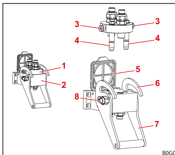
Rys. 21 Budowa osprzęt Fix
