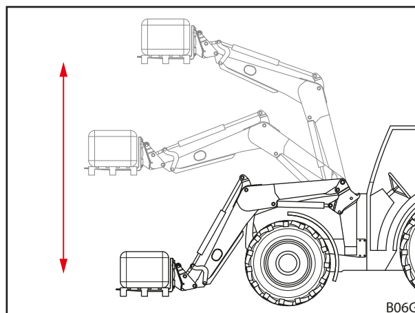
Rys. 41 Mechaniczne prowadzenie równoległe
