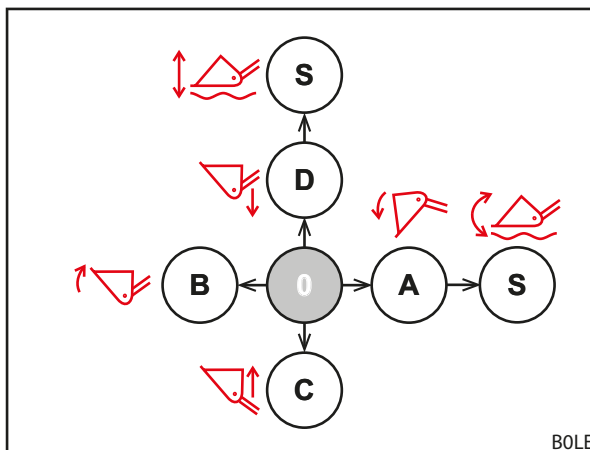
Rys. 67 Przyporządkowanie dźwigni obsługi
