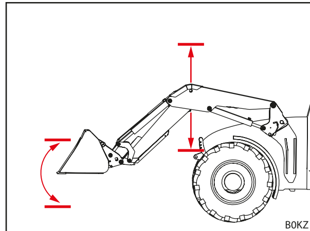
Rys. 35 Zakresy robocze
