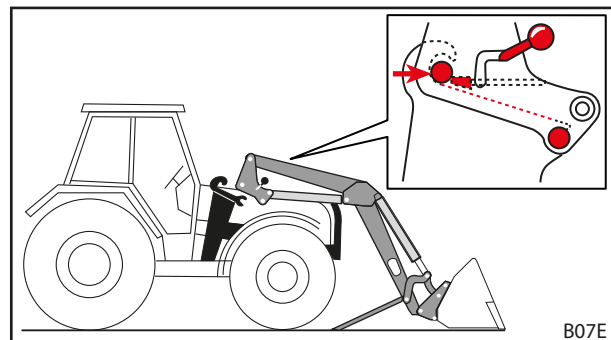
Rys. 53 Wjeżdżanie ciągnikiem w wysięgnik
