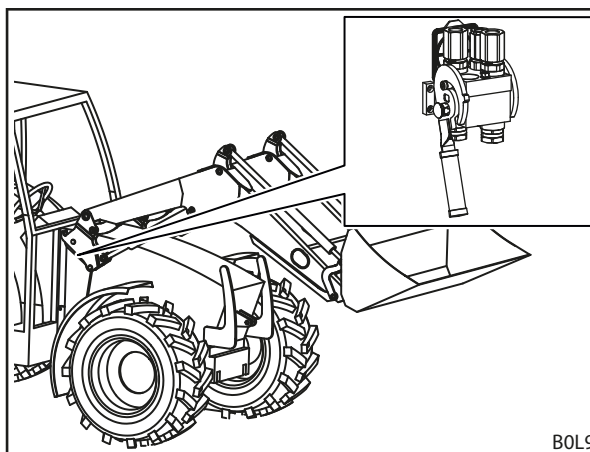
Rys. 18 Hydro-Fix: pozycja na ładowaczu czołowym
