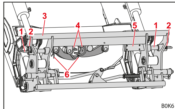
Rys. 13 Kombinowana ramka wymienna Euro-MX (przygotowana pod osprzęt Euro)
