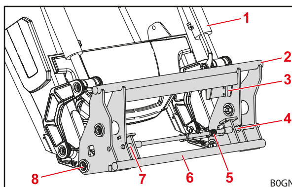
Rys. 10 Ramka wymienna Euro
