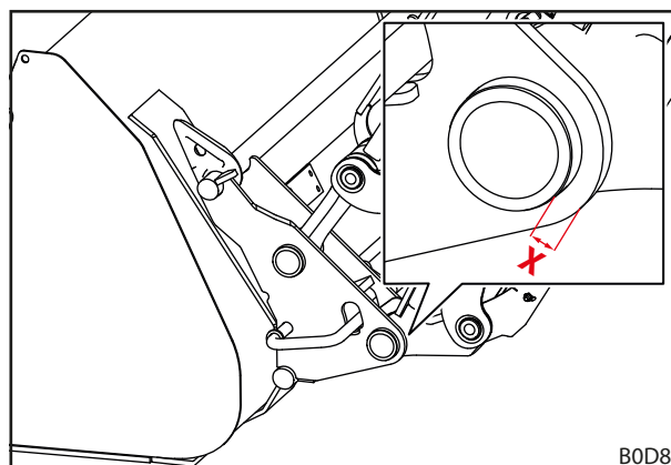
Rys. 119 Wymiar zużycia ramki wymiennej
