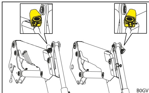
Rys. 45 Reflektor
