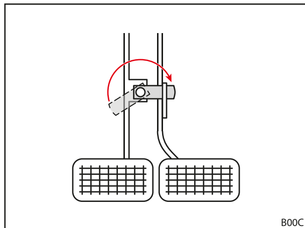
Rys. 48 Łączenie pedałów hamulca
