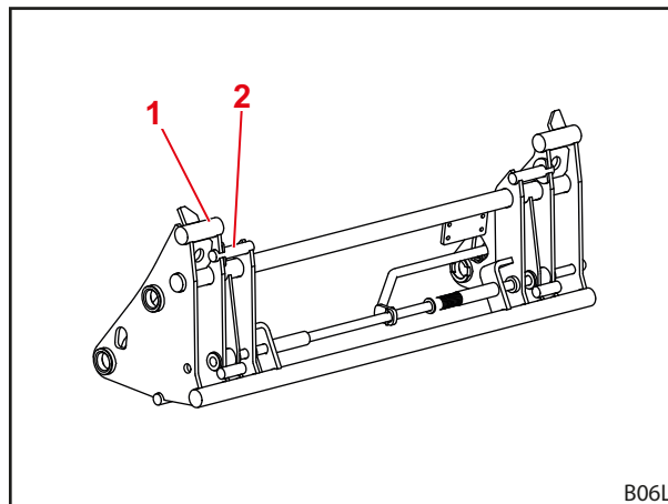
Rys. 13 Kombinowana ramka wymienna Euro-Alö3
