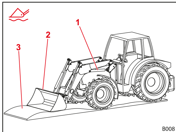
Rys. 31 Ładowacz czołowy w pozycji pływającej
