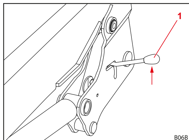
Rys. 117 Kontrola blokady łądownacza czołowego
