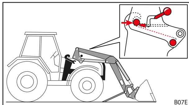
Rys. 48 Wjeżdżanie ciągnikiem w wysięgnik
