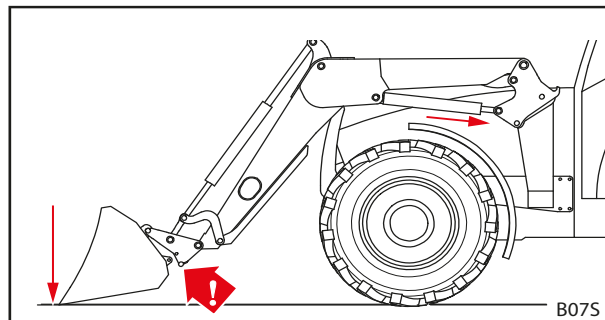
Rys. 84 Dociskanie osprzętu do podłoża
