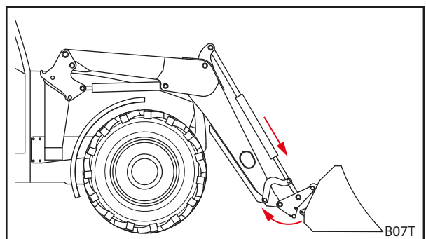
Rys. 106 Odczepianie ramki wymiennej
