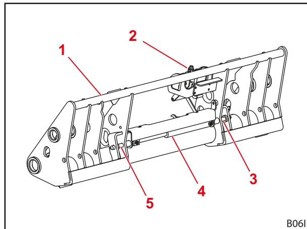
Rys. 16 Wzmocniona ramka wymienna (FZ 100)
