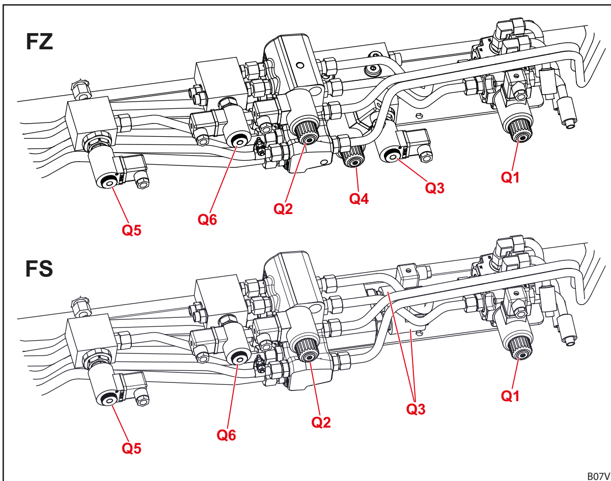
Rys. 133 Rozmieszczenie zaworów hydraulicznych funkcji dodatkowych
