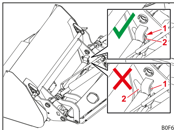
Rys. 90 Kontrola położenia sworzni blokujących
