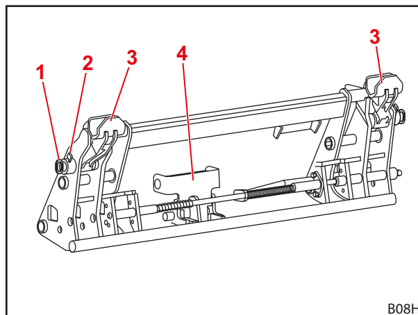
Rys. 14 Kombinowana ramka wymienna Euro-FR
