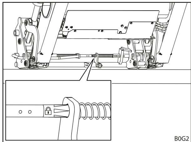
Rys. 82 Kontrola blokady osprzętu za pomocą naklejki (ramka wymienna kombi Euro-FR)
