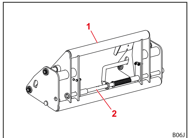
Rys. 11 Ramka wymienna SMS
