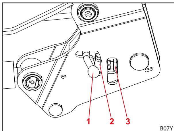
Rys. 57 Otwieranie blokady ładowacza czołowego
