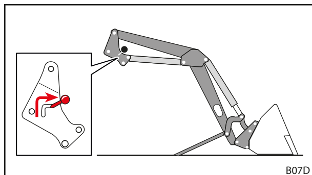
Rys. 47 Otwieranie blokady ładowacza czołowego
