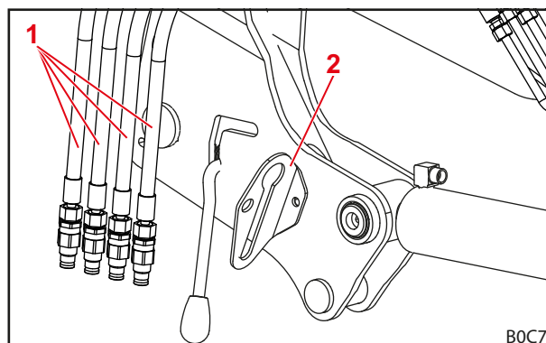
Rys. 126 Zawieszanie przewodów hydraulicznych w uchwycie złącza (widok ze złączkami wtykowymi)
