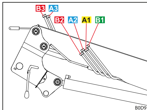
Rys. 18 Przewody hydrauliczne (opcja REAL 3 )
