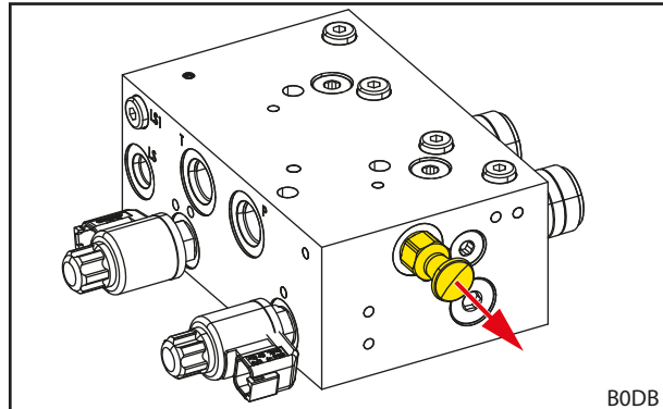
Rys. 72 Wyciąganie zaworu upustowego na zaworze REAL 3
