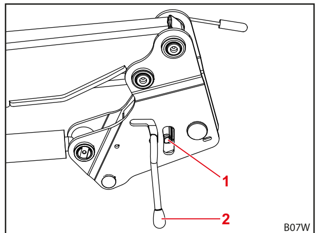
Rys. 118 Kontrola blokady ładowacza czołowego
