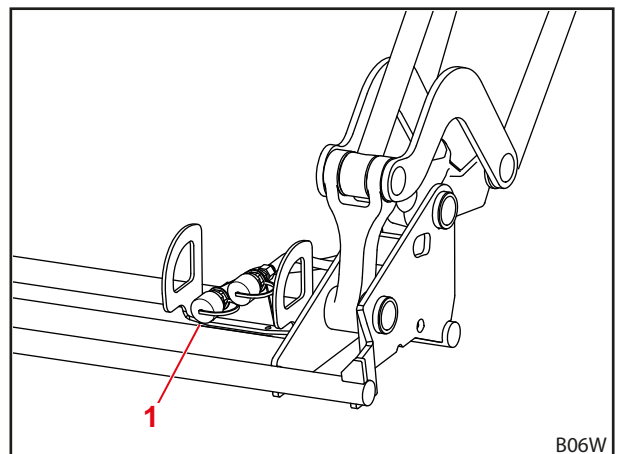
Rys. 37 Dodatkowy 3. obwód sterowniczy
