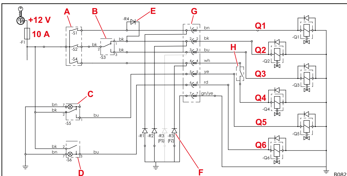
Rys. 131 Schemat elektryczny (w przypadku wyposażenia z 3. i 4. obwodem sterowniczym)
