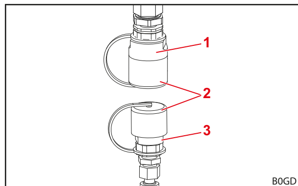
Rys. 76 Złącki gwintowane (rysunek przykładowy)
