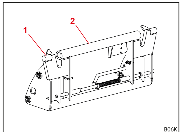
Rys. 12 Kombinowana ramka wymienna Euro-SMS
