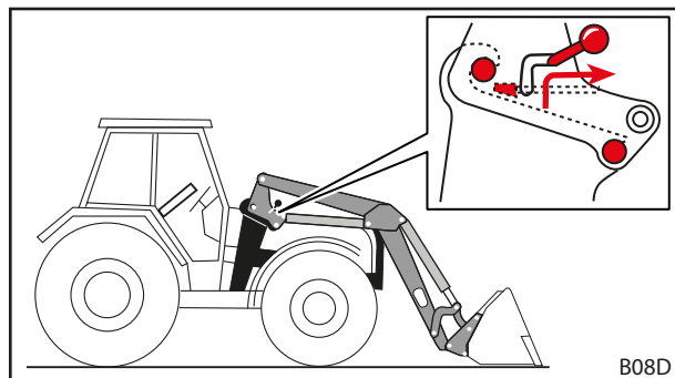
Rys. 122 Zwalnianie blokady ładowacza czołowego
