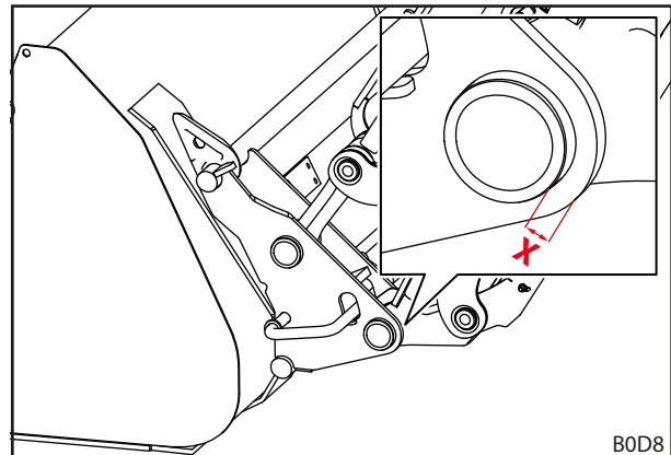
Rys. 91 Wymiar zużycia ramki wymiennej
