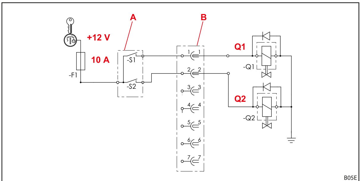
Rys. 98 Schemat elektryczny
