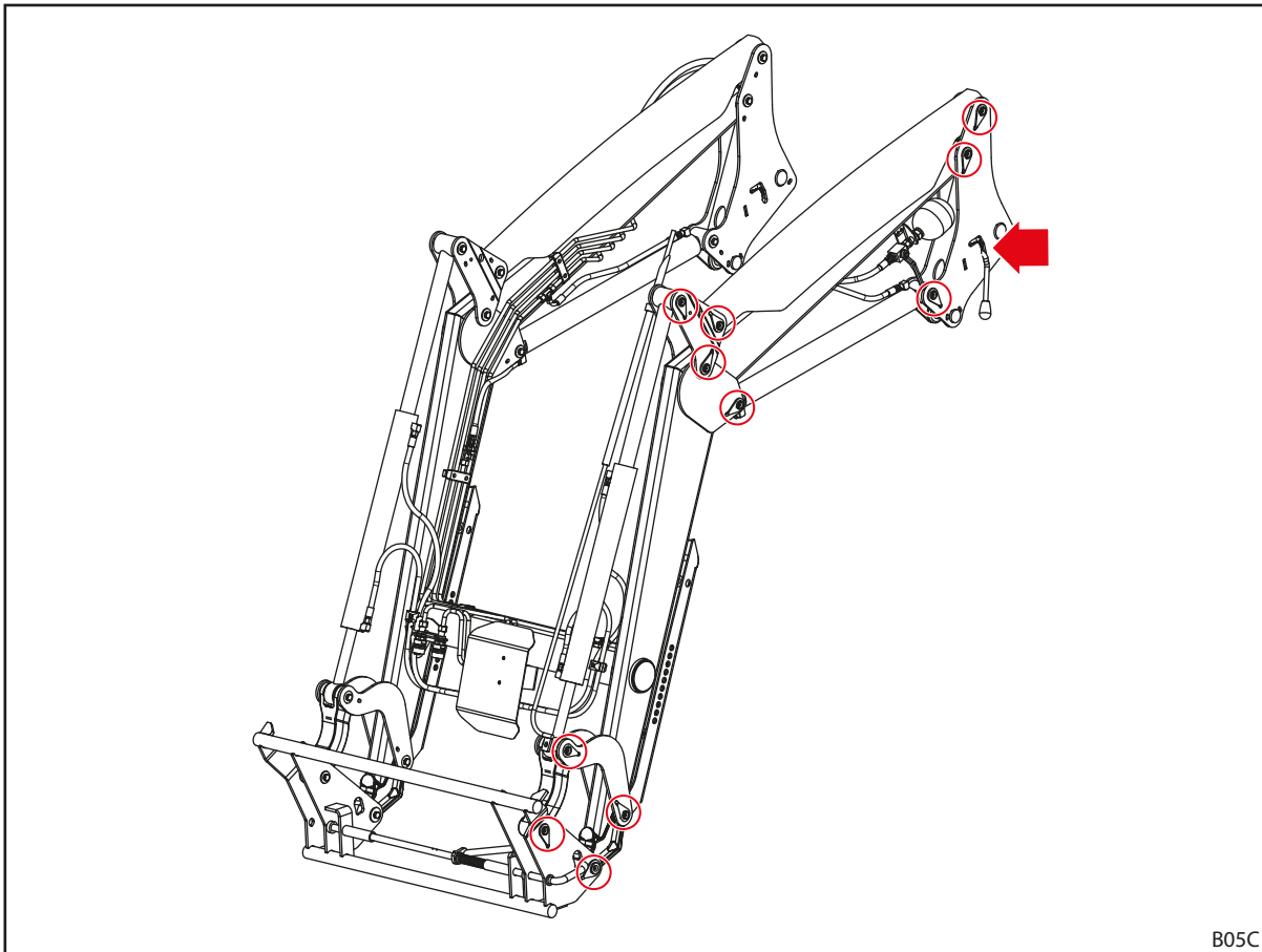
Rys. 88 Punkty smarowania P
