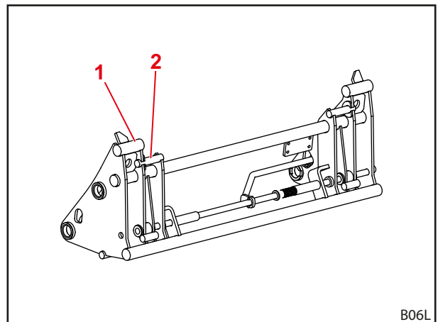
Rys. 13 Kombinowana ramka wymienna Euro-Alö3
