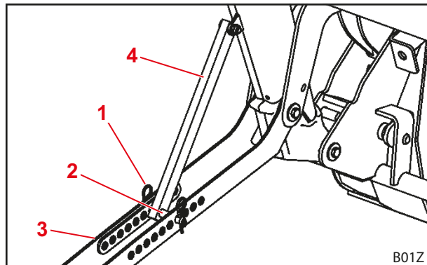
Rys. 55 Podpora
