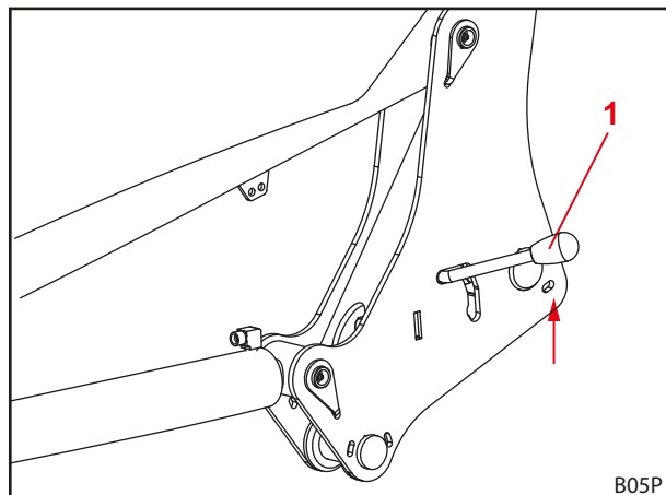
Rys. 42 Otwieranie blokady ładowacza czołowego
