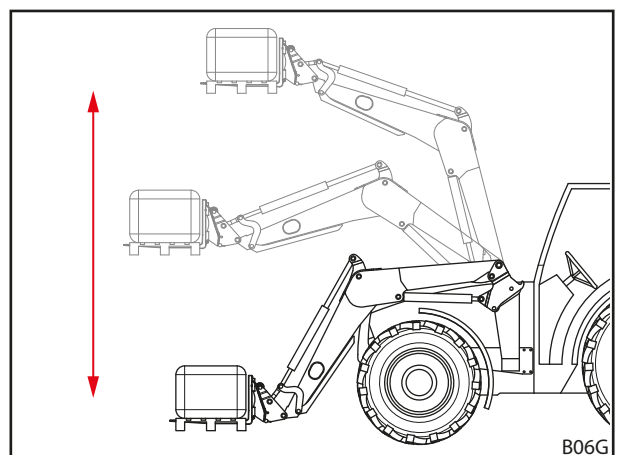
Rys. 27 Prowadzenie równoległe
