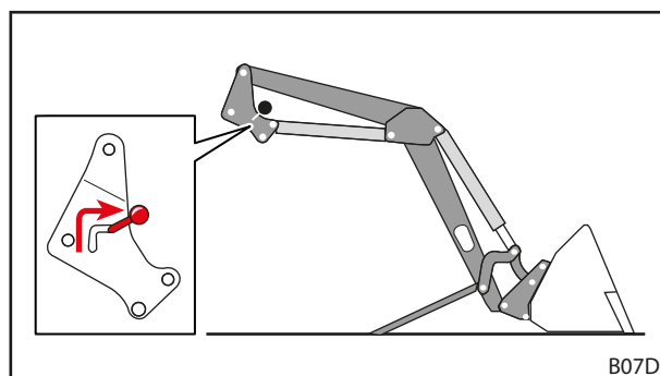
Rys. 36 Otwieranie blokady ładowacza czołowego
