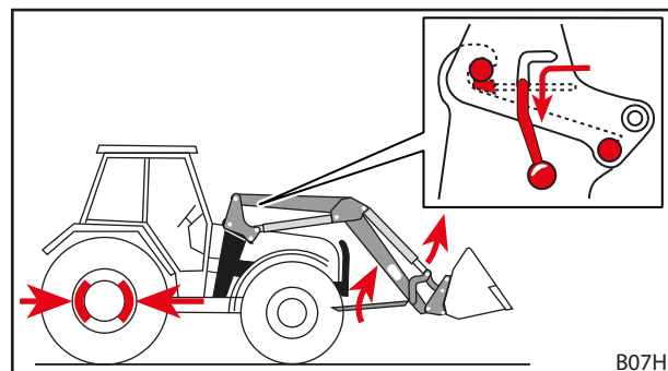
Rys. 40 Składanie podpór i zamykanie blokady ładowacza czołowego
