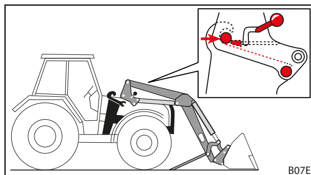
Rys. 37 Wjeżdżanie ciągnikiem w wysięgnik
