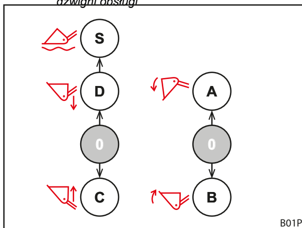
Rys. 47 Przyporządkowanie w przypadku dwóch dźwigni obsługi
