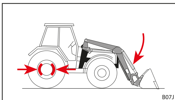
Rys. 92 Zaciągnąć hamulec postojowy i opuścić ładowacz czołowy
