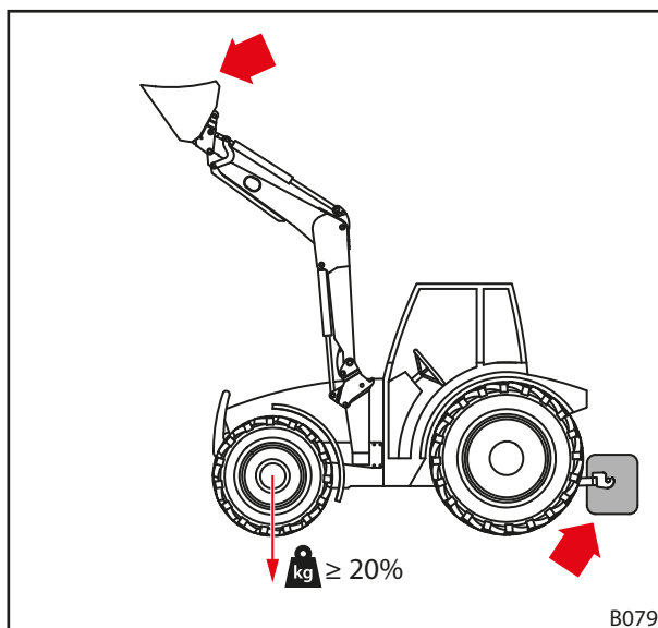
Rys. 34 Obciążenie podczas jazdy po drogach
