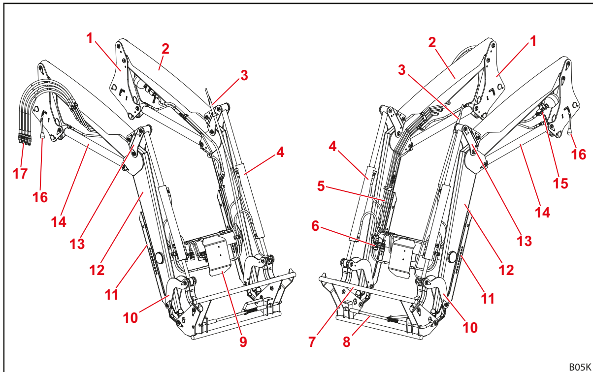
Rys. 8 Ładowacz czołowy P (z mechanicznym prowadzeniem równoległym)
