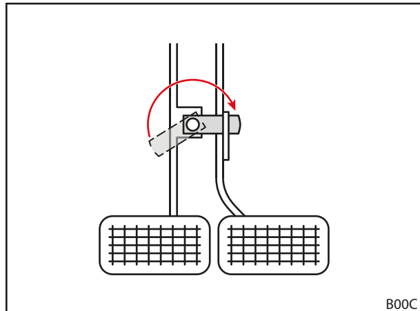
Rys. 32 Łączenie pedałów hamulca
