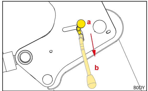
Rys. 44 Czynność naprężania dźwigni blokującej
