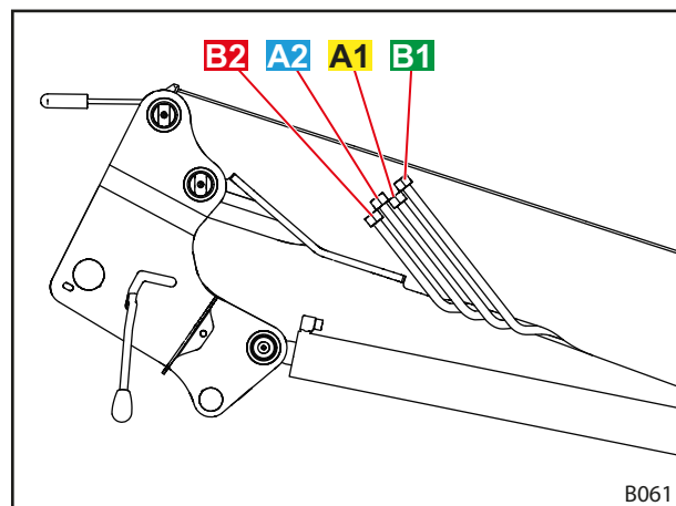
Rys. 15 Przewody hydrauliczne
