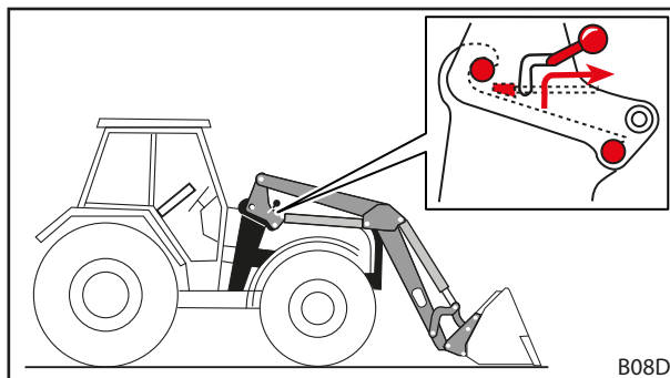
Rys. 93 Zwalnianie blokady ładowacza czołowego
