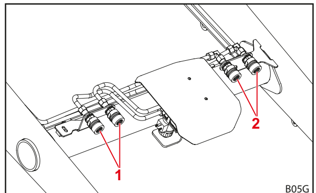
Rys. 29 Dodatkowy 4. obwód sterowniczy
