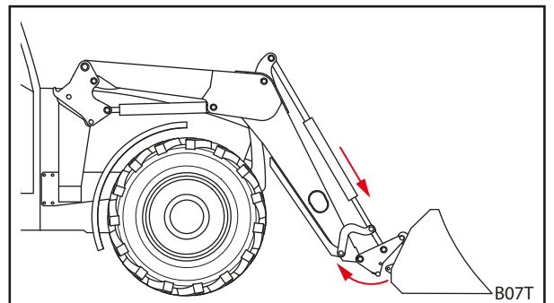
Rys. 78 Odczepianie ramki wymiennej
