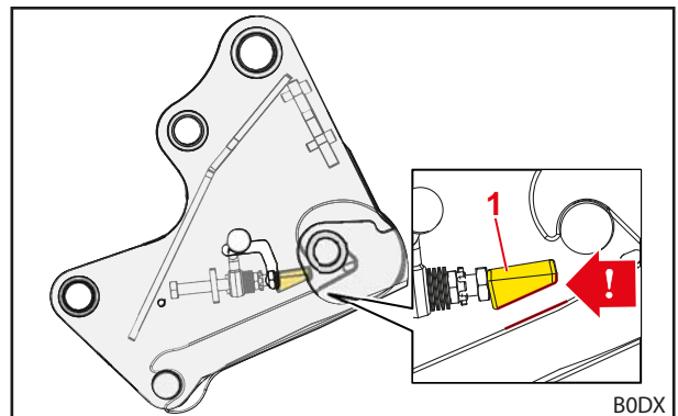
Fig. 57 Posição correta de montagem do calço de aperto
