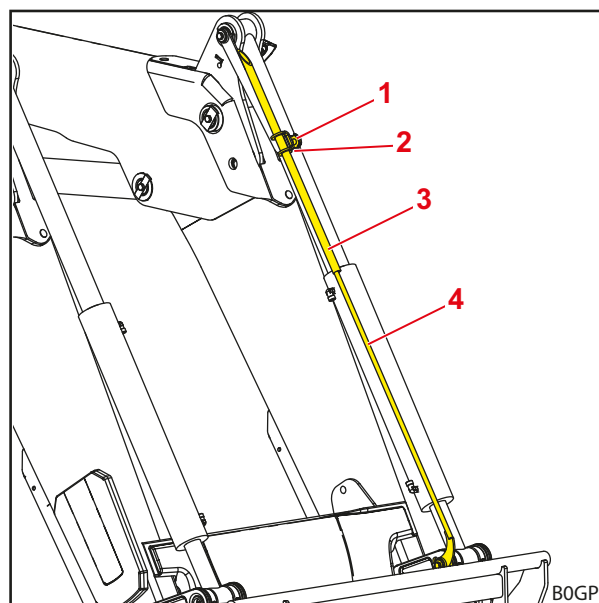
Fig. 40 Indicação visual para colocação da ferramenta
