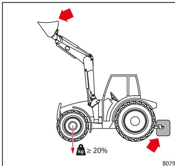
Fig. 50 Carga nos transporte rodoviários em estradas
