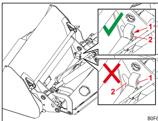
Fig. 84 Verificar a posição dos pernos de bloqueio
