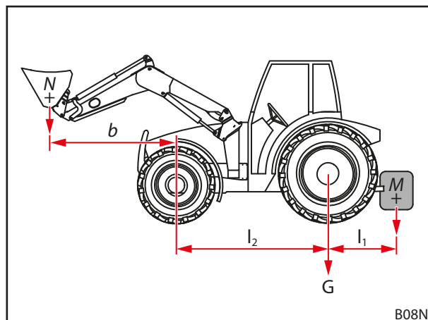
Fig. 51 Cálculo da estabilidade estática
