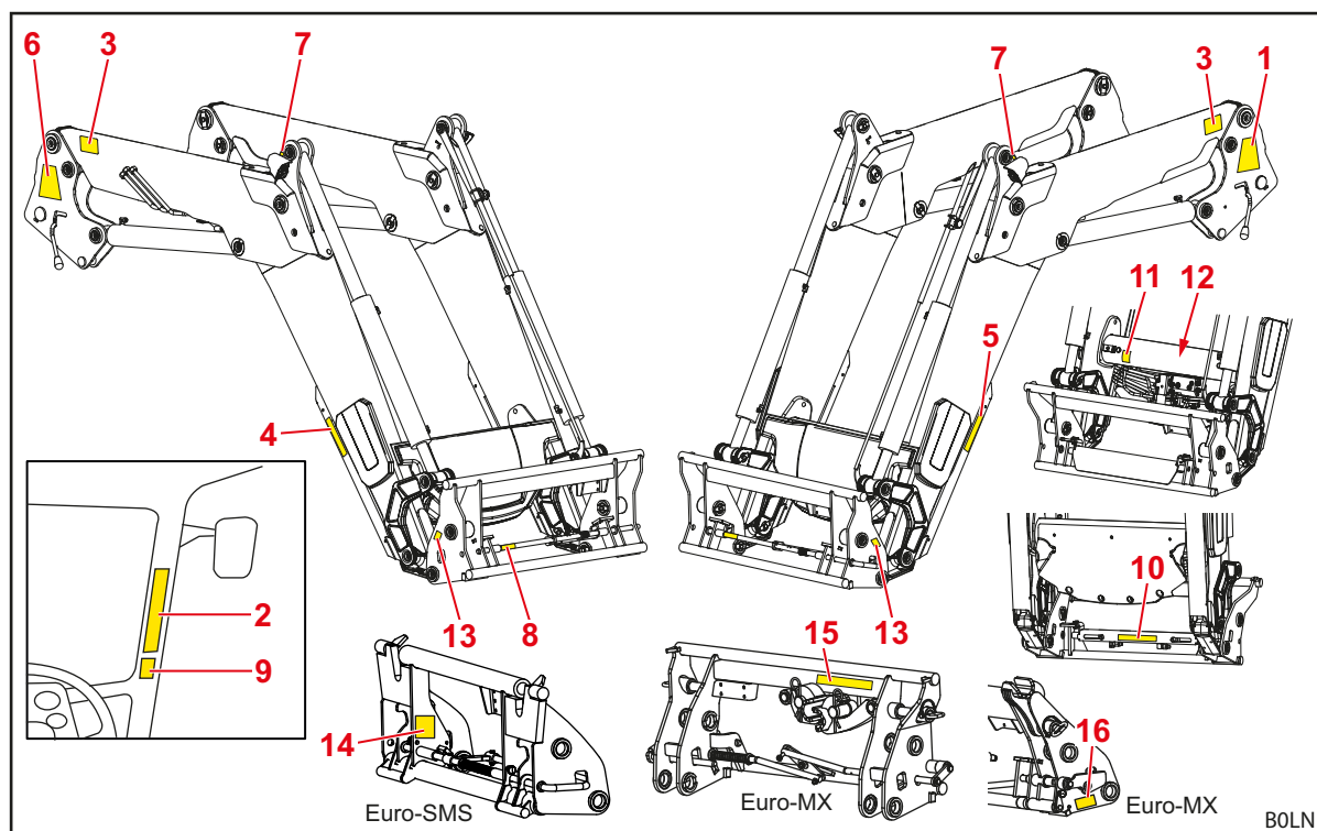
Fig. 4 Carregador frontal FZ IB+ (figura de exemplo)
