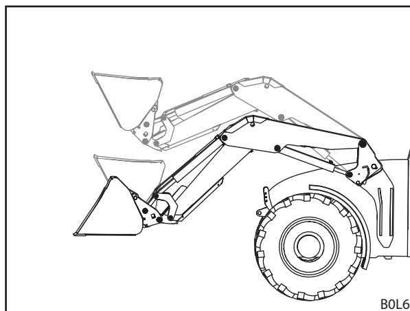
Fig. 38 Ciclo de movimento
