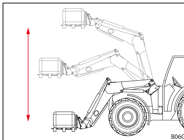
Fig. 41 Versão paralela mecânica
