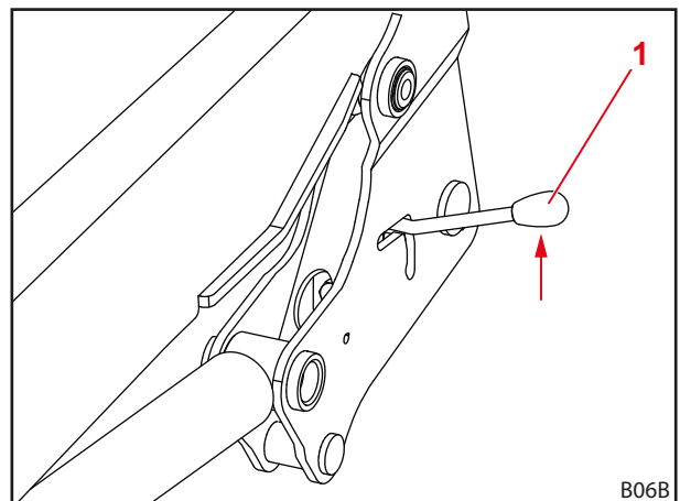
Fig. 58 Abrir o bloqueio do carregador frontal
