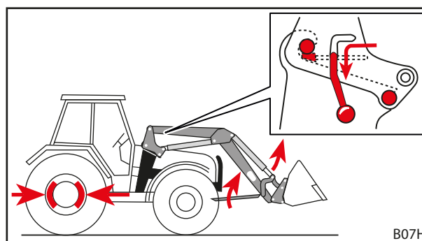
Fig. 56 Dobrar os apoios de descanso para dentro e fechar o bloqueio do carregador frontal
