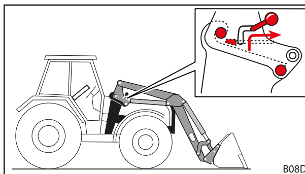
Fig. 121 Soltar o bloqueio do carregador frontal
