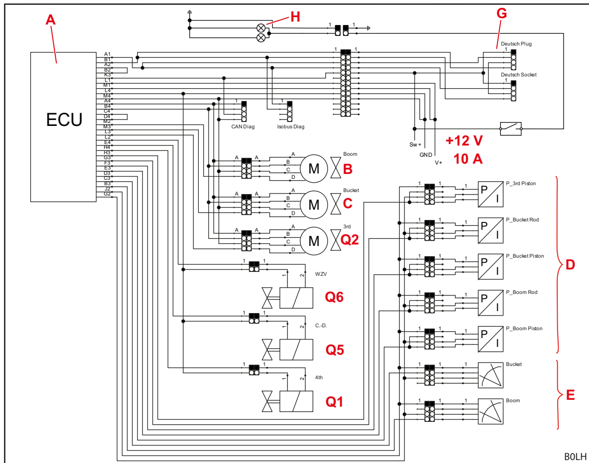
Fig. 127 Esquema elétrico
