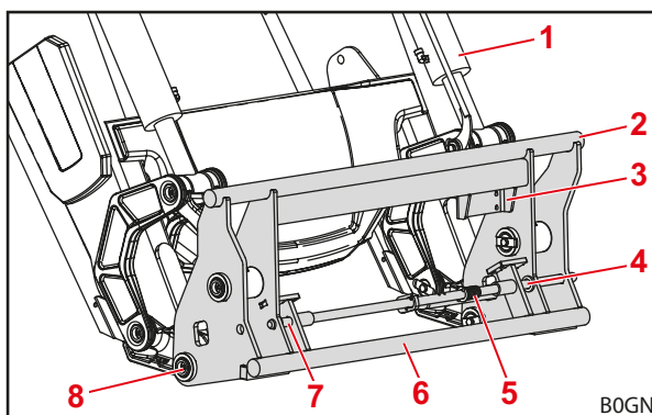
Fig. 10 Armação de troca Euro
