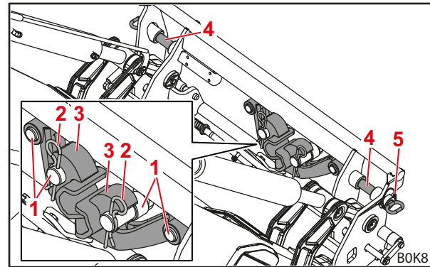
Fig. 91 Adaptador em posição de estacionamento (armação de troca preparada para a ferramenta Euro)
