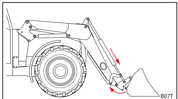
Fig. 103 Desenganchar a armação de troca
