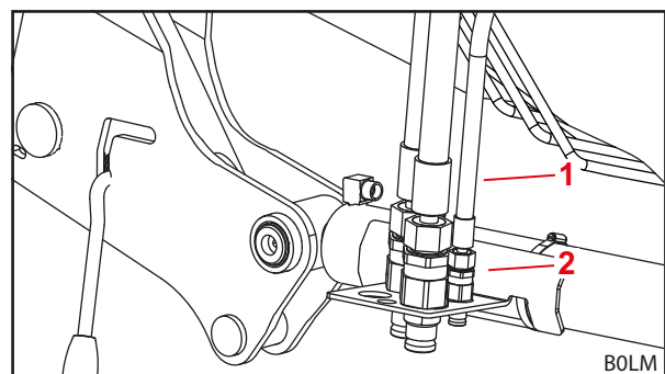
Fig. 125 Pendurar os tubos hidráulicos no suporte de acoplamento (apresentação com engates de encaixe)
