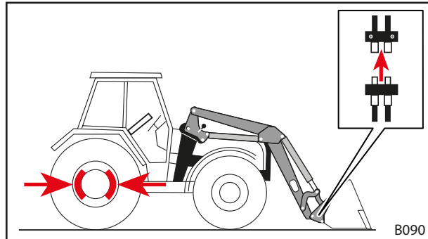
Fig. 102 Soltar os condutores hidráulicos
