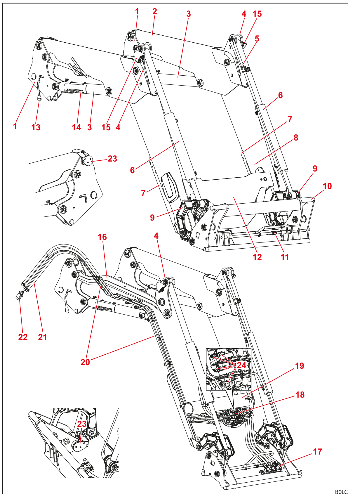
Fig. 8 Carregador frontal FZ IB+
