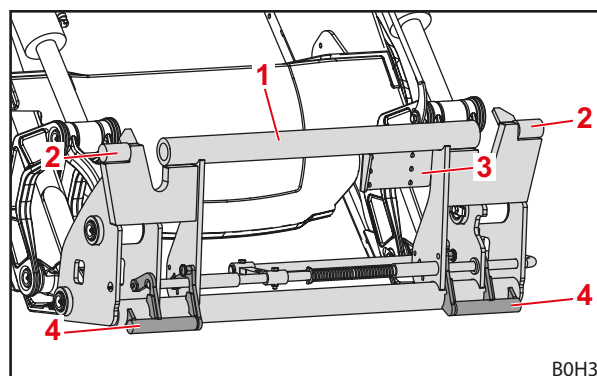
Fig. 11 Armação de troca combinada Euro-SMS (preparada para ferramenta Euro)
