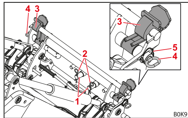
Fig. 92 Adaptador em posição de trabalho (armação de troca preparada para a ferramenta MX)
