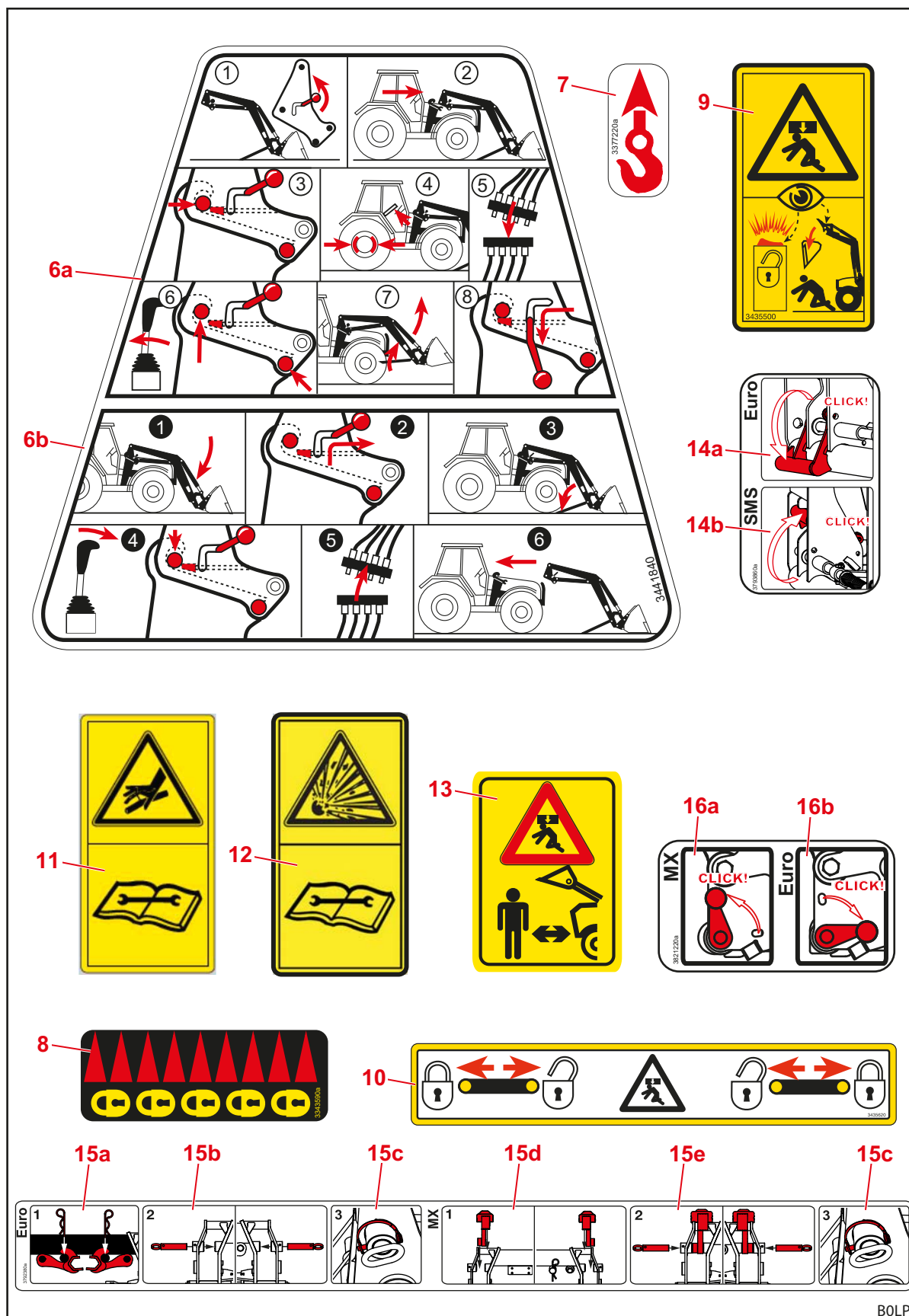
Fig. 6 Autocolantes de segurança Posição 6-16
