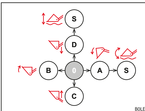
Fig. 67 Atribuição da alavanca de comando
