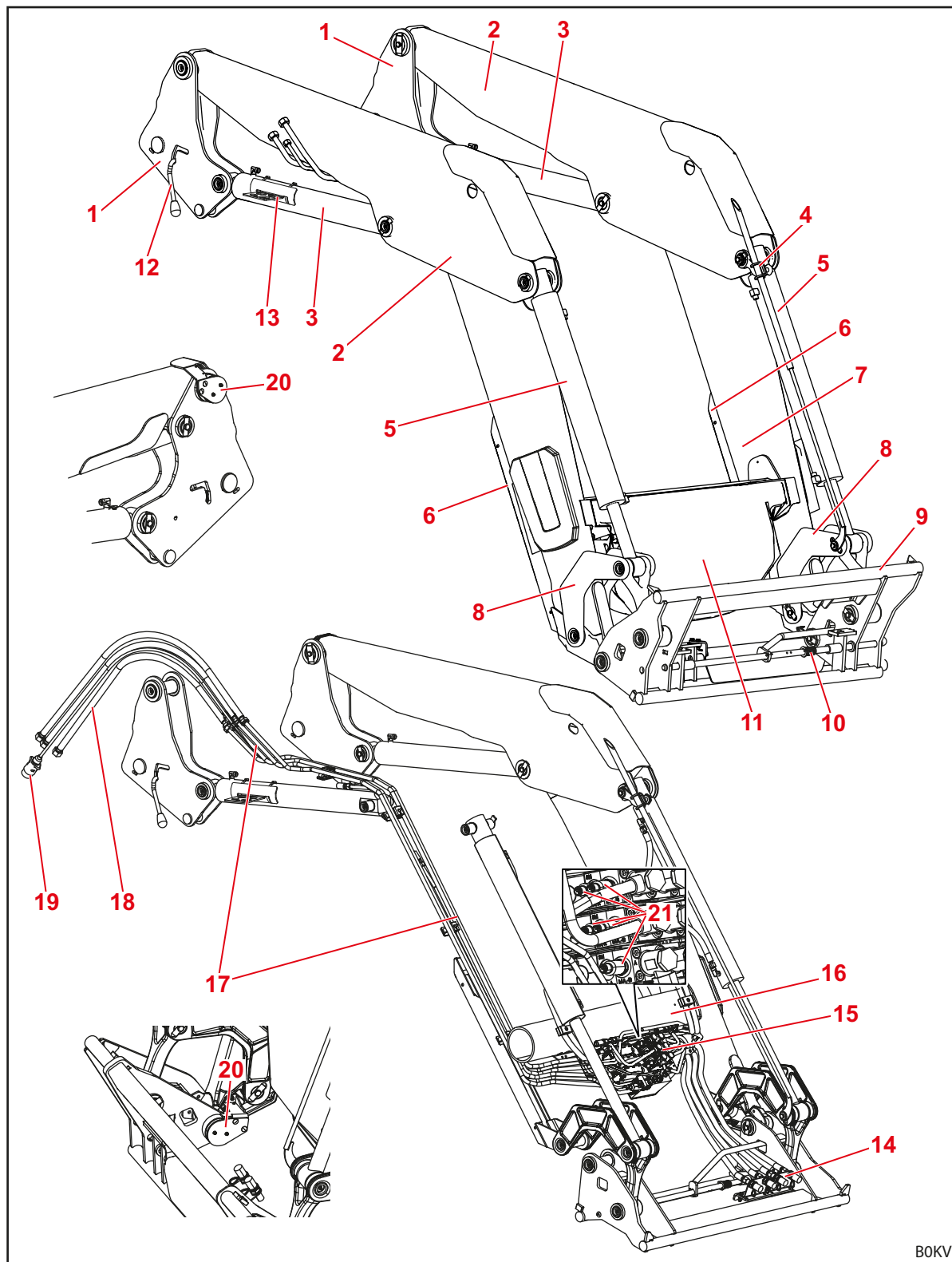
Fig. 7 Carregador frontal FS IB+
