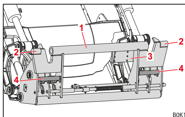
Fig. 12 Armação de troca combinada Euro-SMS (preparada para ferramenta SMS)
