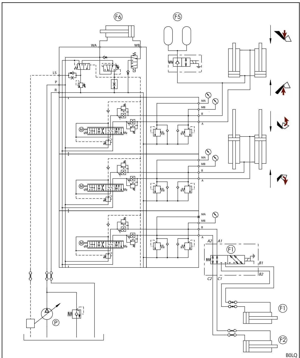
Fig. 126 Esquema hidráulico FS IB+ e FZ IB+
