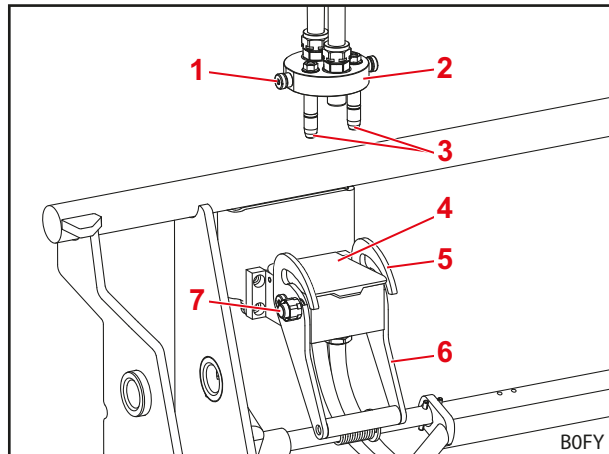
Fig. 74 Implement-Fix desacoplado
