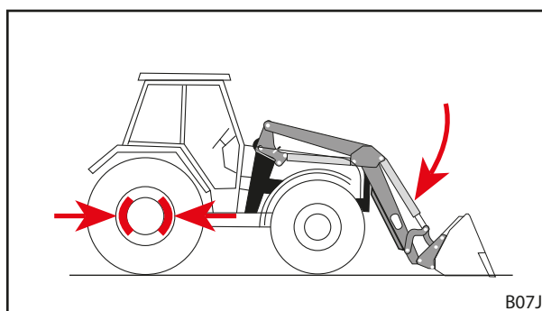
Fig. 120 Puxar o travão de estacionamento e baixar o carregador frontal
