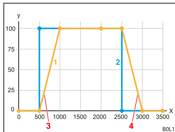
Fig. 31 Comportamento de resposta ajustável
