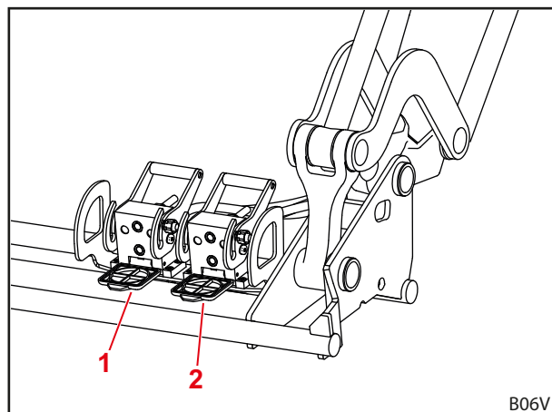
Fig. 43 4.º circuito de comando adicional
