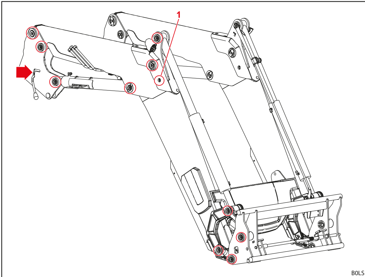
Fig. 114 Pontos de lubrificação FZ IB+
