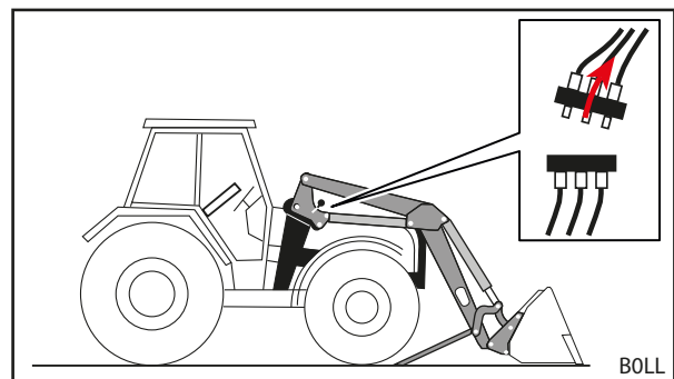
Fig. 123 Desacoplar o sistema hidráulico
