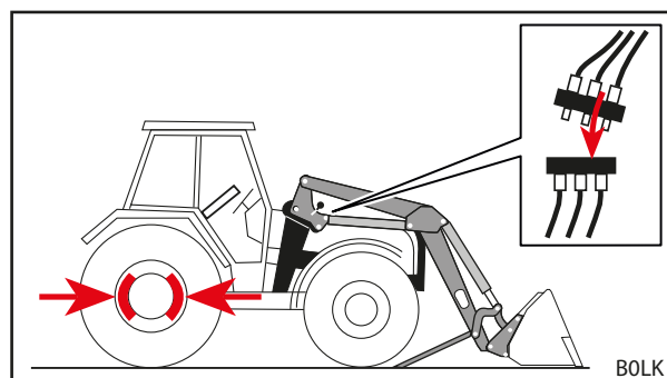
Fig. 54 Desligar o trator e ligar os condutores hidráulicos
