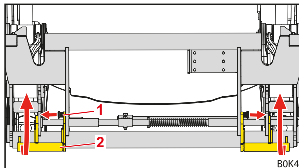
Fig. 88 Girar os sistemas para cima
