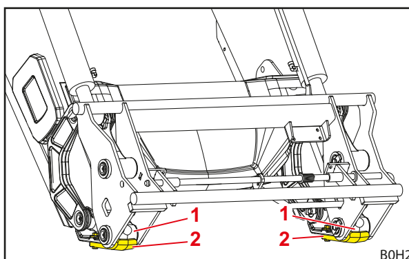
Fig. 15 Patins de desgaste
