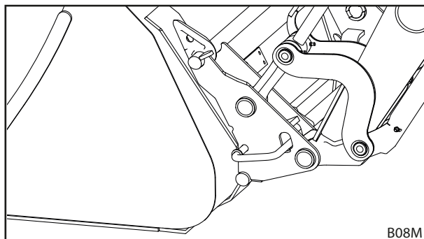
Fig. 93 Abrir o bloqueio da ferramenta
