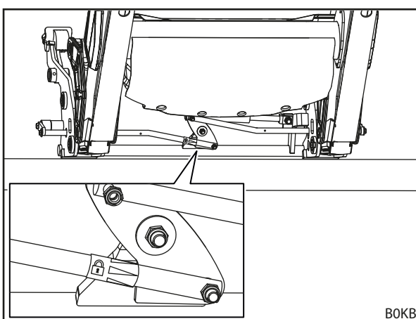
Fig. 83 Verificar o bloqueio da ferramenta através do autocolante
