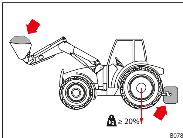
Fig. 49 Carga nos trabalhos com o carregador frontal
