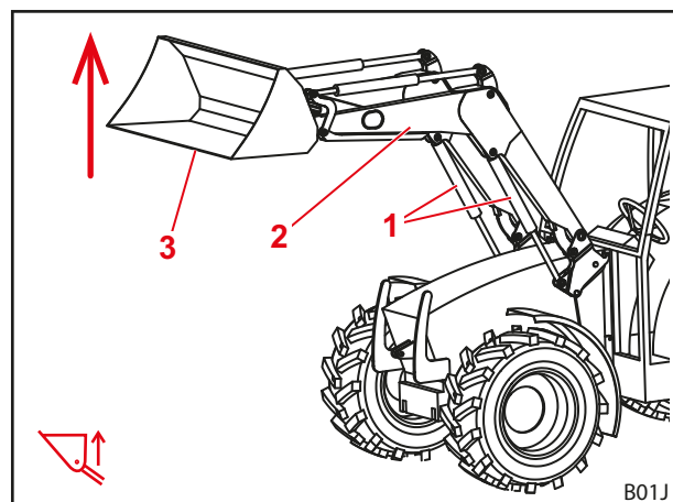
Fig. 23 Função de elevação
