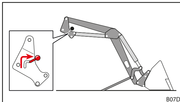
Fig. 52 Abrir o bloqueio do carregador frontal
