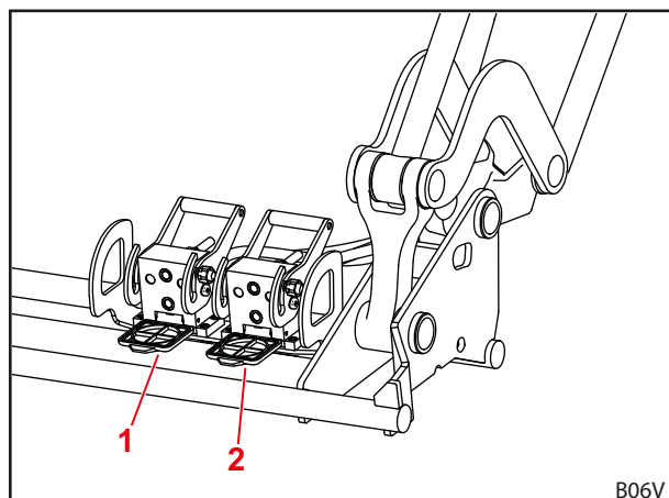
Fig. 36 4.º circuito de comando adicional
