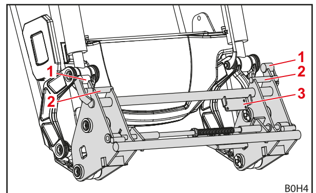
Fig. 12 Armação de troca combinada Euro-Alö 3
