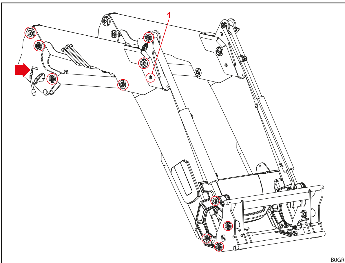
Fig. 119 Pontos de lubrificação FZ
