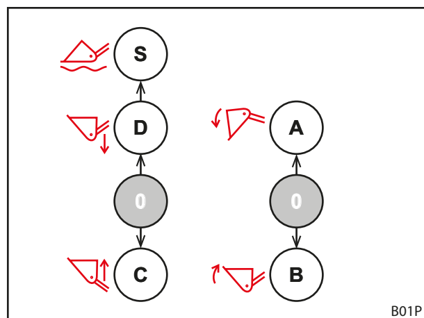
Fig. 66 Atribuição em caso de 2 alavancas de comando
