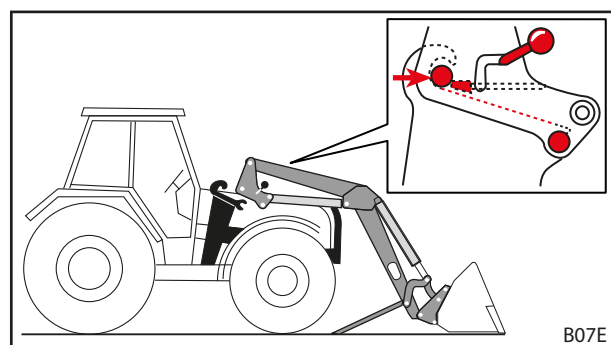
Fig. 51 Recolher o trator até ao braço oscilante
