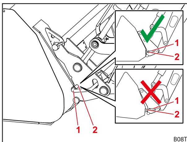
Fig. 86 Verificar a posição dos pernos de bloqueio
