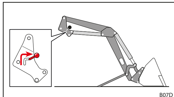
Fig. 50 Abrir o bloqueio do carregador frontal
