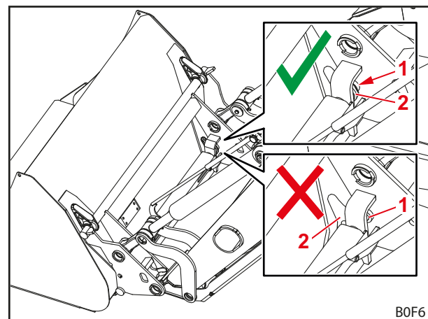
Fig. 93 Verificar a posição das pernos de bloqueio
