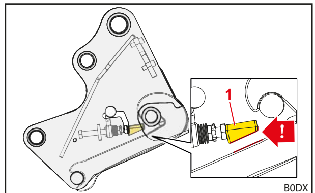
Fig. 55 Posição correta de montagem do calço de aperto
