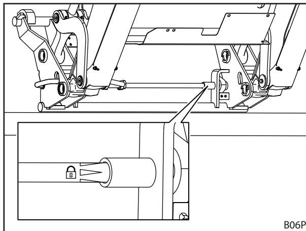
Fig. 85 Verificar o bloqueio da ferramenta através do autocolante
