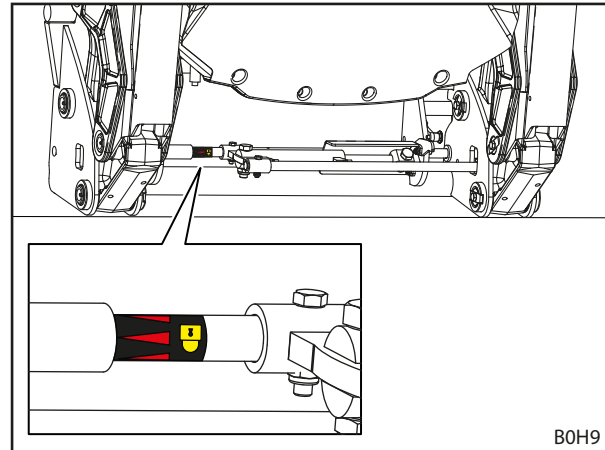
Fig. 92 Verificar o bloqueio da ferramenta através do autocolante
