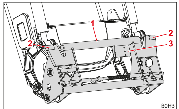
Fig. 11 Armação de troca combinada Euro-SMS
