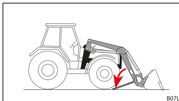
Fig. 127 Dobrar os apoios de descanso para fora
