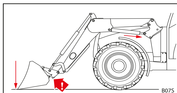
Fig. 89 Pressionar a ferramenta no chão
