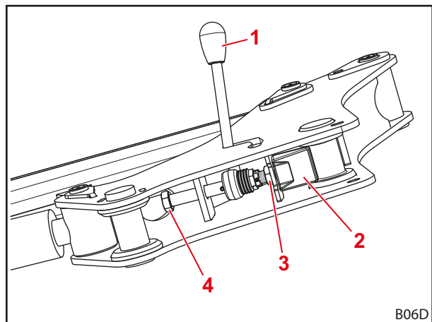
Fig. 59 Vista do bloqueio do carregador frontal de baixo
