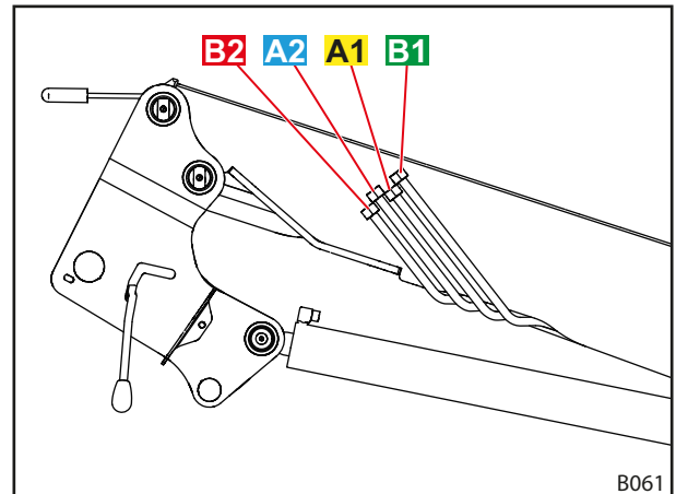
Fig. 15 Condutores hidráulicos
