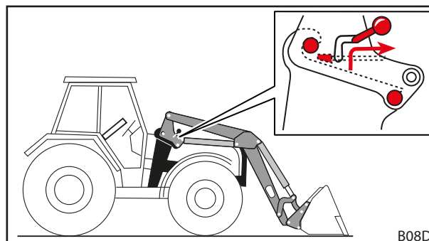
Fig. 126 Soltar o bloqueio do carregador frontal
