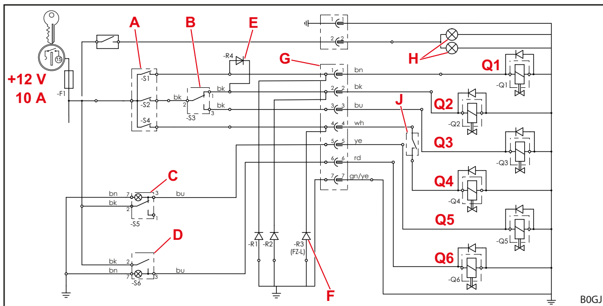
Fig. 137 Diagrama do circuito elétrico (no equipamento com 3.º e 4.º circuito de comando)
