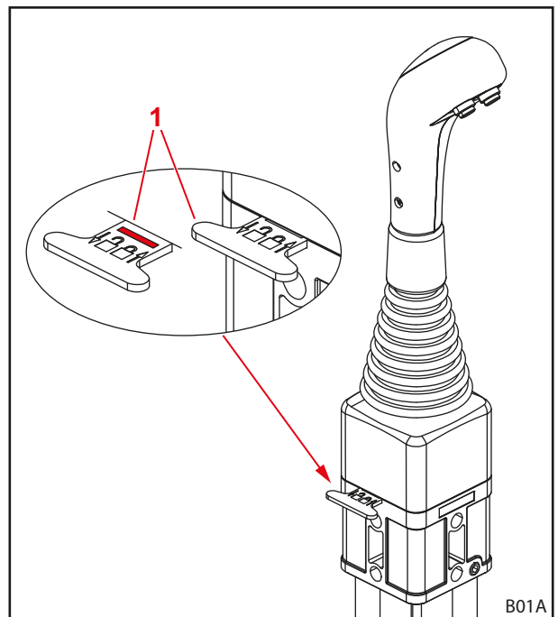
Fig. 68 Bloqueio da alavanca de comando
