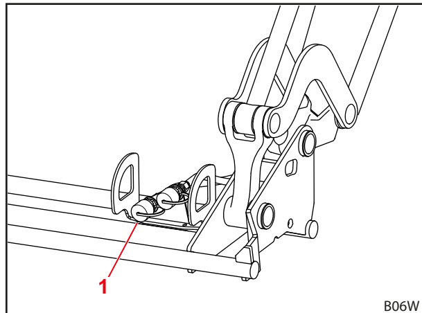
Fig. 35 3.º circuito de comando adicional
