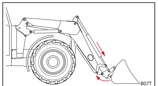
Fig. 109 Desenganchar a armação de troca
