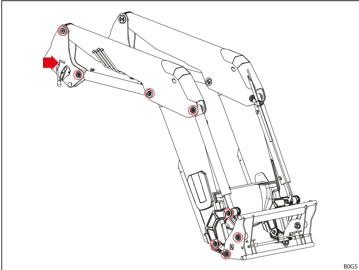
Fig. 118 Pontos de lubrificação FS
