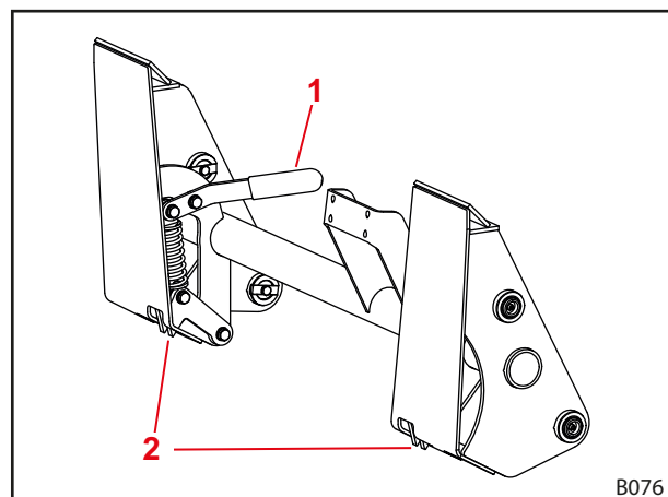
Fig. 88 Bloqueio da ferramenta na armação de troca Skid-Steer
