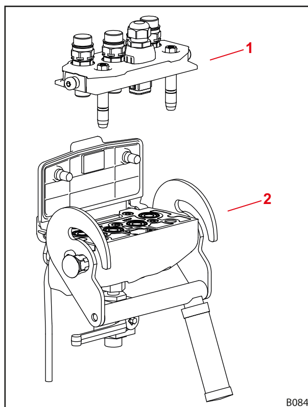
Fig. 20 Estrutura Hydro-Fix
