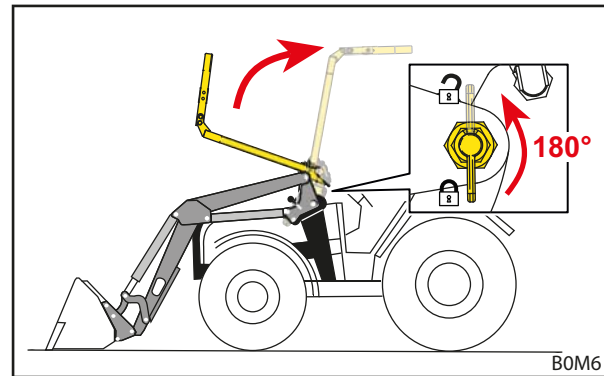
Fig. 36 Dobrar o OPG para cima
