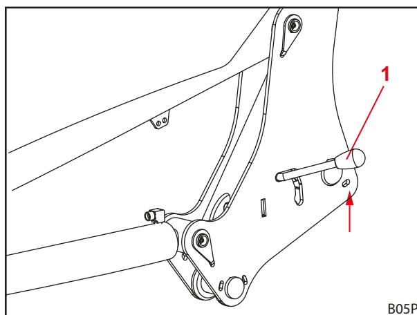
Fig. 53 Abrir o bloqueio do carregador frontal
