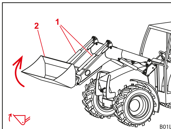
Fig. 28 Função de recolher
