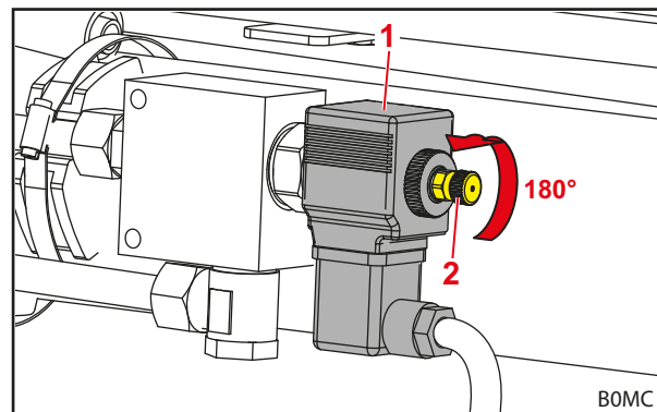
Fig. 33 Abrir a válvula
