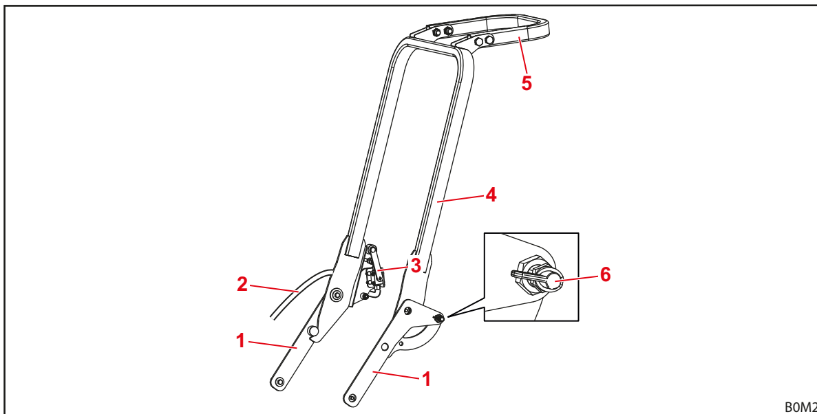
Fig. 11 Operator Protective Guard, OPG (ilustração exemplar)
