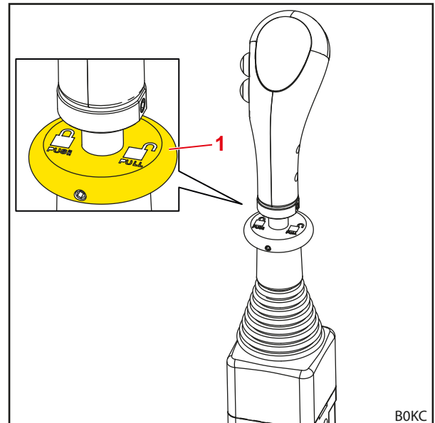
Fig. 61 Bloqueio da alavanca de comando (bloqueio vertical)
