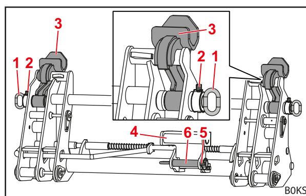
Fig. 87 Adaptador em posição de trabalho (armação de troca preparada para a ferramenta FR)
