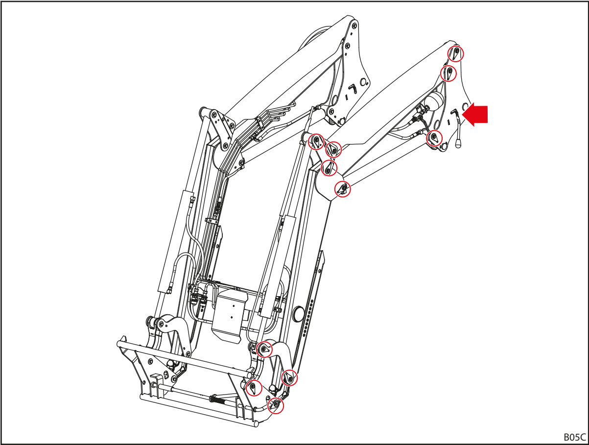
Fig. 110 Pontos de lubrificação P
