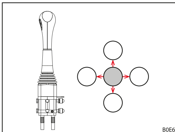
Fig. 62 Mover a alavanca de comando para todas as posições finais
