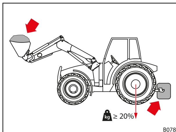
Fig. 43 Carga nos trabalhos com o carregador frontal
