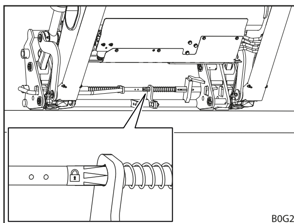
Fig. 77 Verificar o bloqueio da ferramenta através do autocolante (armação de troca combinada Euro-FR)
