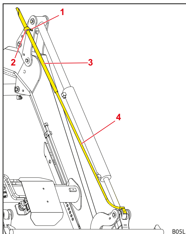
Fig. 31 Indicação visual para o ajuste da ferramenta
