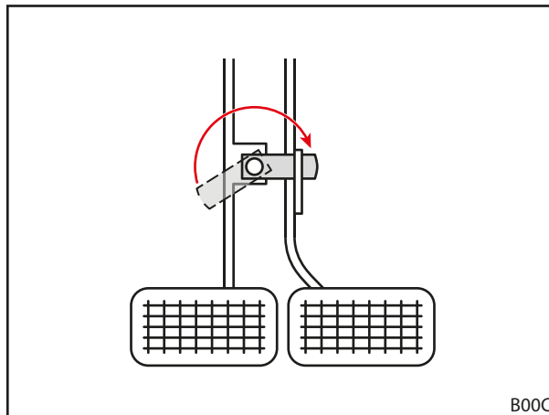
Fig. 42 Acoplar os pedais dos travões
