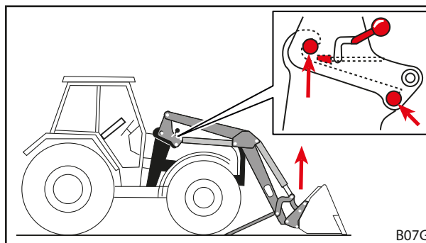
Fig. 50 Utilizar a função Elevação até que as cavilhas do carregador frontal estejam fixadas nos anzóis
