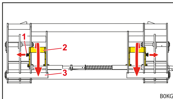
Fig. 82 Girar os sistemas para baixo
