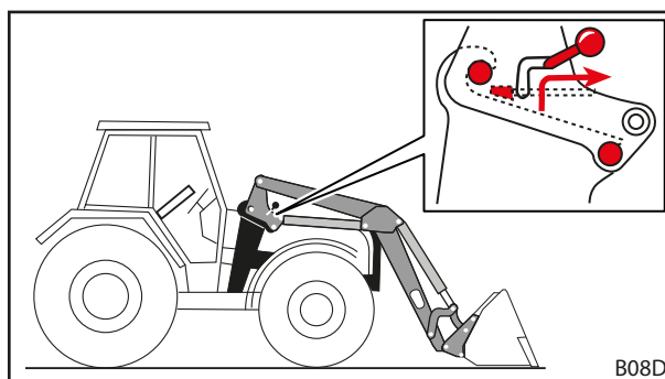
Fig. 115 Soltar o bloqueio do carregador frontal
