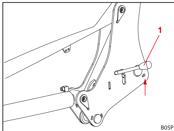
Fig. 112 Verificar o bloqueio do carregador frontal
