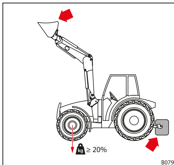
Fig. 44 Carga nos transporte rodoviários em estradas
