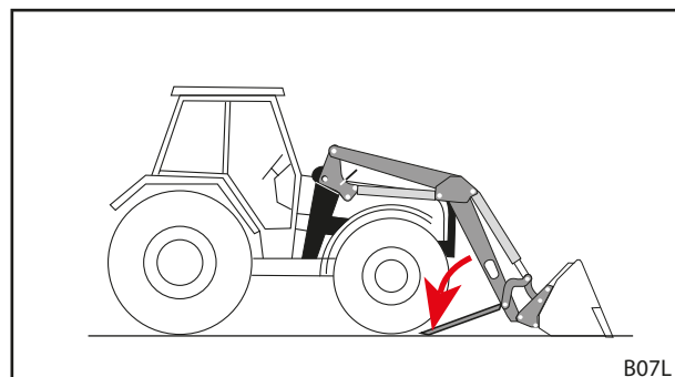
Fig. 116 Dobrar os apoios de descanso para fora
