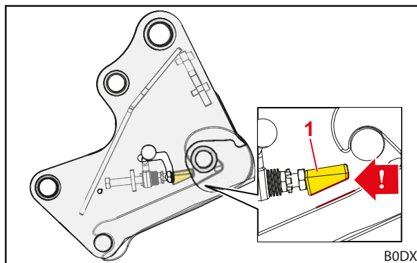
Fig. 52 Posição correta de montagem do calço de aperto
