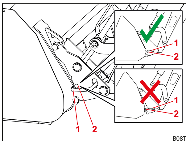
Fig. 78 Verificar a posição dos pernos de bloqueio
