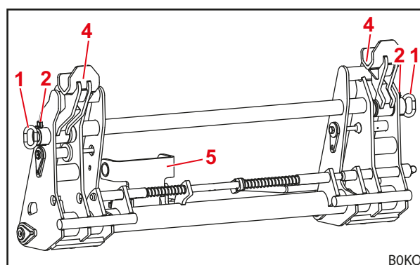
Fig. 19 Armação de troca combinada Euro-FR (preparada para ferramenta FR)
