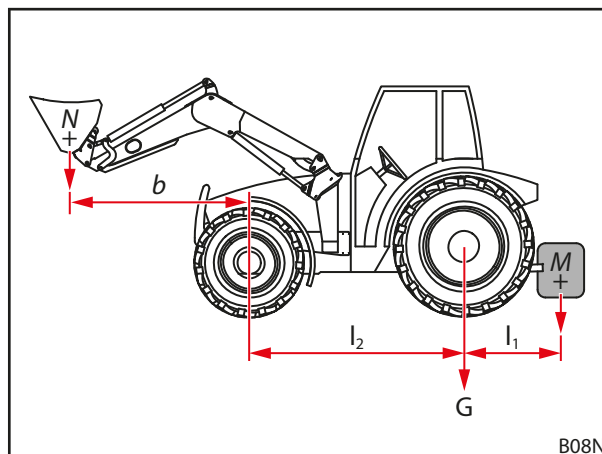
Fig. 45 Cálculo da estabilidade estática
