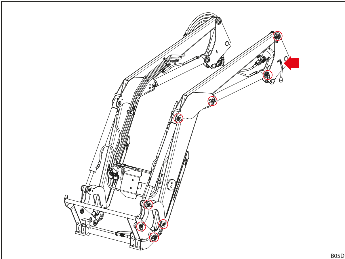
Fig. 109 Pontos de lubrificação H
