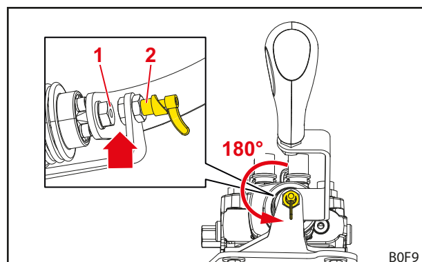
Fig. 65 Alavanca de comando desbloqueado
