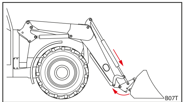
Fig. 100 Desenganchar a armação de troca
