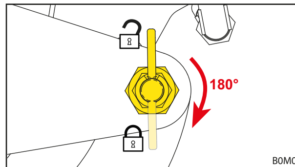
Fig. 37 Colocar o trinco de encaixe na posição bloqueada
