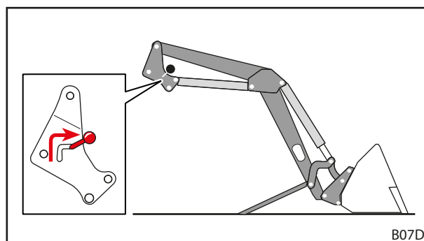
Fig. 46 Abrir o bloqueio do carregador frontal
