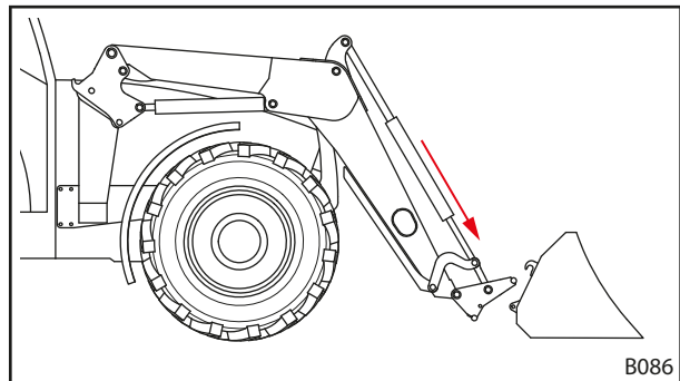
Fig. 89 Poziționarea brațului oscilant
