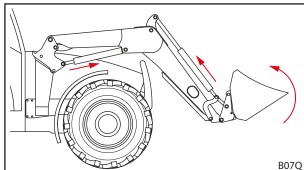
Fig. 92 Desfacerea dispozitivului de blocare a uneltei
