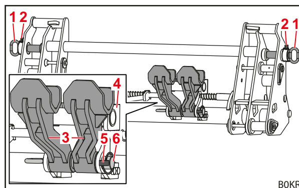
Fig. 86 Adaptor în poziția de parcare (cadru de înlocuire pregătit pentru unealta Euro)
