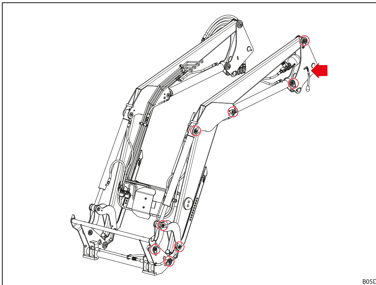
Fig. 109 Puncte de lubrifiere H
