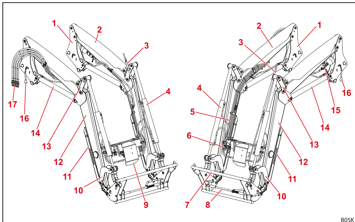
Fig. 10 Încărcător frontal P (cu ghidare mecanică paralelă)
