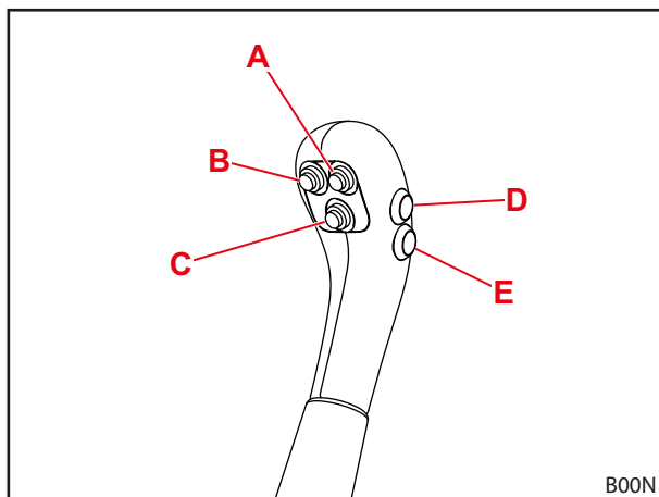
Fig. 59 Base Control cu 5 butoane
