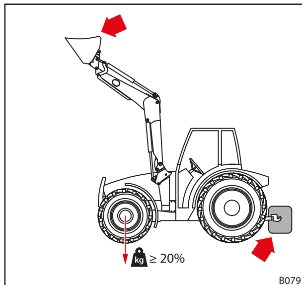
Fig. 44 Încărcare la deplasările pe drumurile publice
