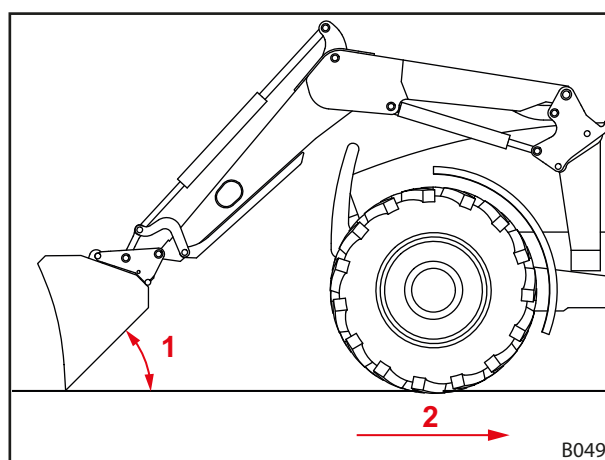
Fig. 102 Nivelarea înapoi
