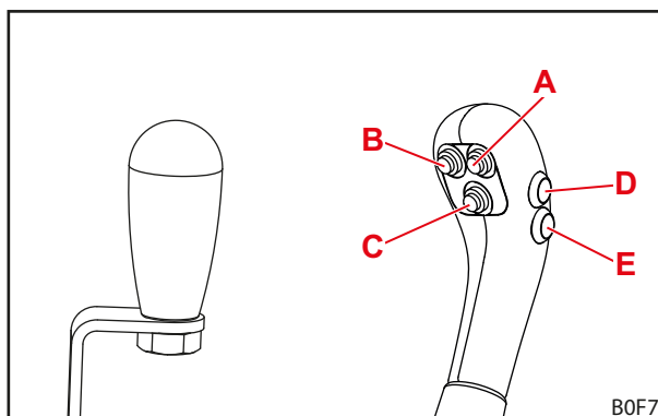
Fig. 63 Manetă de comandă fără buton (stânga) și manetă de comandă cu 5 butoane (dreapta)
