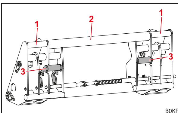
Fig. 16 Cadru de înlocuire combinat Euro-SMS (pregătit pentru scula SMS)
