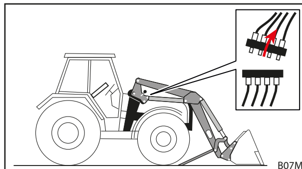
Fig. 117 Decuplarea sistemului hidraulic
