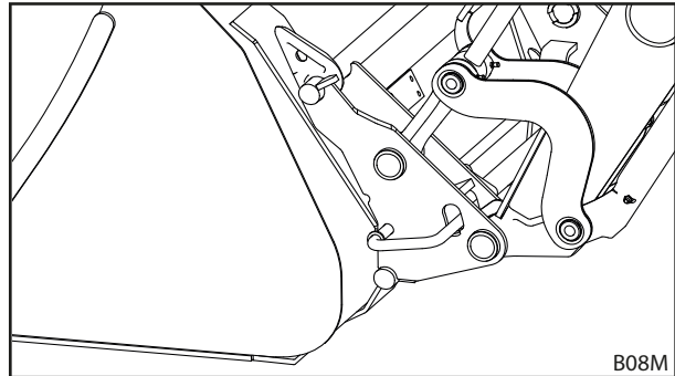
Fig. 88 Deschiderea dispozitivului de blocare a uneltei
