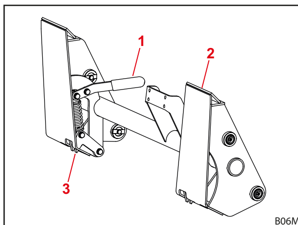
Fig. 25 Operarea dispozitivului de blocare mecanică a uneltei la cadrul de înlocuire Skid-Steer
