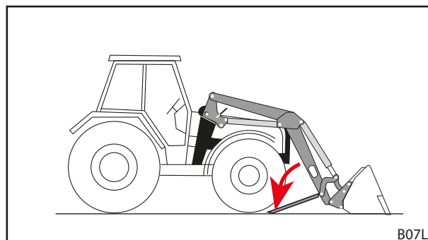
Fig. 116 Rabatați deschis reazemele de parcare
