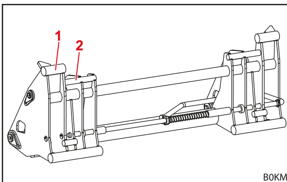
Fig. 17 Cadru de înlocuire combinat Euro-Alö3
