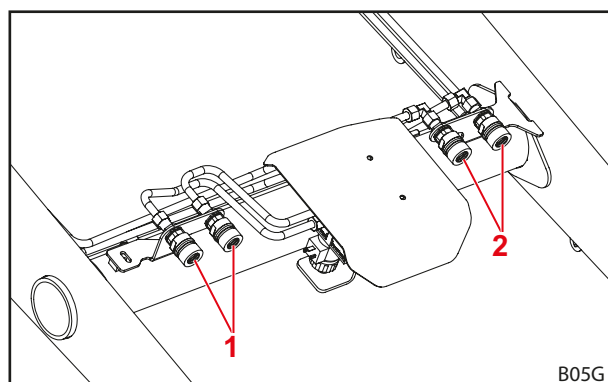
Fig. 39 Al 4-lea circuit de comandă suplimentar
