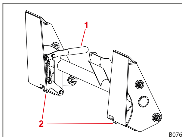
Fig. 80 Dispozitiv de blocare a uneltei la cadrul de înlocuire Skid-Steer
