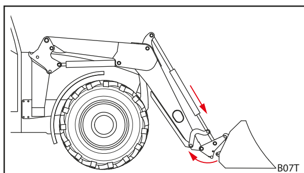
Fig. 100 Scoaterea din cârlig a cadrului de înlocuire
