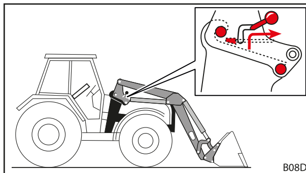
Fig. 115 Eliberarea dispozitivului de blocare al încărcătorului frontal
