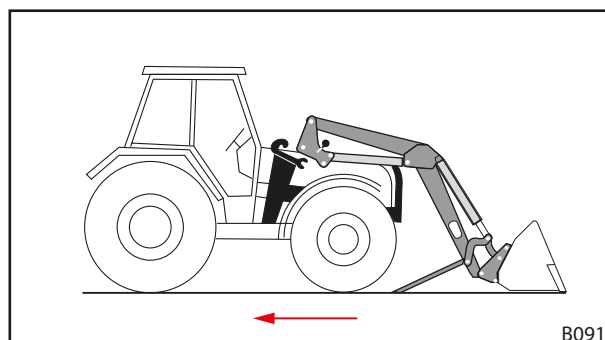
Fig. 118 Scoaterea tractorului prin deplasare înapoi
