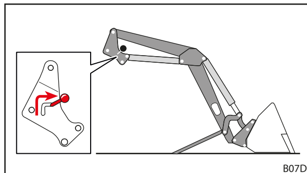
Fig. 46 Deschiderea dispozitivului de blocare a încărcătorului frontal
