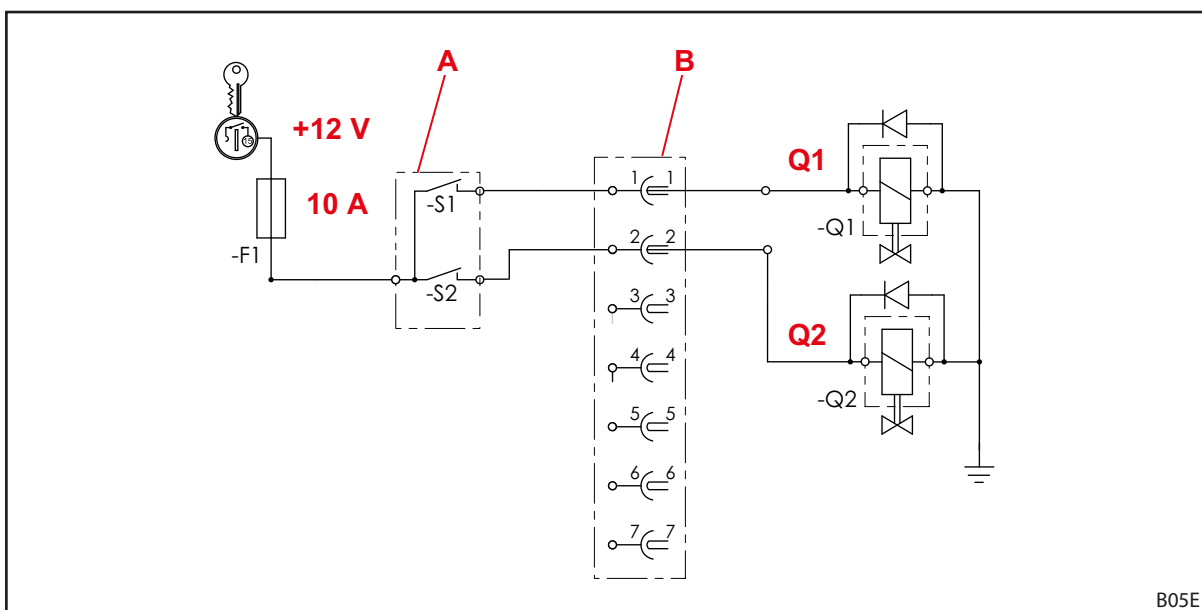
Fig. 121 Schema circuitelor electrice
