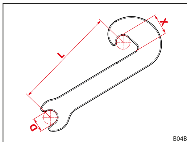
Fig. 111 Cota de uzură a cârligului de prindere
