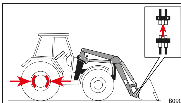
Fig. 99 Desfacerea conductelor hidraulice
