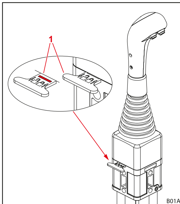
Fig. 60 Blocarea manetei de comandă (element de blocare orizontal)
