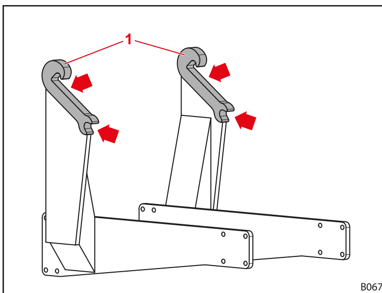
Fig. 108 Puncte de lubrifiere elemente de preluare încărcător frontal
