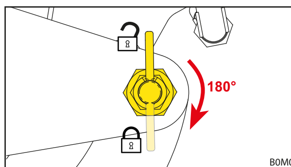
Fig. 35 Aducerea zăvorului de înclichetare în poziția blocat
