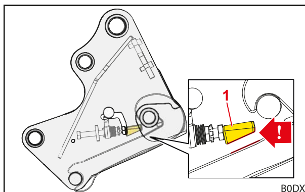
Fig. 52 Poziția de montare corectă a penei de fixare
