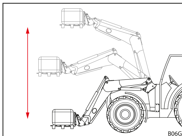
Fig. 32 Ghidare paralelă mecanică
