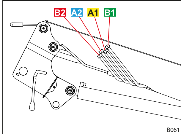
Fig. 20 Conductele hidraulice
