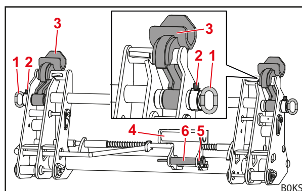
Fig. 87 Adaptor în poziția de lucru (cadru de înlocuire pregătit pentru unealta FR)
