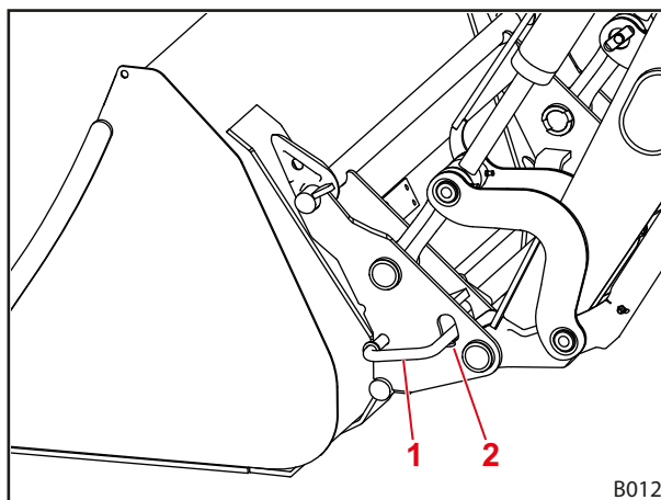
Fig. 75 Dispozitiv mecanic de blocare a uneltei
