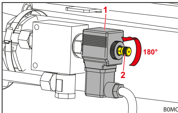
Fig. 33 Deschidere supapă
