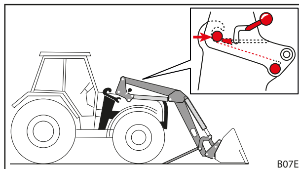
Fig. 47 Deplasați tractorul înspre brațul oscilant
