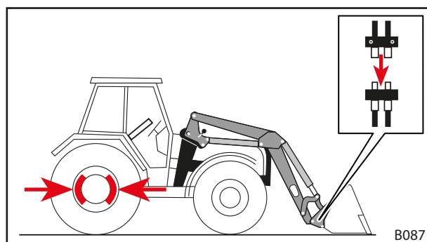
Fig. 93 Dacă este cazul racordați conductele hidraulice ale uneltei la cuplajele încărcătorului frontal
