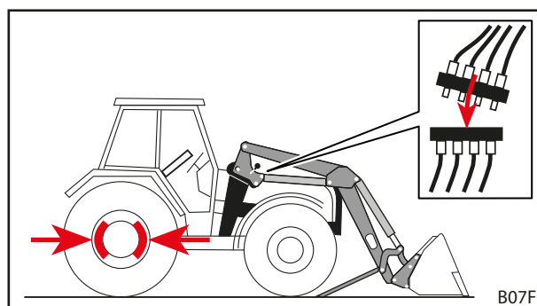
Fig. 48 Deconectarea tractorului și racordarea conductelor hidraulice
