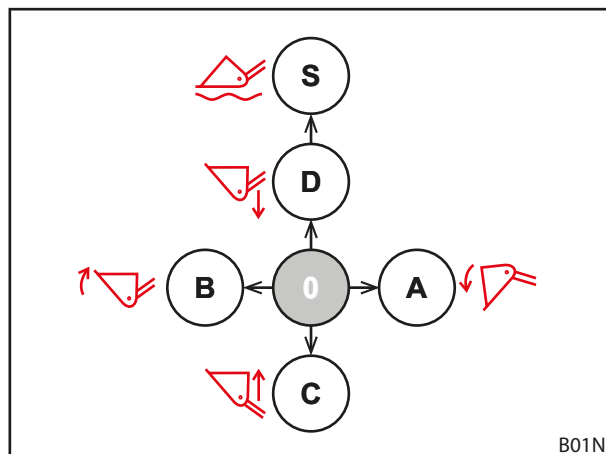
Fig. 57 Alocare la o manetă de comandă
