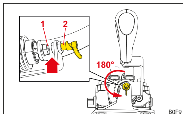
Fig. 65 Maneta de comandă deblocată
