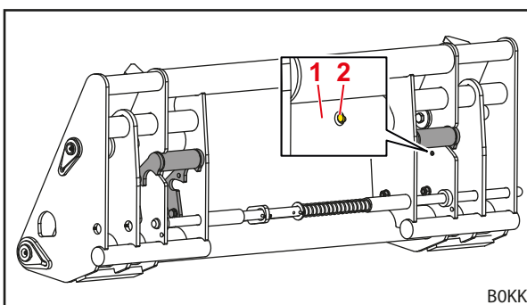
Fig. 85 Instalații pivotate în sus (vedere din spate)
