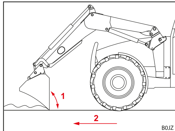
Fig. 103 Evacuare
