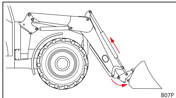
Fig. 91 Introducerea în cârlig
