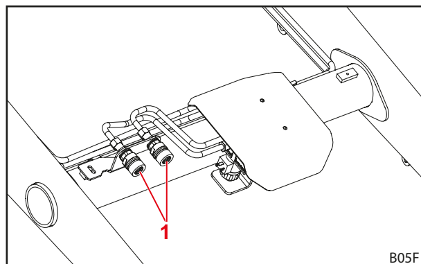
Fig. 38 Al 3-lea circuit de comandă suplimentar
