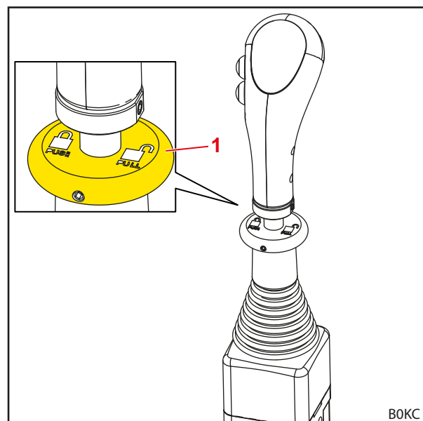
Fig. 61 Blocarea manetei de comandă (element de blocare vertical)
