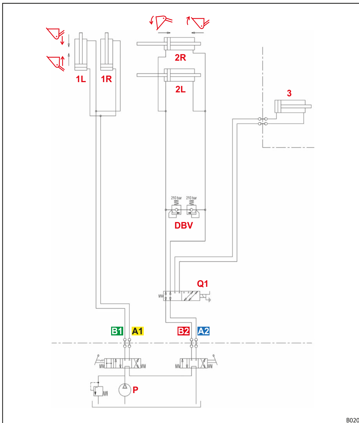
Fig. 120 Schema hidraulică P
