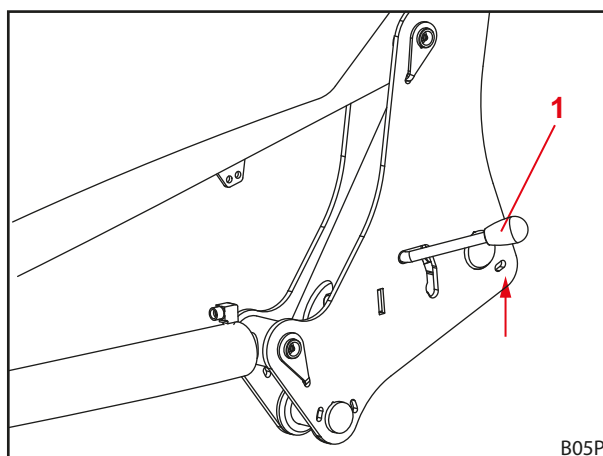
Fig. 53 Deschiderea dispozitivului de blocare a încărcătorului frontal
