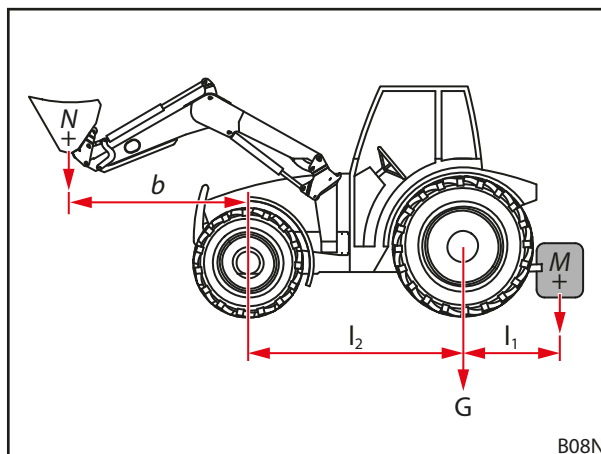
Fig. 45 Calculul stabilității statice
