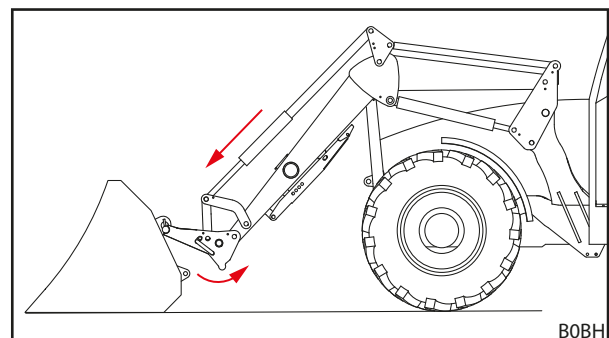
Рис. 93 Снятие сменной рамы
