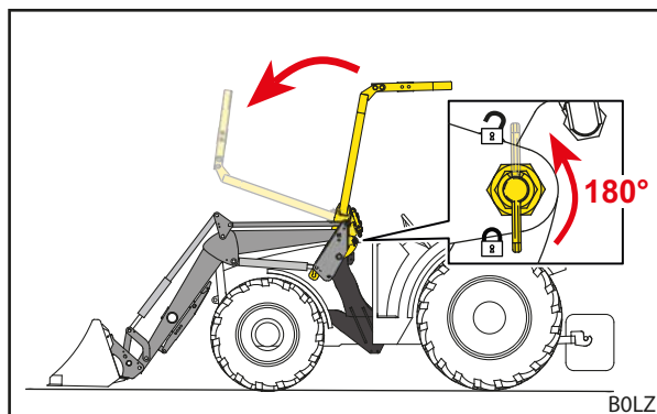
Рис. 33 Опускание OPG
