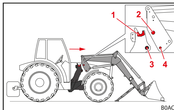
Рис. 45 Заезд трактором в стрелу
