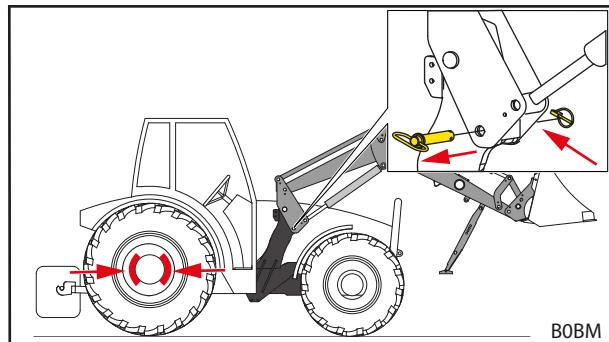
Рис. 110 Затягивание стояночного тормоза и ослабление запирающего механизма фронтального погрузчика
