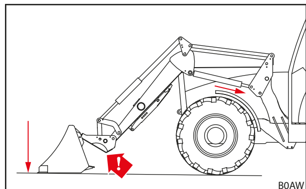
Рис. 71 Прижмите рабочий орган к земле
