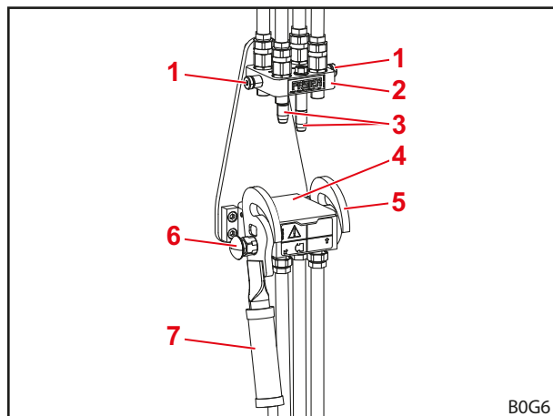
Рис. 62 Снятый узел Hydro-Fix
