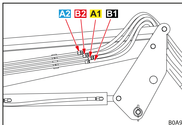
Рис. 16 Трубопроводы гидросистемы
