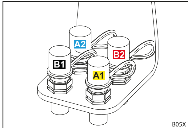
Рис. 17 Штекеры штекерных муфт на монтажном элементе
