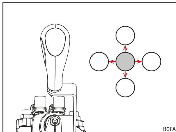
Рис. 58 Перевод рычага управления во все конечные положения
