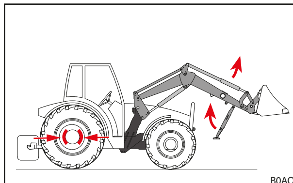
Рис. 49 Складывание стояночных опор
