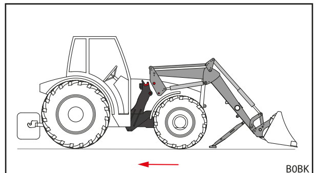
Рис. 113 Подать трактор назад
