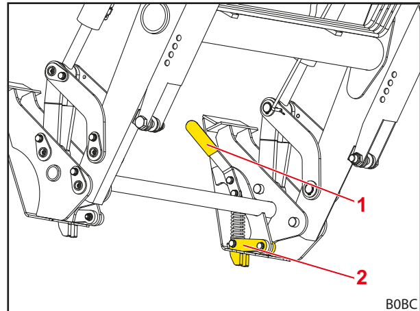
Рис. 70 Механический запирающий механизм рабочего органа на раме Skid-Steer (зафиксированное состояние без рабочего органа)
