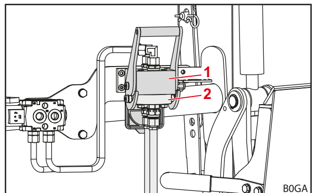
Рис. 65 Подсоединенный Implement-Fix
