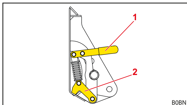
Рис. 66 Механический запирающий механизм рабочего органа на раме Skid-Steer (открытое состояние)
