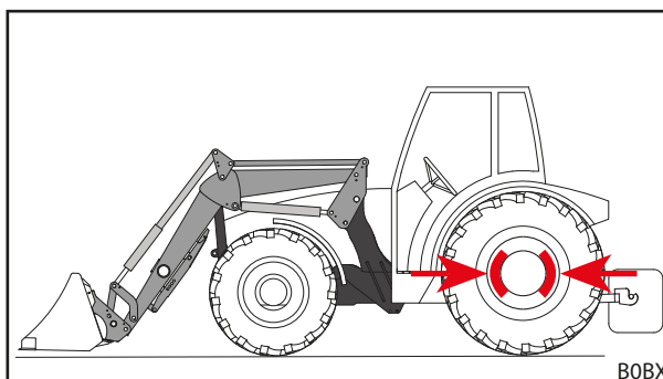
Рис. 95 Установка рабочего органа в положение для снятия и активация стояночного тормоза
