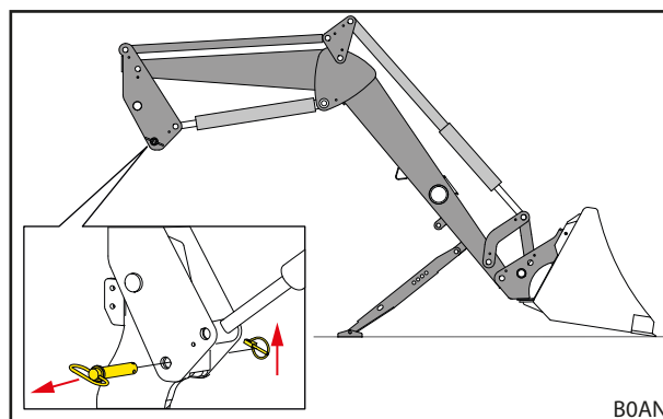
Рис. 44 Открытие запирающего механизма погрузчика
