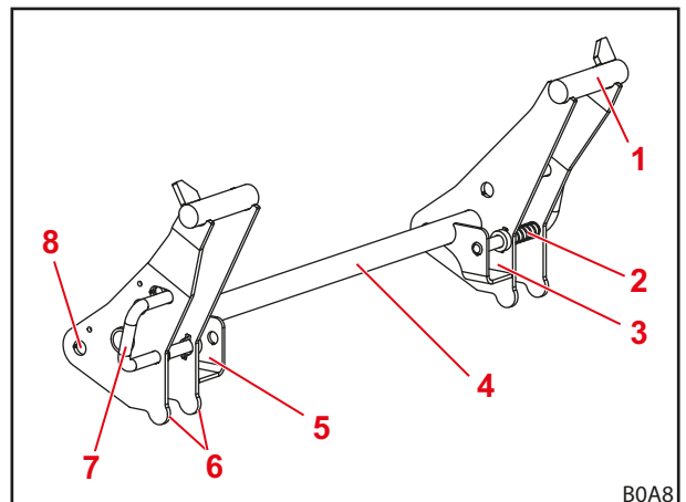
Рис. 72 Запирающий механизм рабочего органа на сменных рамах Euro
