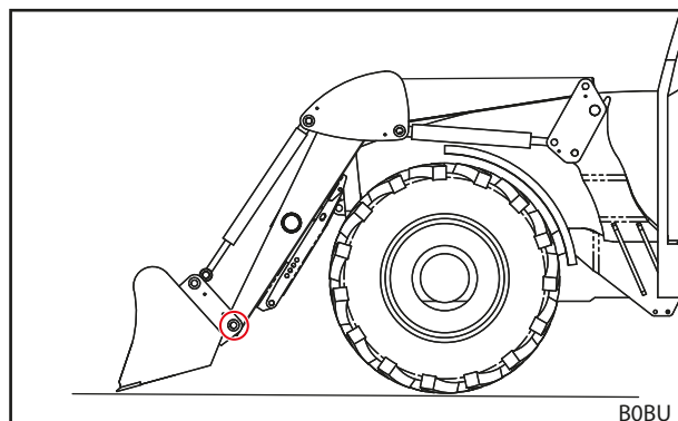
Рис. 87 Соединение рабочего органа через нижние отверстия для пальцев
