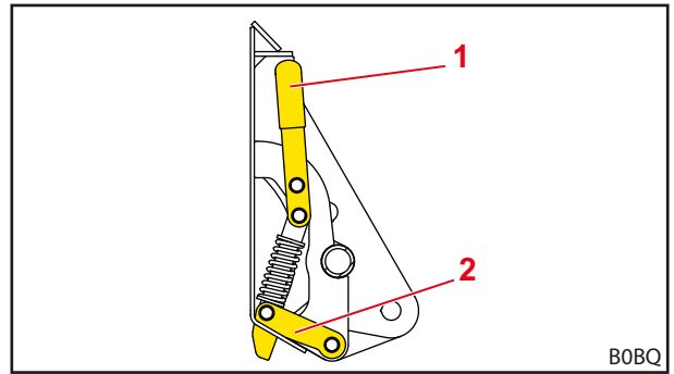
Рис. 68 Механический запирающий механизм рабочего органа на раме Skid-Steer (зафиксированное состояние)
