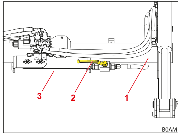
Рис. 39 Comfort-Drive с механическим приводом (рычаг в положении включения Comfort-Drive)
