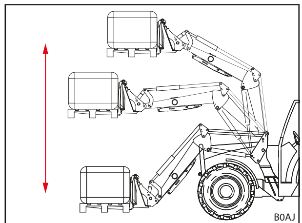
Рис. 32 Устройство параллельного ведения
