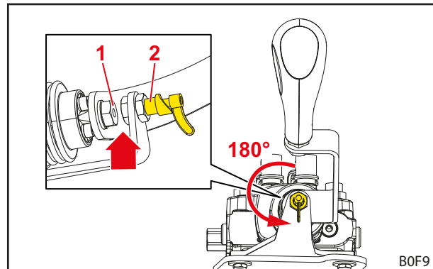
Рис. 57 Разблокированный рычаг управления
