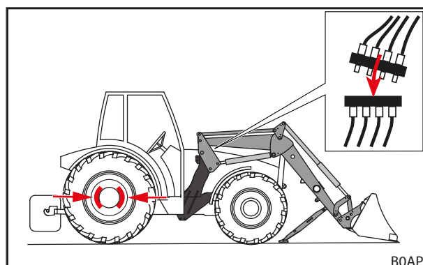
Рис. 46 Выключение трактора и подключение гидравлических шлангов
