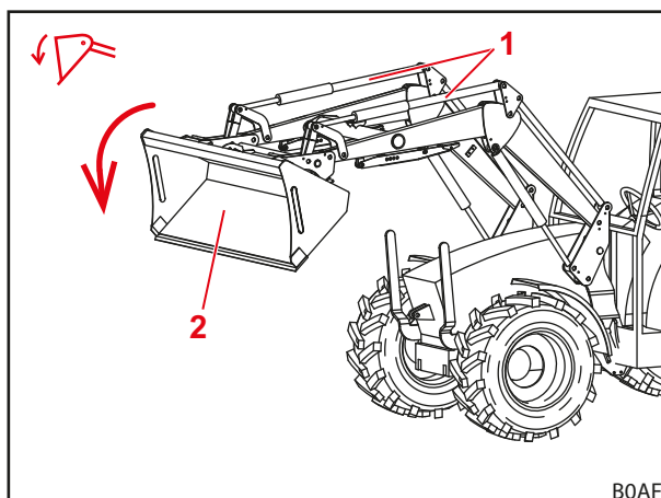
Рис. 29 Функция «Опрокидывание»
