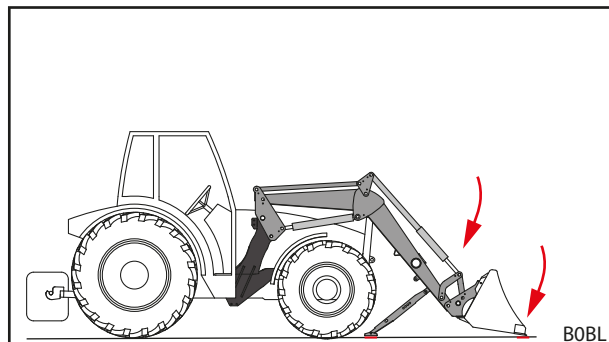
Рис. 111 Опускание фронтального погрузчика и опрокидывание рабочего органа
