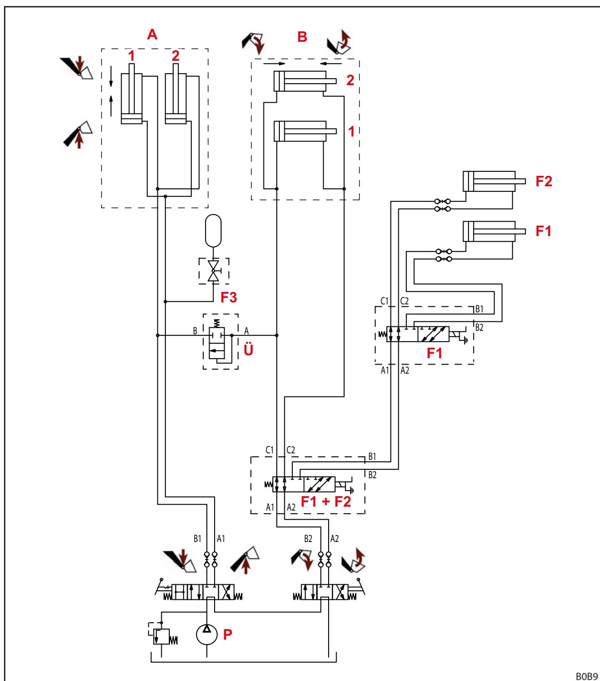
Рис. 114 Гидросхема фронтального погрузчика FC
