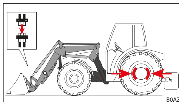
Рис. 80 Подсоединение линии гидравлики
