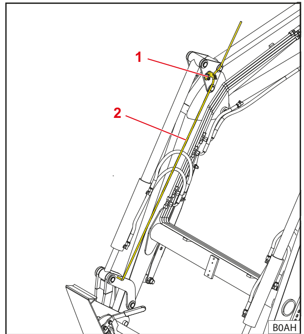
Рис. 31 Визуальный индикатор положения рабочего органа
