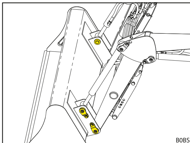
Рис. 89 Подсоединенный рабочий орган
