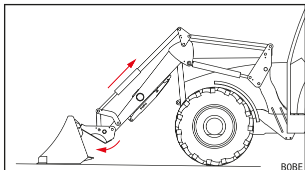
Рис. 78 Зацепление
