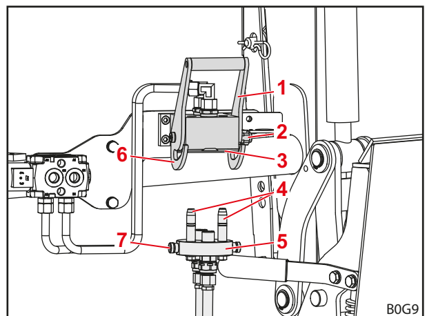
Рис. 64 Снятый узел Implement-Fix
