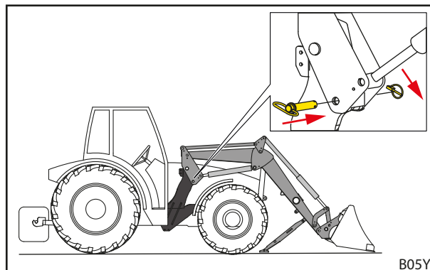
Рис. 48 Вставьте фиксирующие пальцы и закрепите их шплинтом с кольцом.
