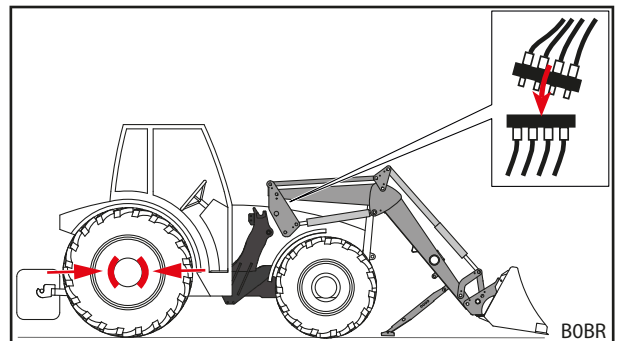
Рис. 112 Отсоединить гидравлику
