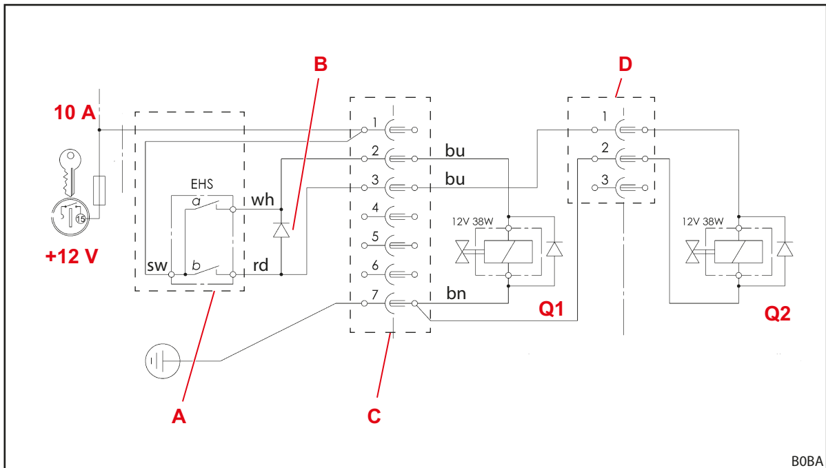
Рис. 115 Схема электрики
