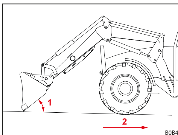
Рис. 99 Планировка задним ходом
