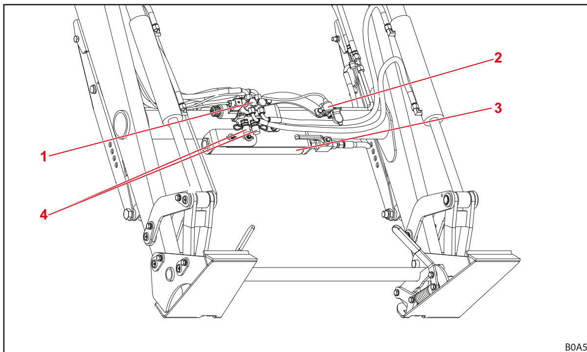
Рис. 12 Дополнительное оборудование для фронтальных погрузчиков L, H и P (примерное изображение)
