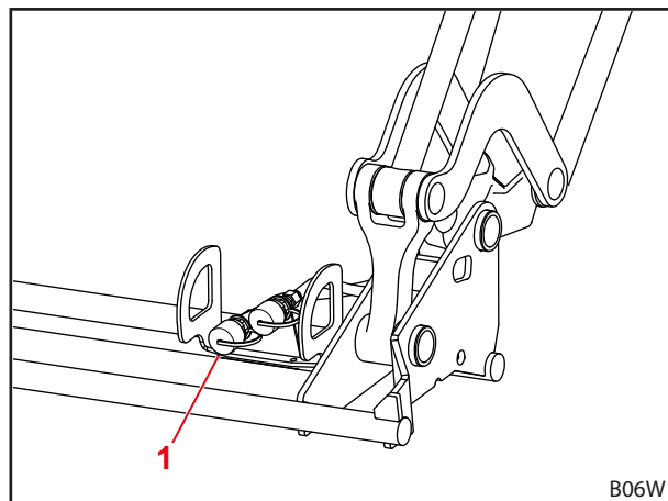
Рис. 44 REAL 3
