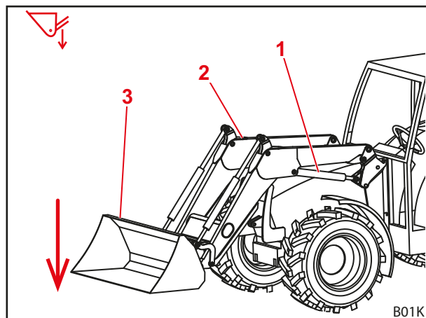
Рис. 24 Функция «Опускание»
