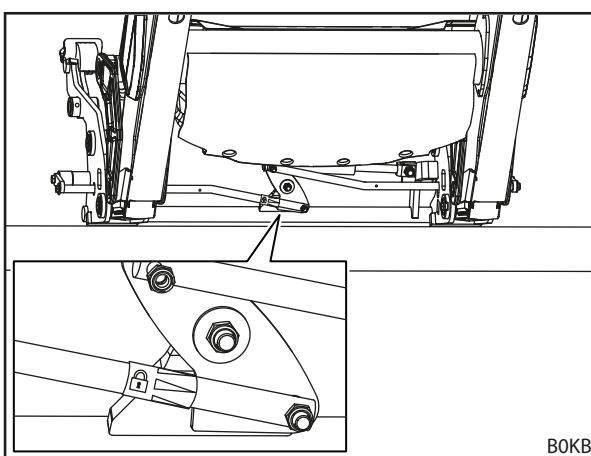
Рис. 83 Проверка запирающего механизма рабочего органа по наклейке
