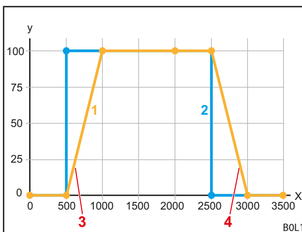
Рис. 31 Регулируемый отклик
