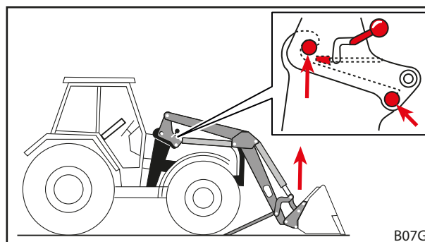
Рис. 55 Использование функции «Подъем», пока пальцы фронтального погрузчика не будут находиться в захватных крюках
