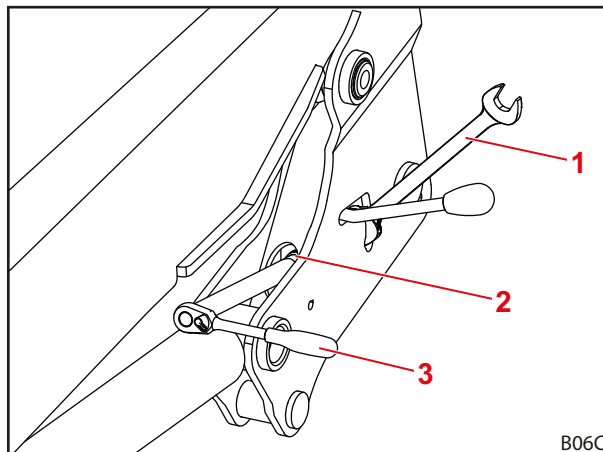
Рис. 59 Применение инструмента
