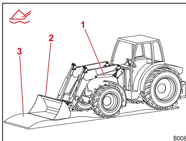
Рис. 39 Фронтальный погрузчик в плавающем положении
