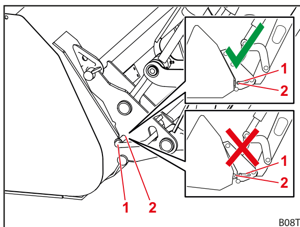
Рис. 79 Проверка положения фиксирующих пальцев
