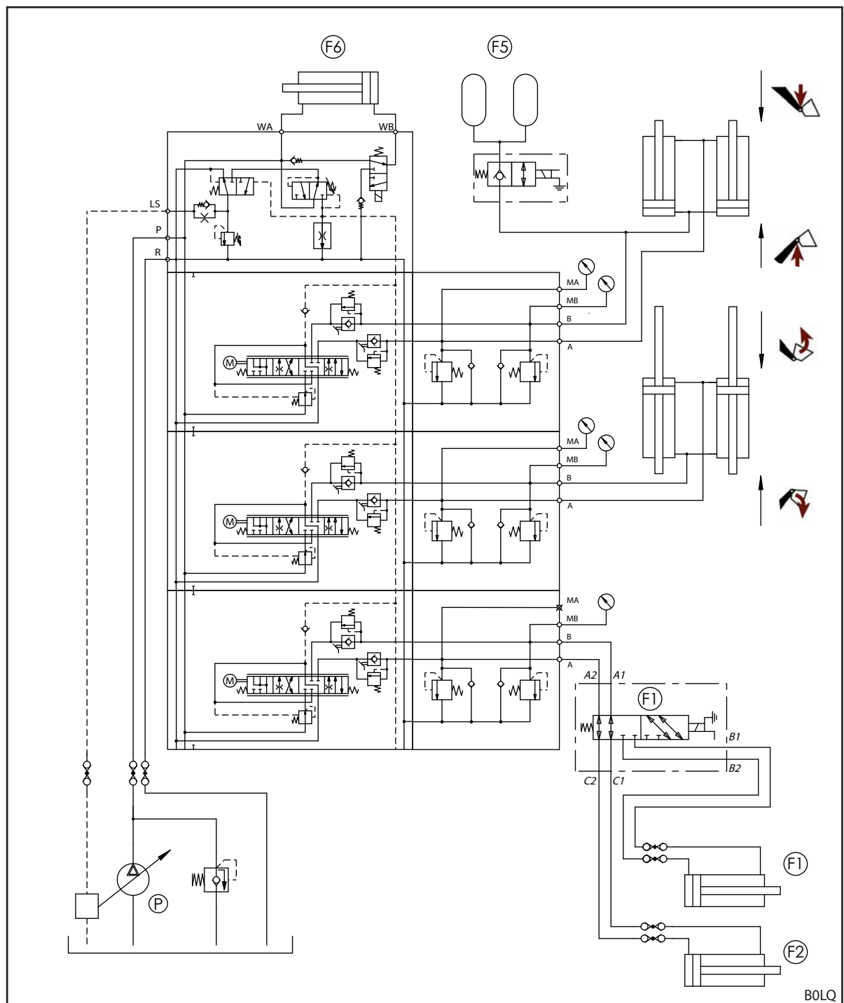
Рис. 126 Гидросхема погрузчика FS IB+ и FZ IB+
