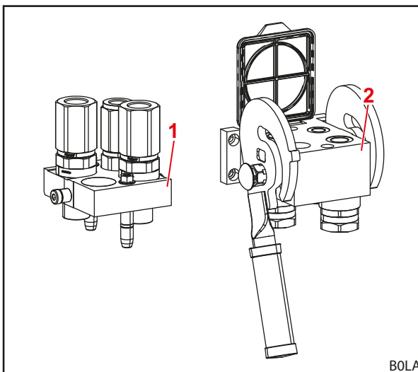
Рис. 19 Конструкция Hydro-Fix
