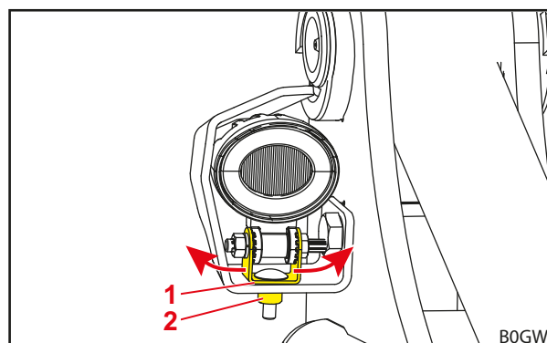
Рис. 46 Регулировка фар в горизонтальной плоскости
