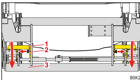
Рис. 86 Опустите опоры
