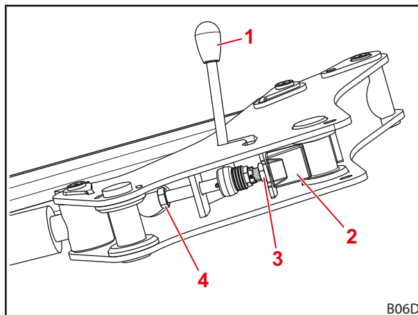
Рис. 61 Вид на механизм запирания погрузчика снизу
