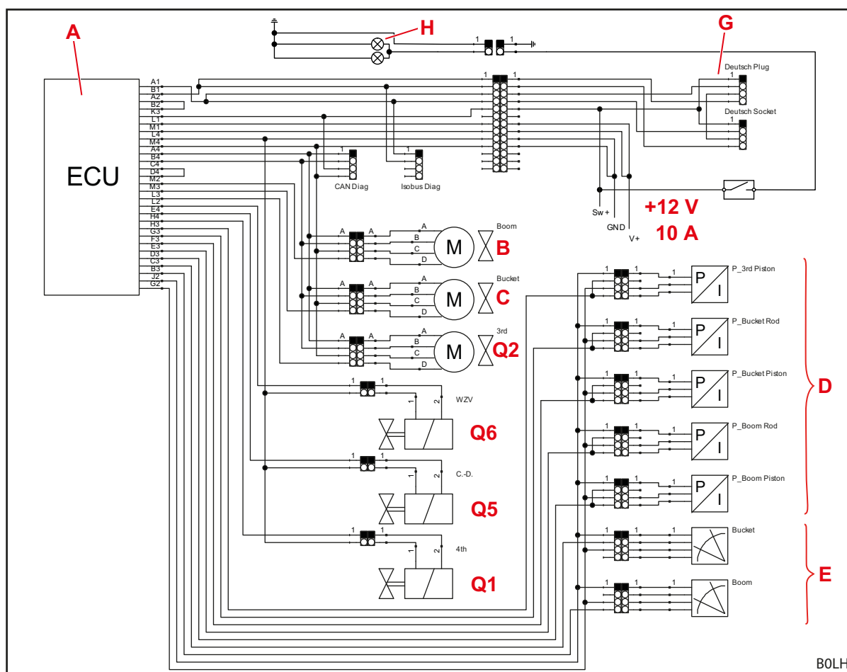
Рис. 127 Схема электрики
