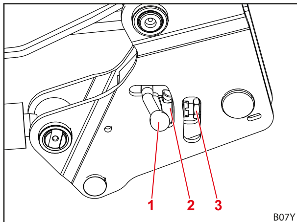
Рис. 62 Открытие запирающего механизма погрузчика
