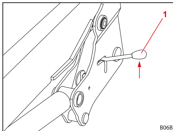
Рис. 58 Открытие запирающего механизма погрузчика
