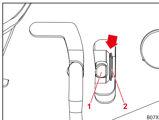
Рис. 118 Проверка зазора
