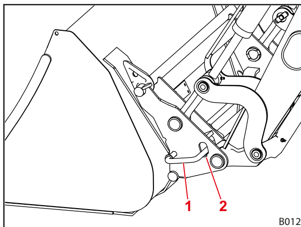
Рис. 76 Механическое запирание рабочего органа
