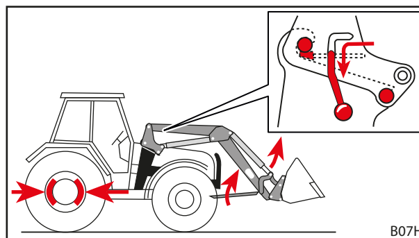
Рис. 56 Складывание стояночных опор и запирание запорного механизма погрузчика
