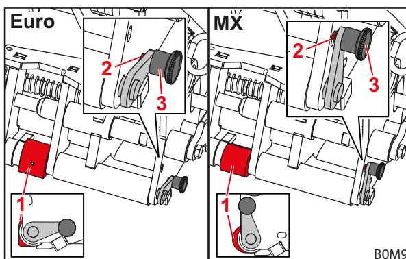
Рис. 90 Положения минификсатора
