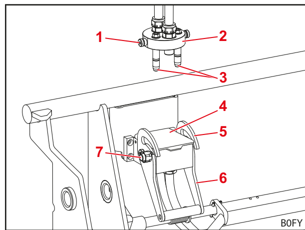
Рис. 74 Снятый узел Implement-Fix
