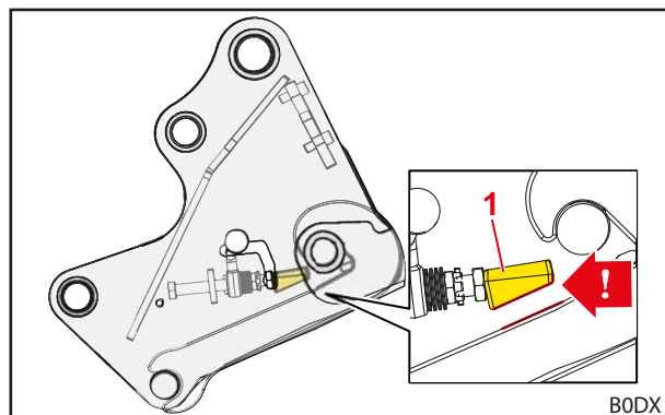
Рис. 57 Правильное монтажное положение зажимного клина
