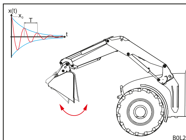
Рис. 34 Встряхивание ковша
