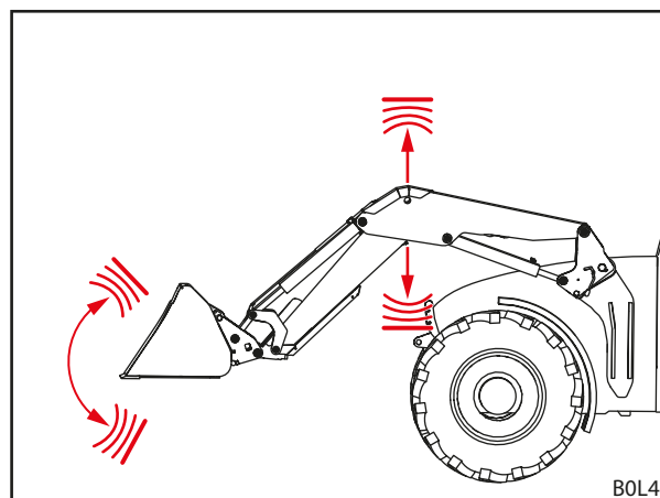
Рис. 33 Демпфирование в конечном положении
