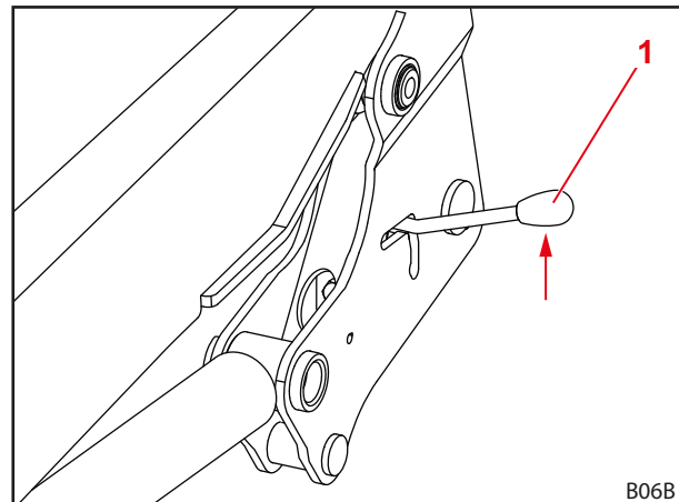
Рис. 116 Проверка запирающего механизма погрузчика
