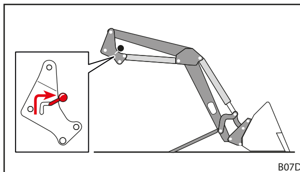
Рис. 52 Открытие запирающего механизма погрузчика
