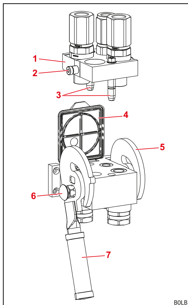
Рис. 73 Hydro-Fix
