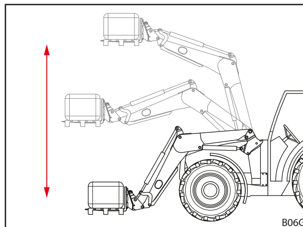
Рис. 41 Механическое устройство параллельного ведения
