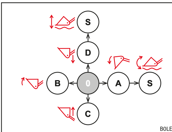
Рис. 67 Назначение положения рычага управления
