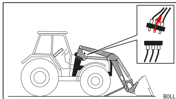
Рис. 123 Отсоединить гидравлику
