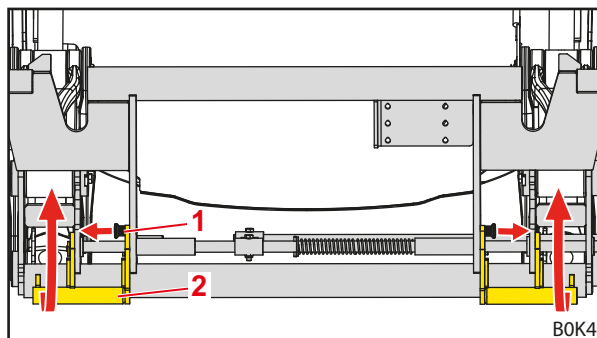
Рис. 88 Подъем опор
