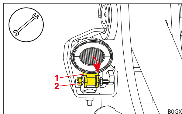
Рис. 47 Регулировка фар в вертикальной плоскости
