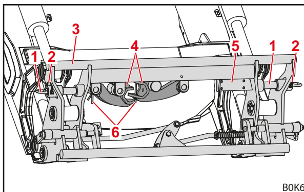
Рис. 13 Комбинированная сменная рама Euro-MX (подготовлена для рабочих органов Euro)
