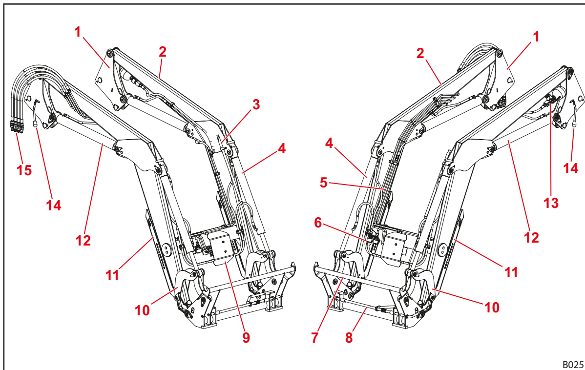
Рис. 9 Фронтальный погрузчик Н (без механического устройства параллельного ведения)
