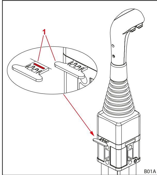
Рис. 60 Блокировка рычага управления (горизонтальная блокировка)
