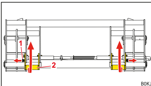
Рис. 84 Подъем опор
