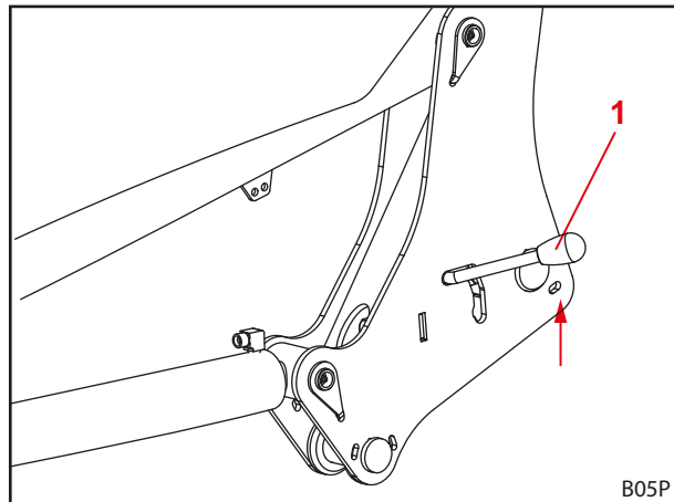
Рис. 53 Открытие запирающего механизма погрузчика
