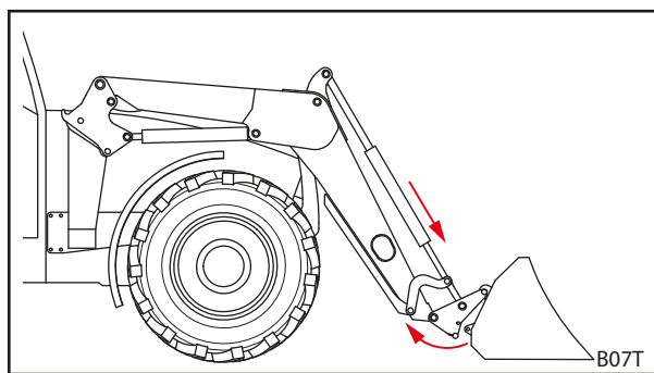
Рис. 100 Снятие сменной рамы
