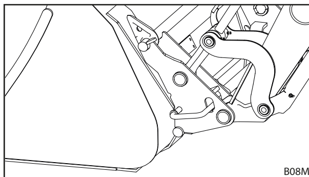
Рис. 88 Открытие запирающего механизма рабочего органа
