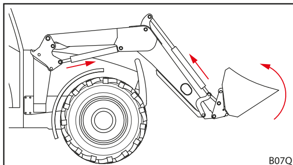
Рис. 92 Срабатывание запирающего механизма рабочего органа
