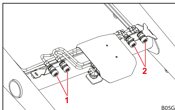
Рис. 39 Дополнительная 4-я линия гидравлики
