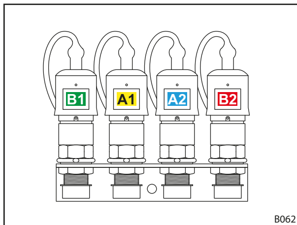
Рис. 21 Соединение штекерных муфт
