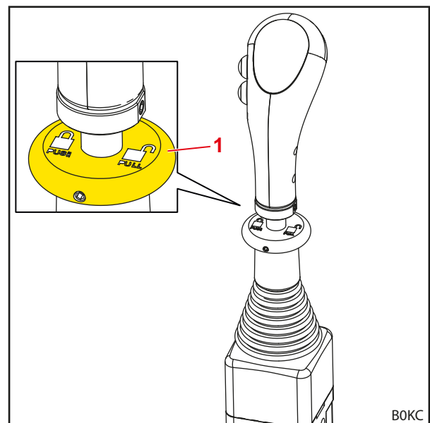
Рис. 61 Блокировка рычага управления (вертикальная блокировка)
