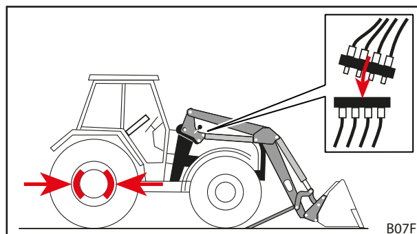
Рис. 48 Выключение трактора и подключение гидравлических шлангов
