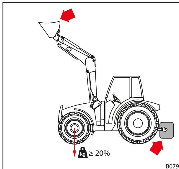
Рис. 44 Нагрузка при движении по дорогам
