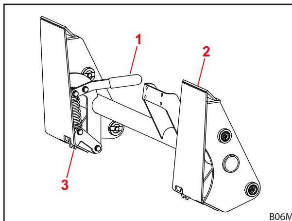
Рис. 25 Механический запирающий механизм рабочего органа на сменных рамах Skid-Steer
