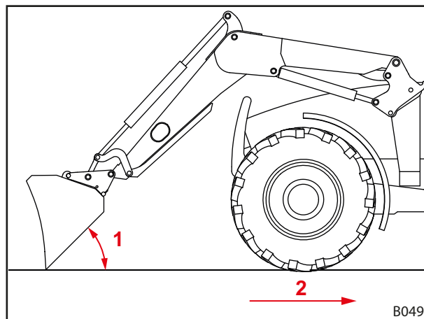
Рис. 102 Планировка задним ходом
