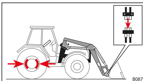
Рис. 93 Соедините гидравлические шланги рабочего органа с муфтами погрузчика
