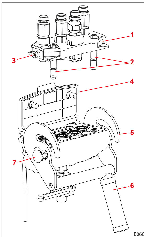
Рис. 74 Hydro-Fix (пример: Hydro-Fix с 4 разъемами)
