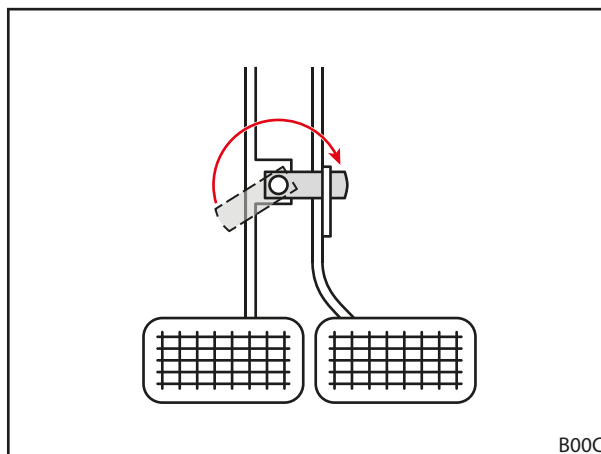
Рис. 42 Объединение педалей тормоза
