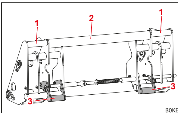
Рис. 15 Комбинированная сменная рама Euro-SMS (подготовлена для рабочих органов Euro)
