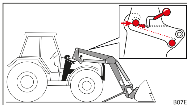
Рис. 47 Заезд трактором в стрелу
