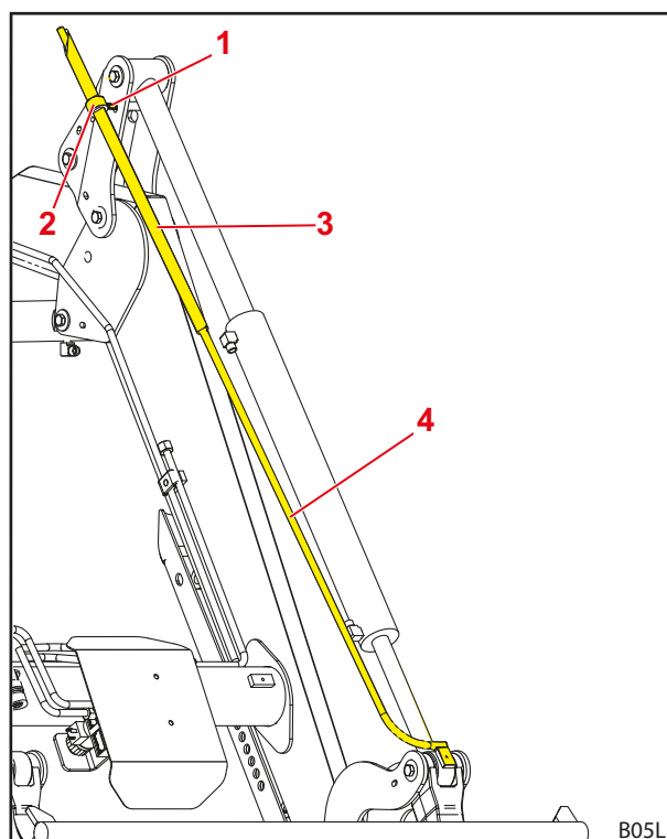
Рис. 31 Визуальный индикатор настройки рабочего органа
