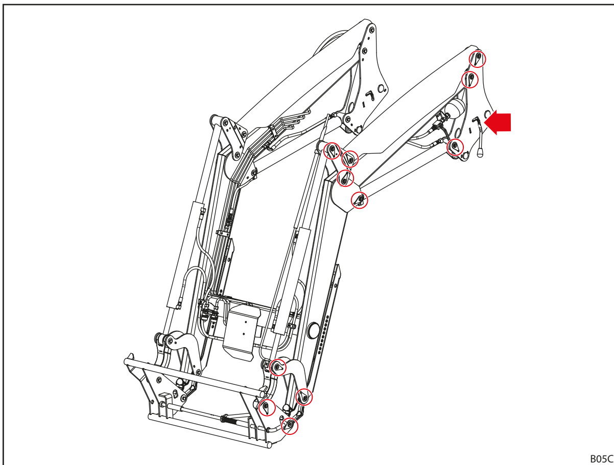
Рис. 110 Точки смазки Р
