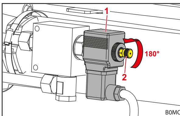
Рис. 33 Открыть клапан
