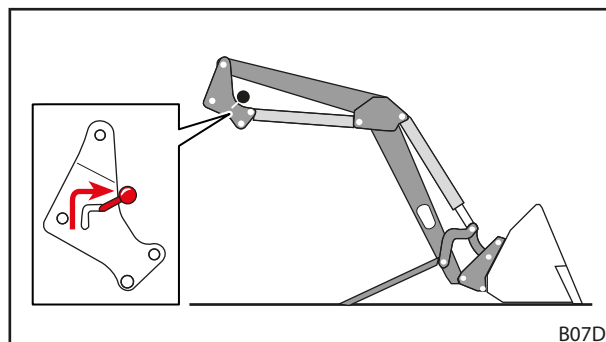
Рис. 46 Открытие запирающего механизма погрузчика
