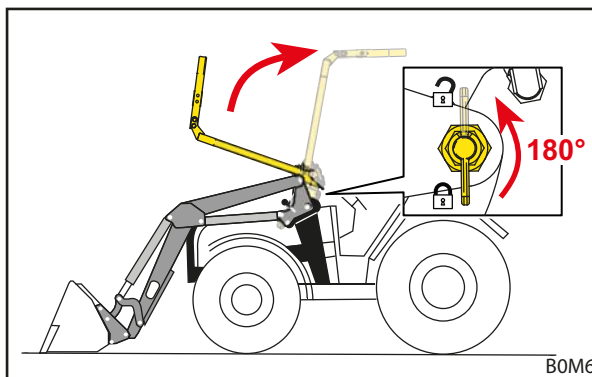
Рис. 36 Подъем OPG
