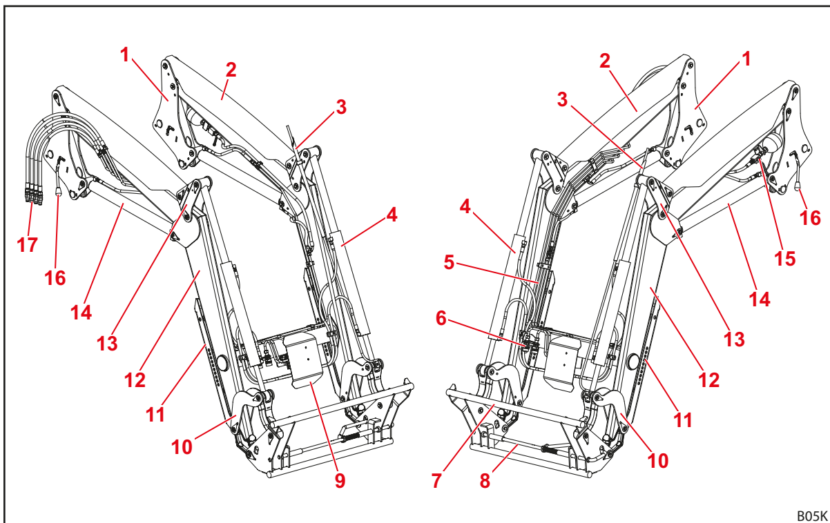
Рис. 10 Фронтальный погрузчик Р (с механическим устройством параллельного ведения)
