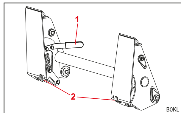
Рис. 14 Сменная рама Skid-Steer
