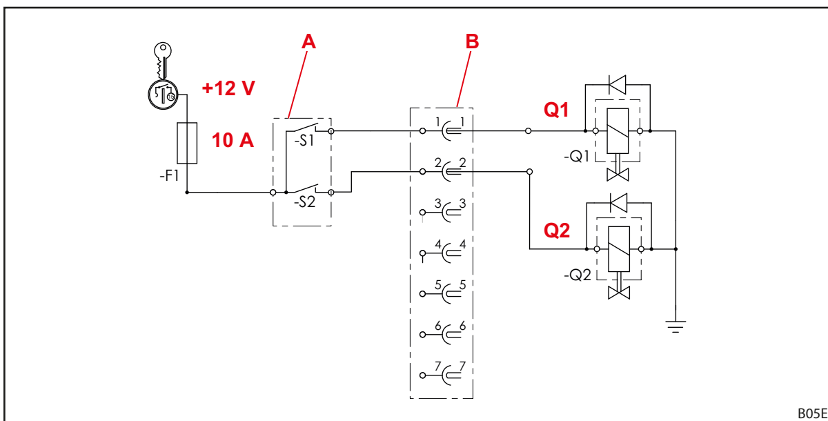
Рис. 121 Схема электрики
