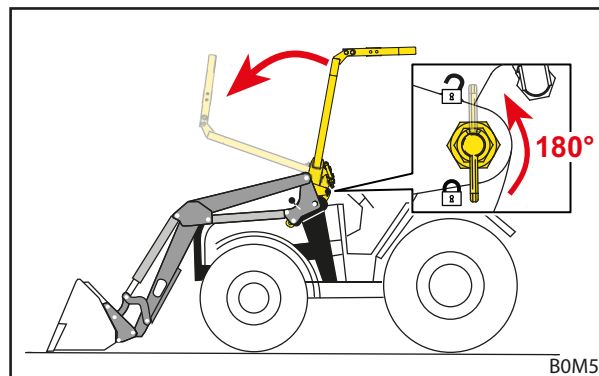
Рис. 34 Опускание OPG
