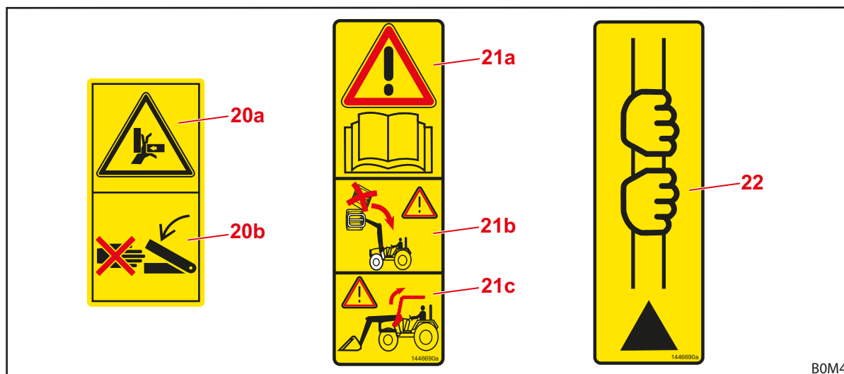
Рис. 8 Предупредительные наклейки
