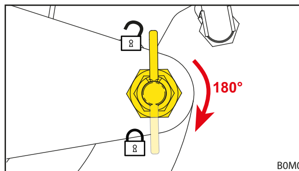
Рис. 35 Установка стопорного затвора в заблокированное положение
