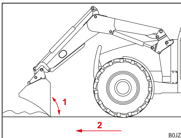
Рис. 110 Уборка
