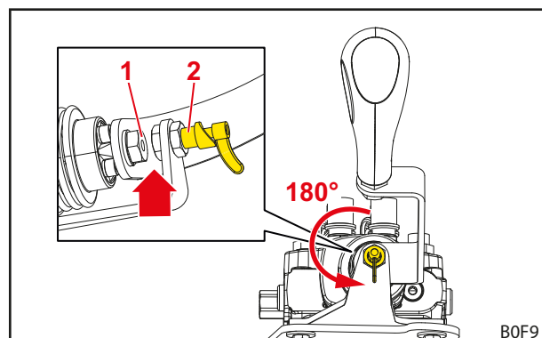
Рис. 72 Разблокированный рычаг управления
