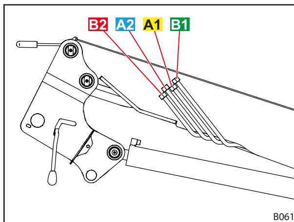
Рис. 22 Трубопроводы гидросистемы
