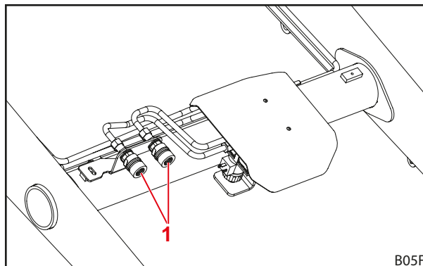
Рис. 45 Дополнительная 3-я линия гидравлики
