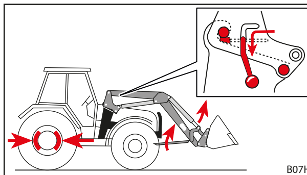
Рис. 58 Складывание стояночных опор и запирание запорного механизма погрузчика
