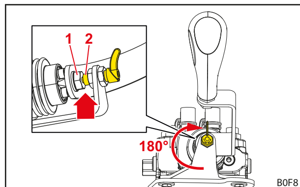
Рис. 71 Блокированный рычаг управления
