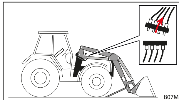
Рис. 124 Отсоединить гидравлику
