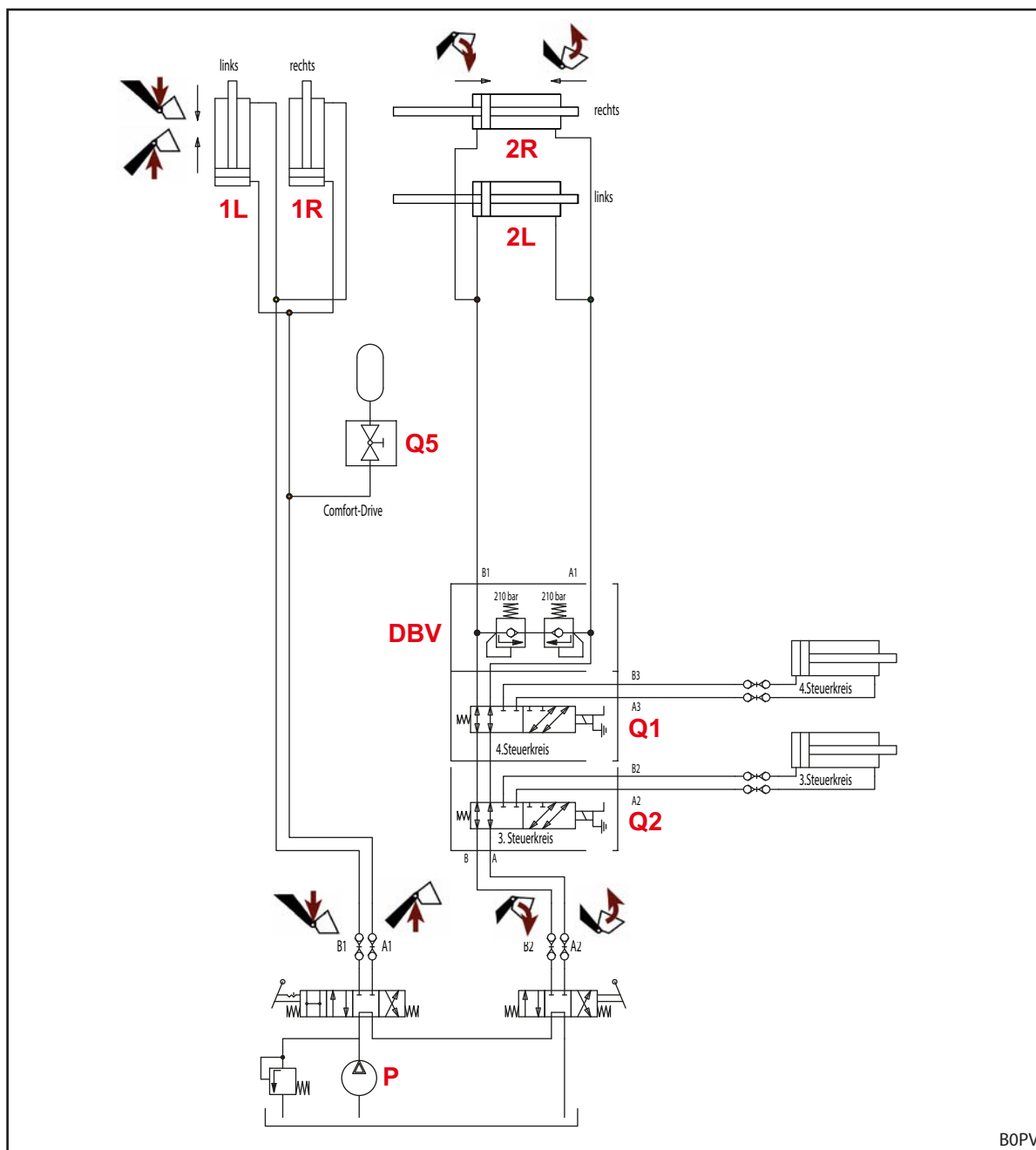
Рис. 127 Гидросхема P
