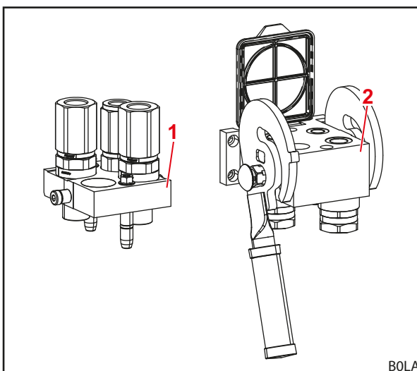
Sl. 19 Zgradba spojke Hydro-Fix
