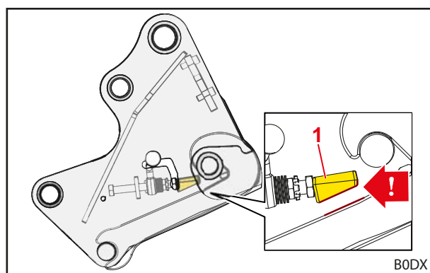
Sl. 57 Pravilen vgradni položaj prižemnega klina
