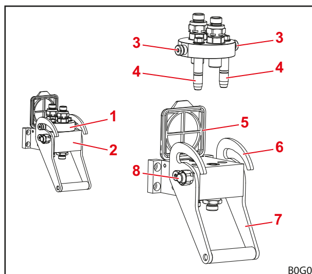
Sl. 21 Zgradba spojke Implement-Fix
