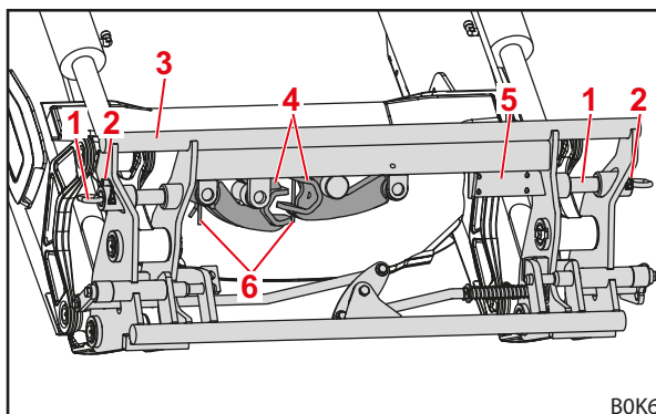
Sl. 13 Kombinirani priklopni okvir Euro-MX (pripravljen za orodje Euro)
