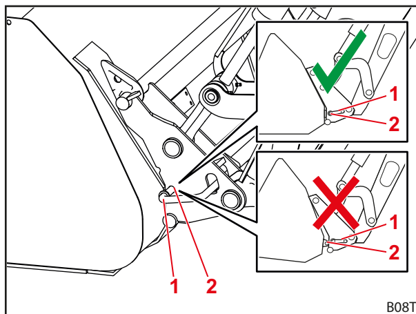
Sl. 79 Preverjanje položaja zapornega zatiča
