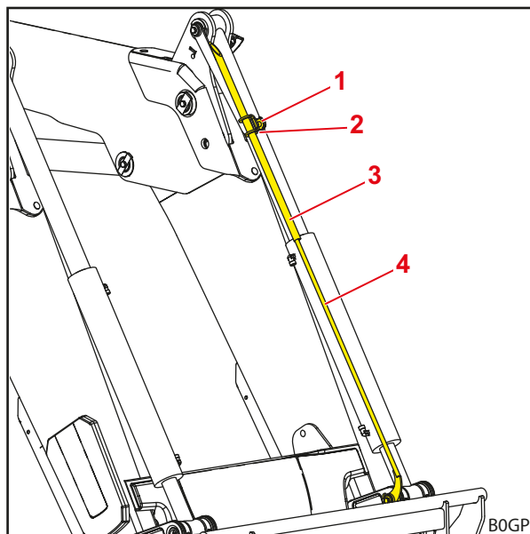
Sl. 40 Vizualni indikator za položaj orodja
