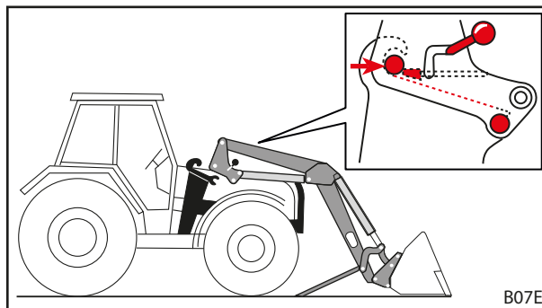
Sl. 53 Zapeljite traktor med roki
