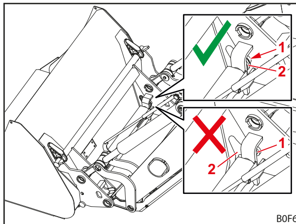
Sl. 84 Preverjanje položaja zapornega zatiča
