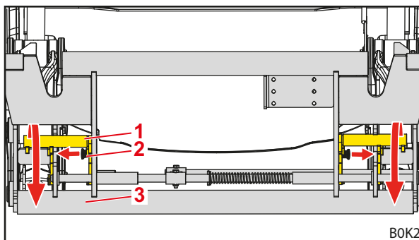
Sl. 86 Spuščanje naslonov
