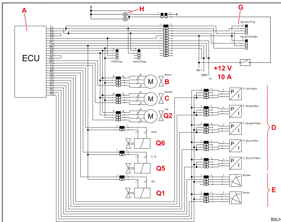
SI. 127 Električna stikalna shema
