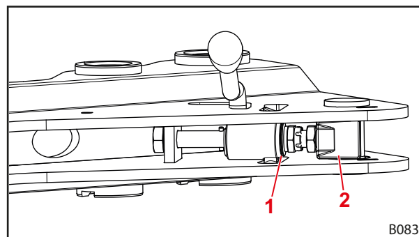
Sl. 65 Pogled na zaklep čelnega nakladalnika od spodaj
