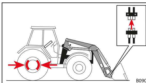
Sl. 102 Odklapljanje hidravličnih vodov
