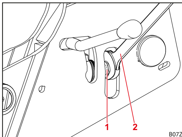
Sl. 66 Zategnite protimatico
