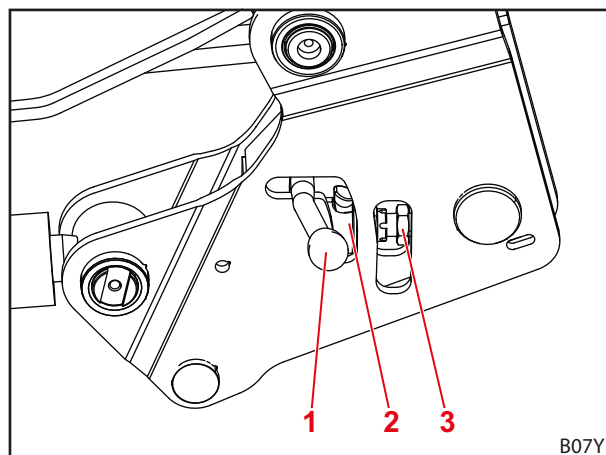
Sl. 62 Odpiranje zaklepa čelnega nakladalnika
