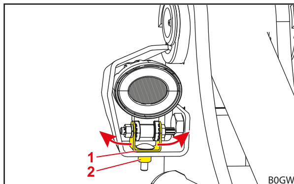
Sl. 46 Horizontalna nastavitev žarometa
