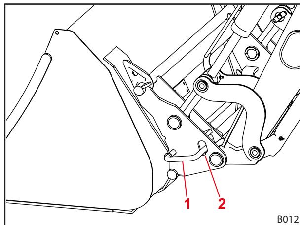
Sl. 76 Mehanski zaklep orodja
