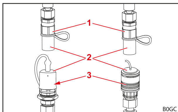
Sl. 71 Vtične spojke (primer)
