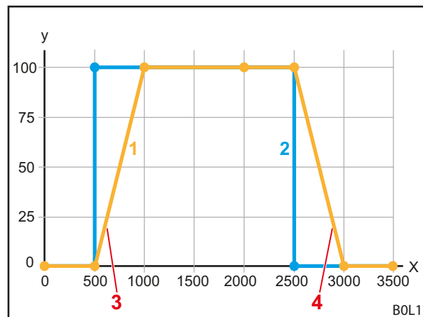
Sl. 31 Nastavljivo odzivanje
