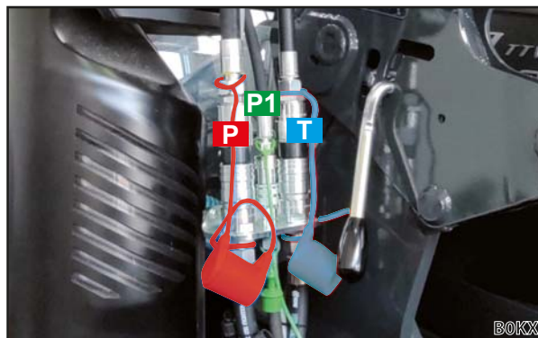
Sl. 17 Povezane spojke
