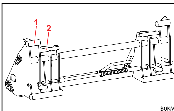
Sl. 17 Kombinirani priklopni okvir Euro-Alö3
