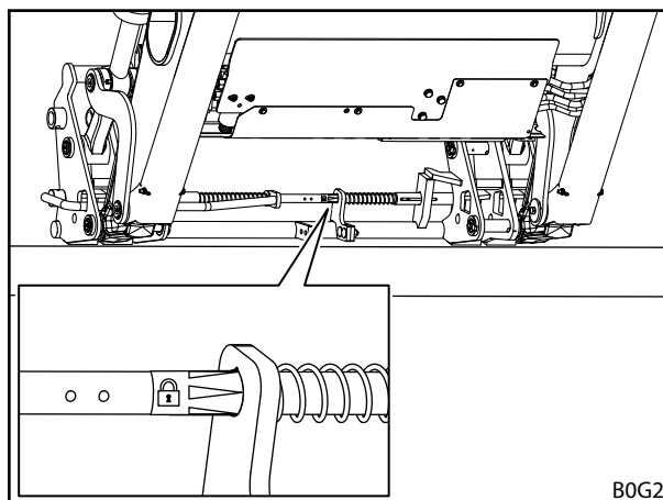
Sl. 77 Preverjanje zaklepa orodja s pomočjo nalepke (priklopni okvir Kombi Euro-FR)
