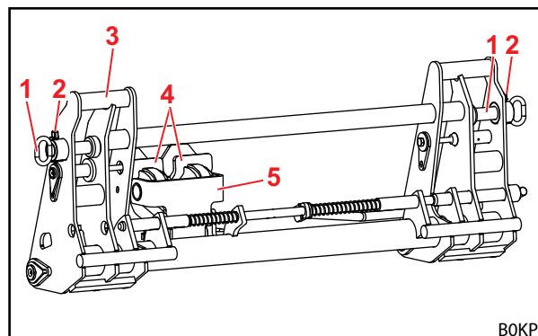
Sl. 18 Kombinirani priklopni okvir Euro-FR (pripravljen za orodje Euro)
