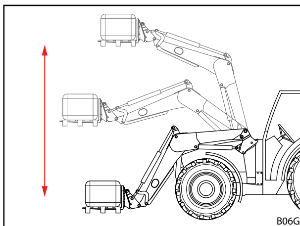
Sl. 32 Mehansko vzporedno vodenje
