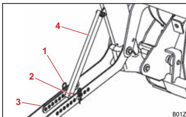
Sl. 71 Parkirni opornik
