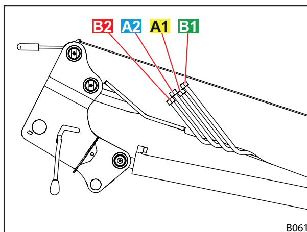
Sl. 20 Hidravlični vodi
