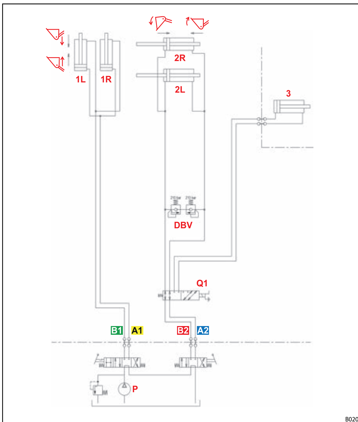
Sl. 120 Hidravlični načrt P
