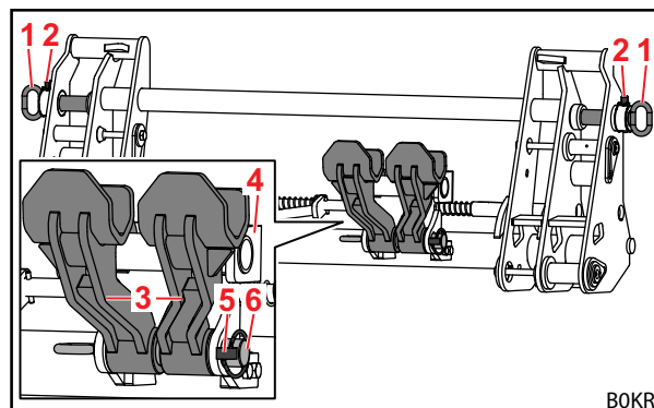
Sl. 86 Adapter v parkirnem položaju (priklopni okvir pripravljen za orodje Euro)
