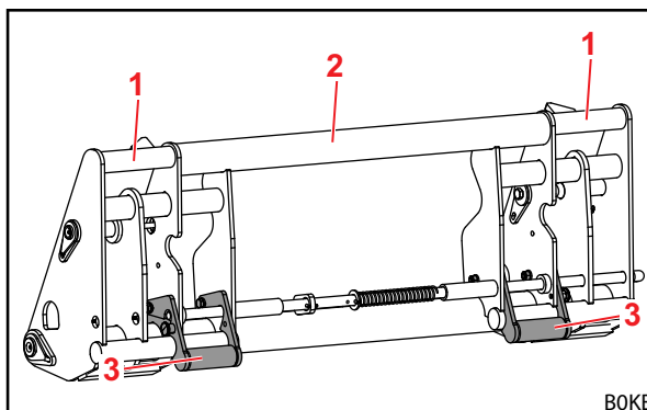
Sl. 15 Kombinirani priklopni okvir Euro-SMS (pripravljen za orodje Euro)
