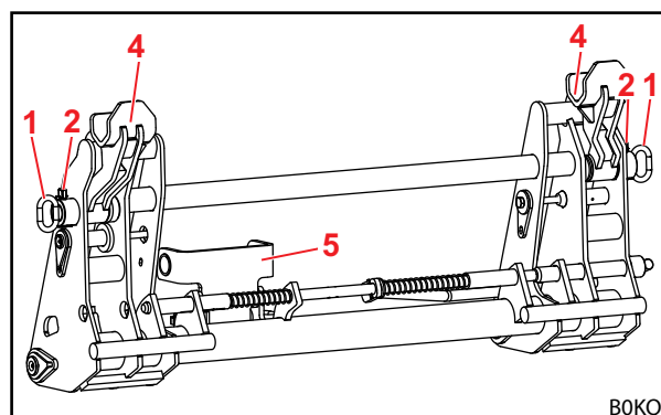
Sl. 19 Kombinirani priklopni okvir Euro-FR (pripravljen za orodje FR)
