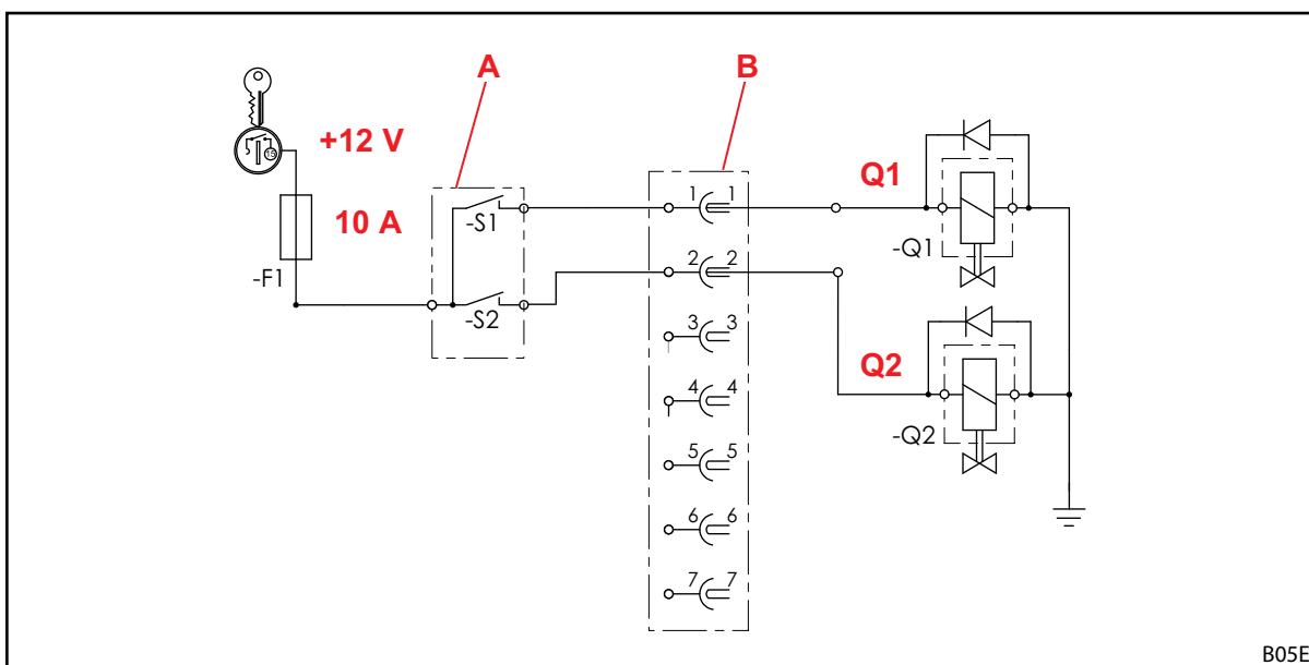
Sl. 121 Električna stikalna shema
