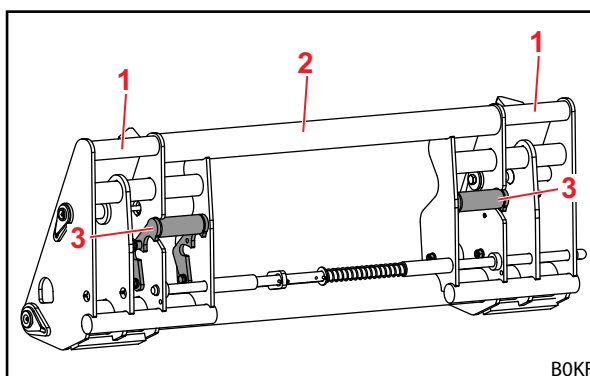
Sl. 16 Kombinirani priklopni okvir Euro-SMS (pripravljen za orodje SMS)
