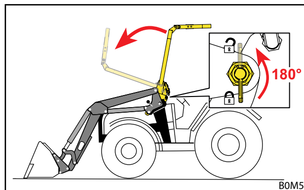
Sl. 34 Spuščanje sistema OPG
