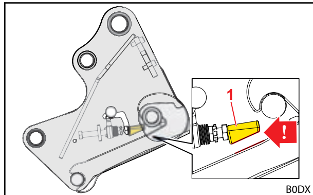
Sl. 52 Pravilen vgradni položaj prižemnega klina
