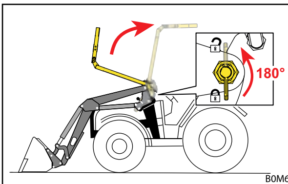
Sl. 36 Dvigovanje sistema OPG
