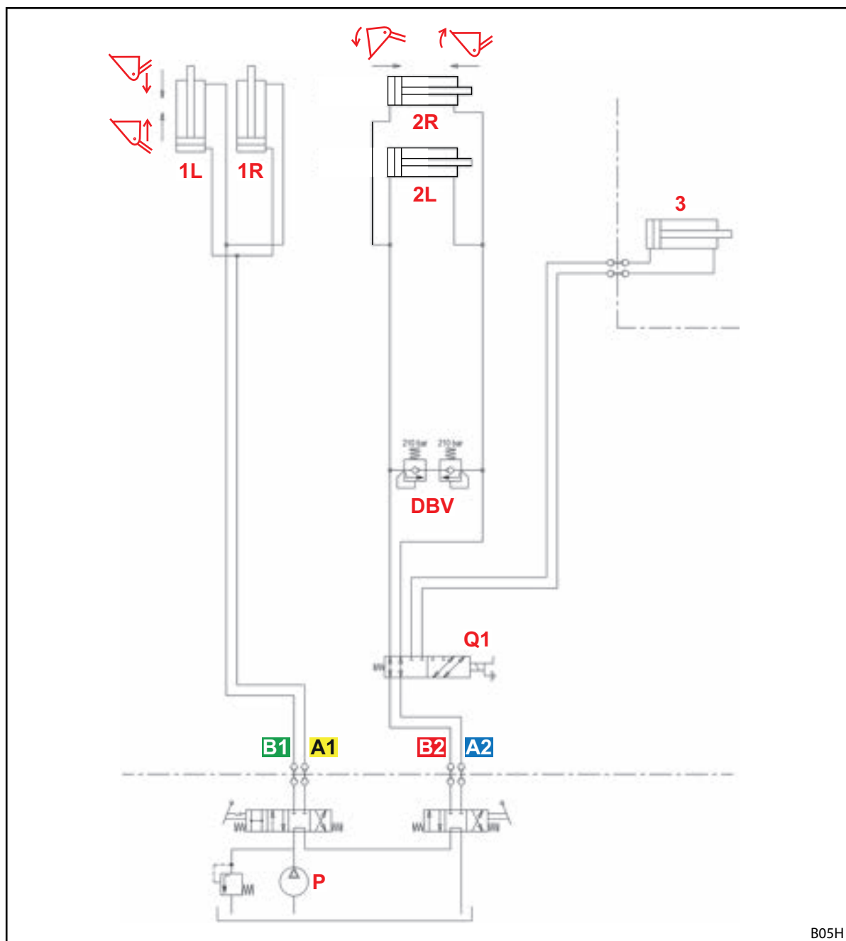
Sl. 119 Hidravlični načrt H
