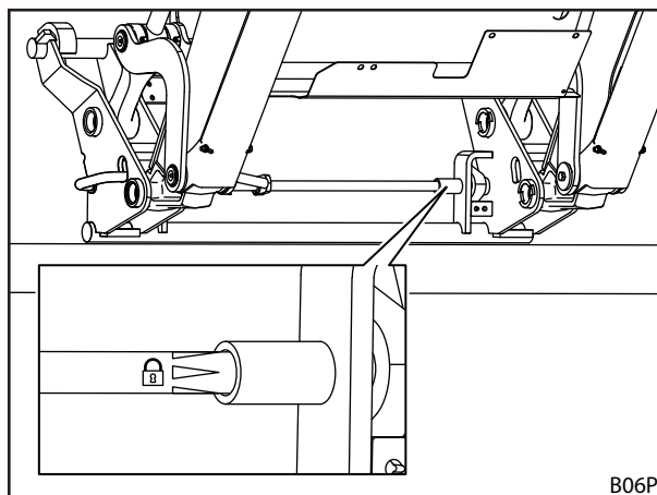
Sl. 76 Preverjanje zaklepa orodja s pomočjo nalepke
