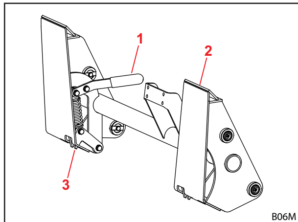
Sl. 25 Mehanski zaklep orodja pri priklopnih okvirjih Skid-Steer
