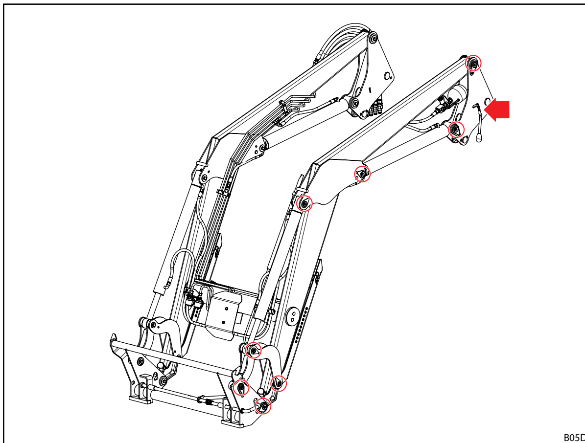
Sl. 109 Mazalna mesta pri tipu H
