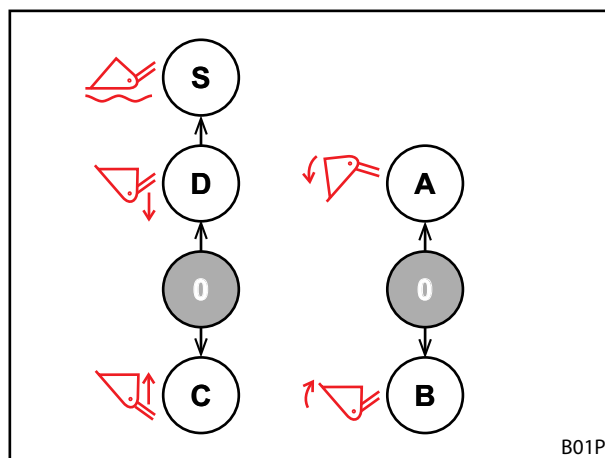
Sl. 58 Shema funkcij pri dveh upravljalnih ročicah
