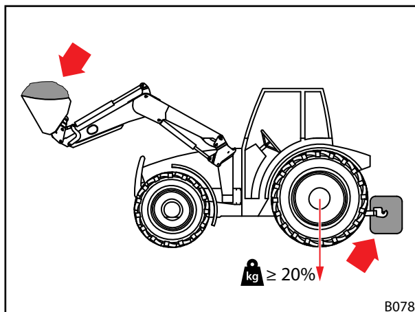
Sl. 43 Obtežitev pri uporabi čelnega nakladalnika
