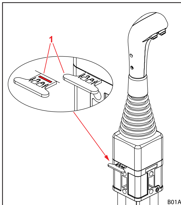
Sl. 60 Zaklepanje upravljalne ročice (vodoravni zaklep)
