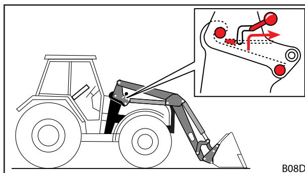
Sl. 115 Sprostitev zaklepa čelnega nakladalnika
