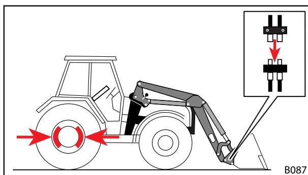
Sl. 93 Priključitev hidravličnih vodov orodja v spojke čelnega nakladalnika
