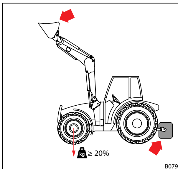
Sl. 44 Obtežitev pri vožnji po cesti
