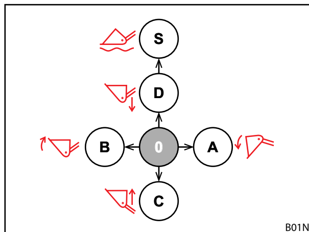
Sl. 57 Shema funkcij pri eni upravljalni ročici
