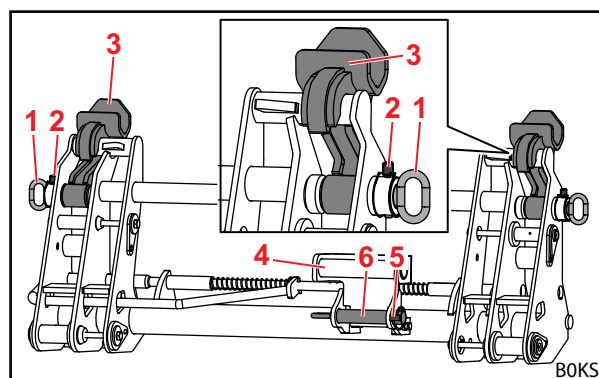
Sl. 87 Adapter v delovnem položaju (priklopni okvir pripravljen za orodje FR)
