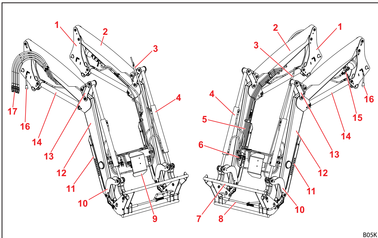
Sl. 10 Čelni nakladalnik P (z mehanskim vzporednim vodenjem)
