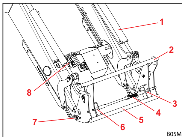
Sl. 13 Priklopni okvir Euro
