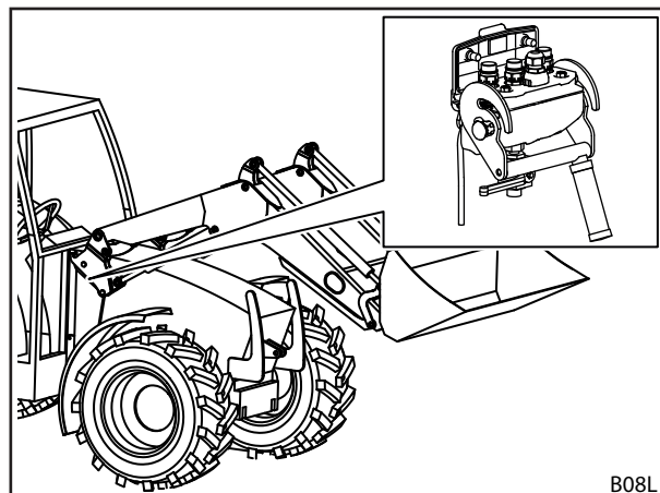
Sl. 22 Hydro-Fix: mesto na čelnem nakladalniku
