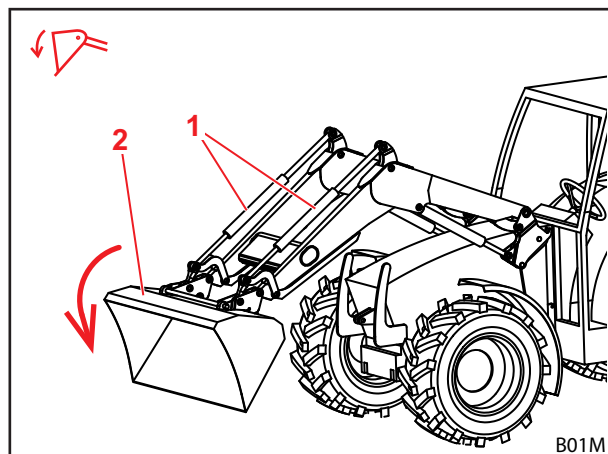
Sl. 29 Funkcija praznjenja
