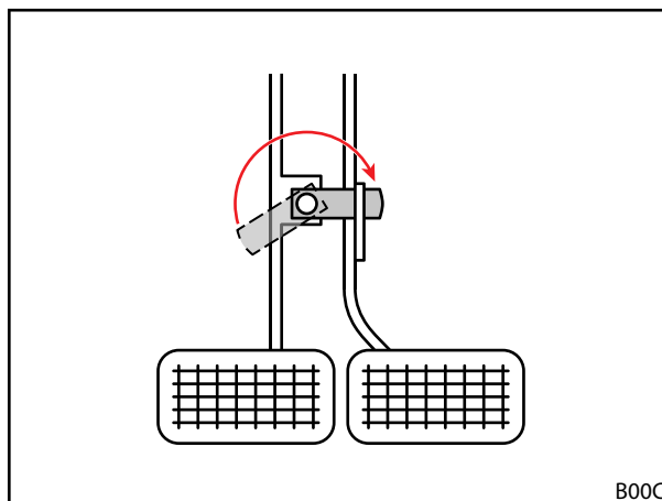
Sl. 42 Povezovanje zavornih pedalov
