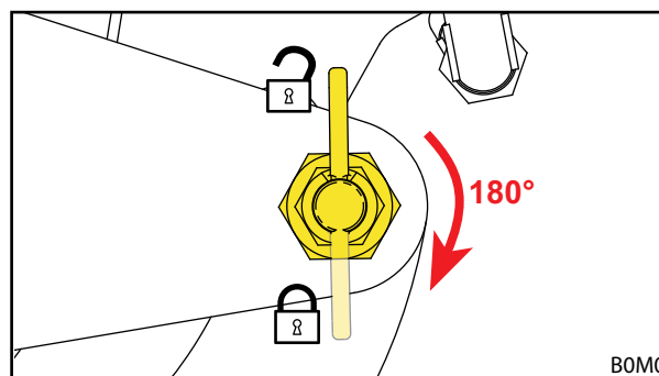
Sl. 35 Premik zapaha v zaklenjeni položaj
