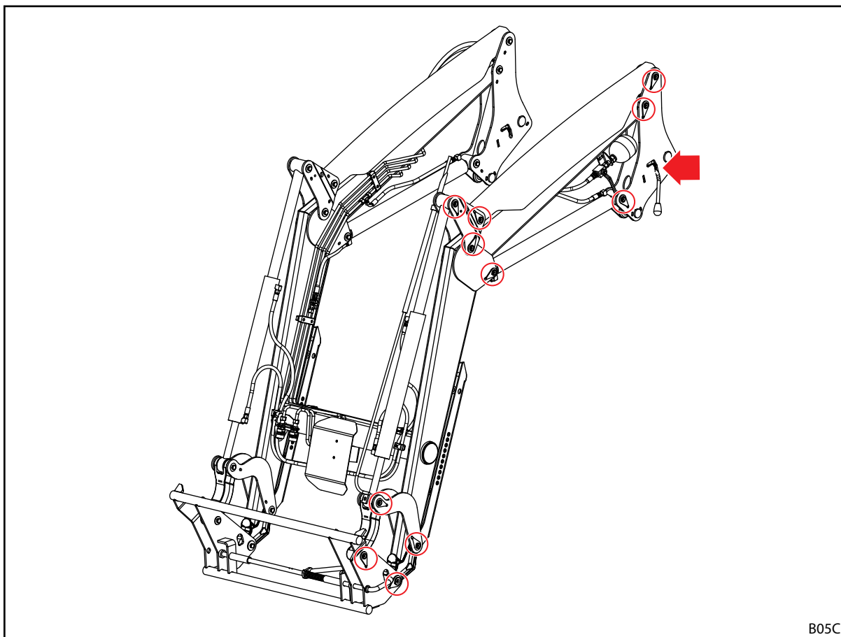
Sl. 110 Mazalna mesta pri tipu P
