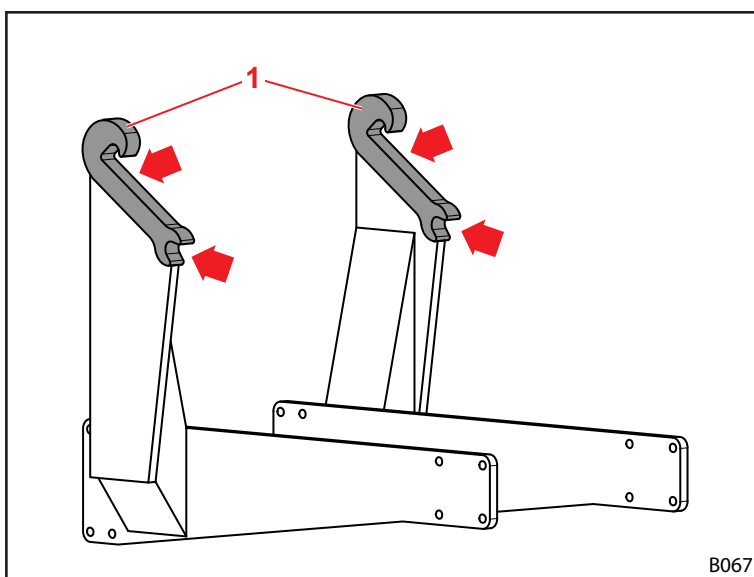
Sl. 108 Mazalna mesta na ležiščih čelnega nakladalnika
