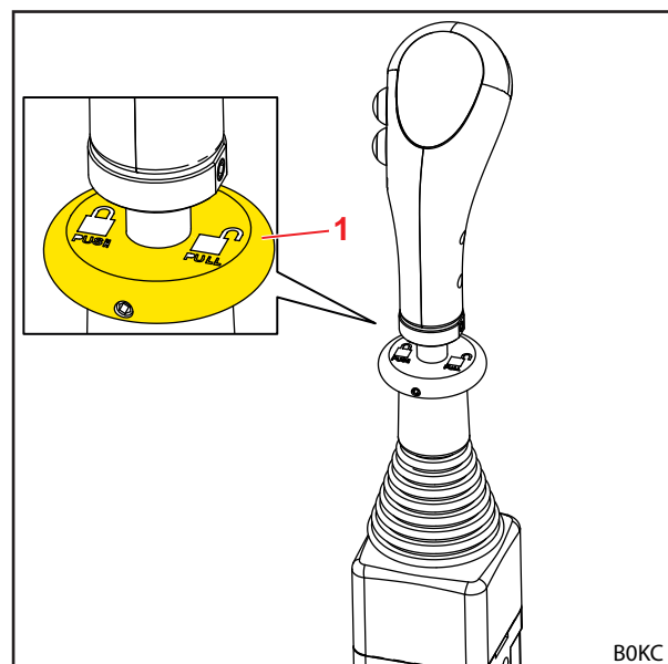
Sl. 61 Zaklepanje upravljalne ročice (navpični zaklep)
