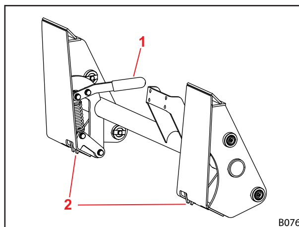
Sl. 80 Zaklep orodja na priklopnem okvirju Skid-Steer
