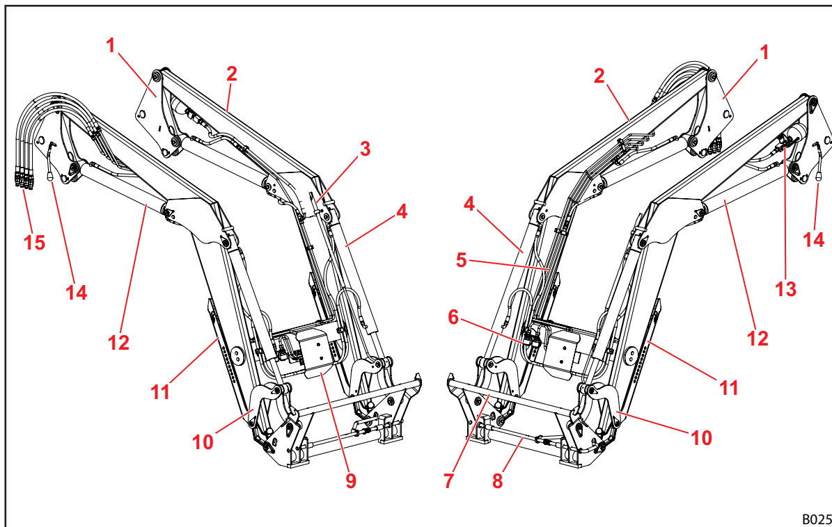
Sl. 9 Čelni nakladalnik H (brez mehanskega vzporednega vodenja)
