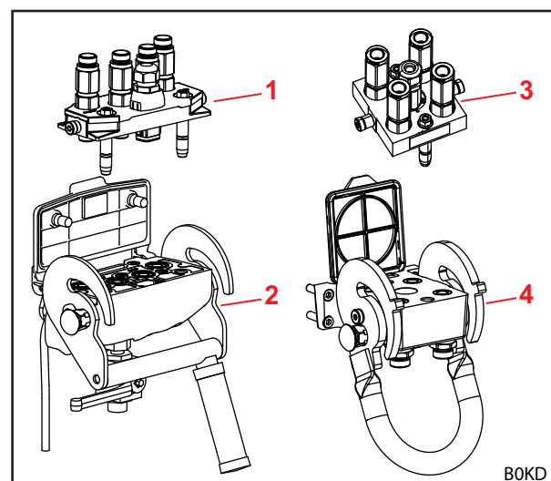
Sl. 23 Sestava spojke Hydro-Fix in večkratnih vtičev
