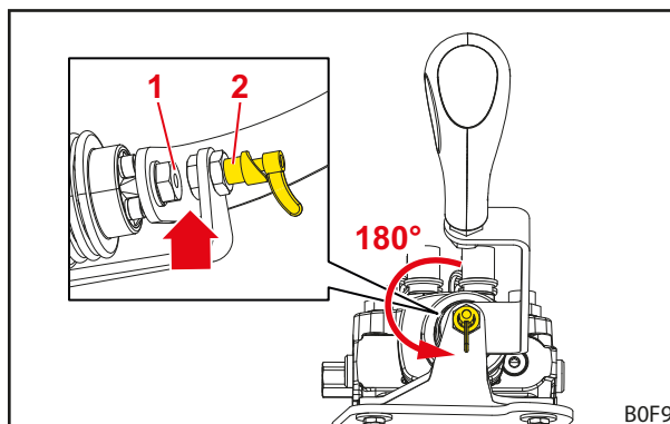
Sl. 72 Odklenjena upravljalna ročica
