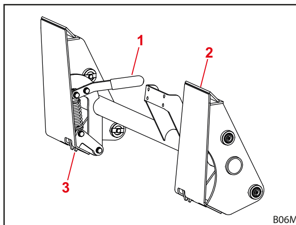
Sl. 27 Mehanski zaklep orodja pri priklopnih okvirjih Skid-Steer
