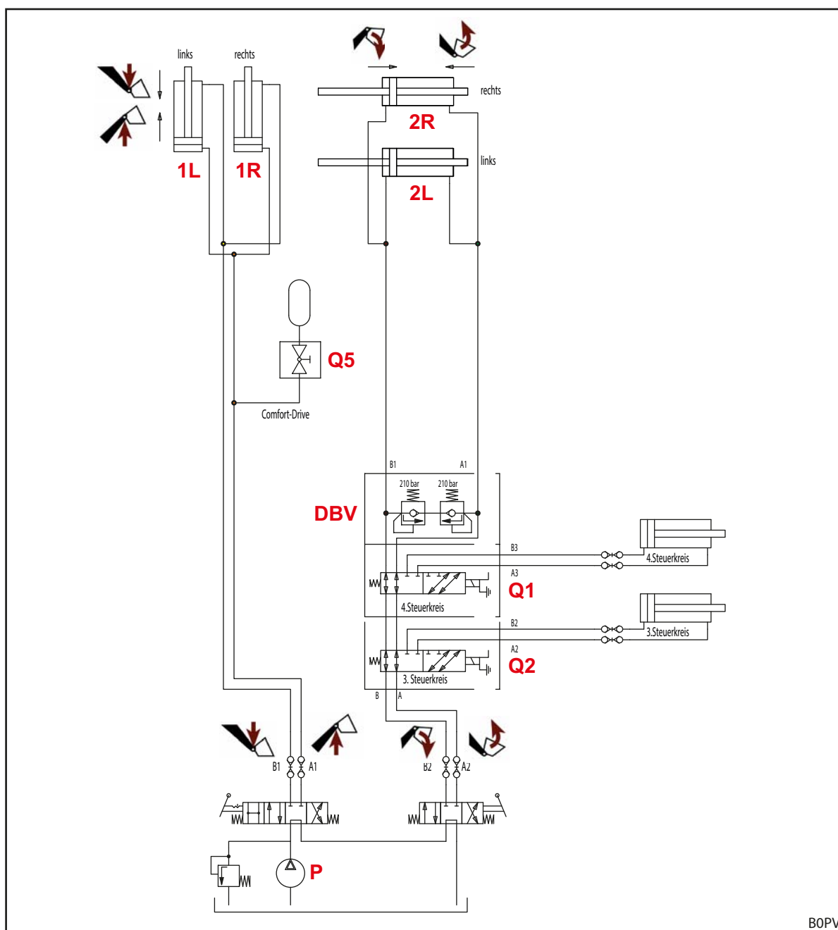
Sl. 127 Hidravlični načrt P
