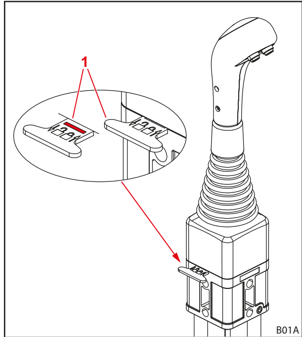
Fig. 67 Bloqueo de la palanca de mando (bloqueo horizontal)
