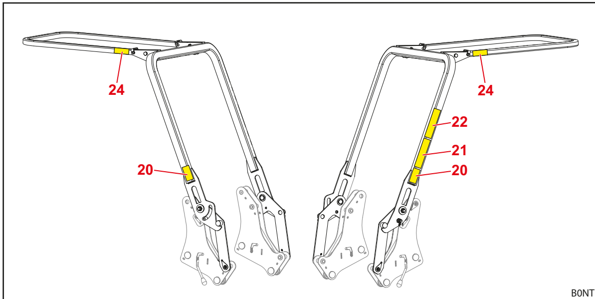
Fig. 8 OPG para tractores con equipo de protección antivuelco de 2 columnas colocado delante (ilustración de ejemplo)
