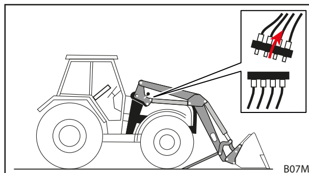
Fig. 124 Desacoplar la hidráulica
