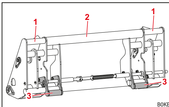
Fig. 17 Cuadro de cambio combinado Euro-SMS (preparado para implemento Euro)
