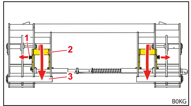
Fig. 89 Girar los apoyos hacia abajo
