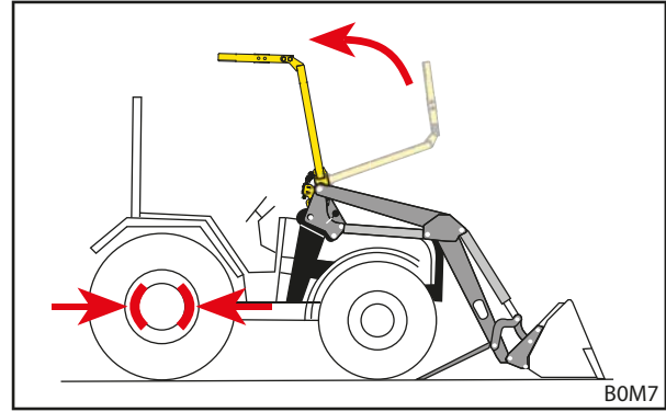
Fig. 56 Plegar el OPG hacia arriba
