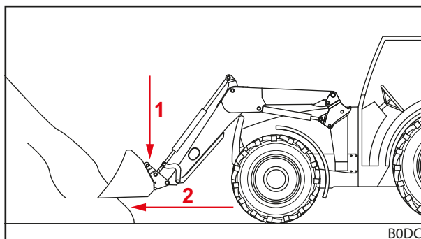
Fig. 111 Bajar el cargador frontal y entrar recto en la carga.
