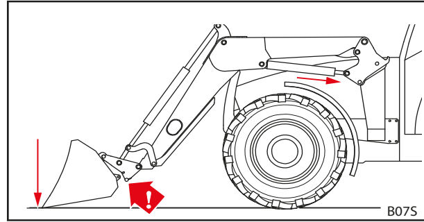
Fig. 88 Presionar el implemento contra el suelo
