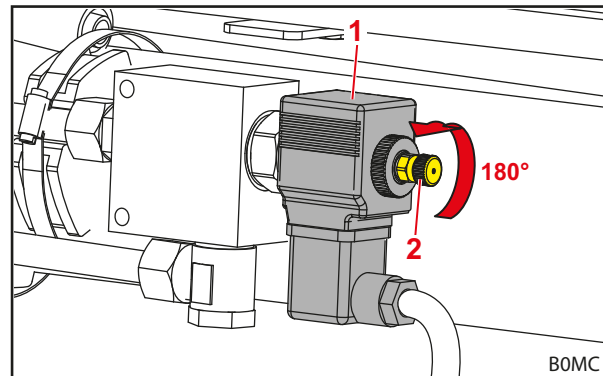
Fig. 35 Abrir válvula
