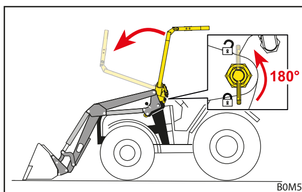
Fig. 36 Plegar hacia abajo el OPG
