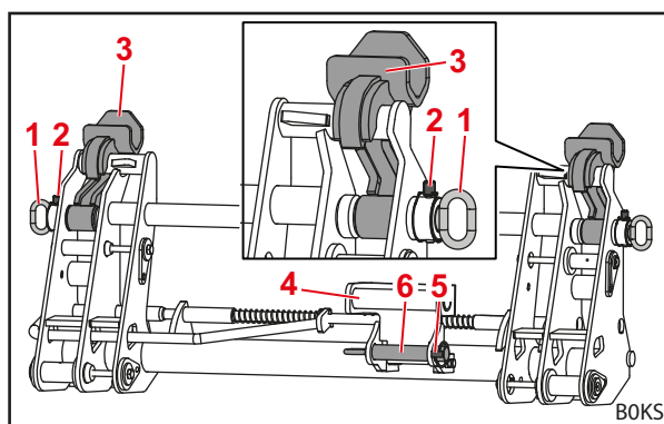
Fig. 94 Adaptador en posición de trabajo (cuadro de cambio preparado para implemento FR)
