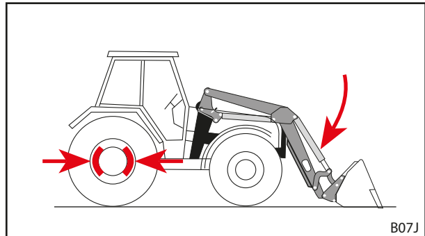
Fig. 121 Aplicar el freno de estacionamiento y bajar el cargador frontal
