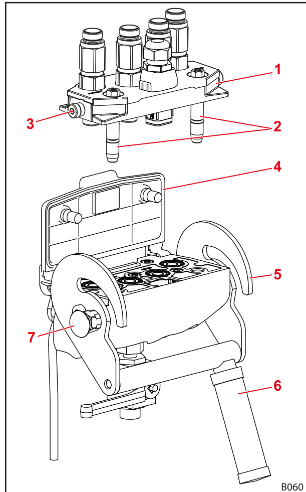
Fig. 81 Hydro-Fix (ejemplo: Hydro-Fix cuádruple)
