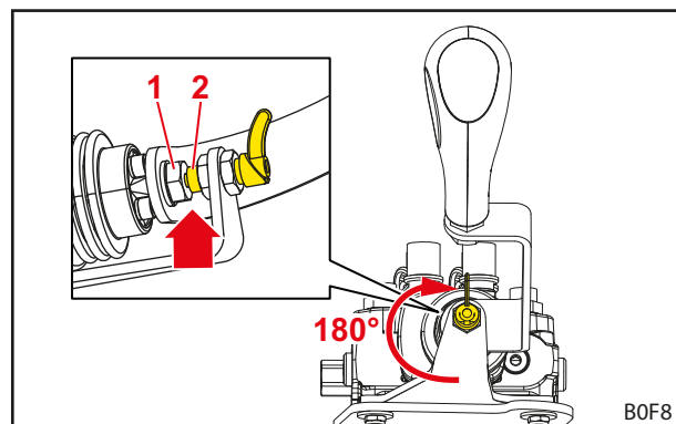
Fig. 71 Palanca de mando bloqueada
