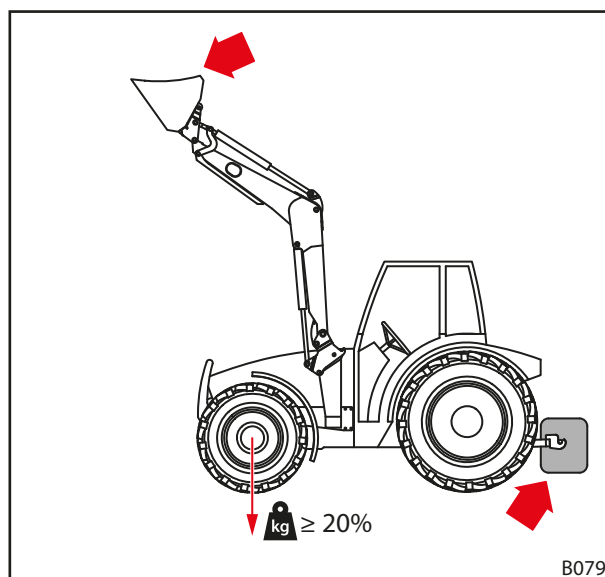
Fig. 51 Carga durante los desplazamientos por carretera
