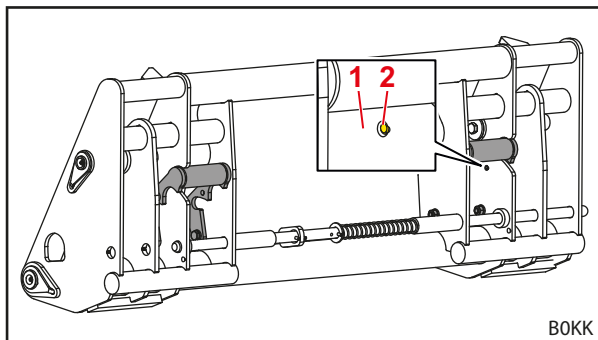
Fig. 92 Apoyos girados hacia arriba (vista posterior)
