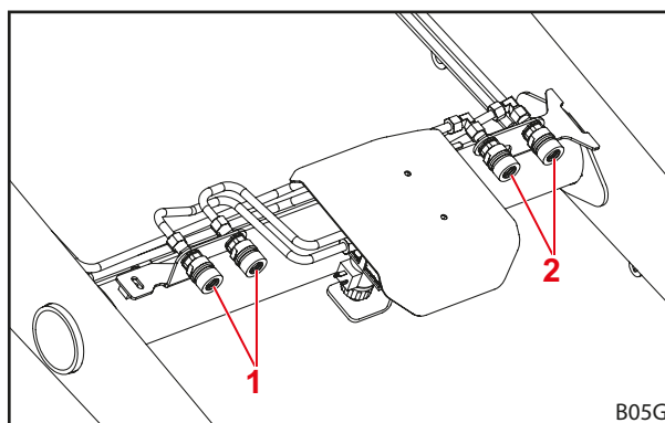
Fig. 46 4.º circuito de control adicional
