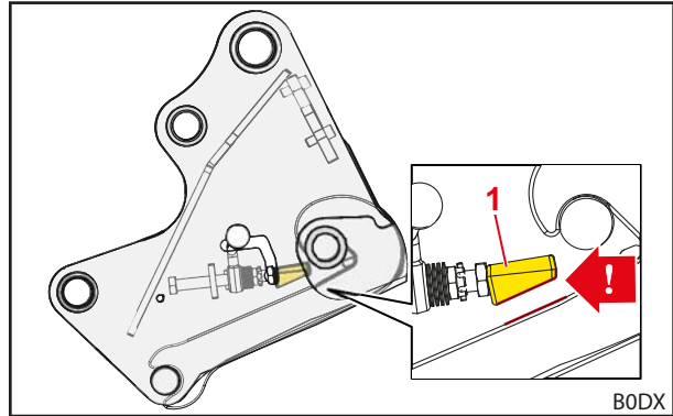
Fig. 59 Posición de montaje correcta de la cuña de apriete
