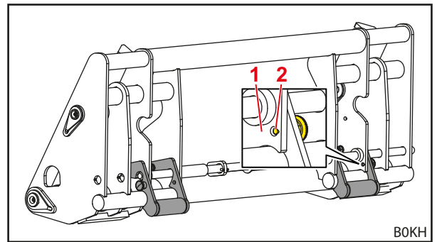
Fig. 90 Apoyos girados hacia abajo
