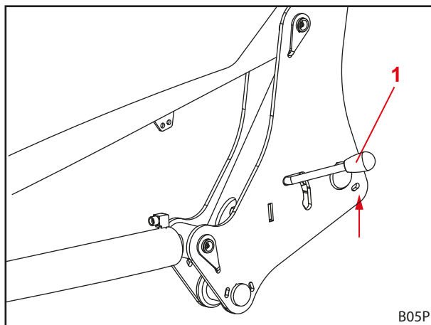
Fig. 119 Comprobar el bloqueo del cargador frontal
