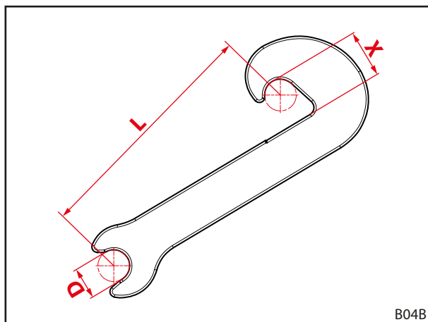
Fig. 118 Valores de desgaste del gancho de retenida
