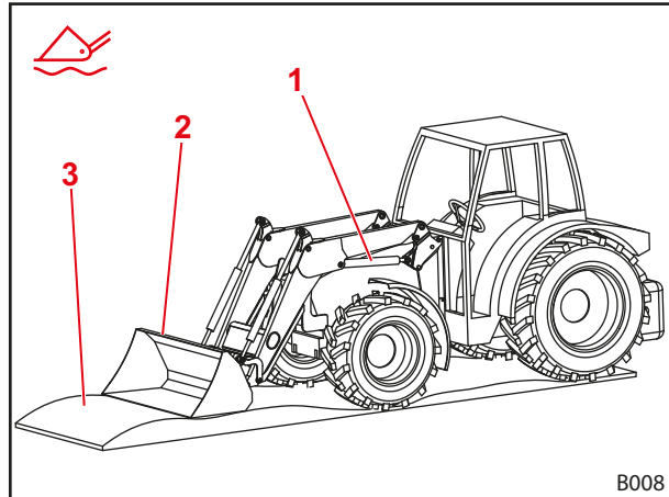
Fig. 32 Cargador frontal en posición flotante
