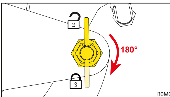
Fig. 39 Colocar el pasador de retención en posición bloqueada
