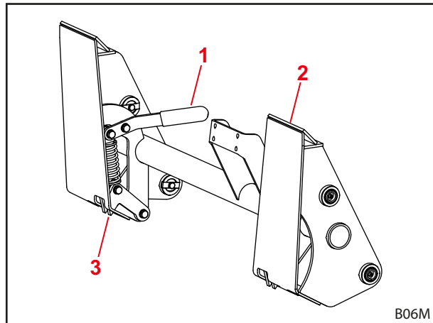
Fig. 27 Bloqueo mecánico del implemento en cuadros de cambio Skid-Steer
