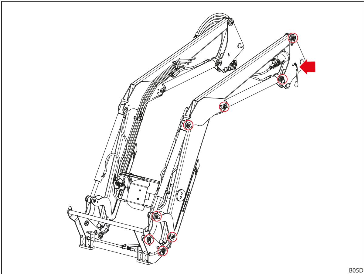
Fig. 116 Puntos de engrase H
