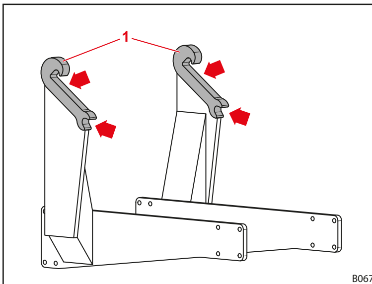
Fig. 115 Puntos de engrase de los alojamientos del cargador frontal
