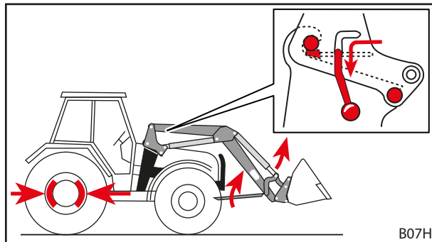
Fig. 58 Plegar los pies soporte y cerrar el bloqueo del cargador frontal
