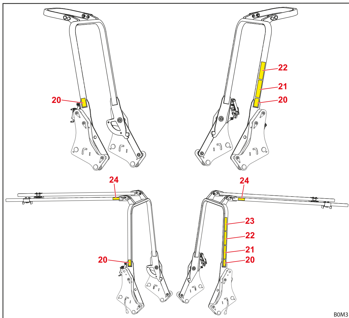
Fig. 7 OPG para tractores con equipo de protección antivuelco de 2 columnas colocado detrás (ilustración de ejemplo)
