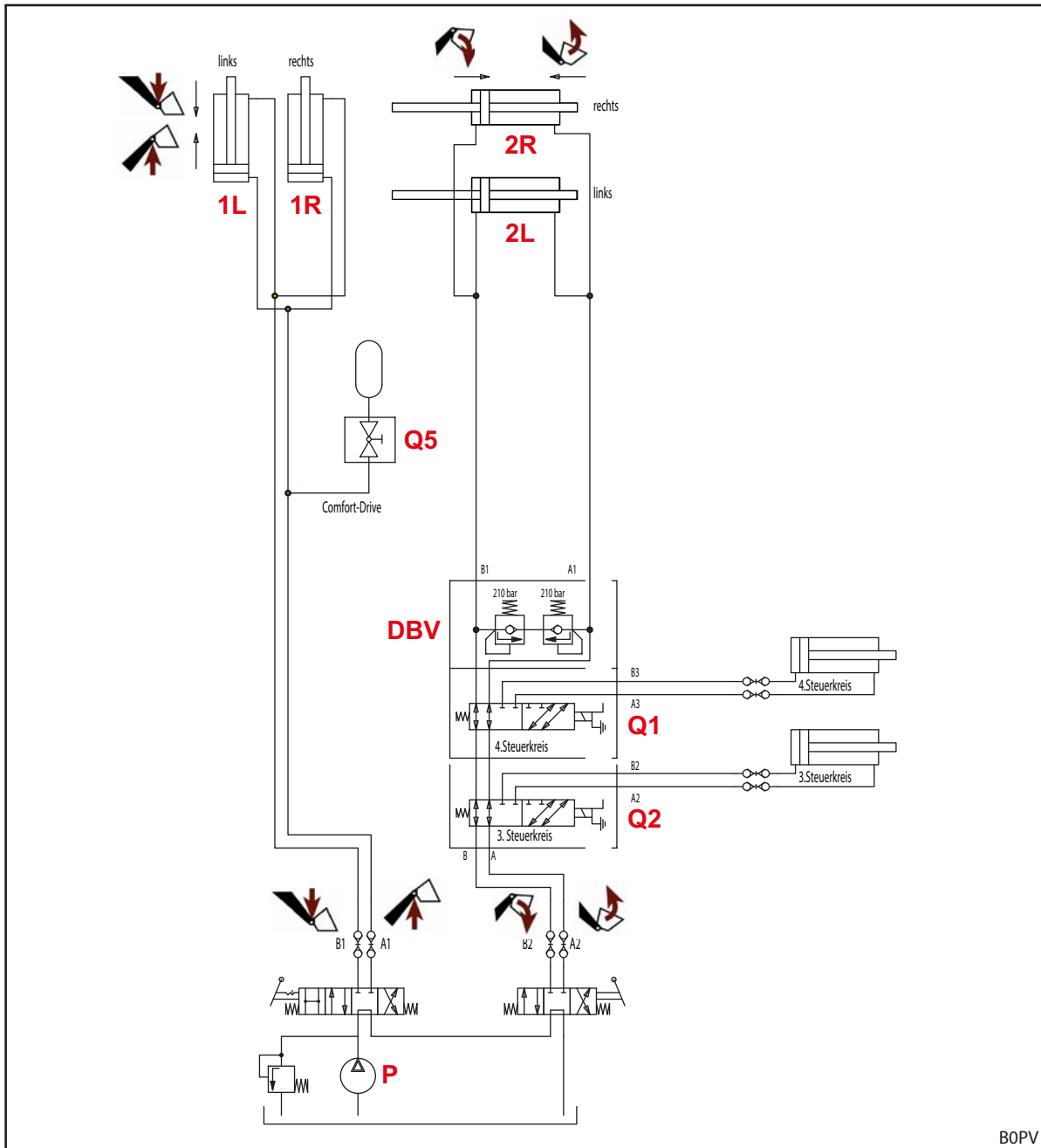
Fig. 127 Esquema hidráulico P
