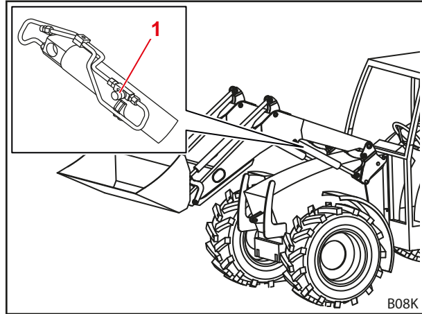
Fig. 48 Válvula de control de descenso
