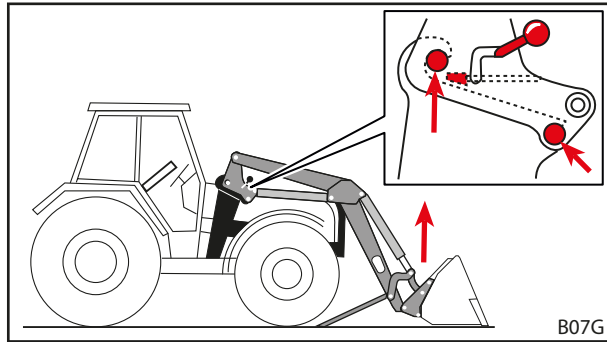
Fig. 57 Utilizar la función Elevar hasta que los bulones tengan contacto con el gancho de retenida
