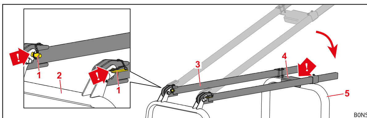
Fig. 42 Travesaños plegados hacia abajo y asegurados en los taladros superiores
