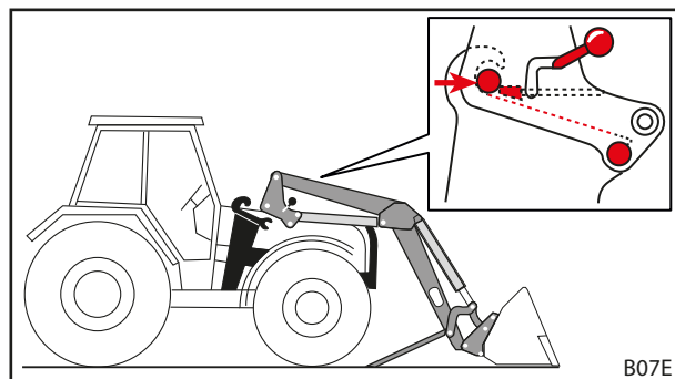
Fig. 54 Introducir el tractor en el brazo oscilante
