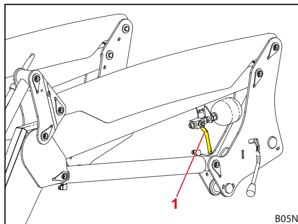
Fig. 47 Comfort-Drive accionado mecánicamente
