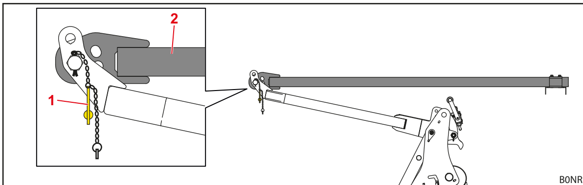
Fig. 41 Travesaños completamente plegados hacia abajo
