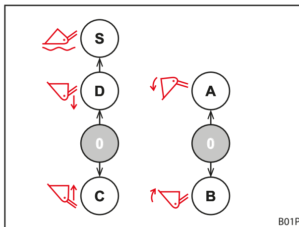
Fig. 65 Asignación con dos palancas de mando
