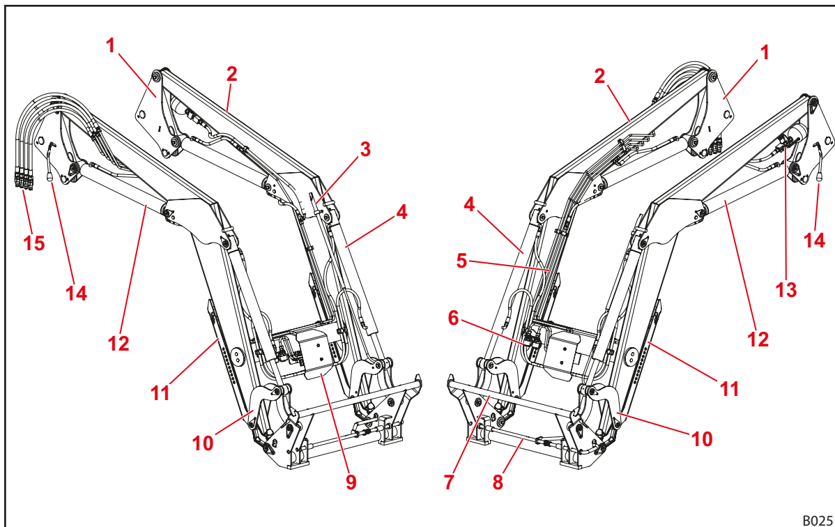
Fig. 10 Cargador frontal H (sin guía paralela mecánica)
