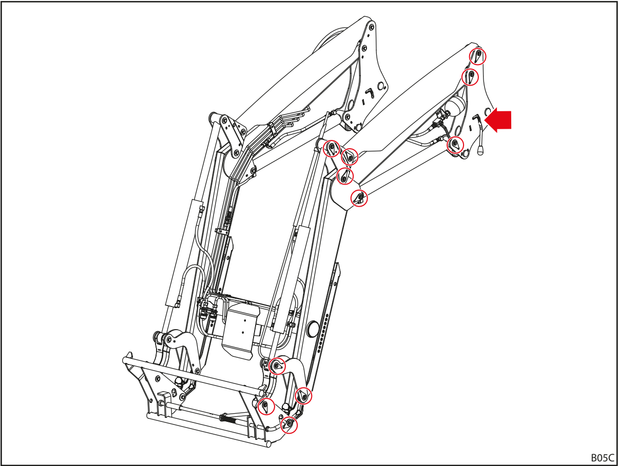
Fig. 117 Puntos de engrase P
