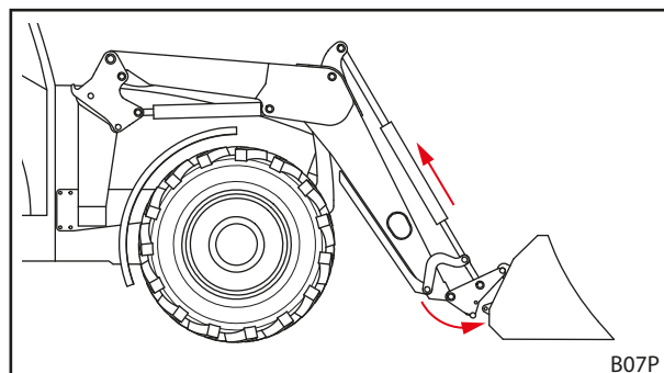
Fig. 98 Enganche
