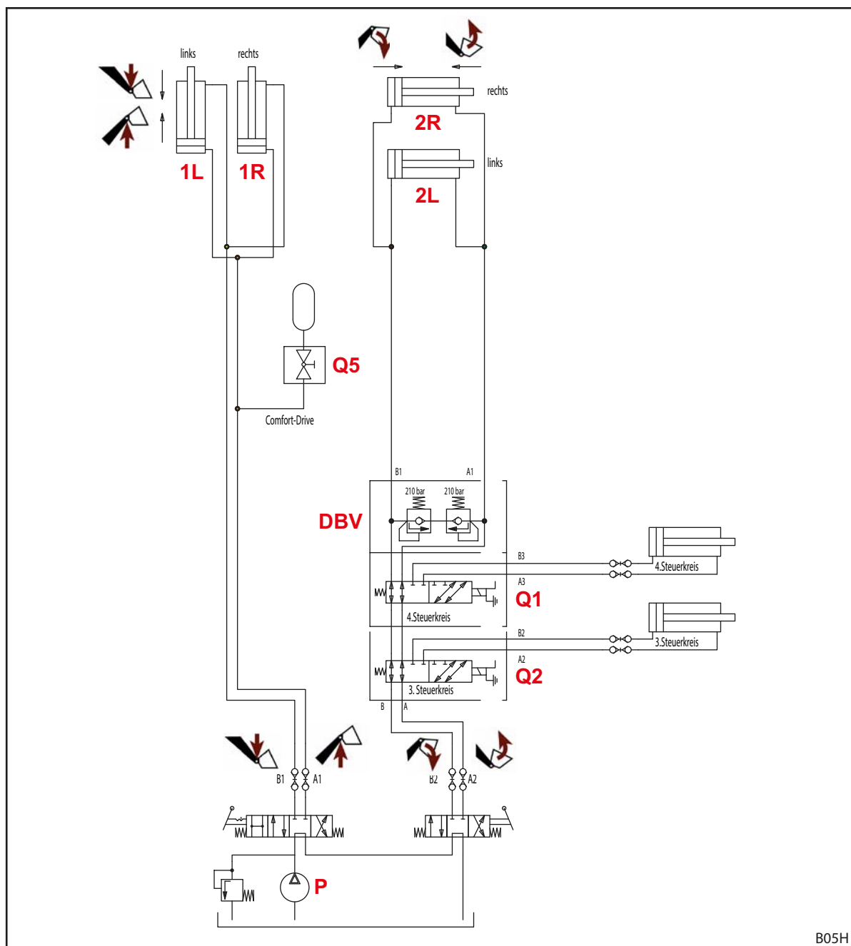
Fig. 126 Esquema hidráulico H
