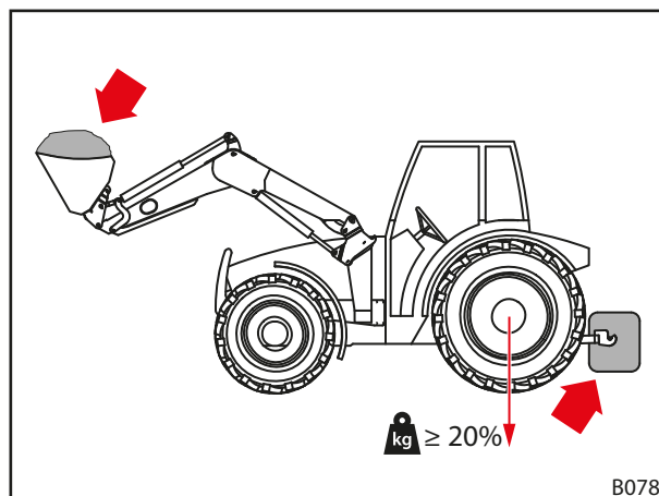
Fig. 50 Carga al trabajar con el cargador frontal
