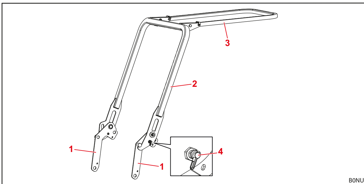
Fig. 13 Operator Protective Guard (OPG) para tractores con equipo de protección antivuelco de 2 columnas colocado delante (ilustración de ejemplo)
