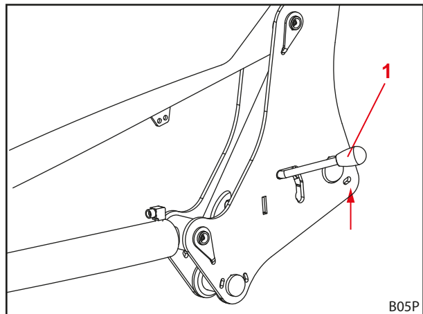
Fig. 60 Abrir el bloqueo del cargador frontal
