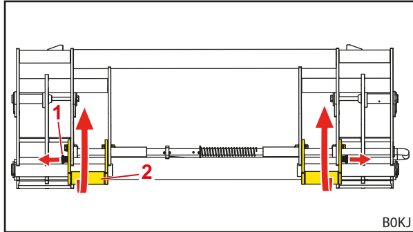
Fig. 91 Girar los apoyos hacia arriba
