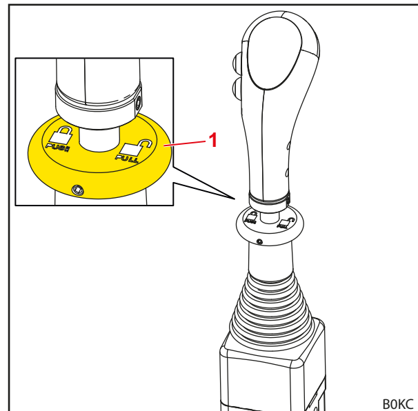
Fig. 68 Bloqueo de la palanca de mando (bloqueo vertical)
