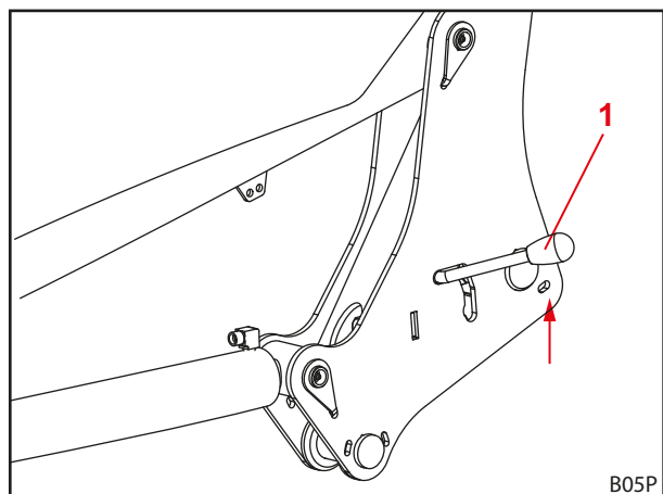
Fig. 42 Abrir el bloqueo del cargador frontal
