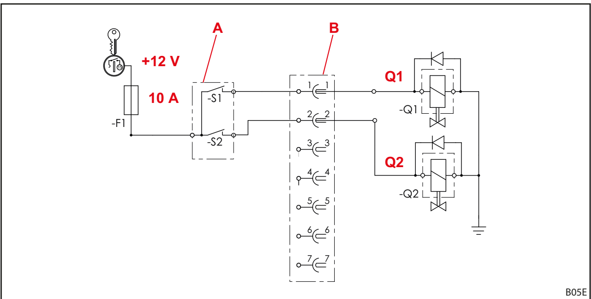
Fig. 98 Esquema eléctrico
