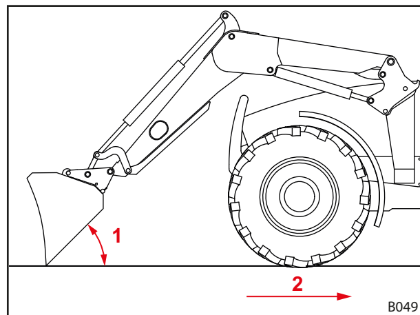
Fig. 80 Aplanamiento hacia atrás
