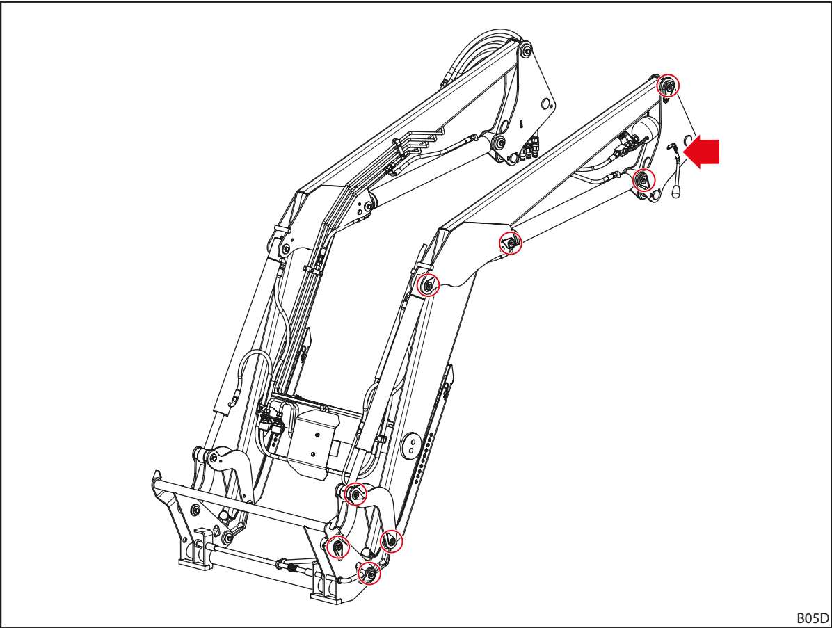
Fig. 87 Puntos de engrase H
