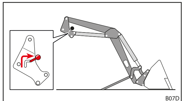
Fig. 36 Abrir el bloqueo del cargador frontal
