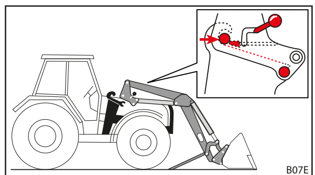
Fig. 37 Introducir el tractor en el brazo oscilante
