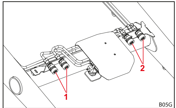
Fig. 29 4.º circuito de control adicional
