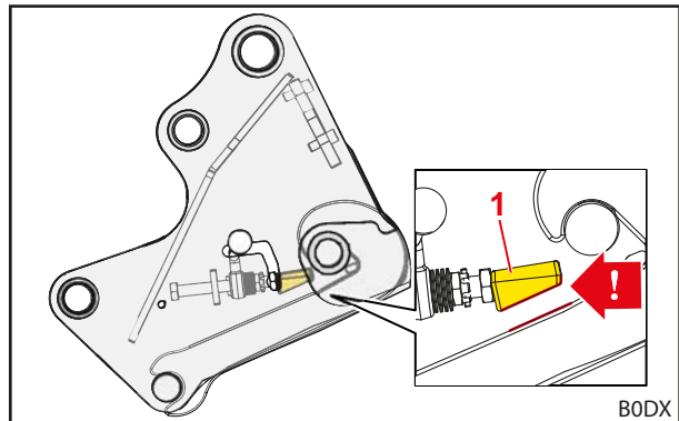
Fig. 41 Posición de montaje correcta de la cuña de apriete
