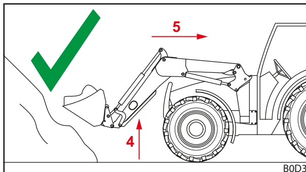
Fig. 85 Marcha atrás bajo carga – correcta
