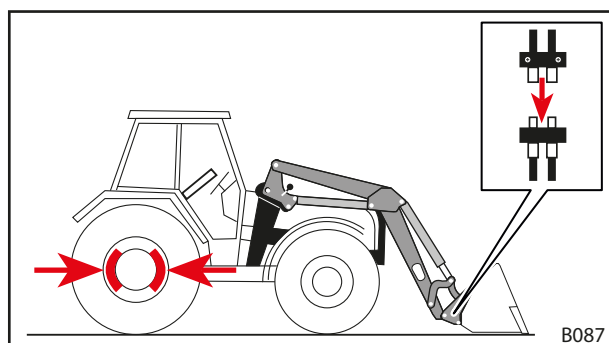
Fig. 71 Unir los conductos hidráulicos del implemento con acoplamientos del cargador frontal
