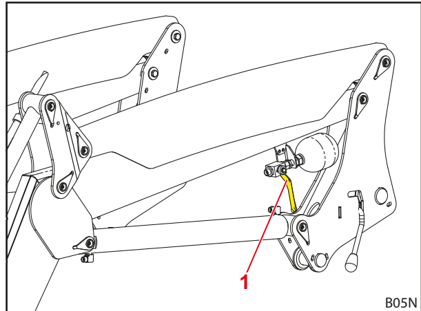
Fig. 30 Comfort-Drive con accionamiento manual
