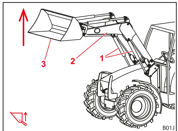
Fig. 21 Función Elevar
