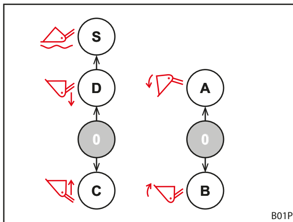
Fig. 47 Asignación con dos palancas de mando
