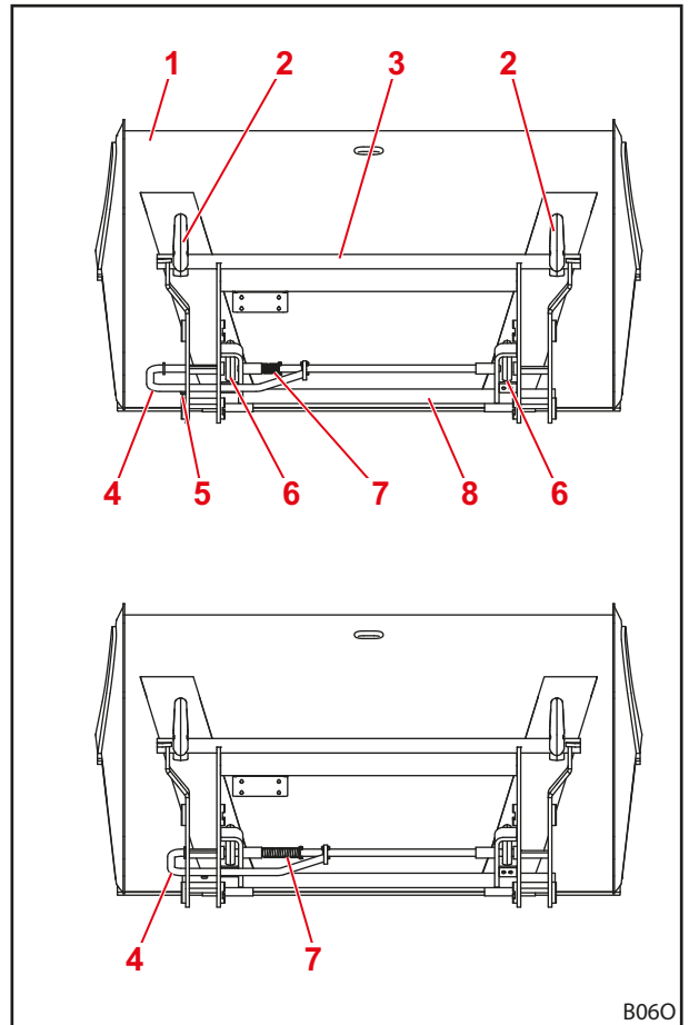
Fig. 19 Bloqueo abierto (arriba) y cerrado (abajo)
