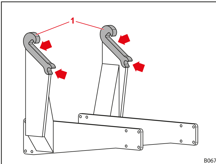
Fig. 86 Puntos de engrase de los alojamientos del cargador frontal
