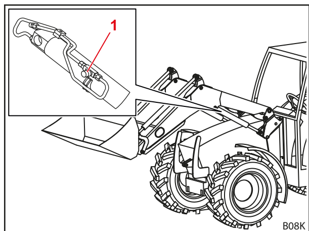
Fig. 31 Válvula de control de descenso
