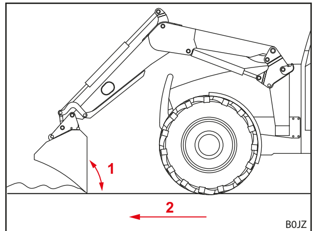
Fig. 81 Retirada
