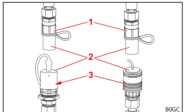
Fig. 56 Acoplamientos por enchufe (figuras de ejemplo)
