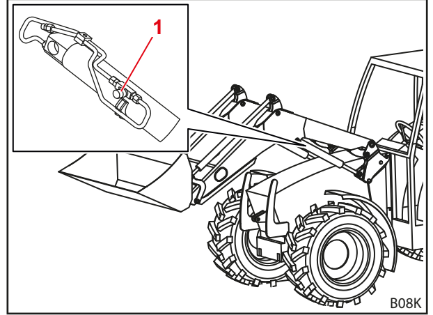
Şek. 42 İndirme kelebeği
