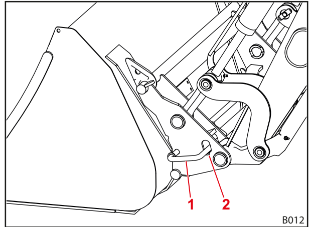
řek. 80 Mekanik alet kilidi
