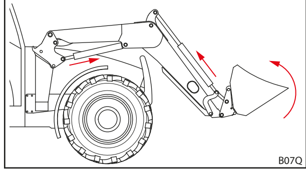
Şek. 96 Alet kilidinin çalıştırılması
