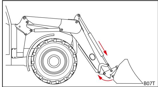
Şek. 106 Değiştirilebilir çerçevenin yerinden çıkartılması
