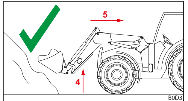
Şek. 112 Yük altında geri sürüş – doğru
