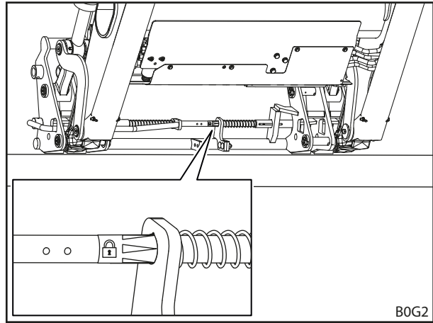
Şek. 82 Alet kilidinin etikete göre kontrol edilmesi (kombine değiştirilebilir çerçeve Euro-FR)
