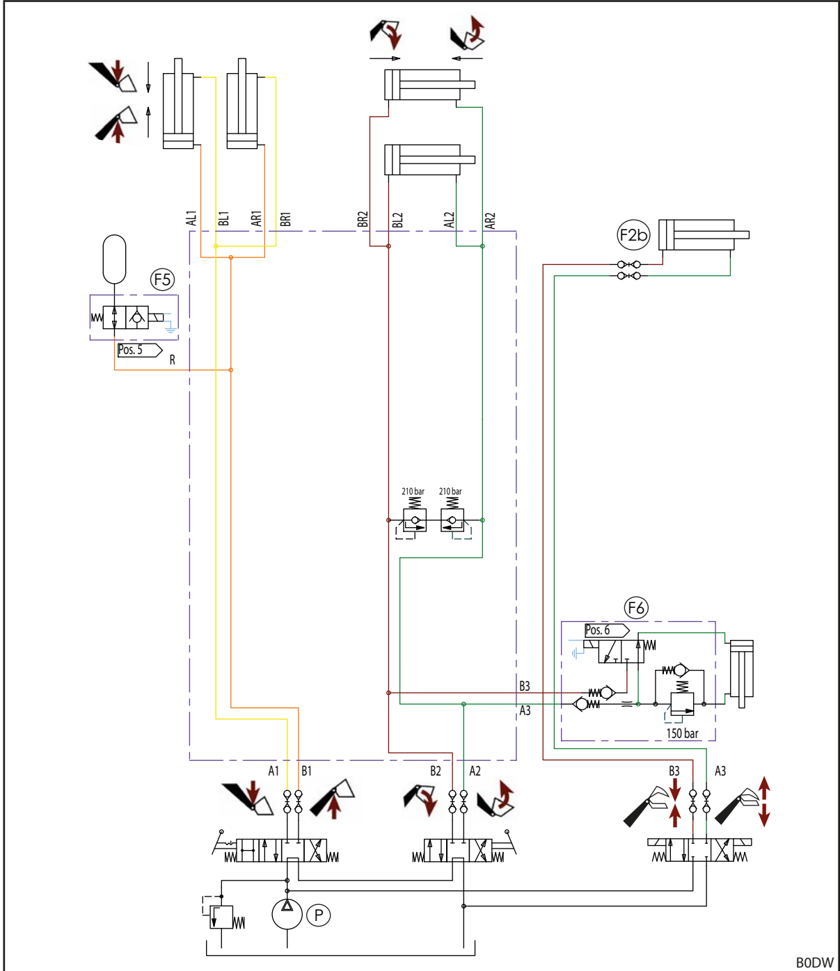
Şek. 128 FS hidrolik planı (REAL 3 ile donatılmışsa)
