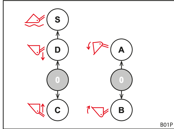
Şek. 63 2 kontrol kolunda fonksiyonlar
