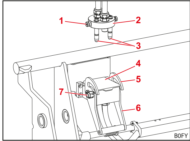
Şek. 78 Ayrılmış alet sabitleyicisi
