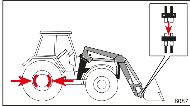
Şek. 97 Aletin hidrolik hatlarının ön yükleyicinin kaplinlerine bağlanması
