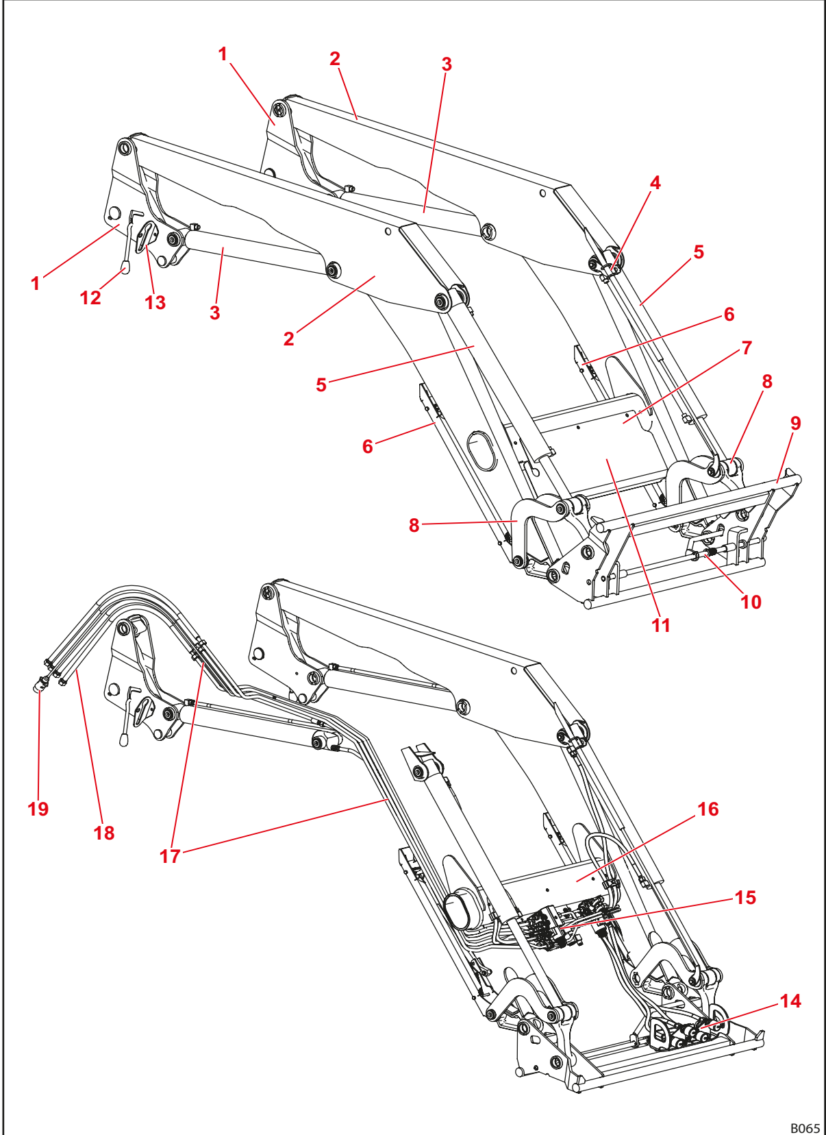
Şek. 7 Ön yükleyci FS
