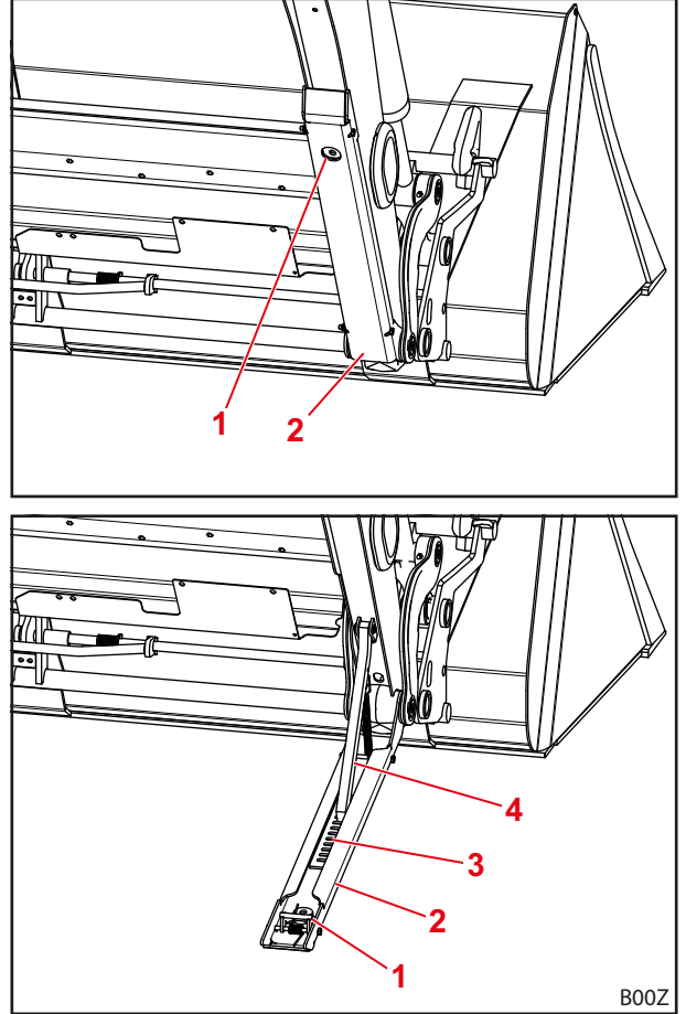
Şek. 74 Park desteği
