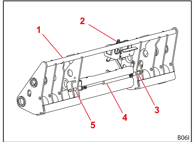
Şek. 16 Kuvvetlendirilmiř Euro deęiřtirilebilir ereve (FZ 100)
