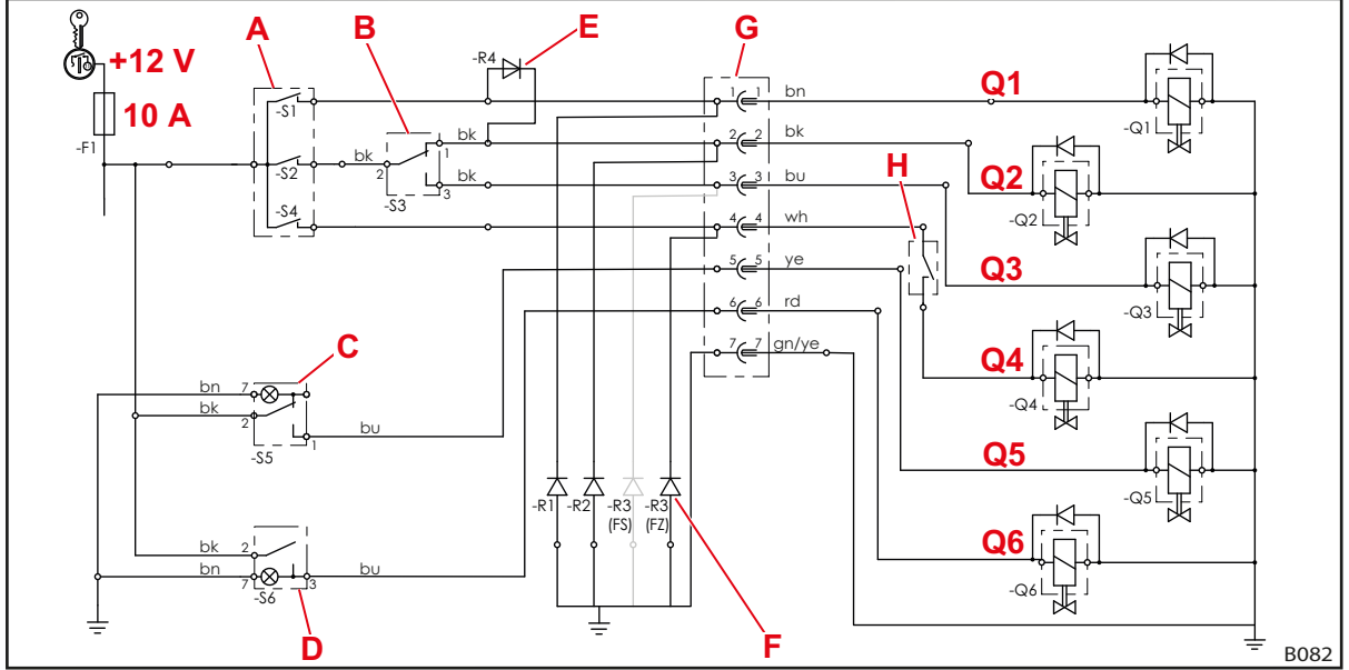
Şek. 131 Elektrik devre şeması (3. ve 4. kontrol devresi ile donatılmışsa)
