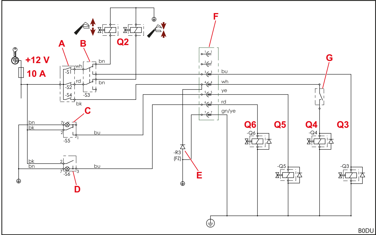
Şek. 132 Elektrik devre şeması (REAL 3 ile donatılmışsa)
