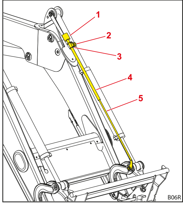
Şek. 36 Ekrandaki Return-To-Level sensörü
