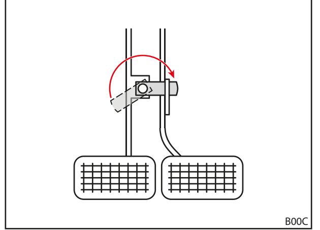
Şek. 43 Fren pedallarının birbirine bağlanması
