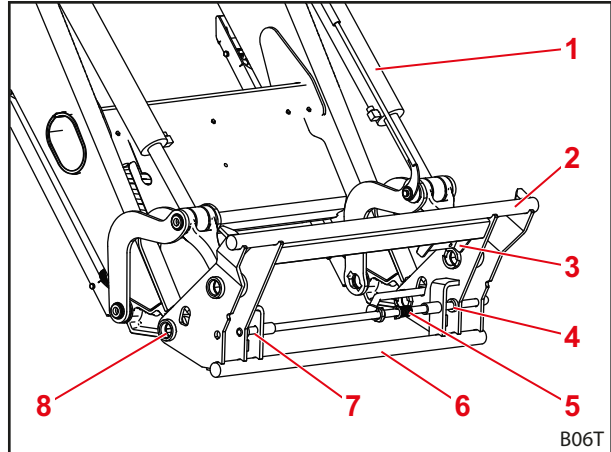
řek. 10 Euro deęiřtirilebilir ereve
