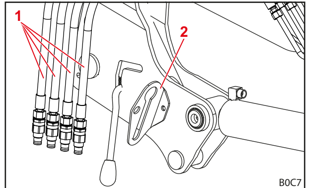
Şek. 126 Hidrolik hatlarını kaplin tutucusuna takma (resimde plug-in kaplin gösterilmektedir)
