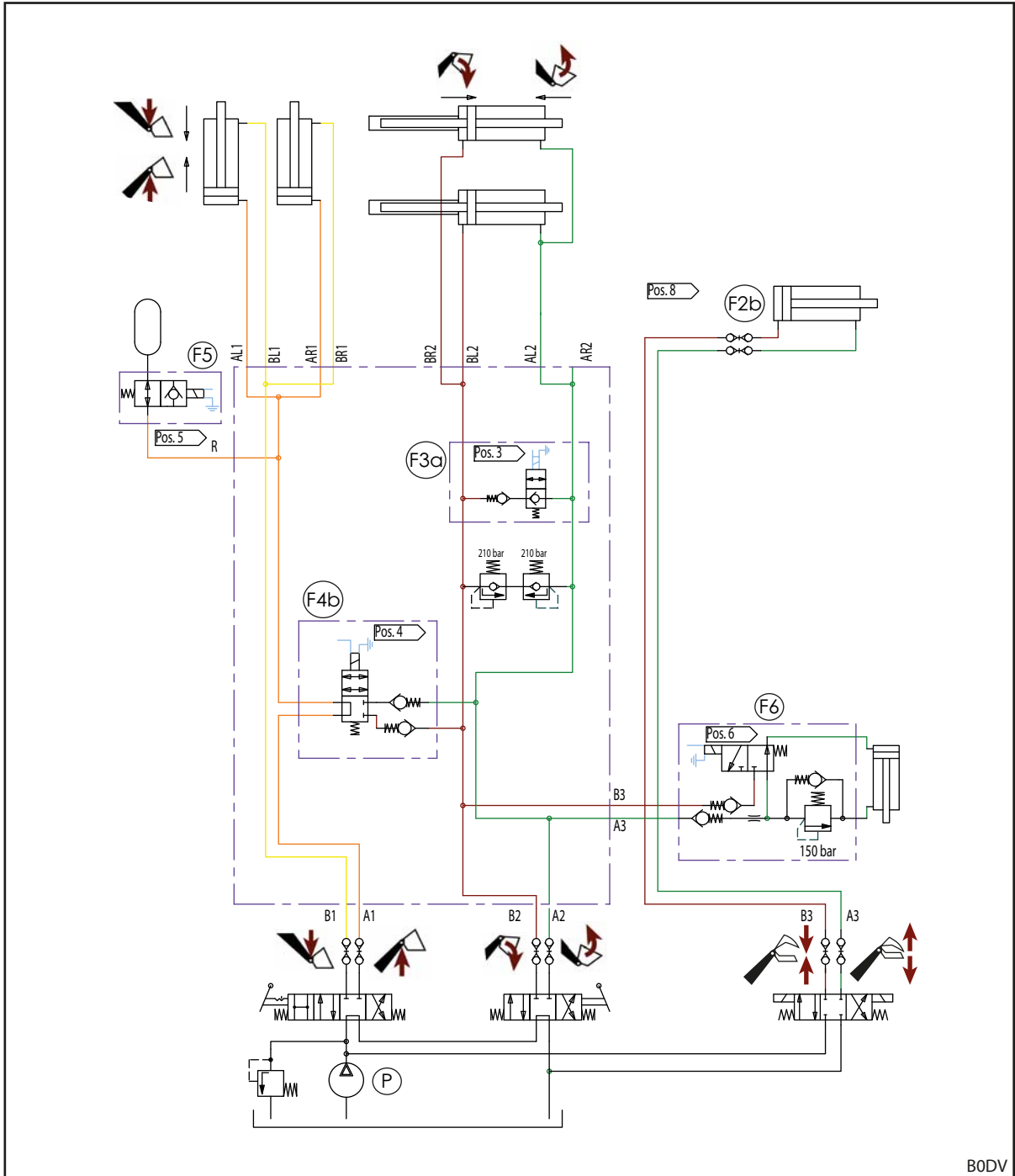
Şek. 130 FZ ve FZ-L hidrolik planı (REAL 3 ile donatılmışsa)
