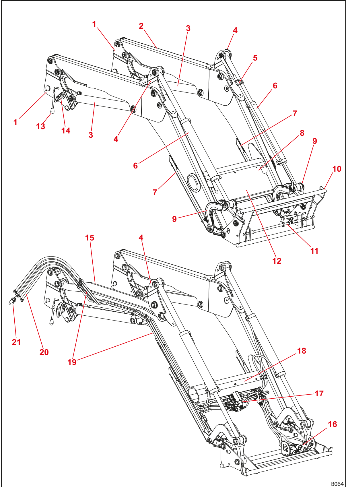
Şek. 8 Ön Yükleyci FZ
