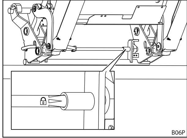
Şek. 81 Alet kilidinin etikete göre kontrol edilmesi
