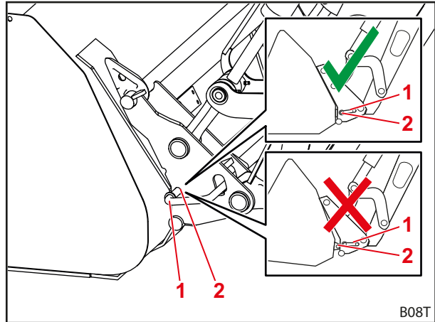
Şek. 83 Kilit civatalarının pozisyonunun kontrol edilmesi
