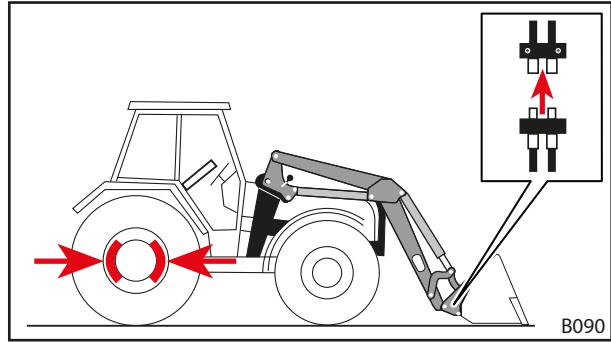
Şek. 105 Hidrolik hatlarının çözülmesi
