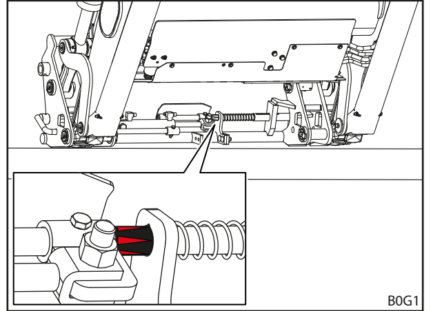
Şek. 88 Alet kilidinin etikete göre kontrol edilmesi
