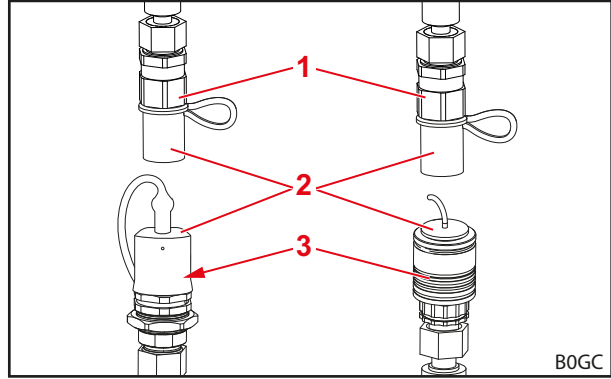
Şek. 75 Plug-in kaplinler (örnek resimler)
