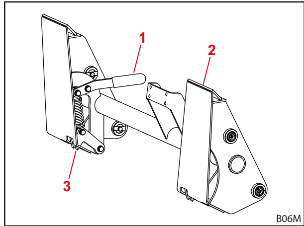
Şek. 26 Skid-Steer değişirilebilir çerçeveler üzerindeki mekanik alet kilidi
