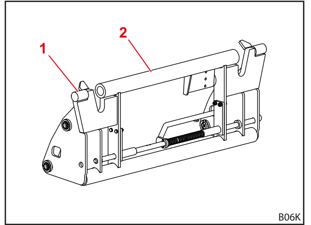
Şek. 12 Euro-SMS kombine değiştirilebilir çerçeve
