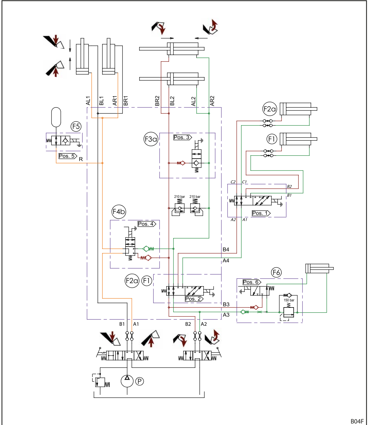
Şek. 129 FZ ve FZ-L hidrolik planı (3. ve 4. kontrol devresi ile donatılmışsa)
