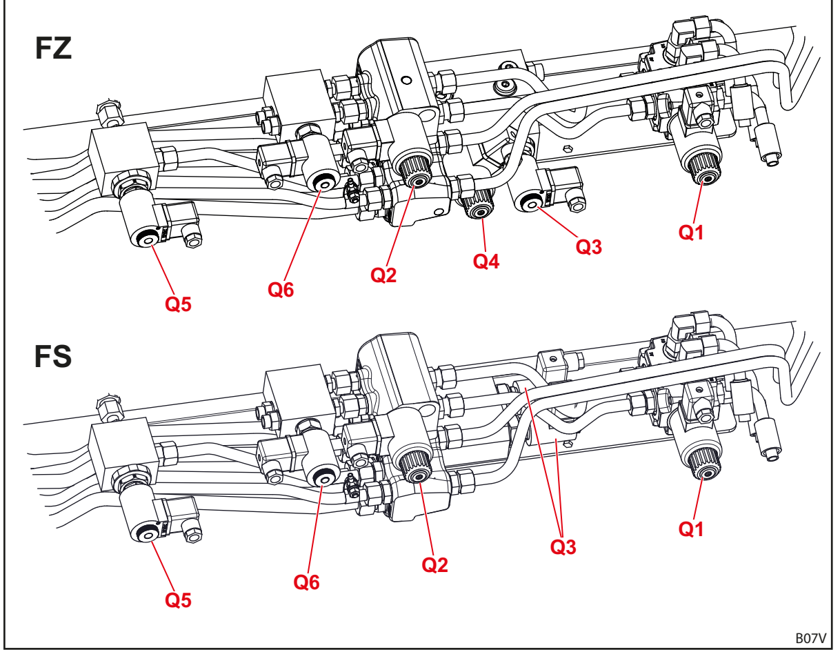
Şek. 133 Ek fonksiyonlar için hidrolik vana düzeni
