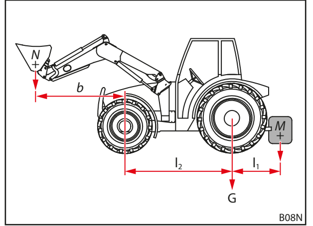
Şek. 46 Statik duruş emniyeti hesaplaması
