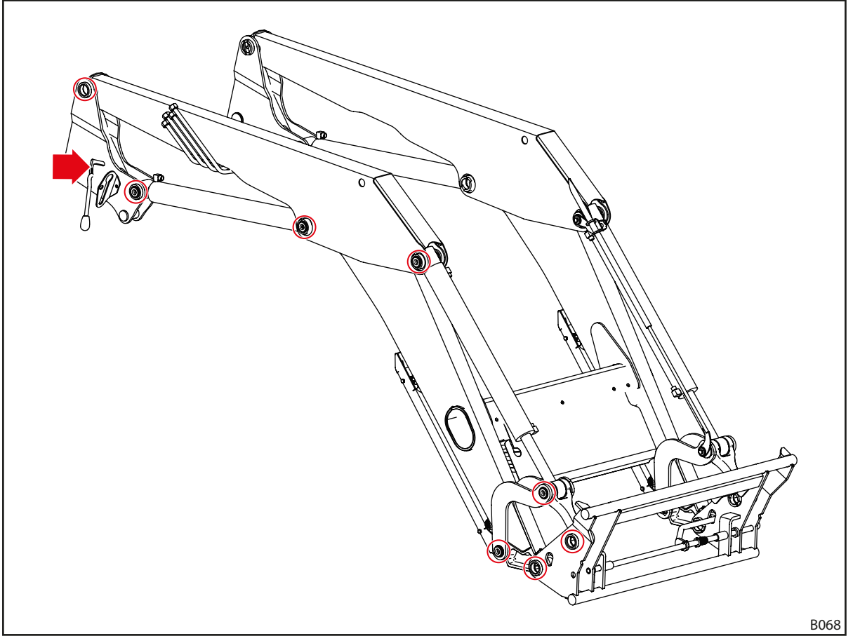
Şek. 114 Yağlama noktaları FS
