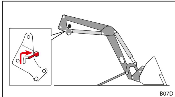
Şek. 47 Ön yükleyici kilidinin açılması
