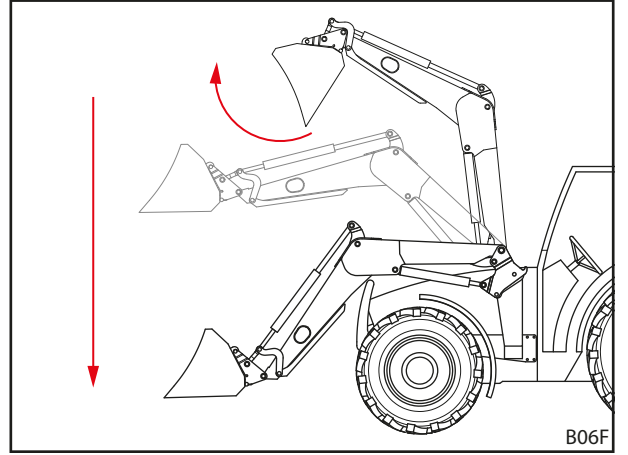
Şek. 35 Return-To-Level fonksiyonu
