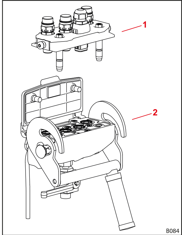
Şek. 22 Hydro-Fix'in yapısı
