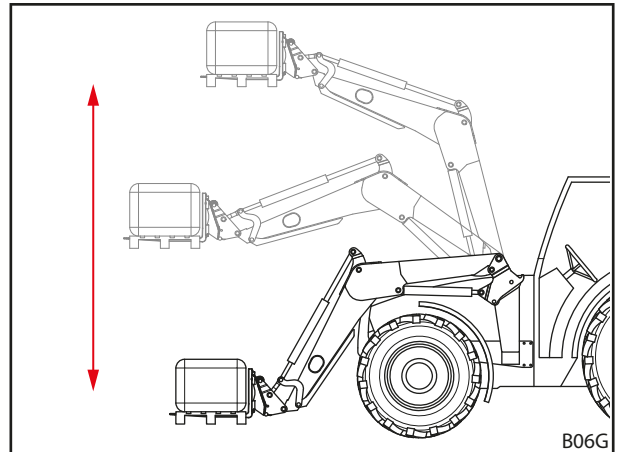
Şek. 33 Paralel kılavuz
