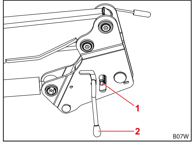
Şek. 118 Ön yükleyici kilidinin kontrolü
