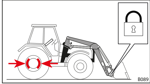
Şek. 101 Alet kilidinin kapatılması
