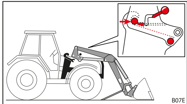
Şek. 48 Traktörün kanadın içine sürülmesi
