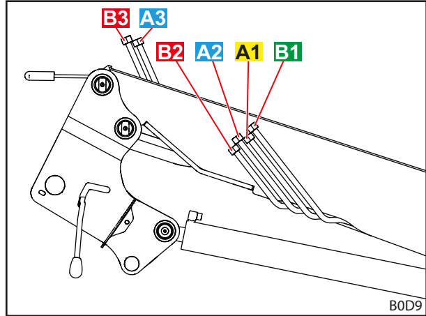
Şek. 18 Hidrolik hatları (opsiyonel REAL 3 )
