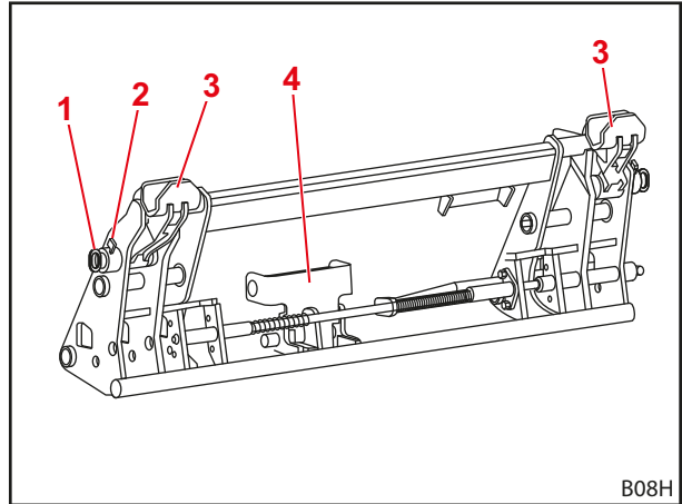
Şek. 14 Euro-FR kombine deęiřtirilebilir çerçeve
