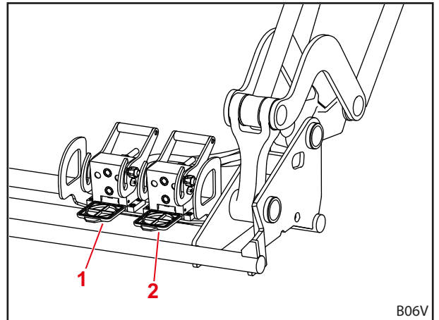
Şek. 38 Ek 4. kontrol devresi
