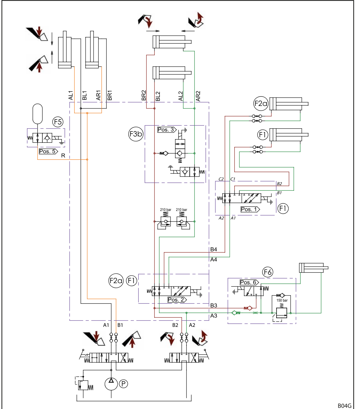
Şek. 127 FS ve FS hızlı travers hidrolik planı (3. ve 4. kontrol devresi ile donatılmışsa)
