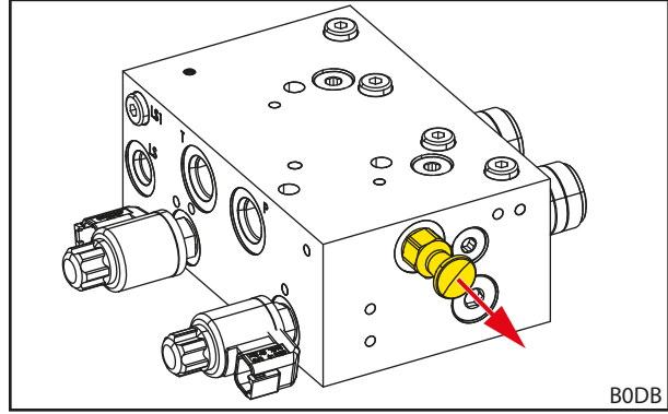
Şek. 72 REAL 3 valfindeki basınç boşaltma valfinin dışarı çekilmesi
