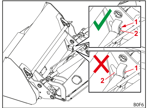
Şek. 90 Kilit civatalarının pozisyonunun kontrol edilmesi
