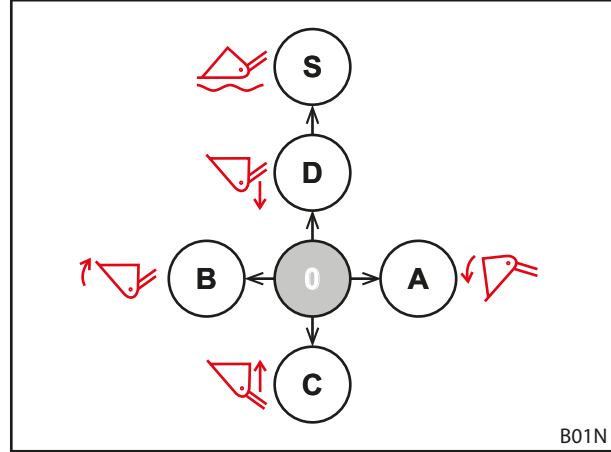
Şek. 62 Tek kontrol kolunda fonksiyonlar
