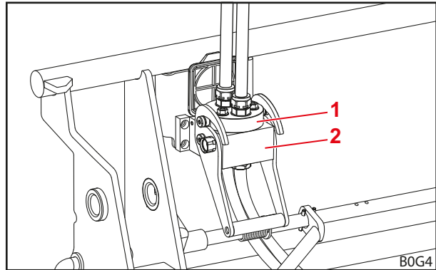
Şek. 79 Takılı alet sabitleyicisi
