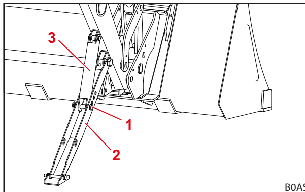
Obr. 52 Odstavná podpěra vyklopená
