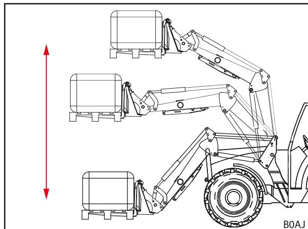
Obr. 29 Paralelní vedení
