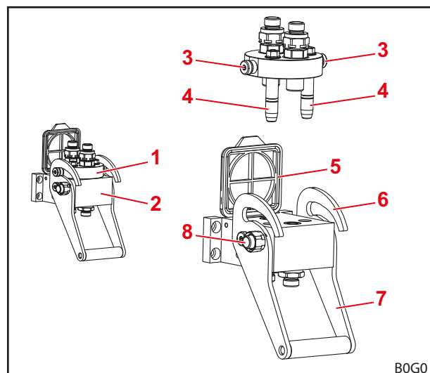
Obr. 19 Konstrukce nástroj-Fix
