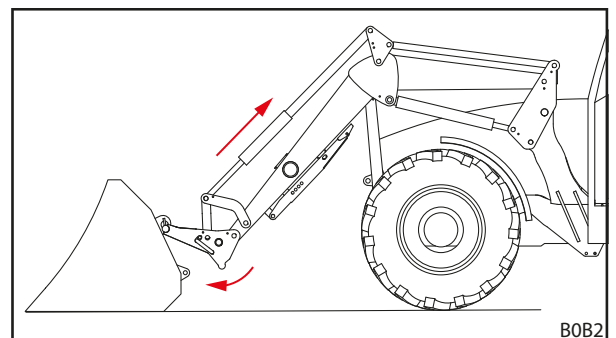
Obr. 75 Zaháknutí
