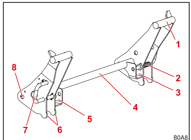
Obr. 22 Výměnný rám Euro
