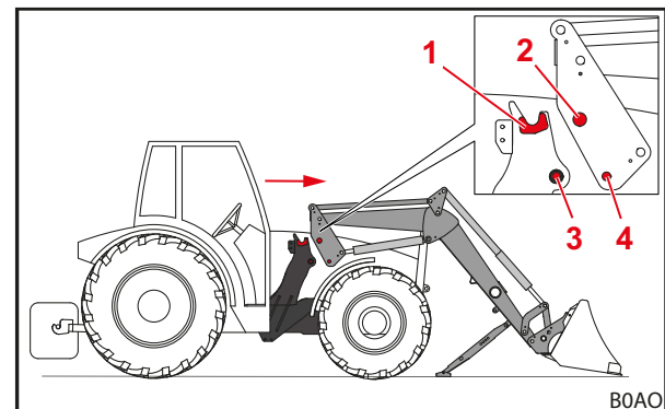
Obr. 38 Zajetí traktorem do výložníku
