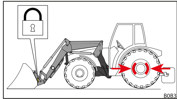
Obr. 76 Uzavření zamykacího mechanismu nářadí
