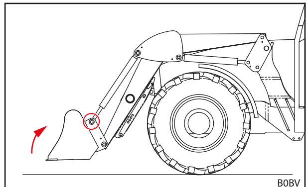
Obr. 80 Připojení nářadí nahoře k hydraulickým válcům
