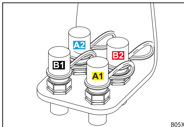
Obr. 14 Zástrčky rychlospojek na připojovaném dílu
