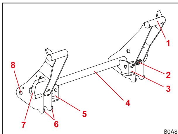
Obr. 64 Zamykací mechanismus nářadí na výměnných rámech Euro
