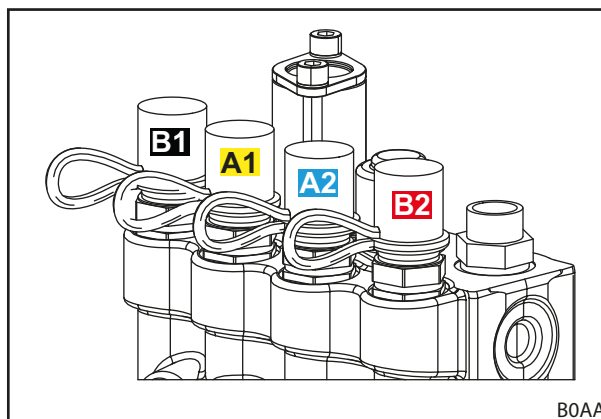
Obr. 15 Zástrčky rychlospojek přímo na hydraulickém ventilu
