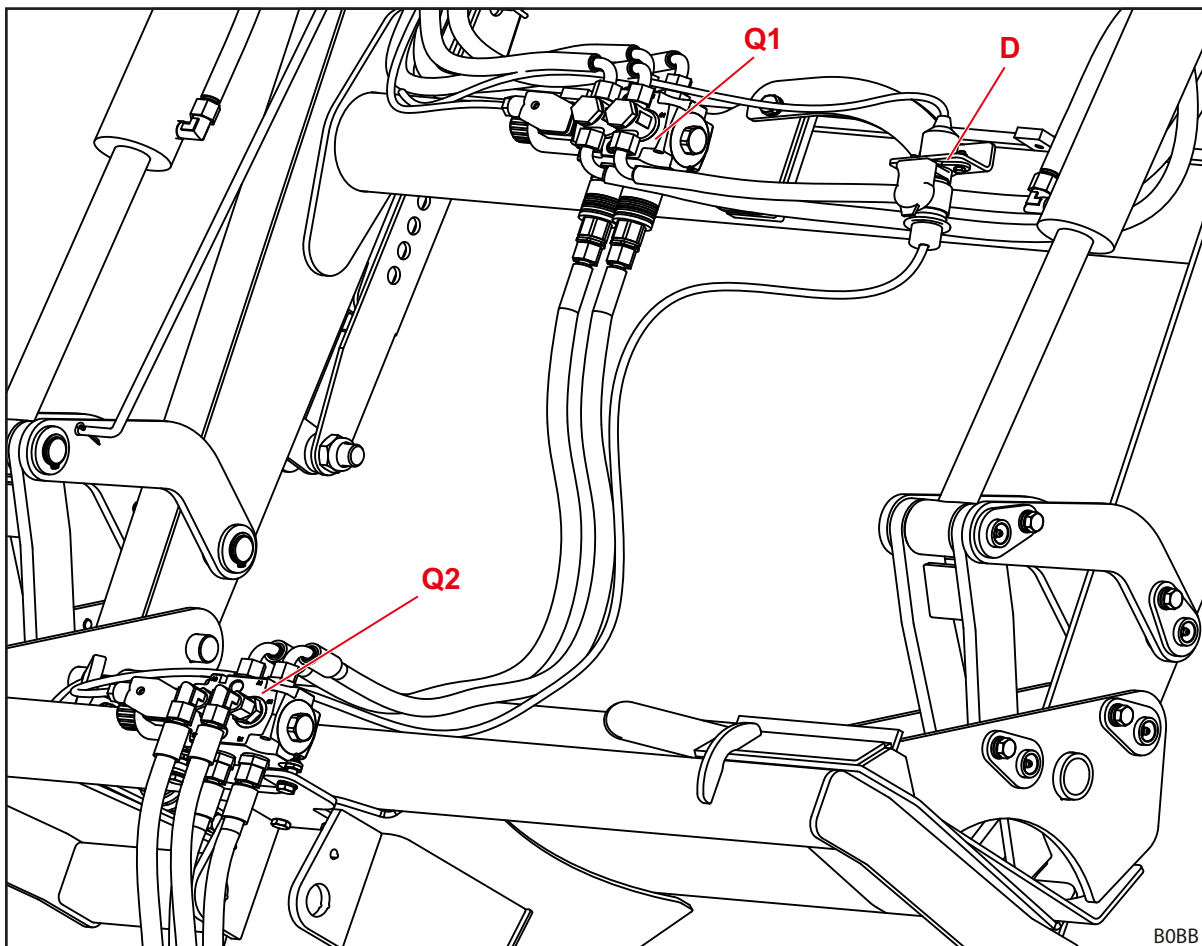
Obr. 107 Přiřazení hydraulických ventilů pro doplňkové funkce
