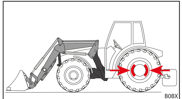
Obr. 83 Nastavte nářadí do polohy k odložení a zatáhněte parkovací brzdu
