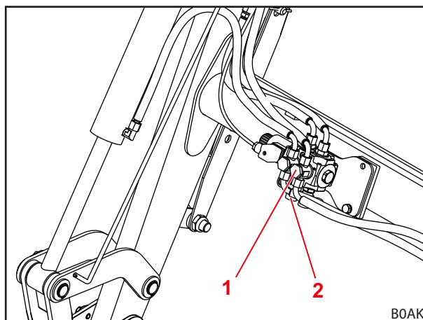
Obr. 30 Přídavný 3. řídicí okruh
