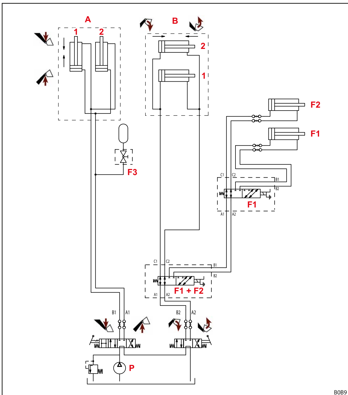
Obr. 105 Hydraulické schéma FC
