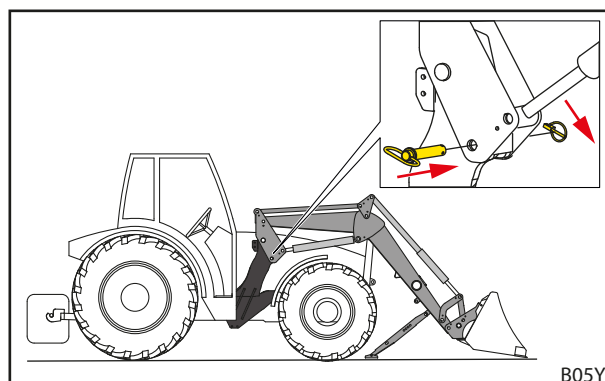
Obr. 40 Zasuňte oba zamykací čepy a zajistěte je sklopnou závlačkou
