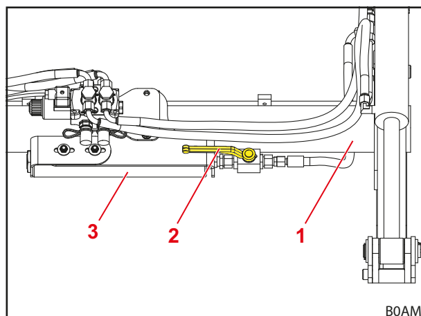
Obr. 32 Ručně ovládaný systém Comfort Drive (poloha páky Comfort-Drive)
