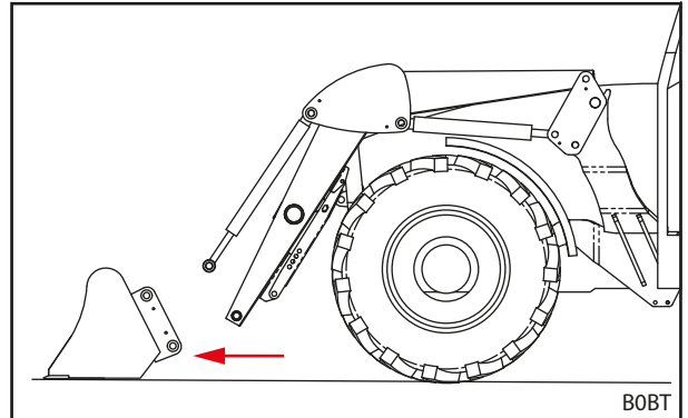
Obr. 78 Najetí
