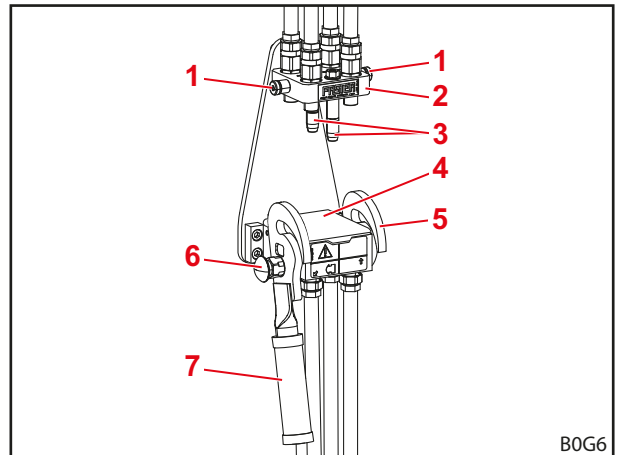
Obr. 54 Odpojená spojka Hydro-Fix
