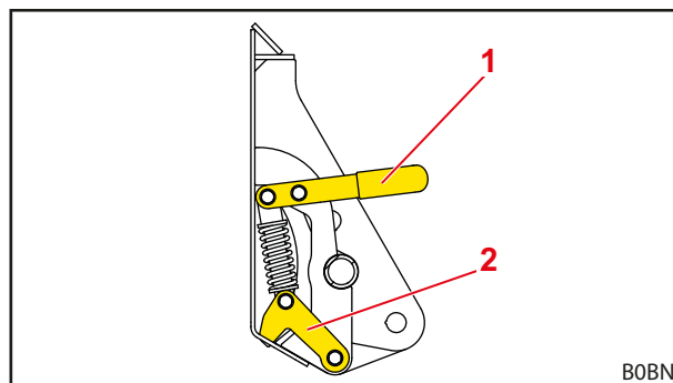
Obr. 58 Mechanický zamykací mechanismus nářadí Skid-Steer (otevřený stav)
