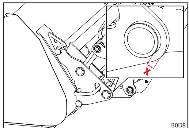
Obr. 100 Míra opotřebení výměnného rámu
