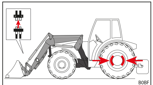
Obr. 84 Uvolnění hydraulických vedení
