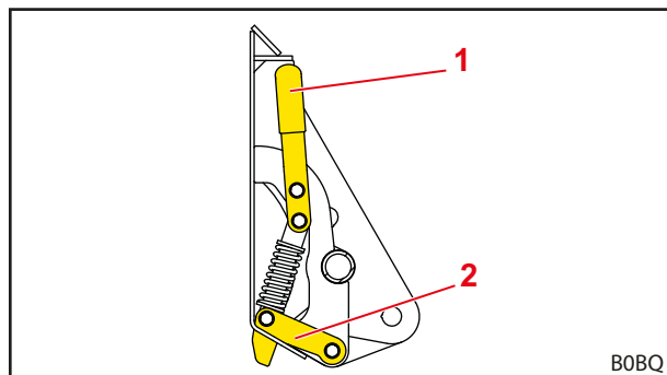
Obr. 60 Mechanický zamykací mechanismus nářadí Skid-Steer (zamknutý stav)
