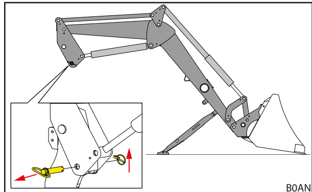
Obr. 37 Otevření uzamykacího mechanismu čelního nakladače
