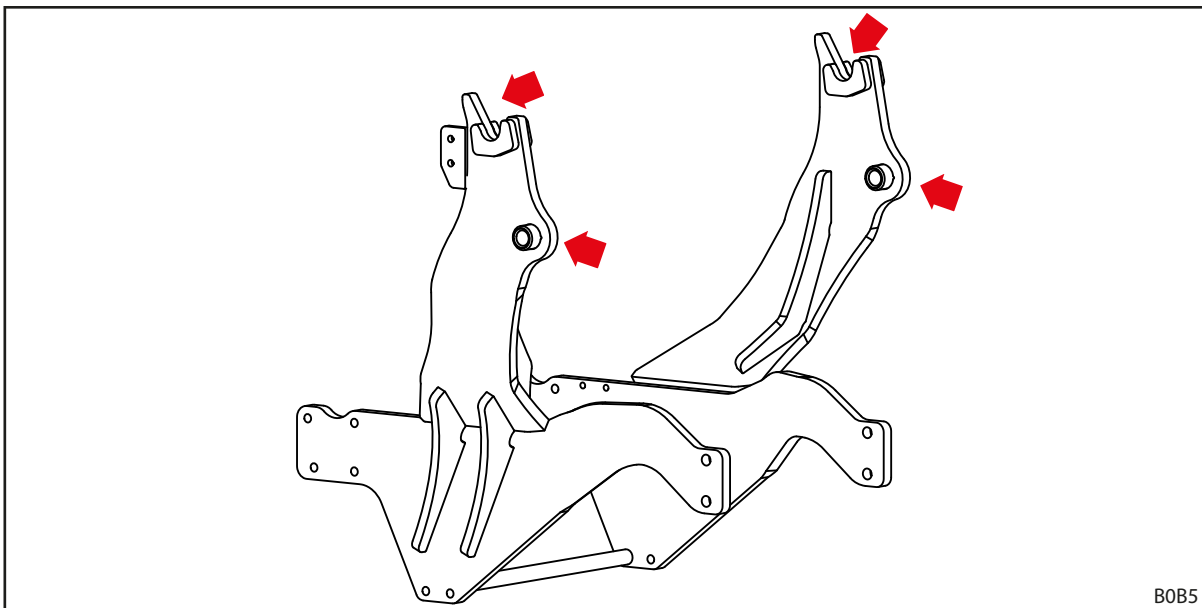
Obr. 96 Mazací místa úchytů čelního nakladače
