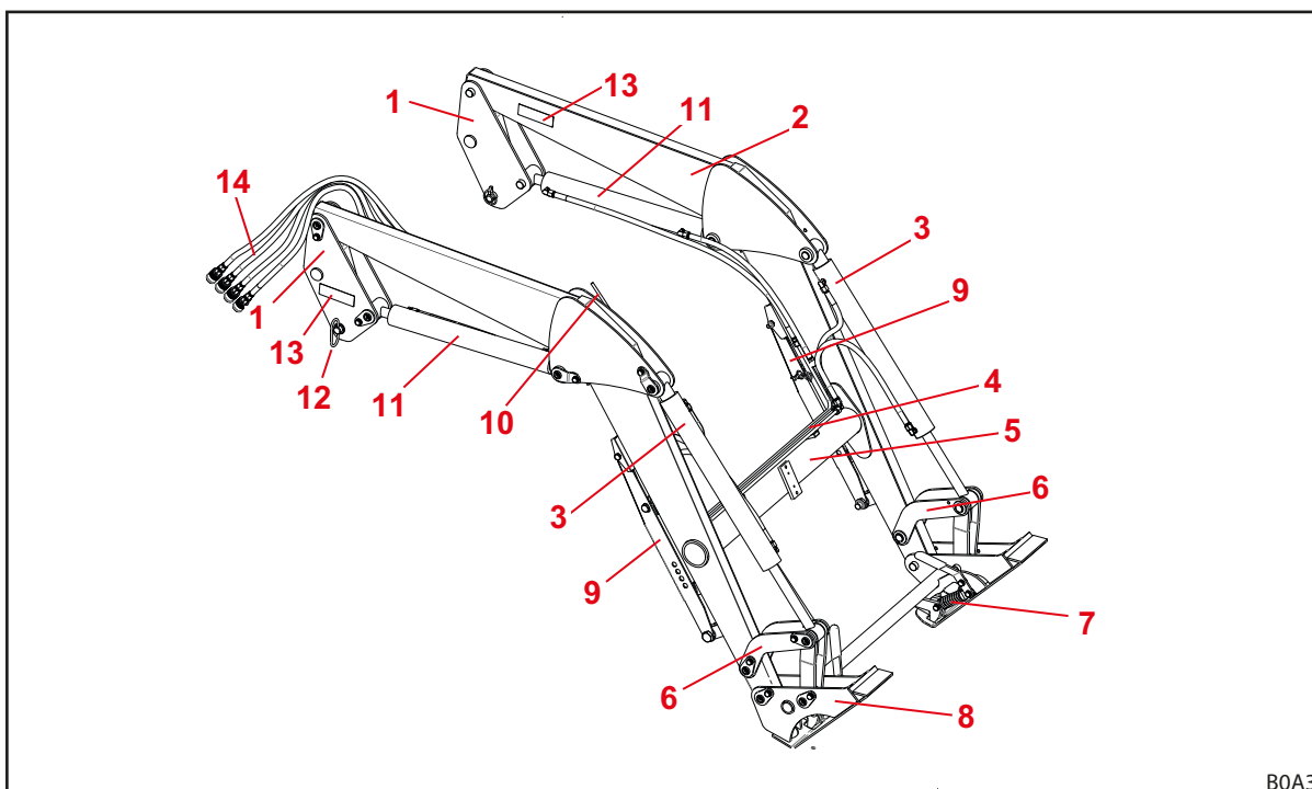
Obr. 7 Čelní nakladač H (ilustrační obrázek)
