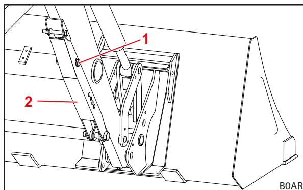
Obr. 51 Odstavná podpěra složená
