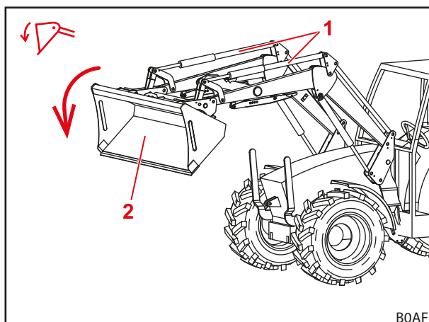
Obr. 26 Funkce vyklápění
